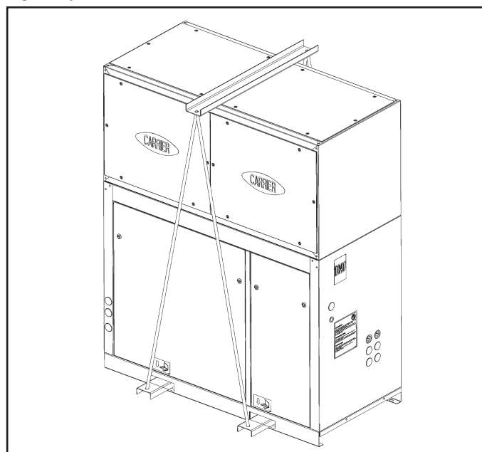
Fig. 2 - Içamento 38ES
