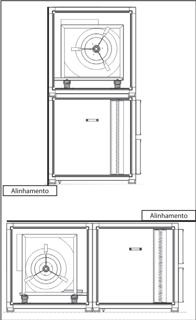
Fig. 16 - Posicionamento dos módulos
