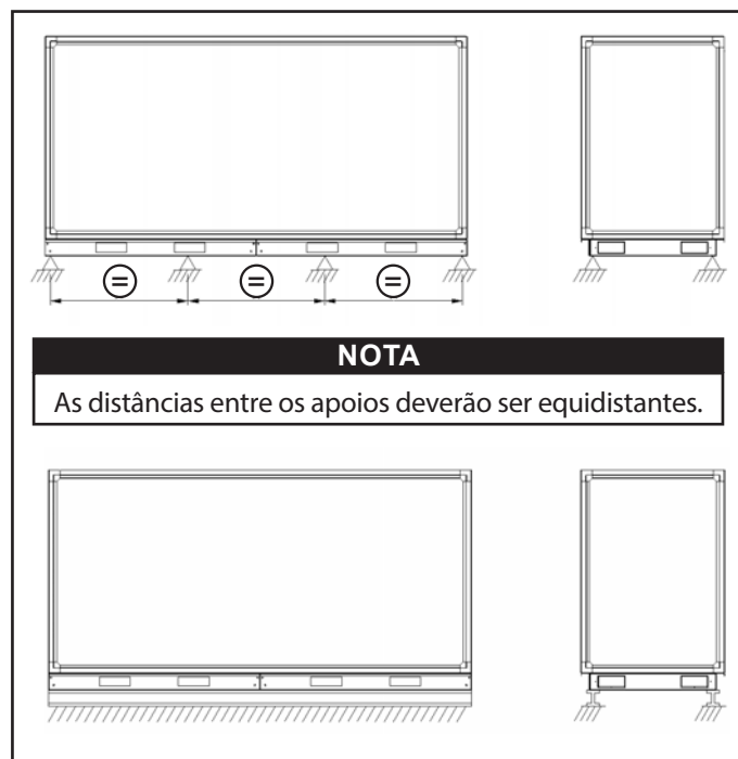
Fig. 10 - Instalação típica - Unidades com base metálica
