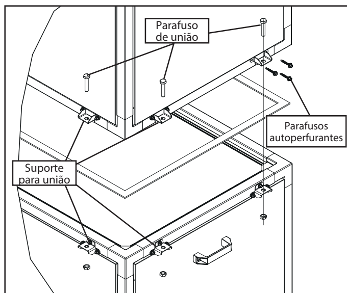
Fig. 17a - Vista explodida união dos módulos
