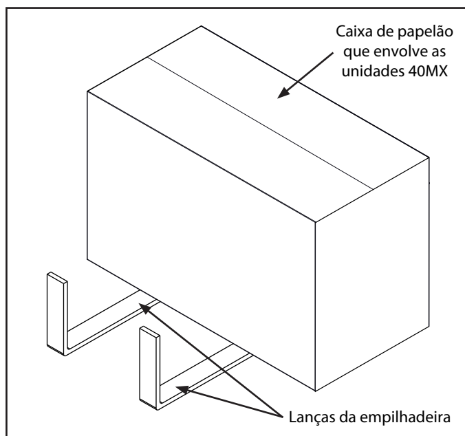
Fig. 6 - içamento 40MX
