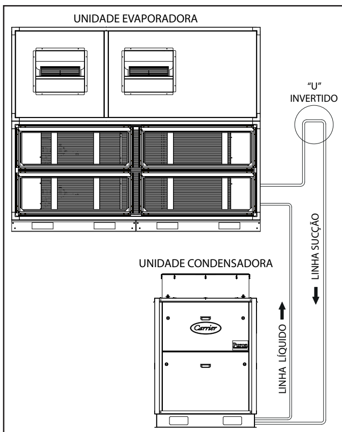
Figura 18a - Tubulações de refrigerante quando evaporadora está acima da condensadora
