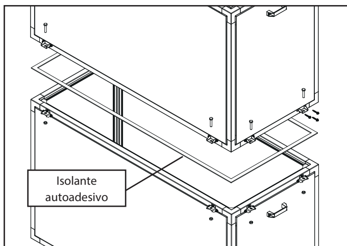
Fig. 17b - Aplicação do isolante autoadesivo
