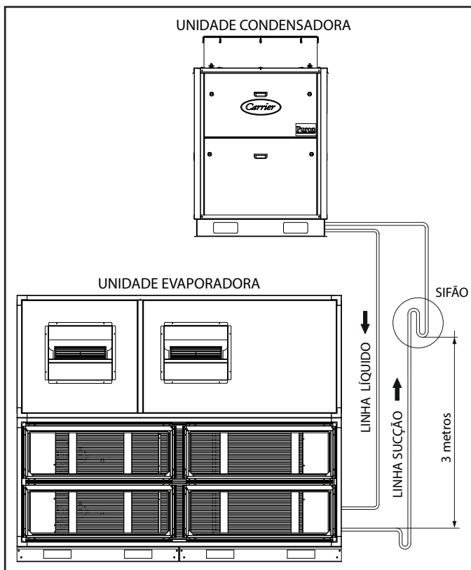
Figura 18b - Tubulações de refrigerante quando condensadora está acima da evaporadora.
