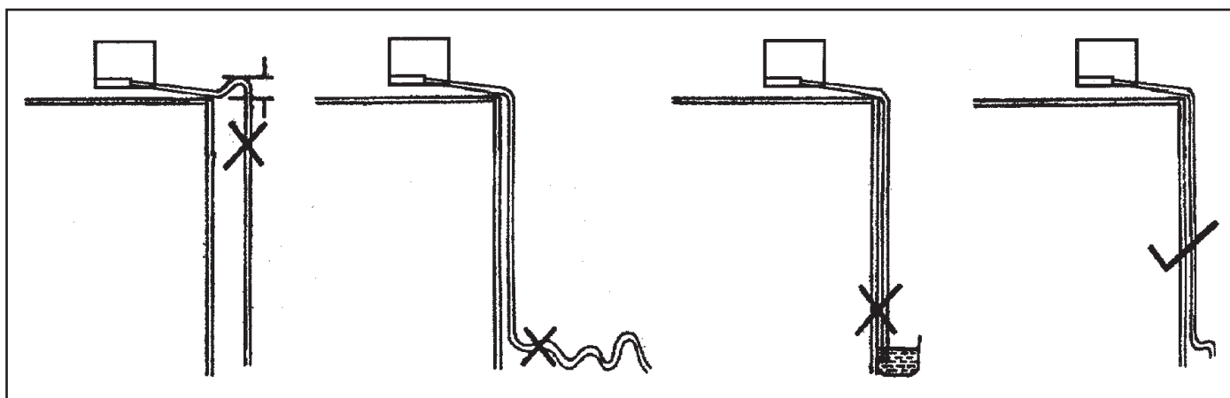
FIG. 4 - SITUAÇÃO INEFICAZ DE SUA TUBULAÇÃO DE DRENAGEM
