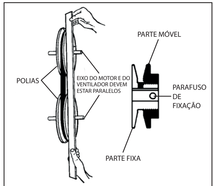
Fig. 4 - Ajuste das polias.
