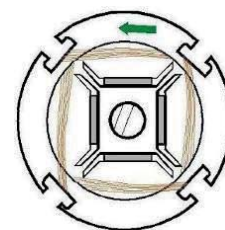
Enrolamento distribuído
