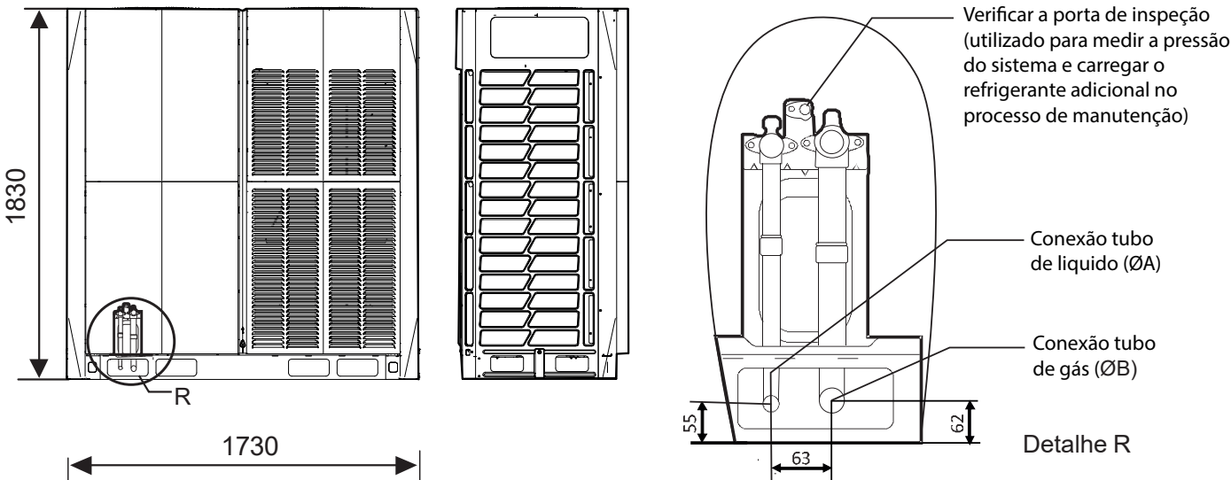
Figura 2-2.4: Dimensões 24/26/28/30/32HP (dimensões em mm)
