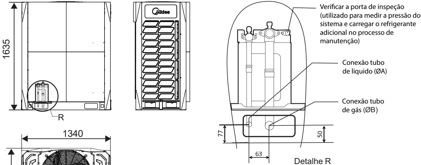
Figura 2-2.2: Dimensões 14/16HP (dimensões em mm)
