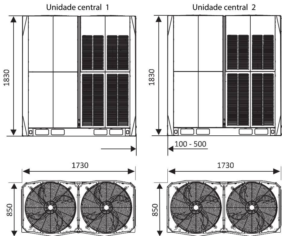
Figura 2-2.10: Dimensões das unidades 52/54/56/58/60/62/64HP (dimensões em mm)
