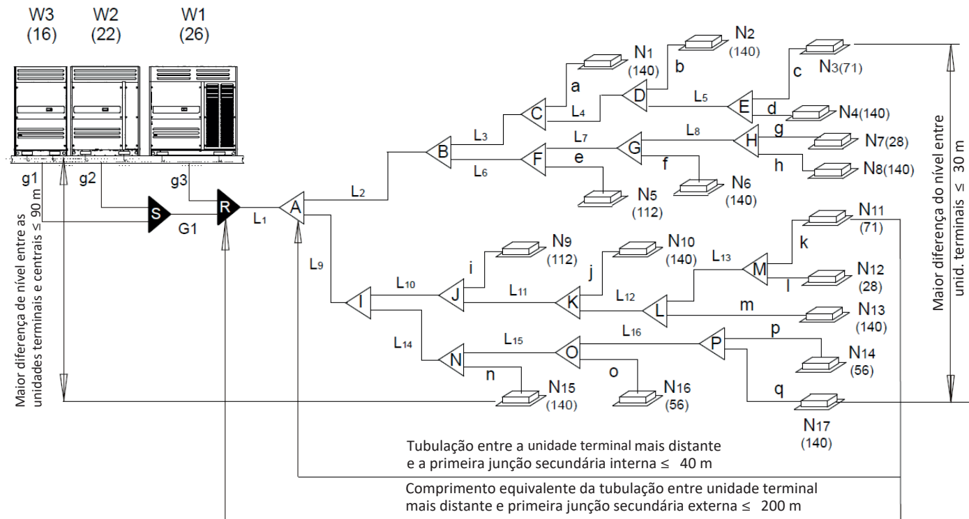
Figura 3-4.2: Comprimentos de tubulação do refrigerante e desníveis permitidos
