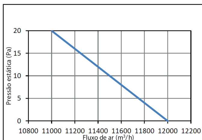
Figura 3-3.10: Desempenho do ventilador em unidades de 18 HP
