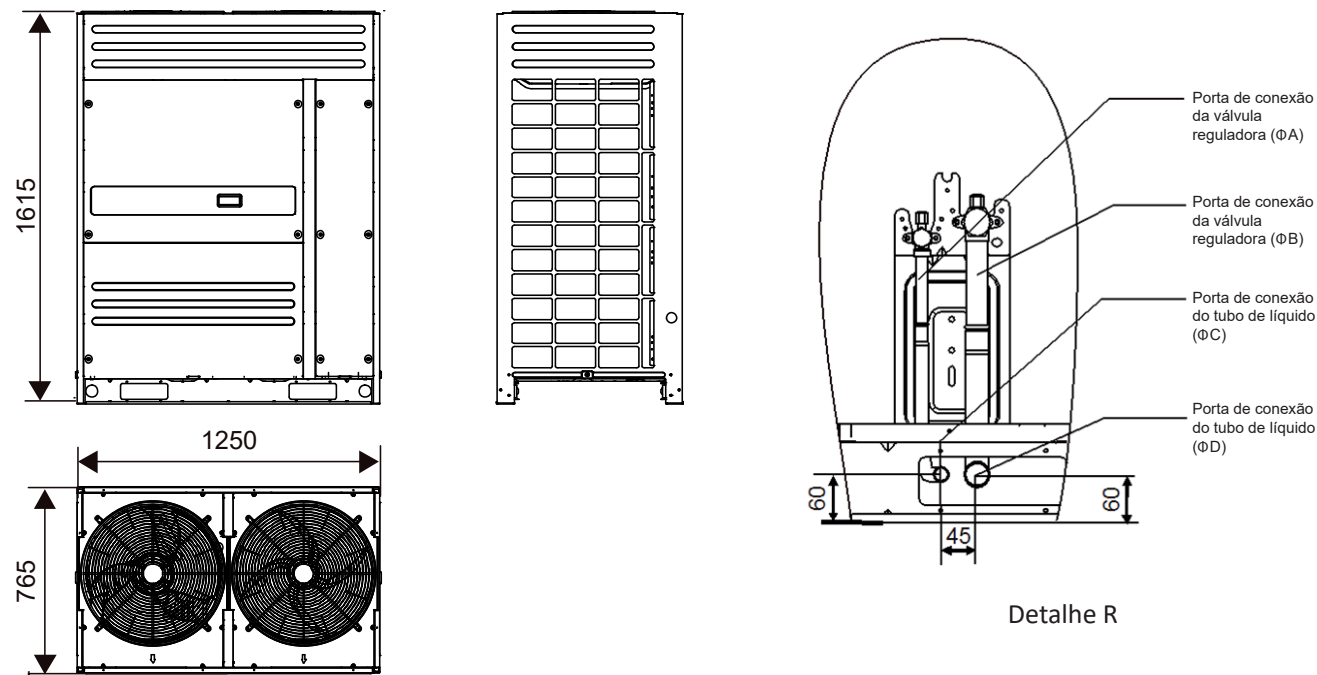
Figura 2-2.5: Dimensões de 18/20/22 HP (unidade: mm)
