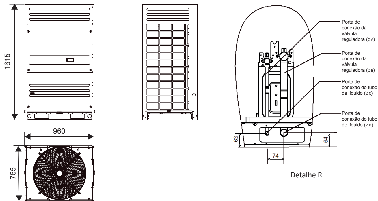
Figura 2-2.4: Dimensões de 8/10/12/14/16 HP (unidade: mm)
