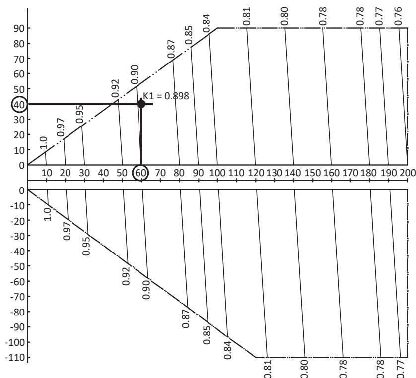
Figura 1-6.3: Taxa de alteração de VC na capacidade de refrigeração
