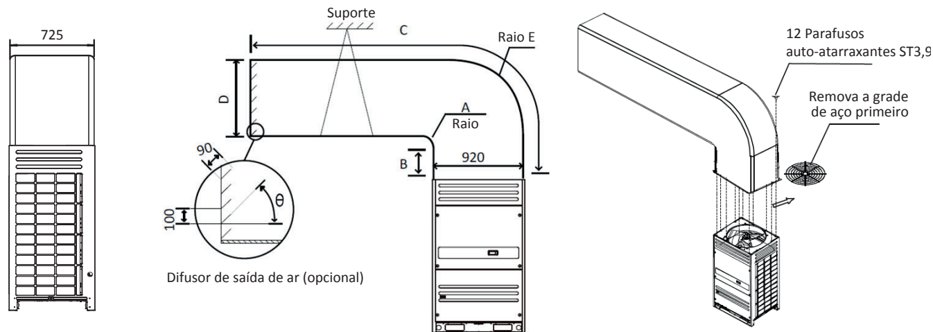
Figura 3-3.3: Dutos longitudinais para unidades de 8-16 HP (unidade: mm)
