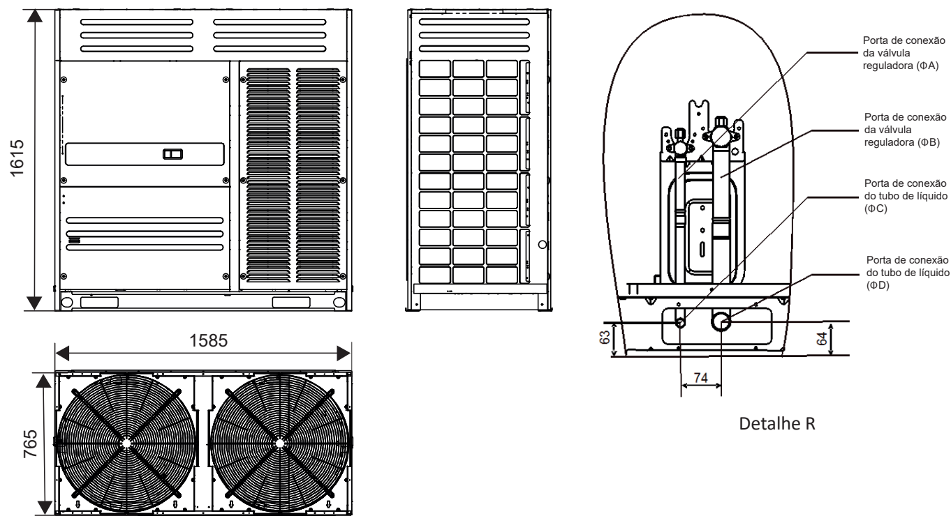
Figura 2-2.6: Dimensões de 24/26/28/30 HP (unidade: mm)
