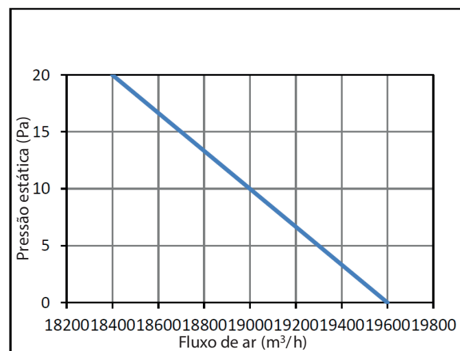
Figura 3-3.12: Desempenho do ventilador em unidades de 24-26 HP
