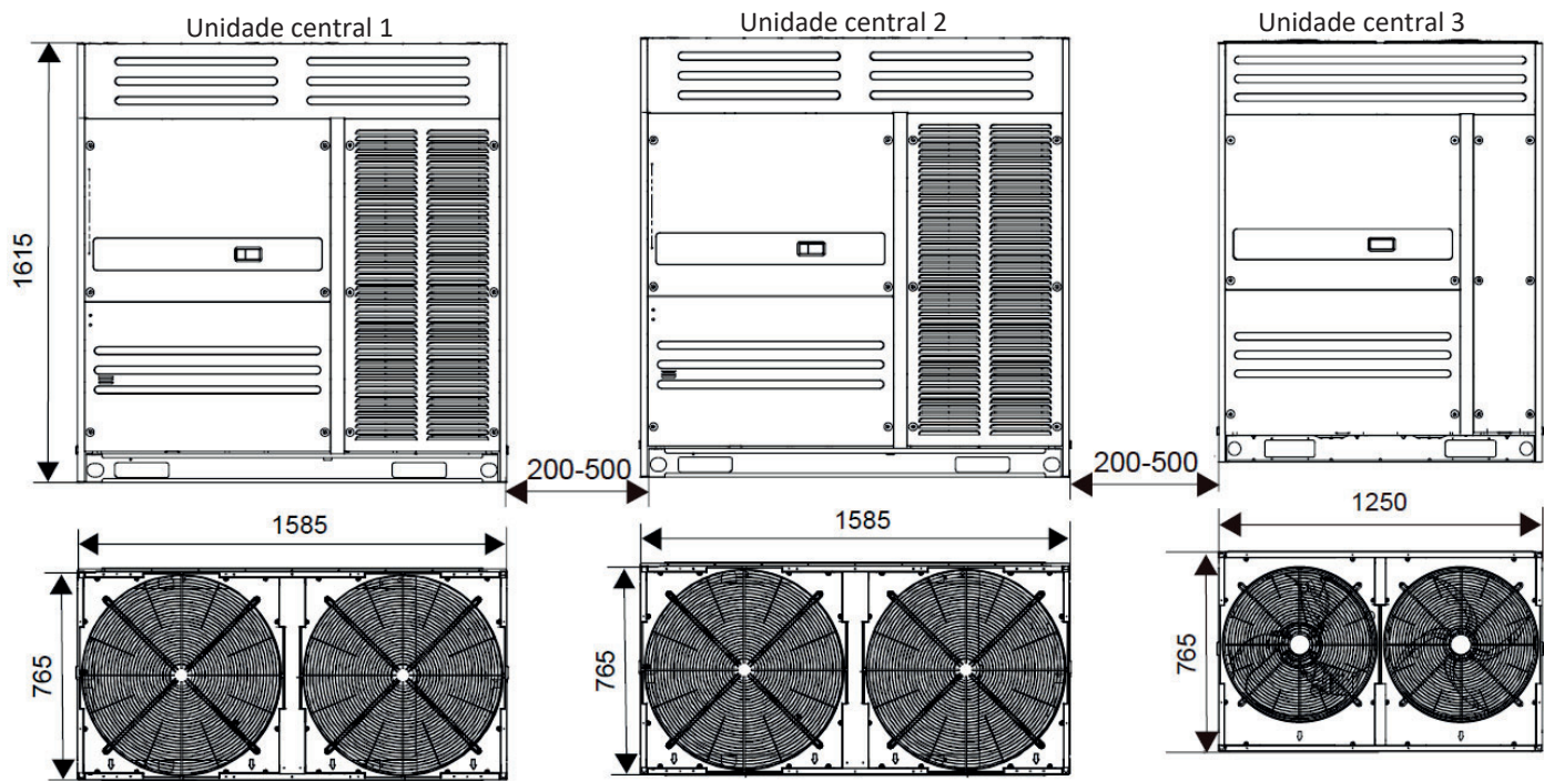
Figura 2-2.15: Dimensões de 78/80/82 HP (unidade: mm)
