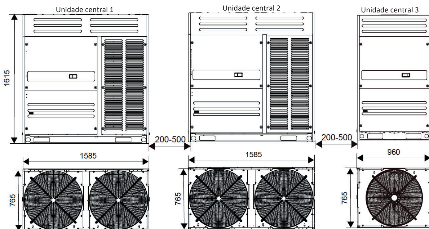
Figura 2-2.14: Dimensões de 70/72/74/76 HP (unidade: mm)
