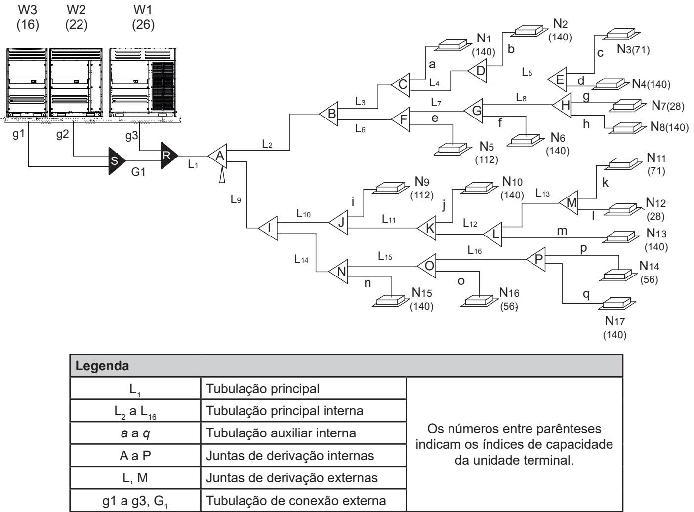
Figura 3-4.4: Exemplo de seleção de tubulação de refrigerante
