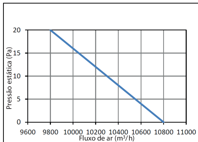
Figura 3-3.8: Desempenho do ventilador em unidades de 12 HP
