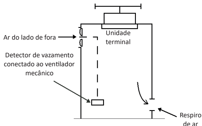
Figura 3-4.7: Ventilador mecânico controlado por detector de vazamento de refrigerante
