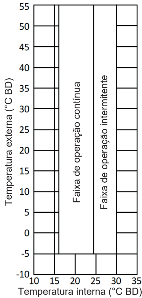
Figura 2-9.1: Limites operacionais de refrigeração
