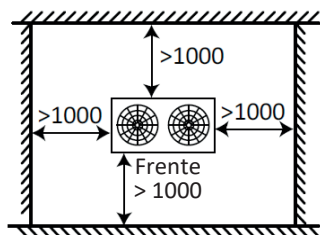
Figura 3-2.1: Instalação da unidade individual (unidade: mm)
