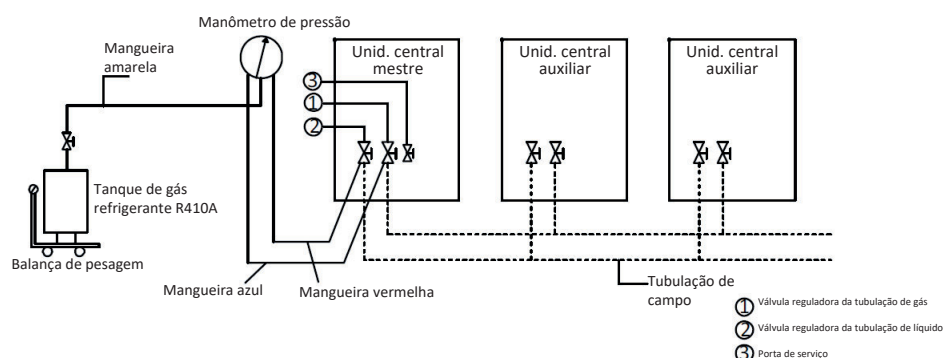
Figura 3-8.1: Carregamento do refrigerante
