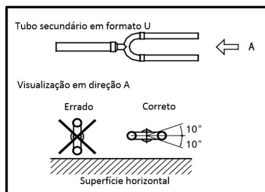
Figura 3-5.8: Orientação da junta de derivação
