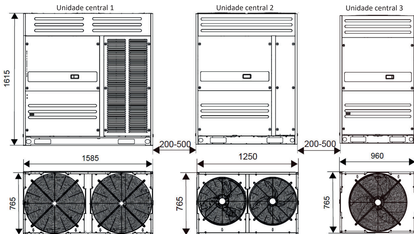
Figura 2-2.13: Dimensões de 64/66/68 HP (unidade: mm)
