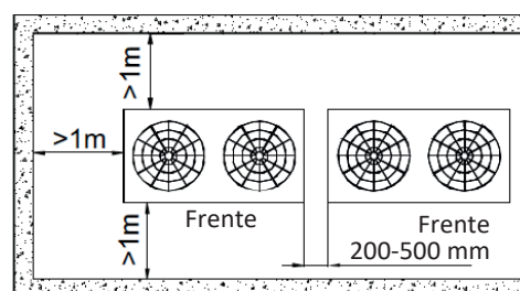
Figura 2-3.2: Instalação em fila única (unidade: mm)
