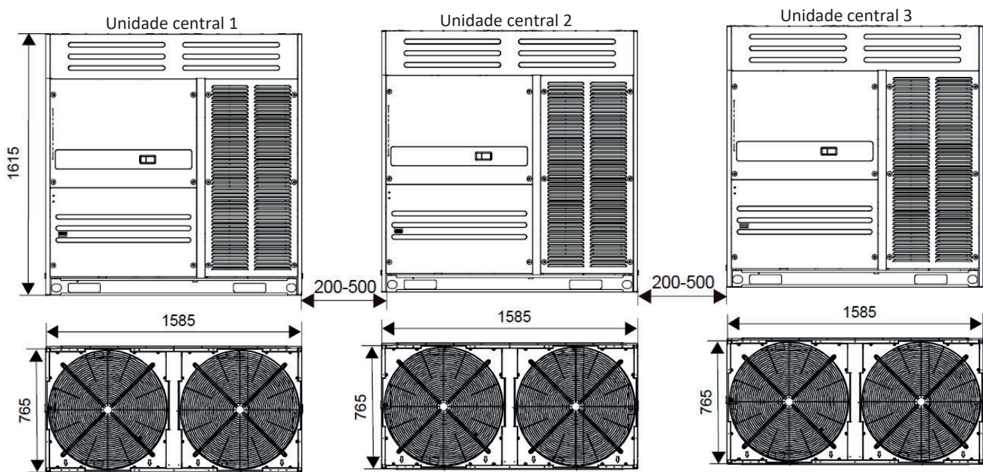
Figura 2-2.16: Dimensões de 84/86/88/90 HP (unidade: mm)
