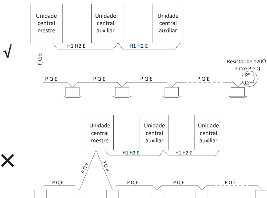
Figura 3-9.5: Configurações da fiação de comunicação - exemplos corretos e incorretos (continua na próxima página)
