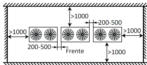
Figura 3-2.2: Instalação em fila única (unidade: mm)
