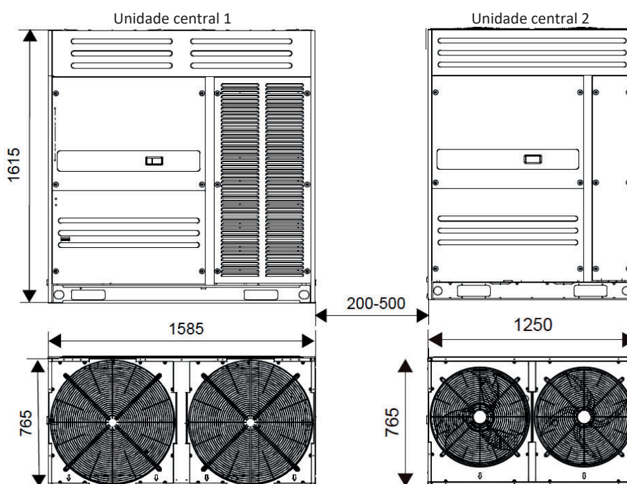
Figura 2-2.10: Dimensões de 48/50/52 HP (unidade: mm)
