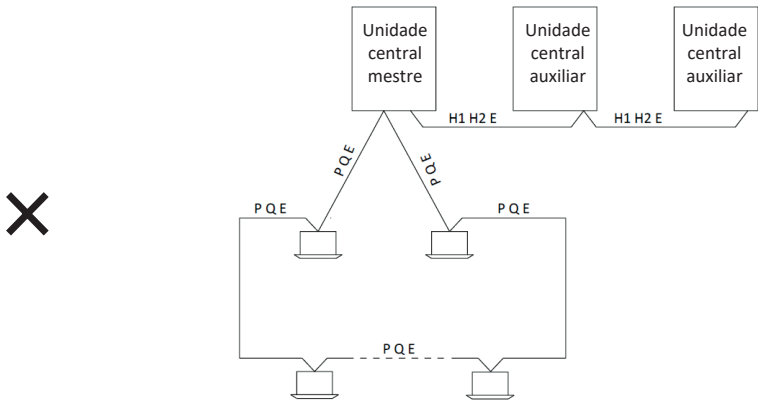
Figura 3-9.5: Configurações da fiação de comunicação - exemplos corretos e incorretos (continuação)
