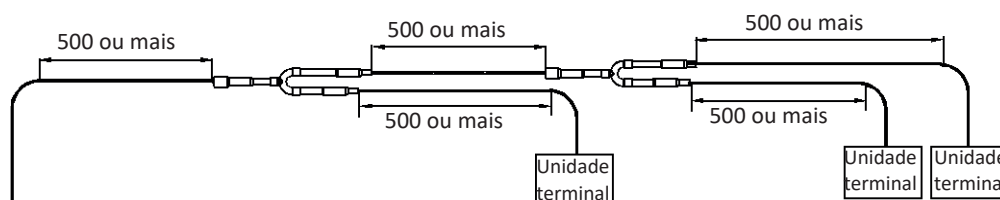
Figura 3-4.5: Espaçamento e separação entre junta de derivação e curvas (unidade: mm)
