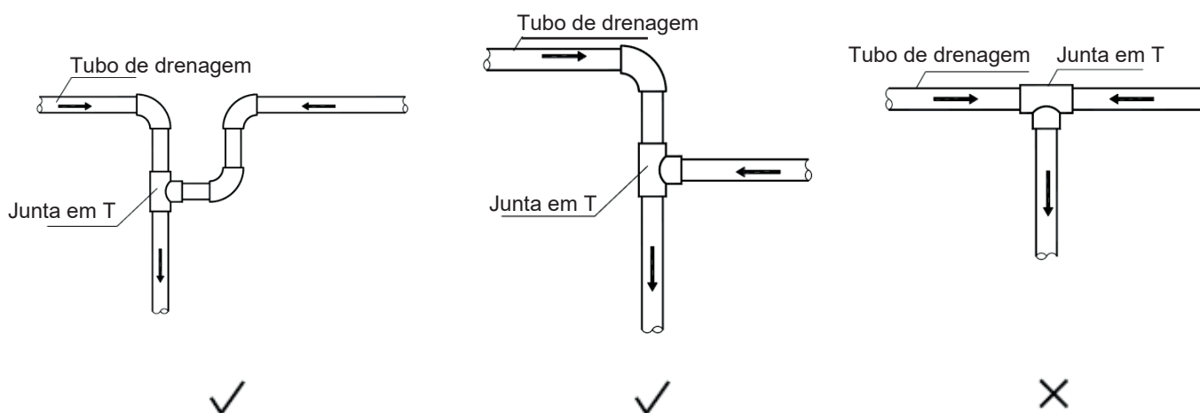
Figura 3-6.2: Junções da tubulação de drenagem - configurações corretas e incorretas
