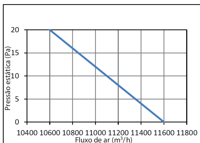
Figura 3-3.9: Desempenho do ventilador de unidades de 14-16 HP
