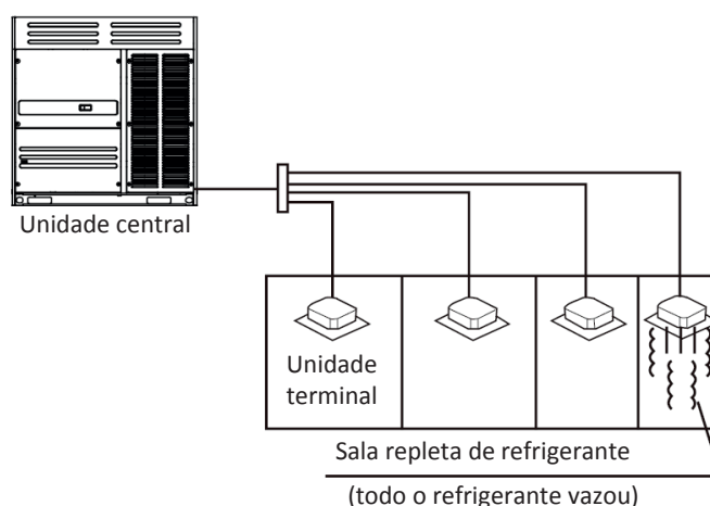
Figura 3-4.6: Cenário de vazamento de refrigerante em potencial
