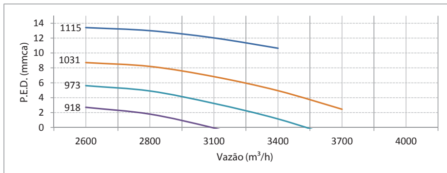
Módulo 40MV_175VH (G4 + M5)
