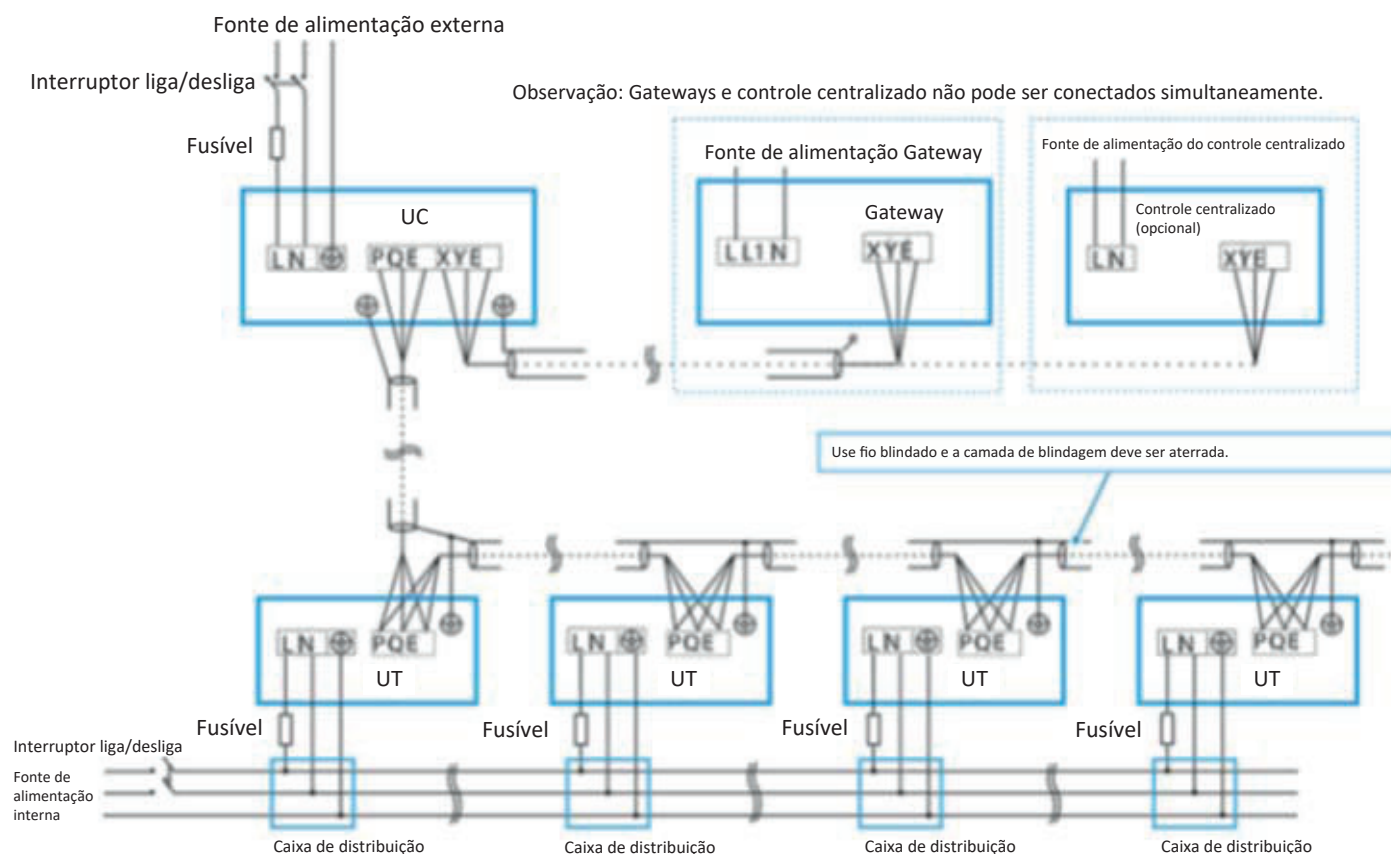
Figura 3-8.4: Exemplo de fiação do sistema de energia
