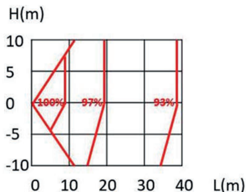
Figura 2-7.3: Taxa de alteração de modelo 100-120 na capacidade de refrigeração
