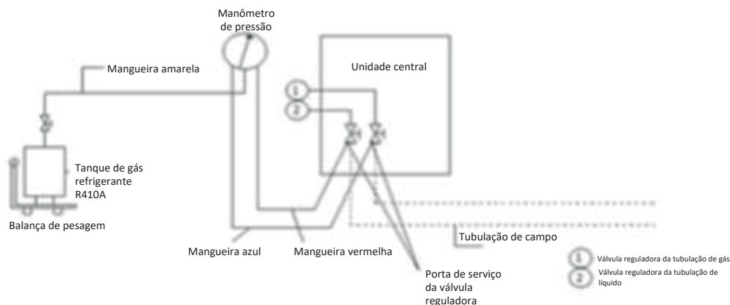
Figura 3-7.1: Carregamento do refrigerante
