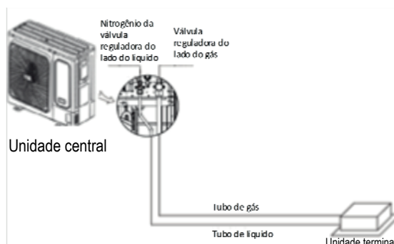
Figura 3-4.11: Teste de estanqueidade de gás
