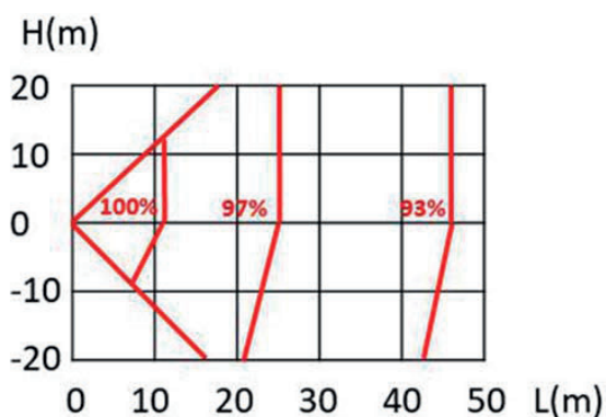
Figura 2-7.5: Taxa de alteração de modelo 140-160 na capacidade de refrigeração
