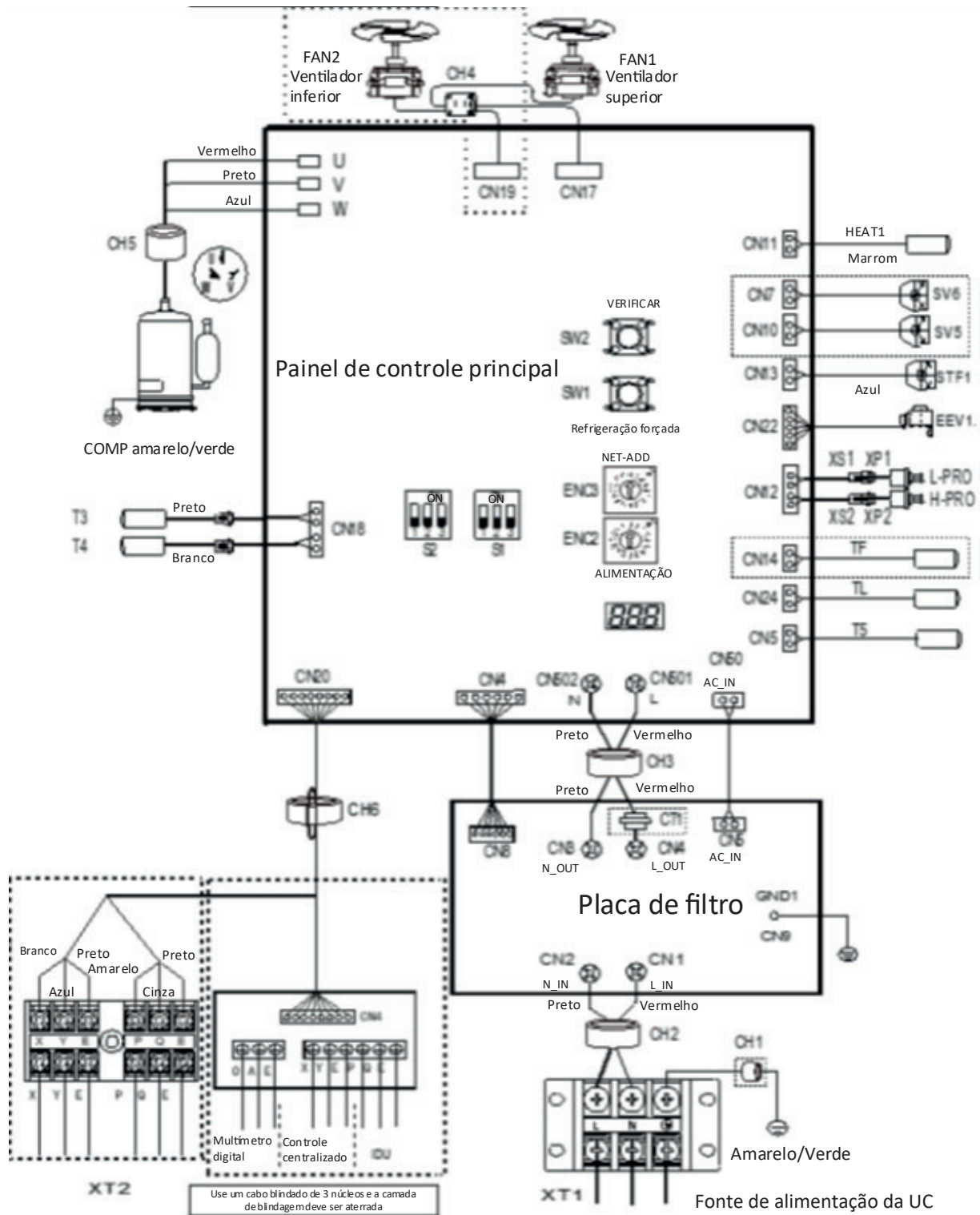
Figura 2-5.3: Diagrama da fiação modelo 140/160
