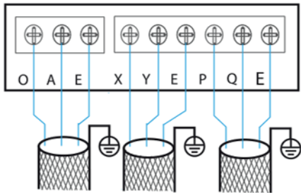
Figura 3-8.3: Terminais de comunicação da unidade central
