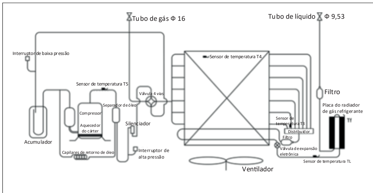
Figura 2-4.3: Diagrama da tubulação 140/160
