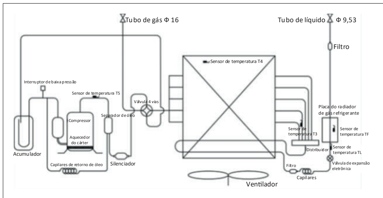
Figura 2-4.1: Diagramas da tubulação 80
