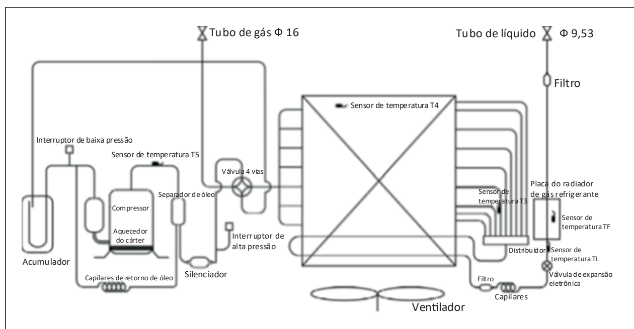
Figura 2-4.2: Diagrama da tubulação 100/120
