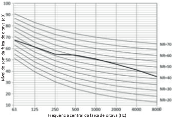
Figura 2-9.3 níveis da faixa de oitava do modelo 100
