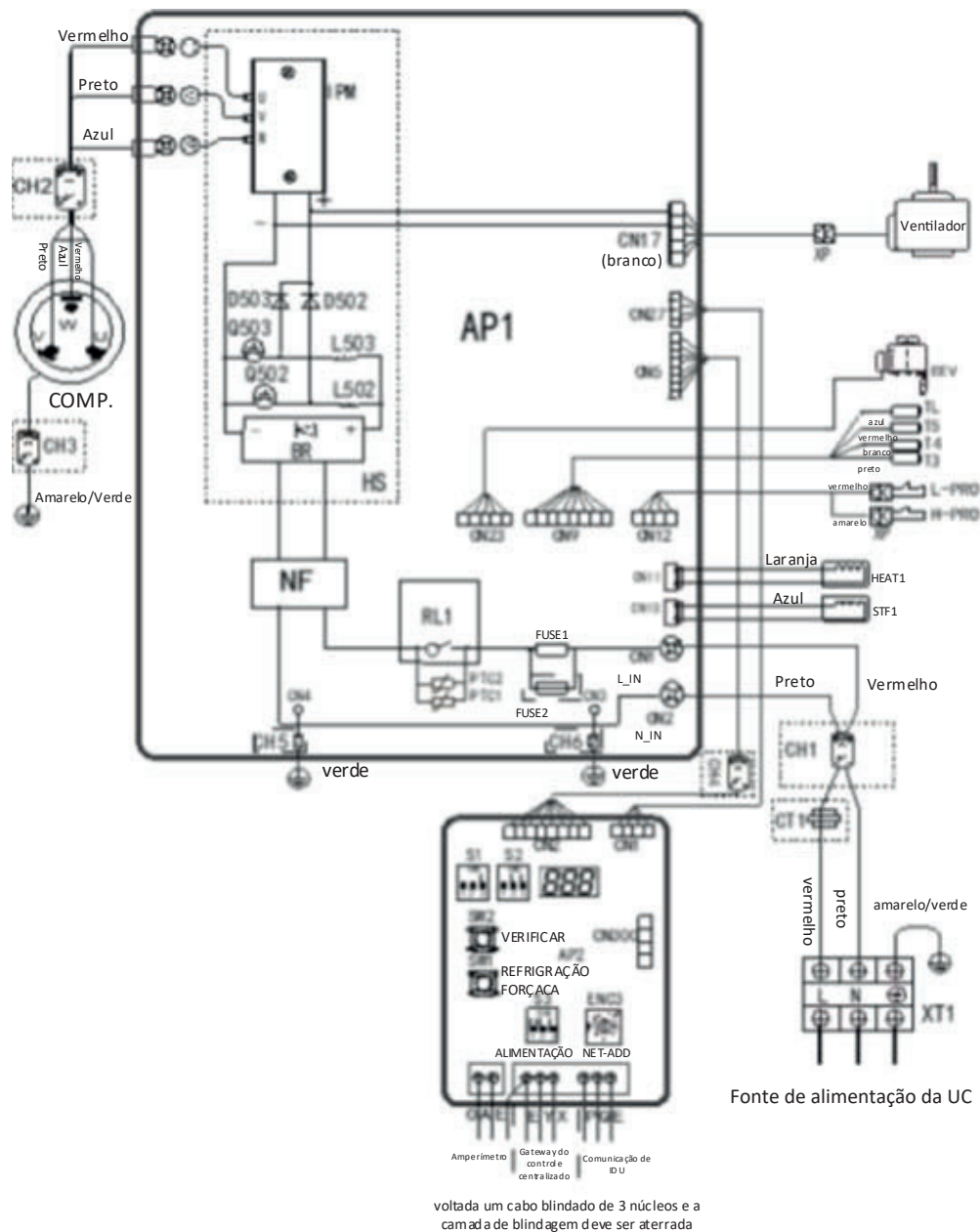
Figura 2-5.2: Diagrama da fiação modelo 100/120
