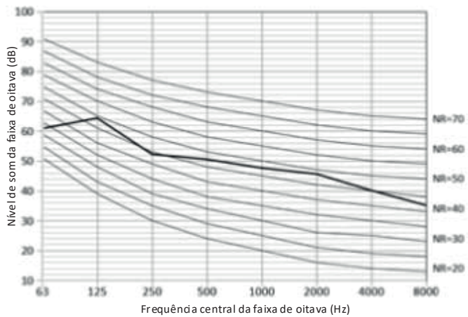
Figura 2-9.5 níveis da faixa de oitava do modelo 140
