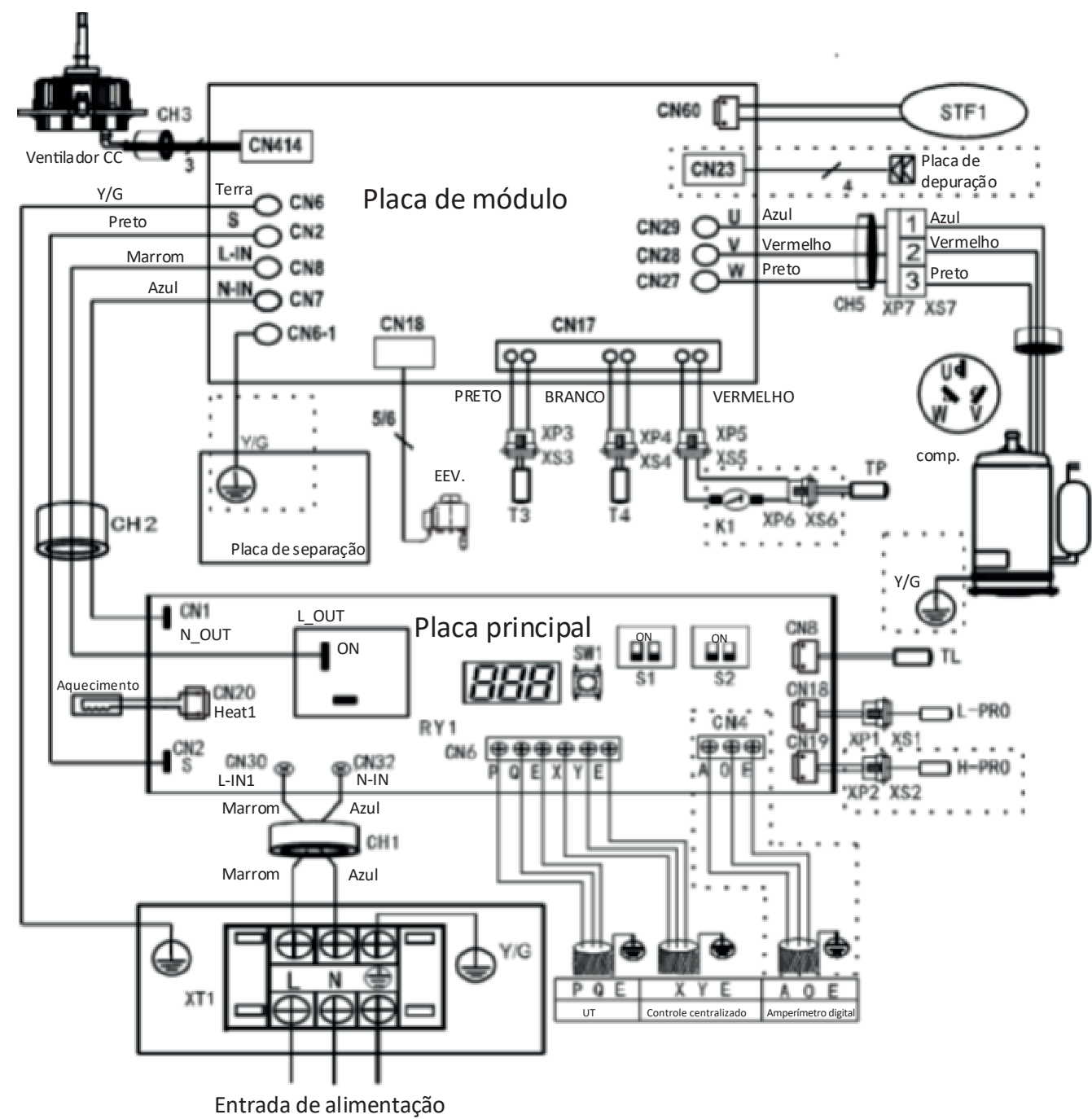
Figura 2-5.1: Diagrama da fiação modelo 80
