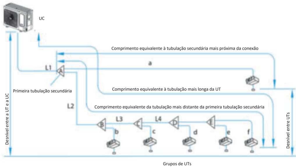
Figura 3-3.1: Primeiro método de conexão
