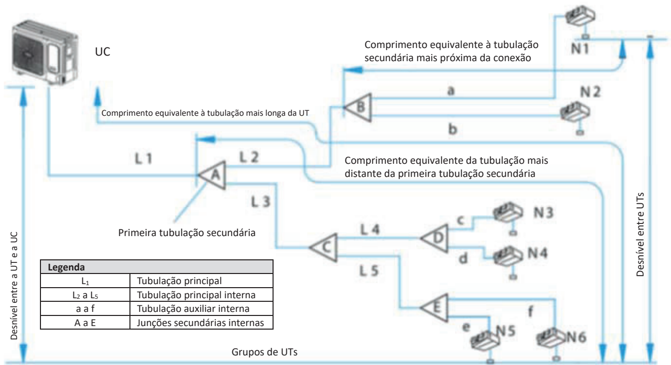
Figura 3-3.2: Segundo método de conexão
