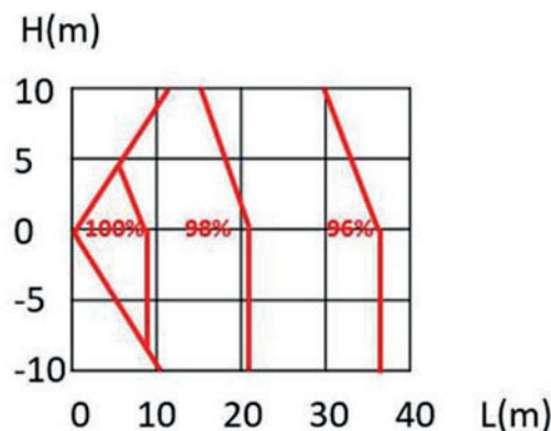
Figura 2-7.4: Taxa de alteração de modelo 100-120 na capacidade de aquecimento
