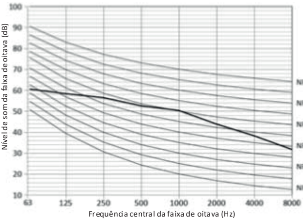
Figura 2-9.2 nível da faixa de oitava do 80
