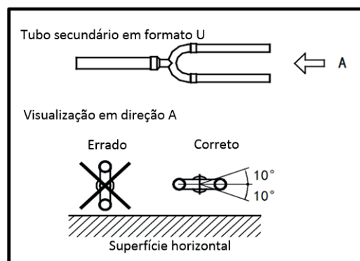
Figura 3-4.8: Orientação da junta de derivação
