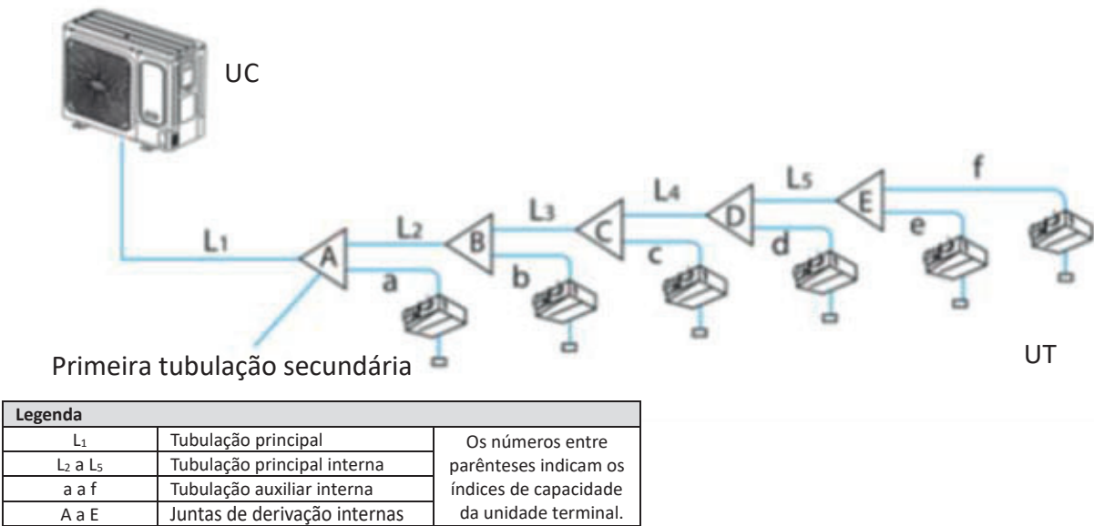
Figura 3-3.3: Seleção dos diâmetros da tubulação
