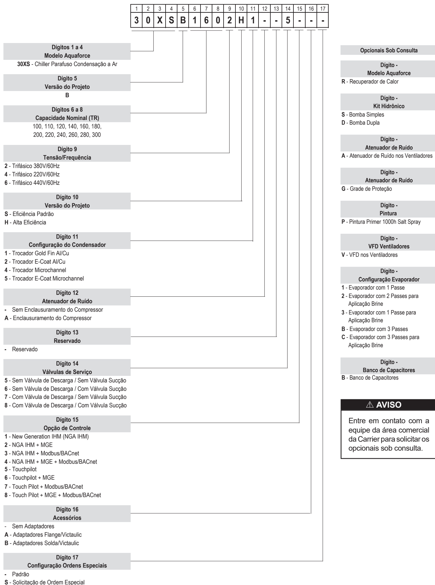
Figura 1 — Nomenclatura
