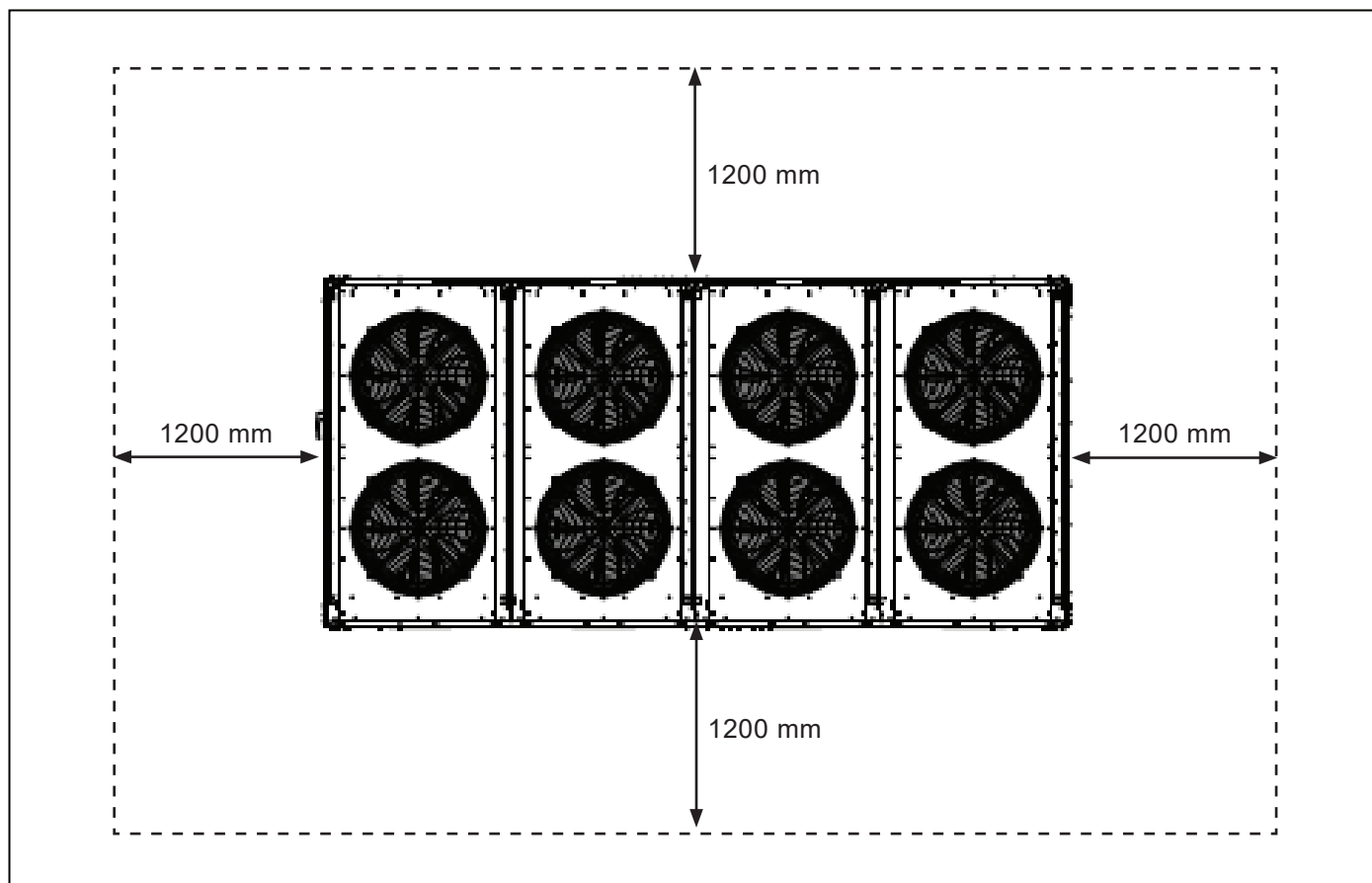
Figura 2c - Dimensional das Unidades 30RSB - Área de Serviço ao Redor da Unidade - Espaços Recomendados
