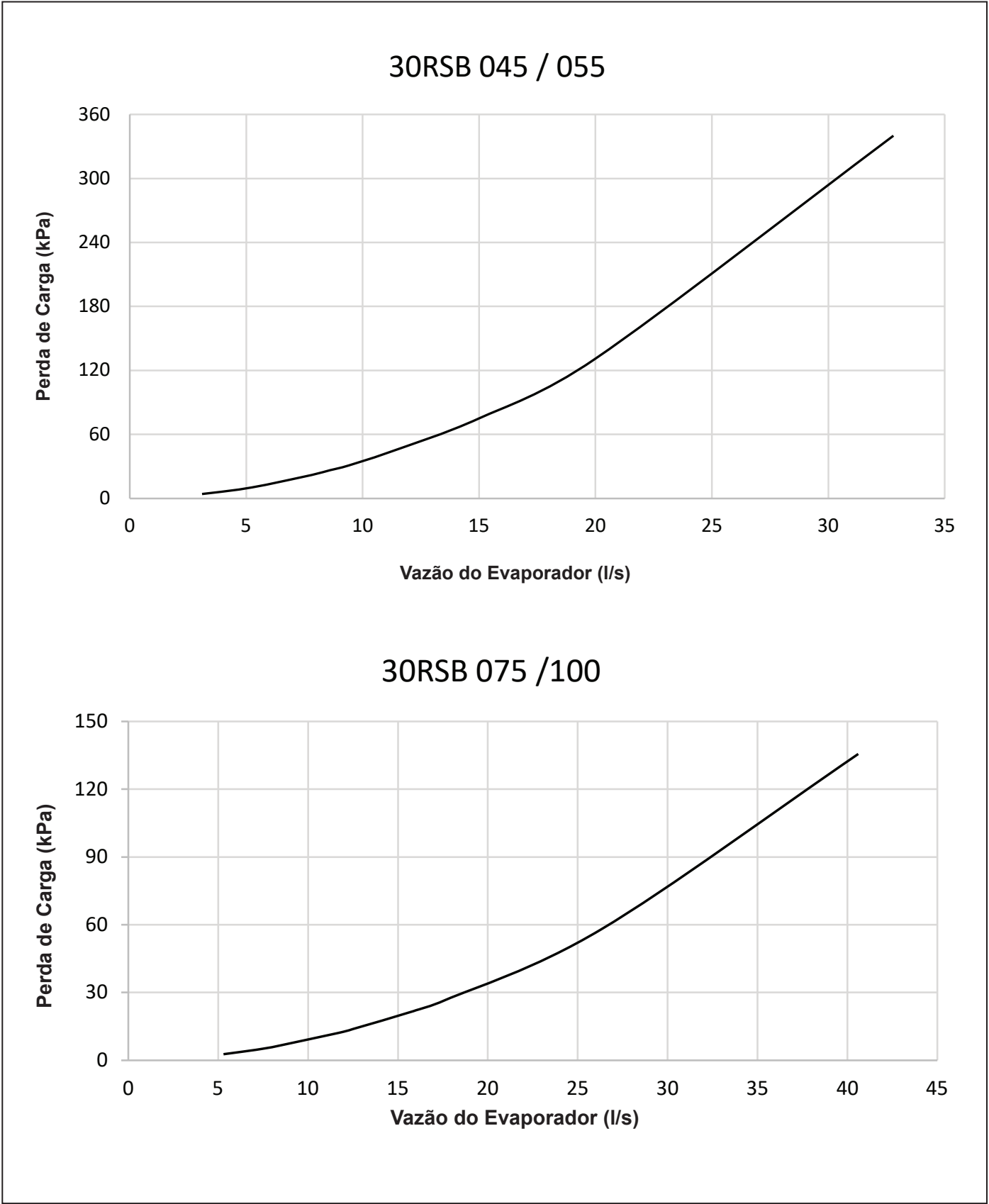
Figura16a - Gráficos Perda de Carga
