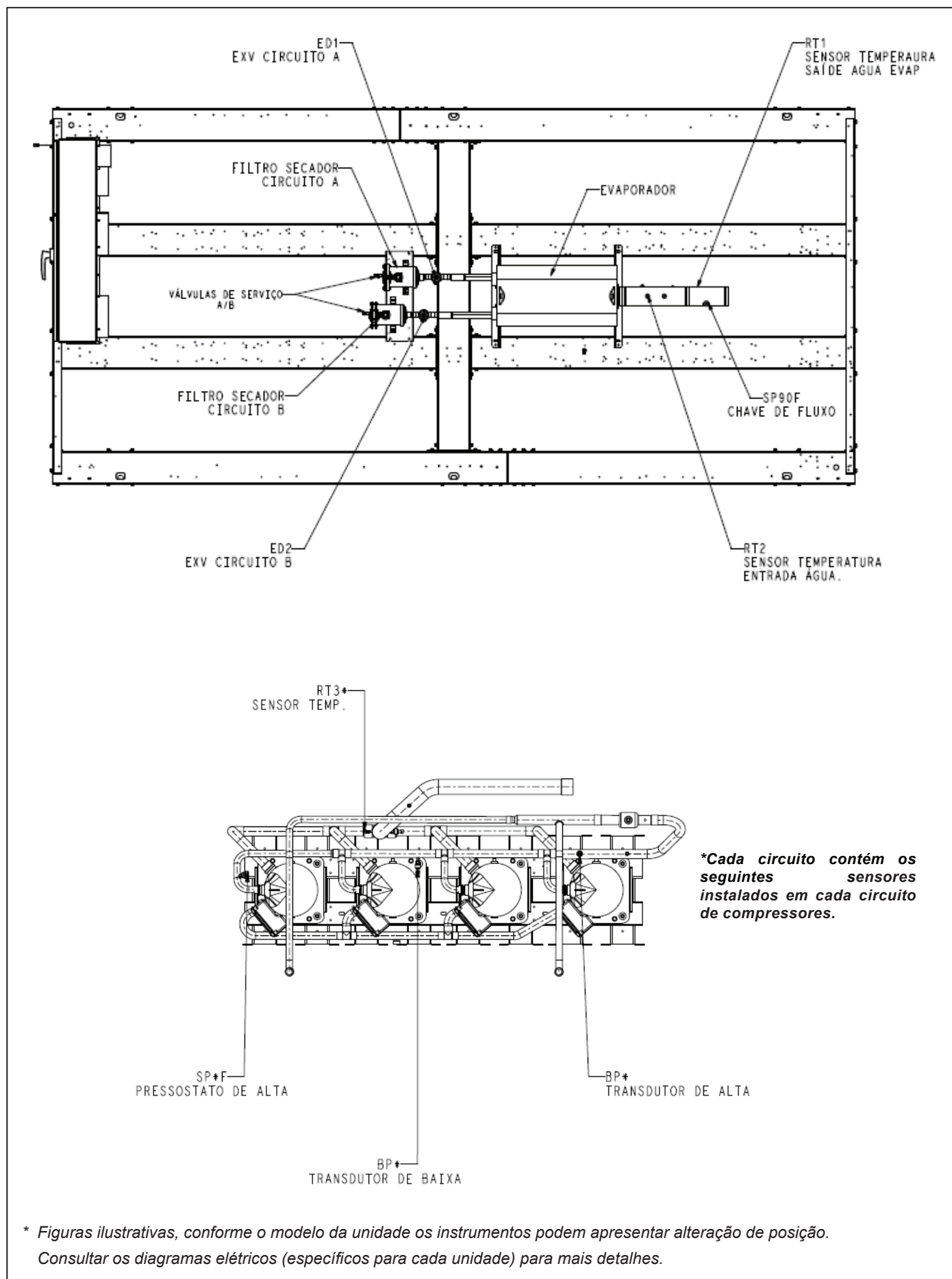
Figura 25 - Posição dos principais instrumentos do chiller
