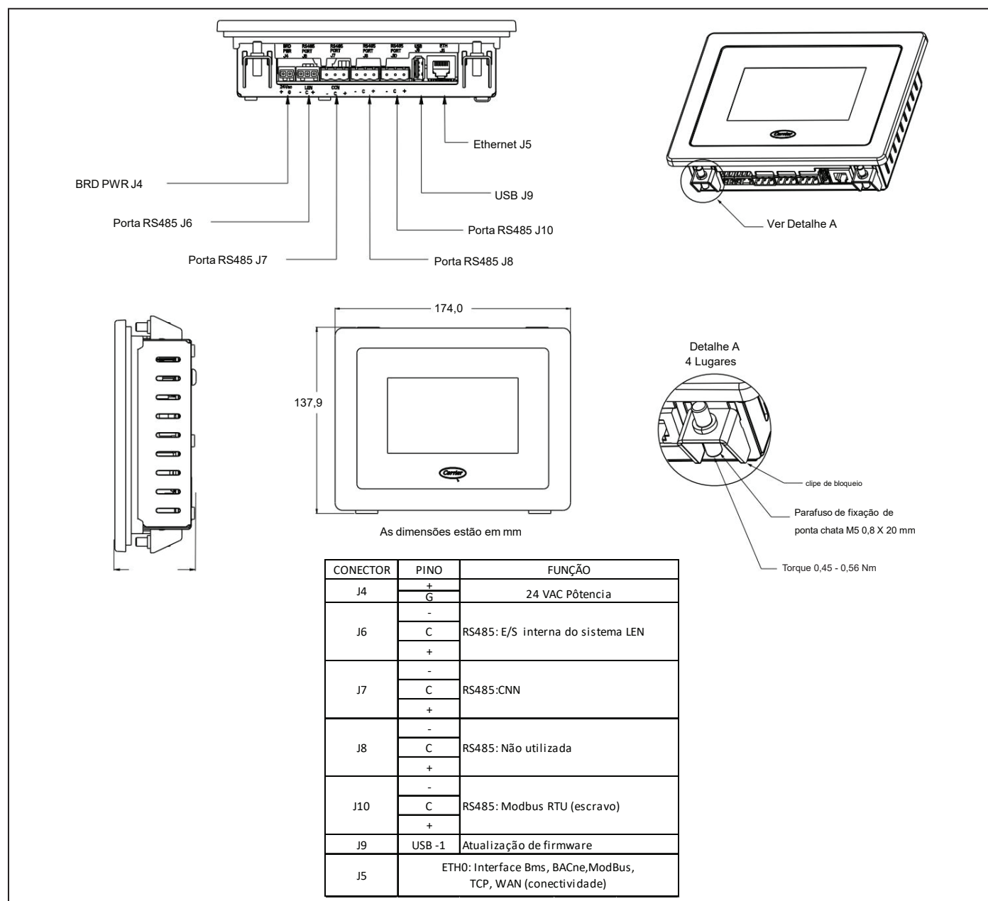
Figura 20 - Entradas IHM
