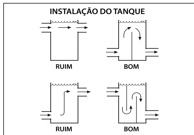
Figura 9 - Fluxo Tanque
