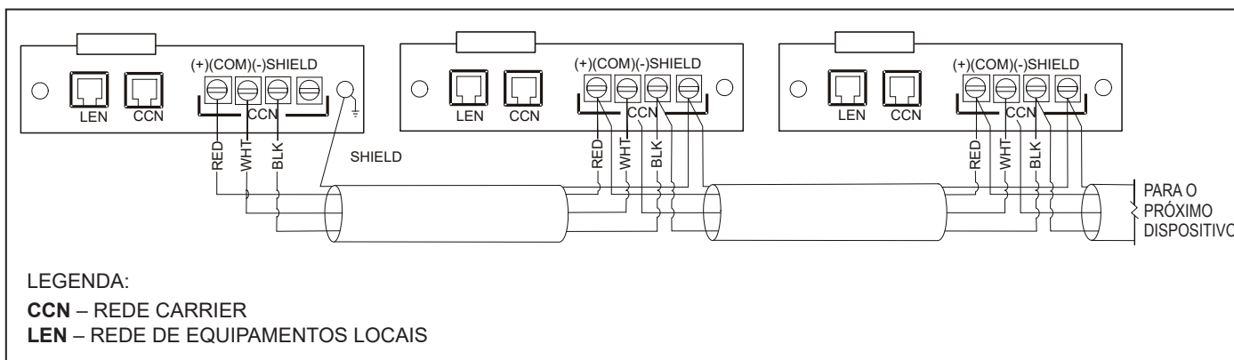
Figura 19 - Cabos para CCN
