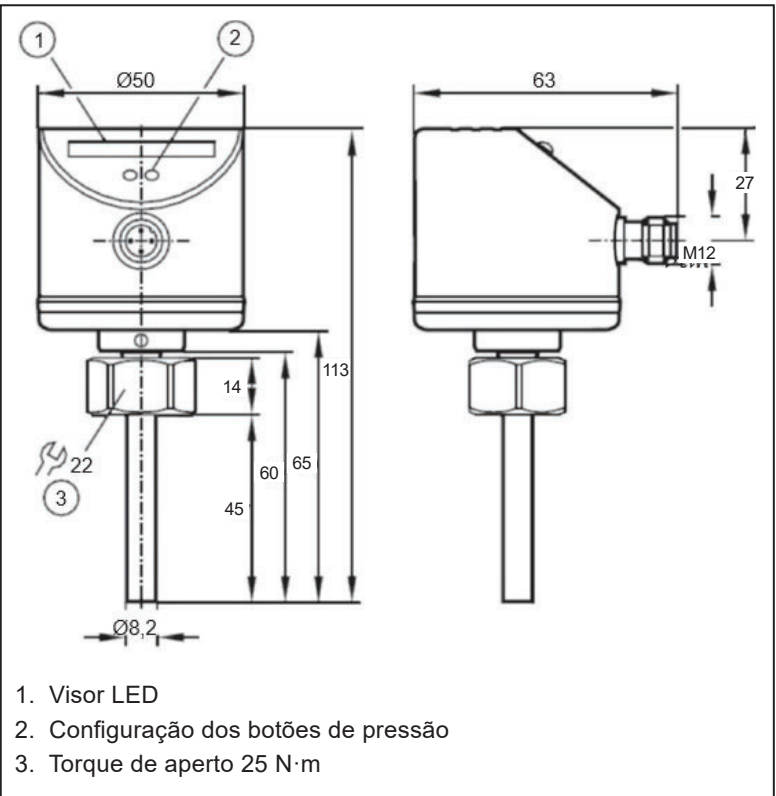
Figura 28 - Chave de fluxo
