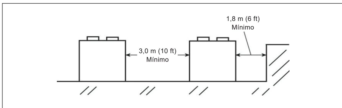
Figura 2d - Dimensional das Unidades 30RSB - Instalação de Múltiplas Unidades - Espaços Mínimos Recomendados
