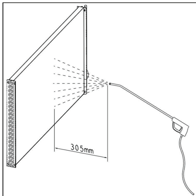
Figura 27 - Processo de limpeza serpentina
