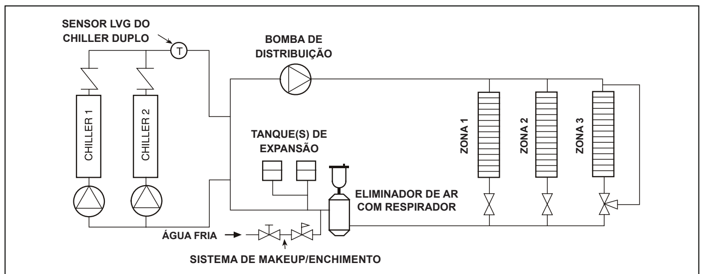
Figura 13 - Esquema chillers múltiplos com eliminador de ar
