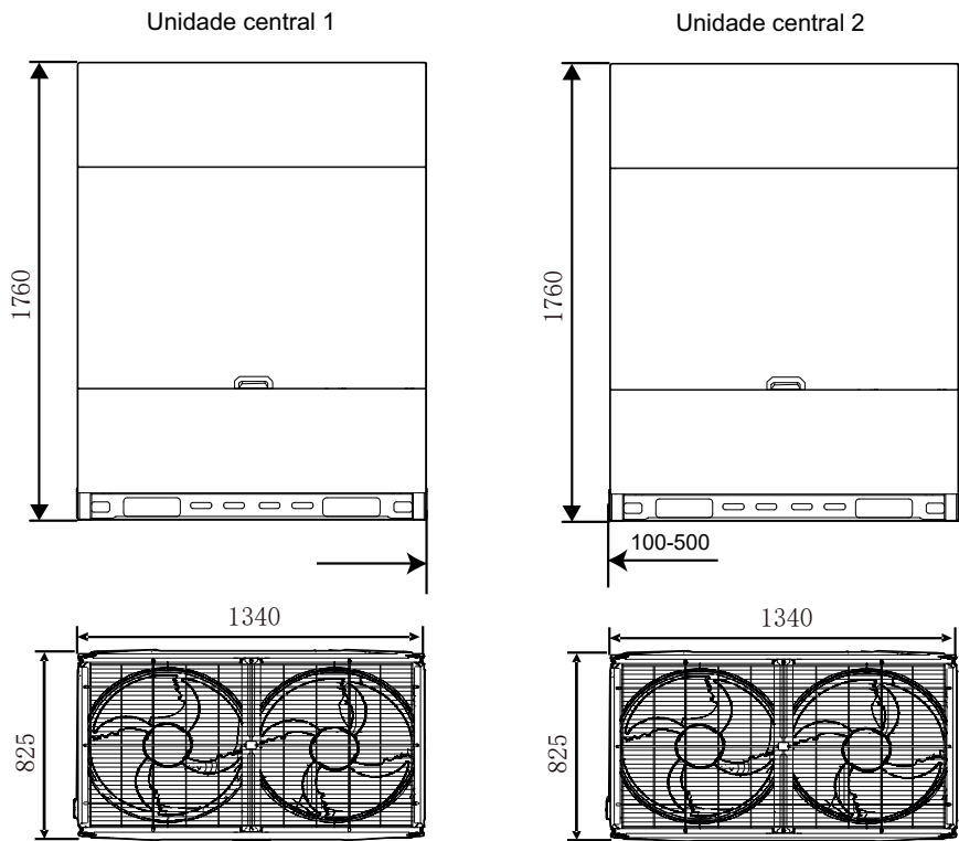
Figura 2-2.8: Dimensões das unidades 46/48HP (dimensões em mm)
