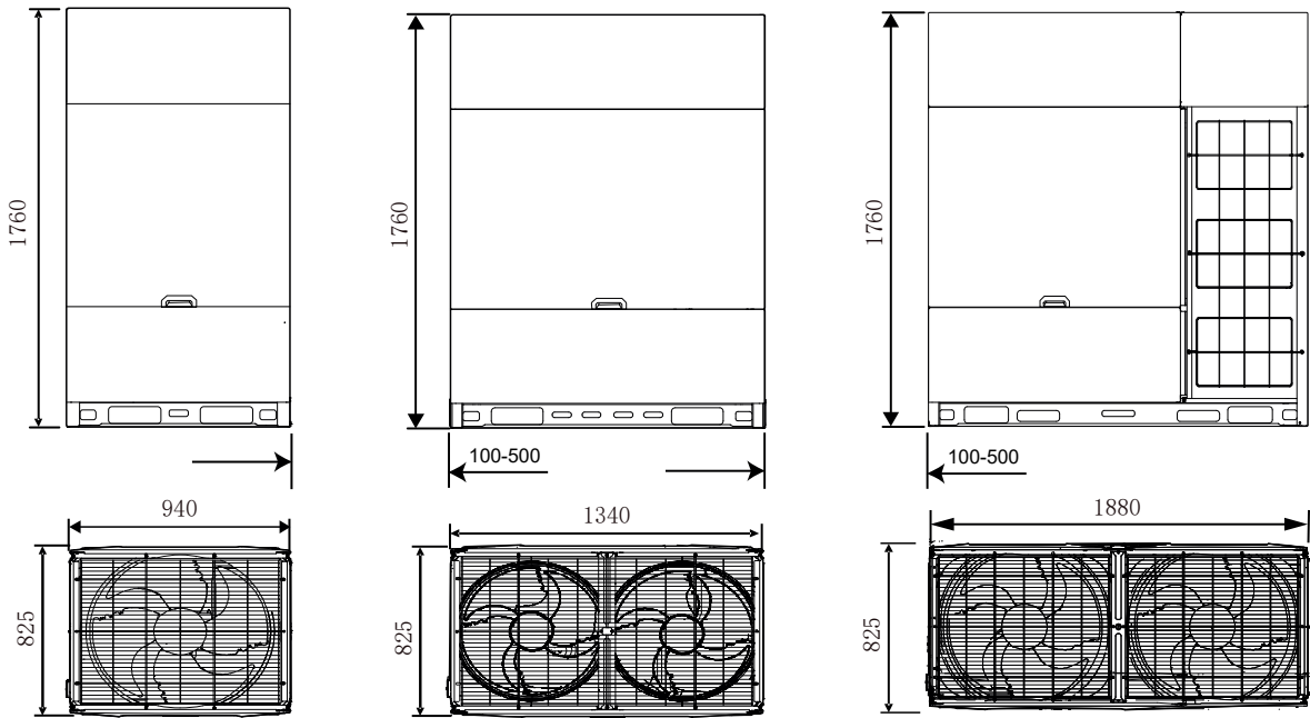
Figura 2-2.12: Dimensões das unidades 62/64/66/68HP (dimensões em mm)
