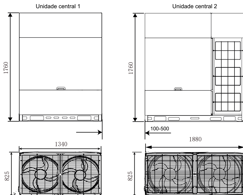
Figura 2-2.9: Dimensões das unidades 50/52HP (dimensões em mm)
