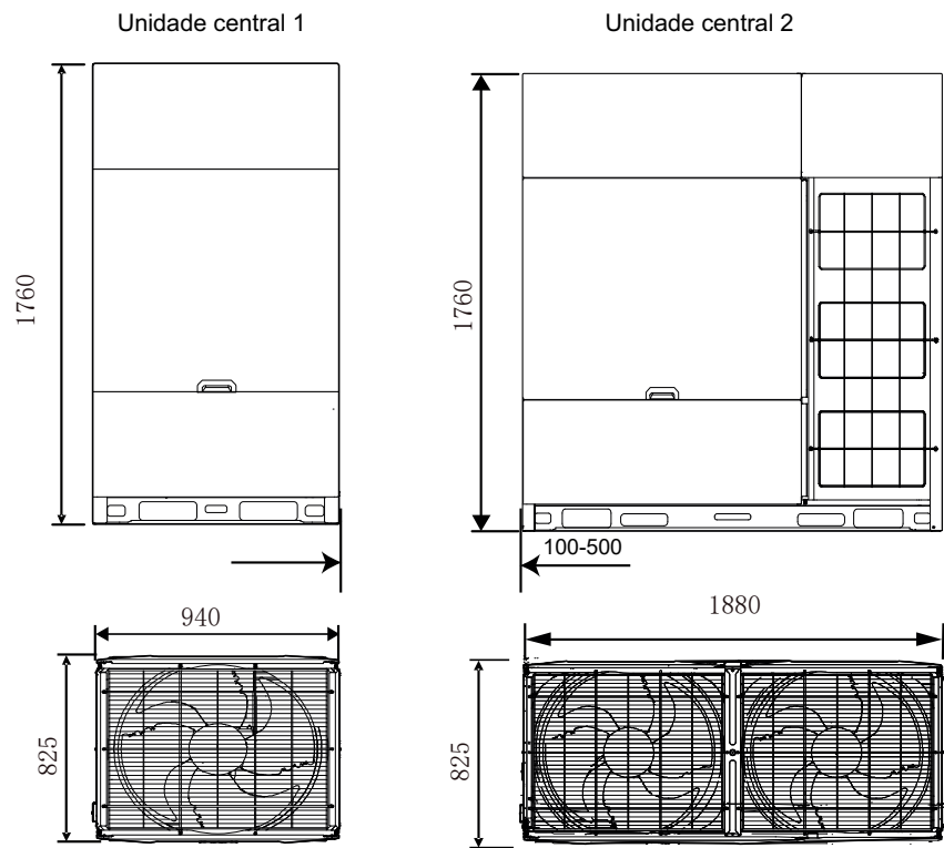
Figura 2-2.7: Dimensões da unidade 42/44HP (dimensões em mm)
