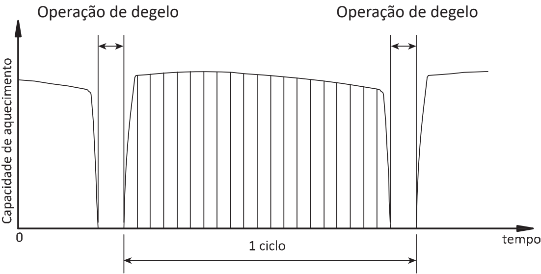
Figura 2-7.3: Ciclo de degelo
