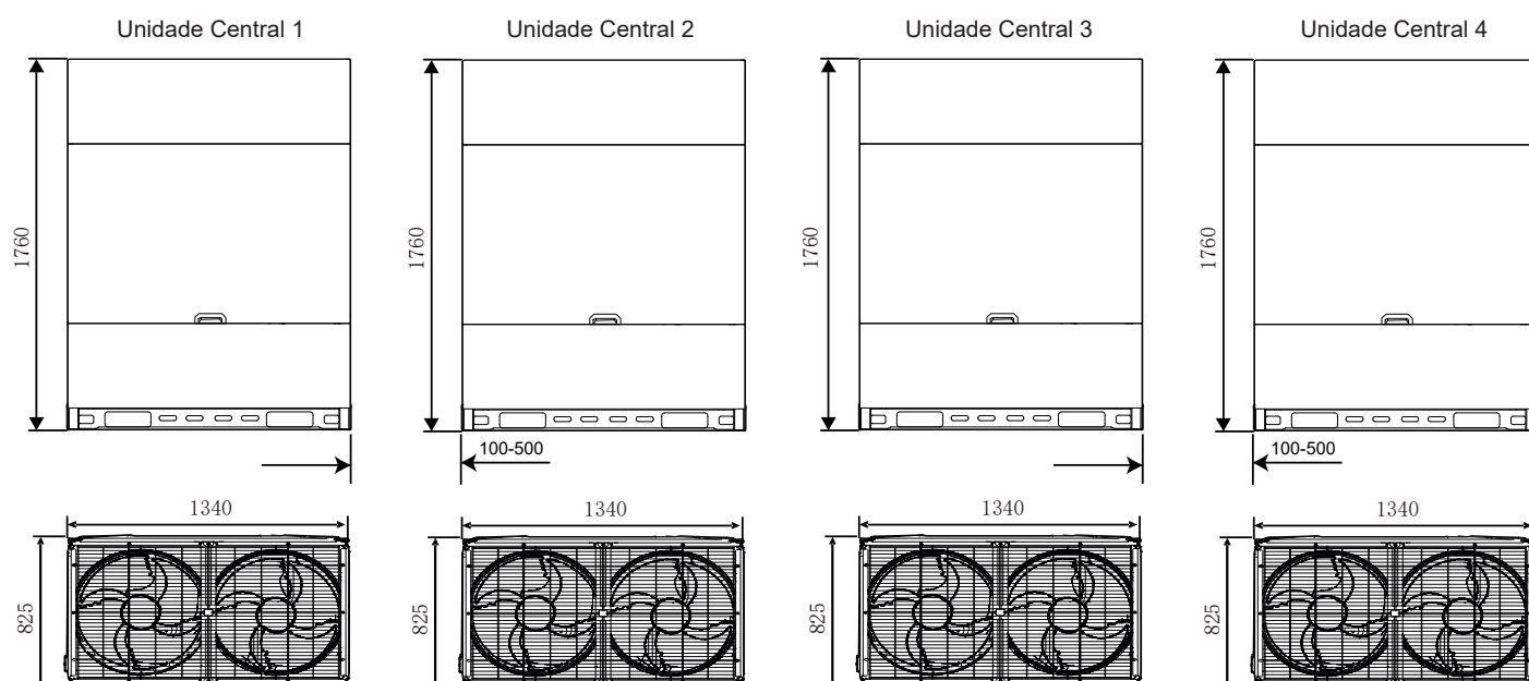
Figura 2-2.18: Dimensões das unidades 90/96HP (dimensões em mm)
