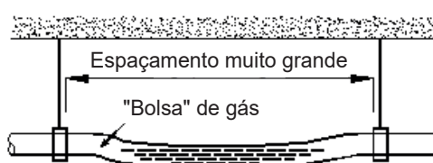
Figura 3-6.4: Efeito da sustentação insuficiente a tubulação de drenagem
