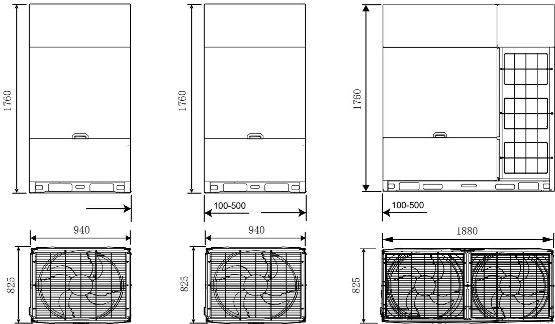
Figura 2-2.11: Dimensões da unidade 58/60HP (dimensões em mm)
