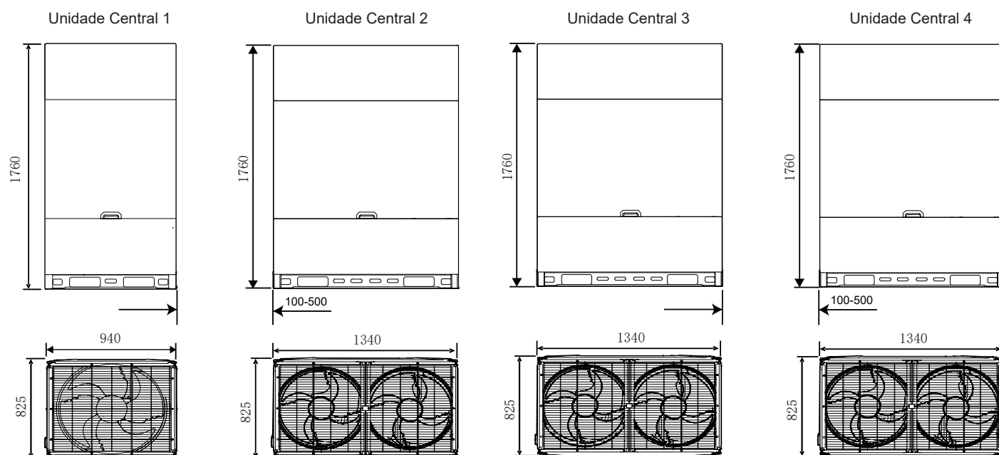
Figura 2-2.17: Dimensões da unidade 86/88HP (dimensões em mm)
