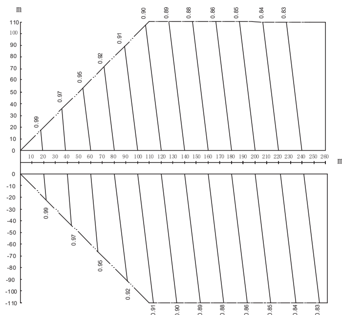
Figura 2-7.1: Taxa de mudança na capacidade de refrigeração
