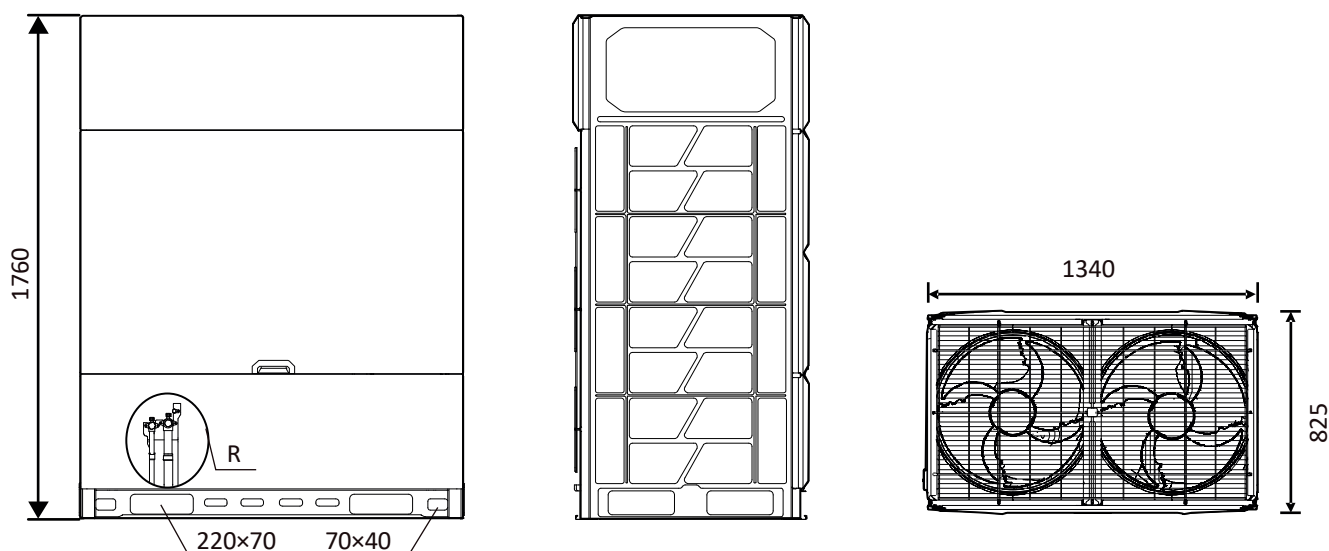
Figura 2-2.2: Dimensões 18/20/22/24HP (dimensões em mm)
