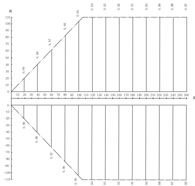
Figura 2-7.2: Taxa de mudança na capacidade de aquecimento
