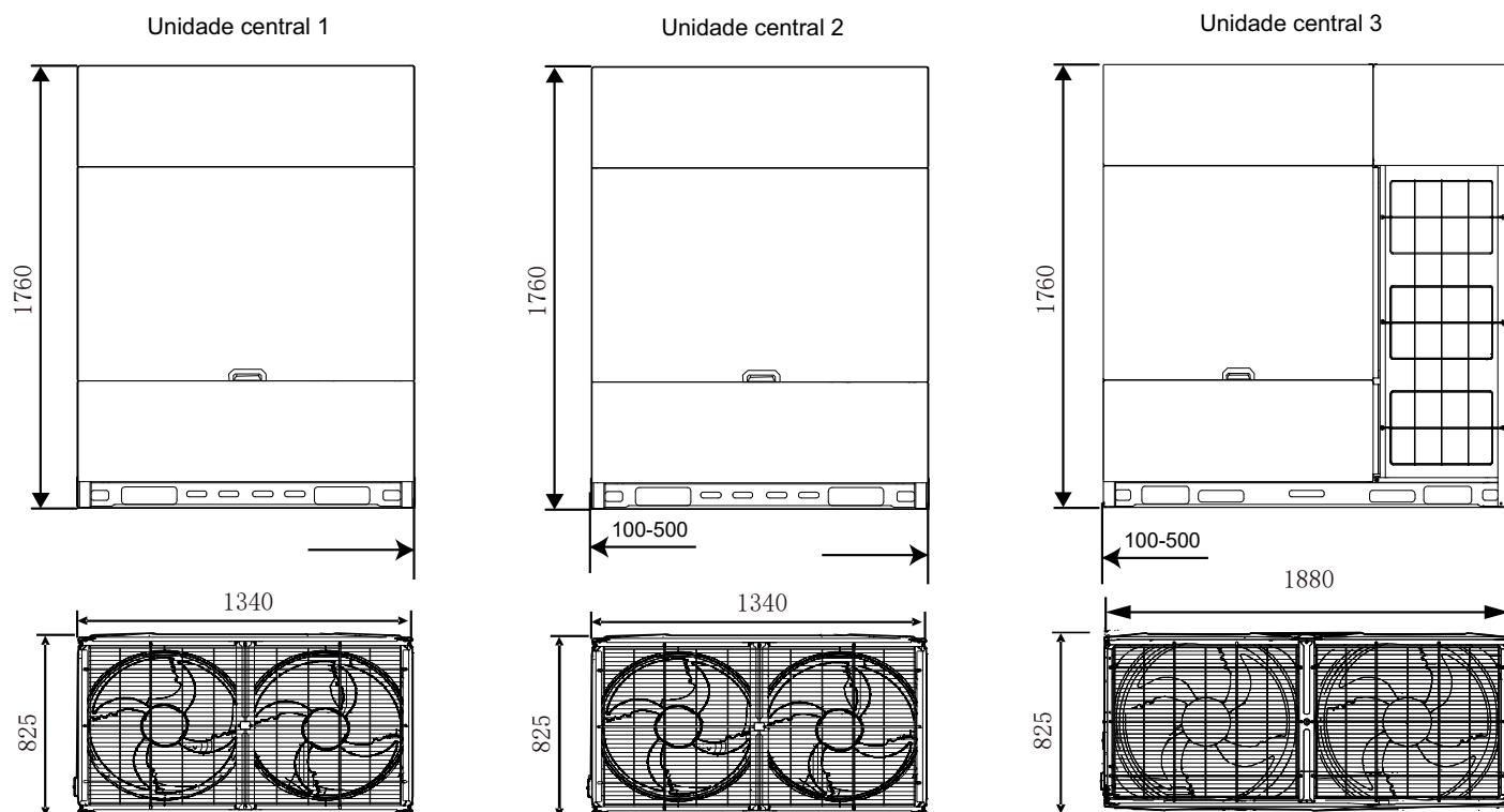
Figura 2-2.14: Dimensões das unidades 74/76HP (dimensões em mm)
