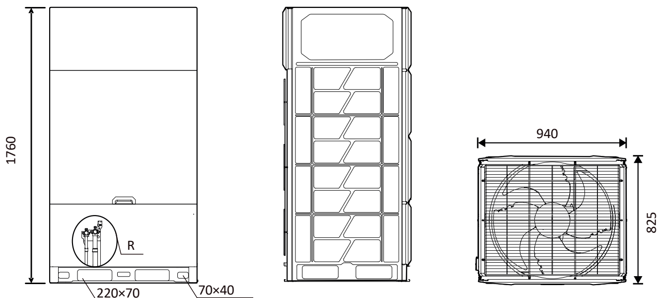
Figura 2-2.1: Dimensões 8/10/12/14/16HP (dimensões em mm)
