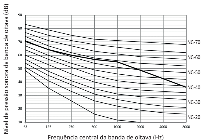
Figura 2-9.4 Nível da banda de oitava de 12HP
