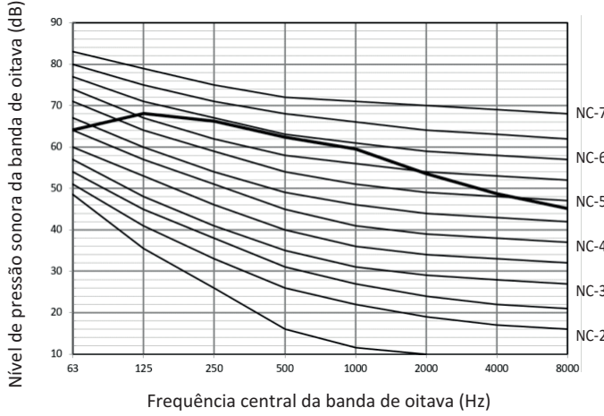
Figura 2-9.10 Nível da banda de oitava de 24HP
