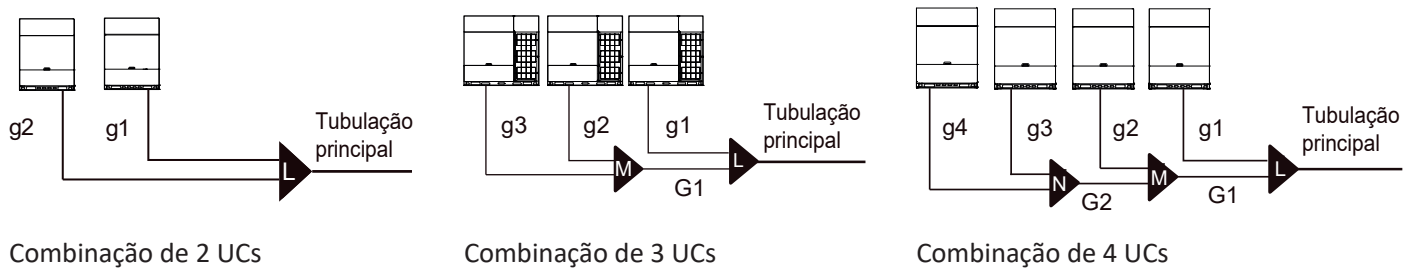
Figura 3-4.4: Conexões das tubulações das unidades centrais
