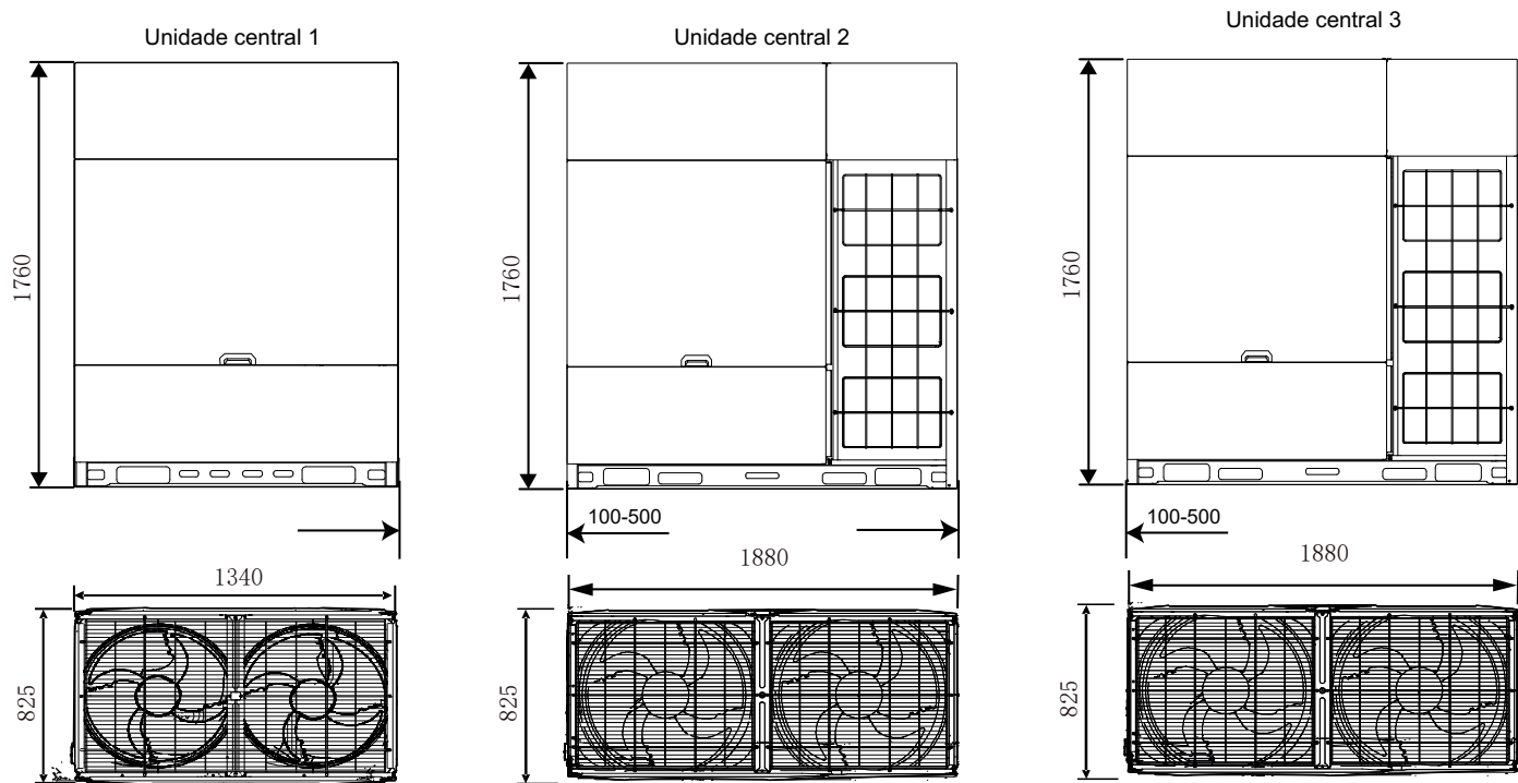
Figura 2-2.15: Dimensões da unidade 78/80HP (dimensões em mm)
