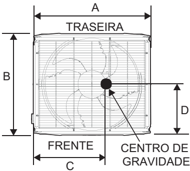
Figura 3-2.9: Centro de gravidade 20-40HP
