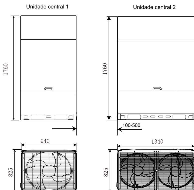
Figura 2-2.6: Dimensões das unidades 34/36/38/40HP (dimensões em mm)
