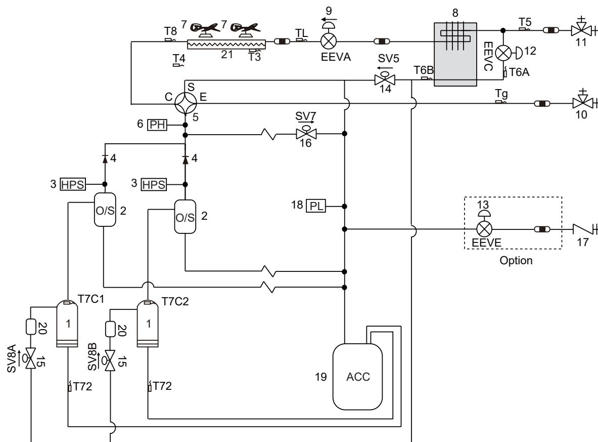
Figura 2-3.2: Diagramas de tubulação 20-24HP
