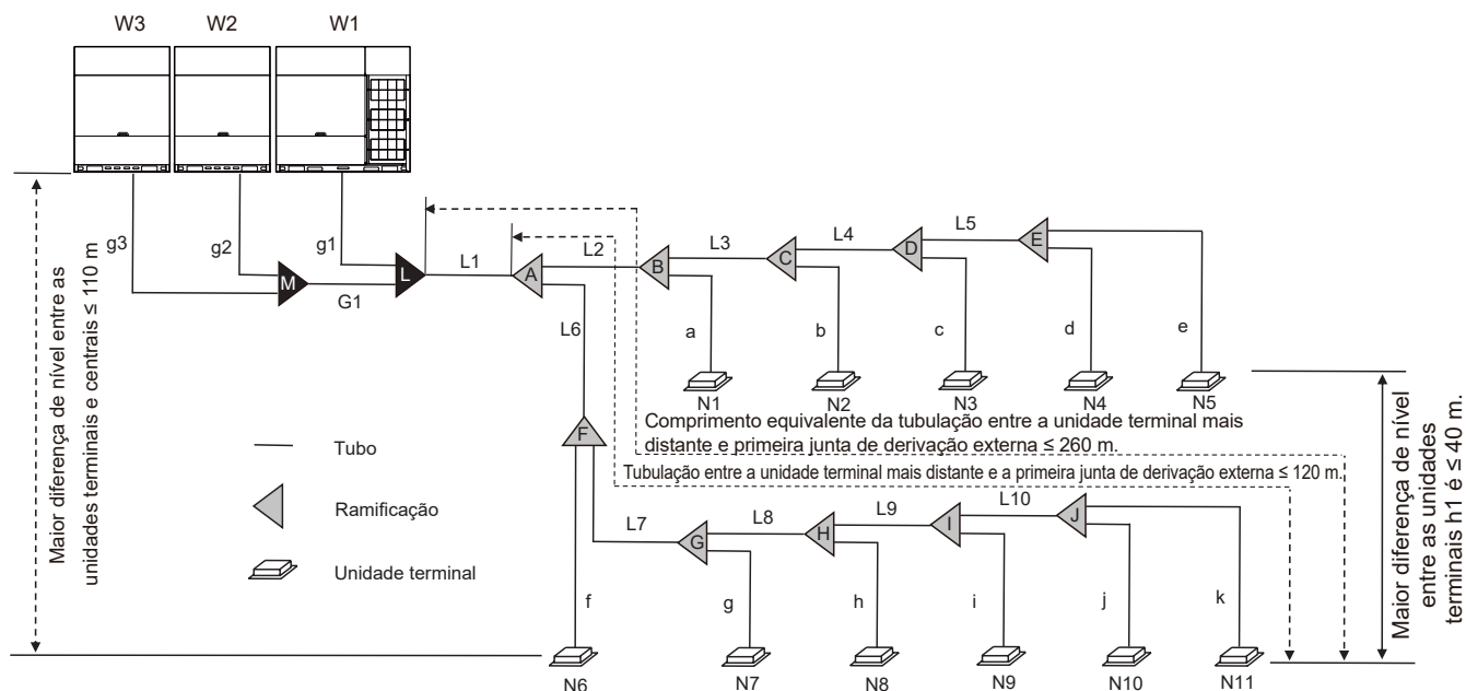
Figura 3-4.3: Seleção de diâmetros de tubulação
