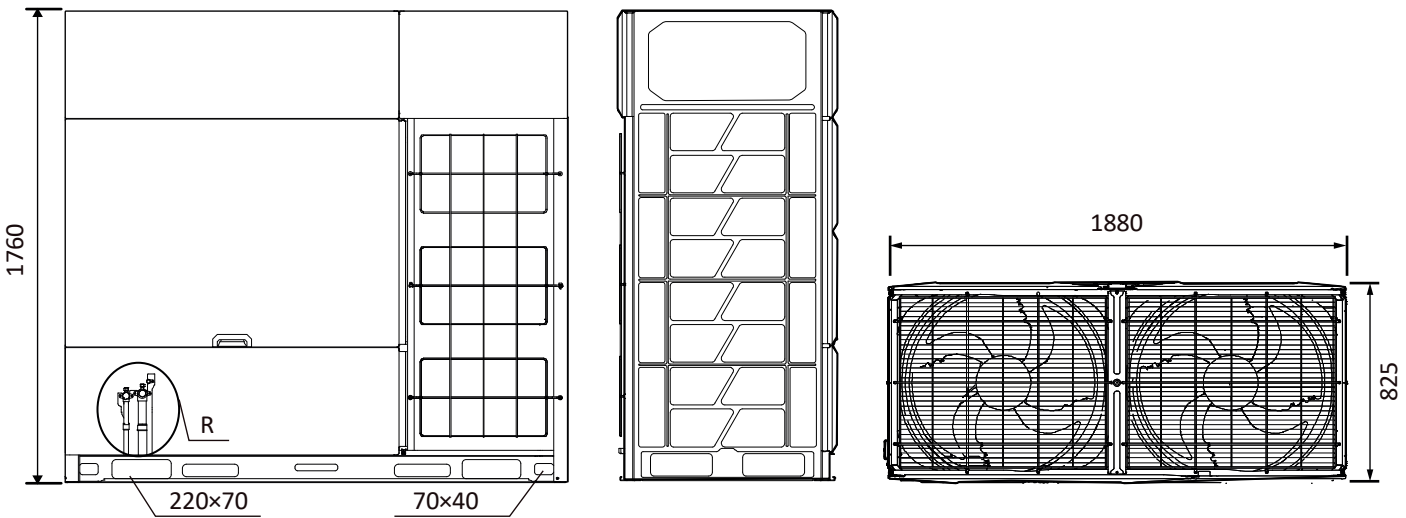
Figura 2-2.3: Dimensões 26/28HP (dimensões em mm)
