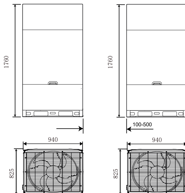
Figura 2-2.5: Dimensões da unidade 30-32HP (dimensões em mm)
