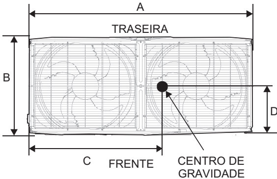
Figura 3-2.9: Centro de gravidade 20-40HP
