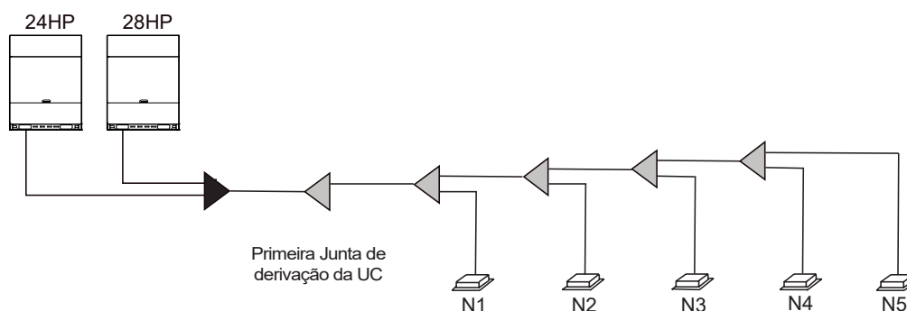
Figura 3-2.4: Posicionamento das unidades centrais mestre & auxiliar
