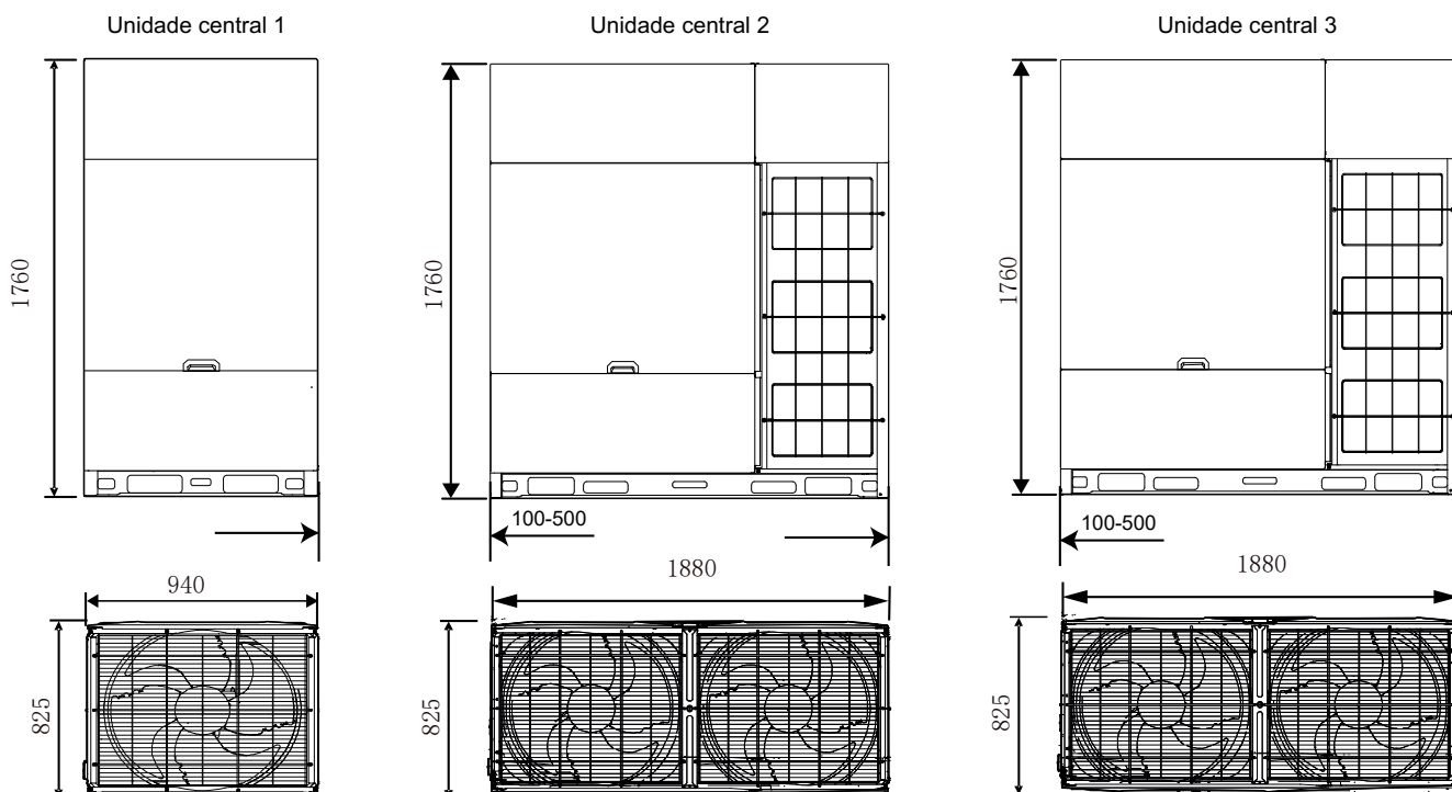
Figura 2-2.13: Dimensões da unidade 70/72HP (dimensões em mm)
