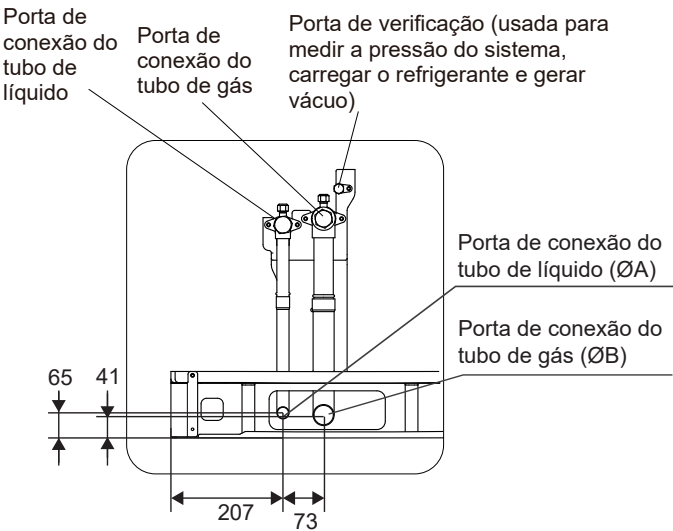
Figura 2-2.4: Detalhe R (dimensões em mm)
