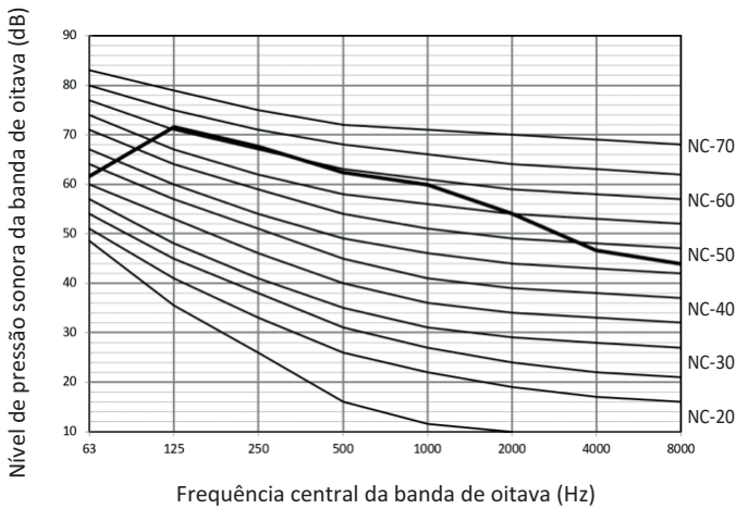
Figura 2-9.8 Nível da banda de oitava de 20HP
