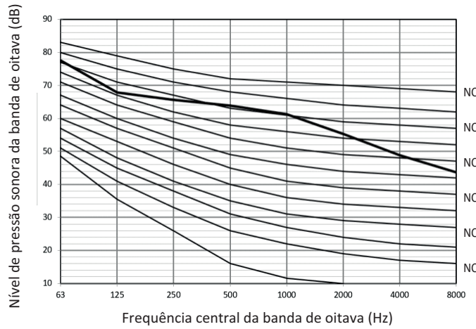
Figura 2-9.12 Nível da banda de oitava de 28HP
