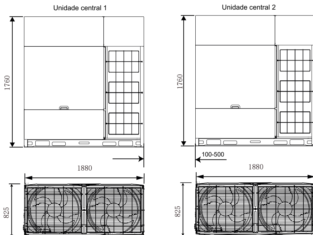
Figura 2-2.10: Dimensões das unidades 54/56HP (dimensões em mm)
