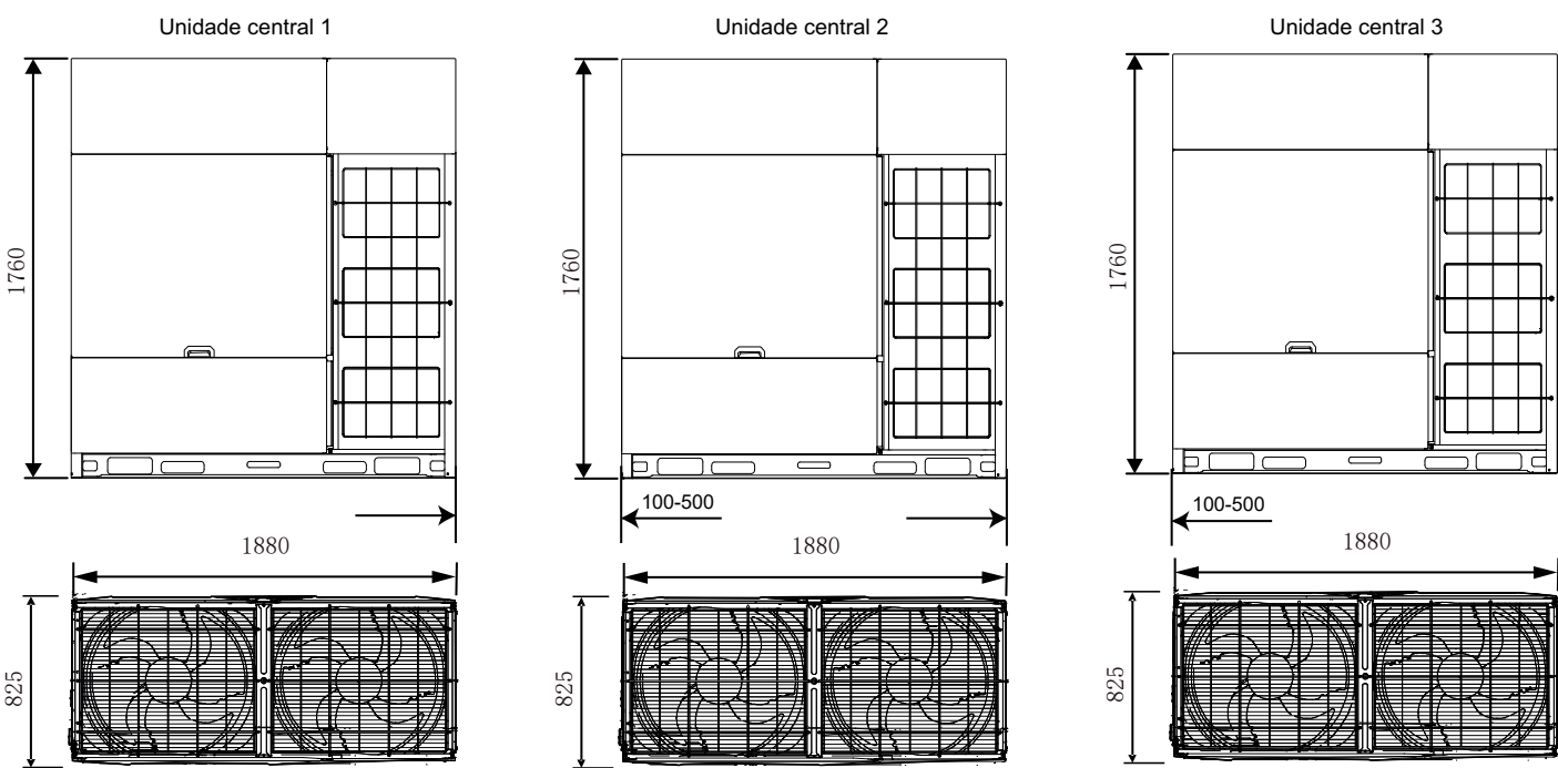
Figura 2-2.16: Dimensões das unidades 82/84HP (dimensões em mm)
