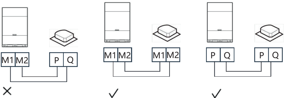
Figura 3-9.5: Fiação de comunicação
