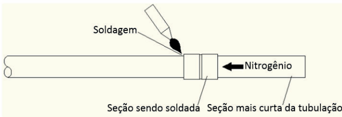
Figura 3-5.5: Fluxo de nitrogênio do lado mais curto durante a soldagem
