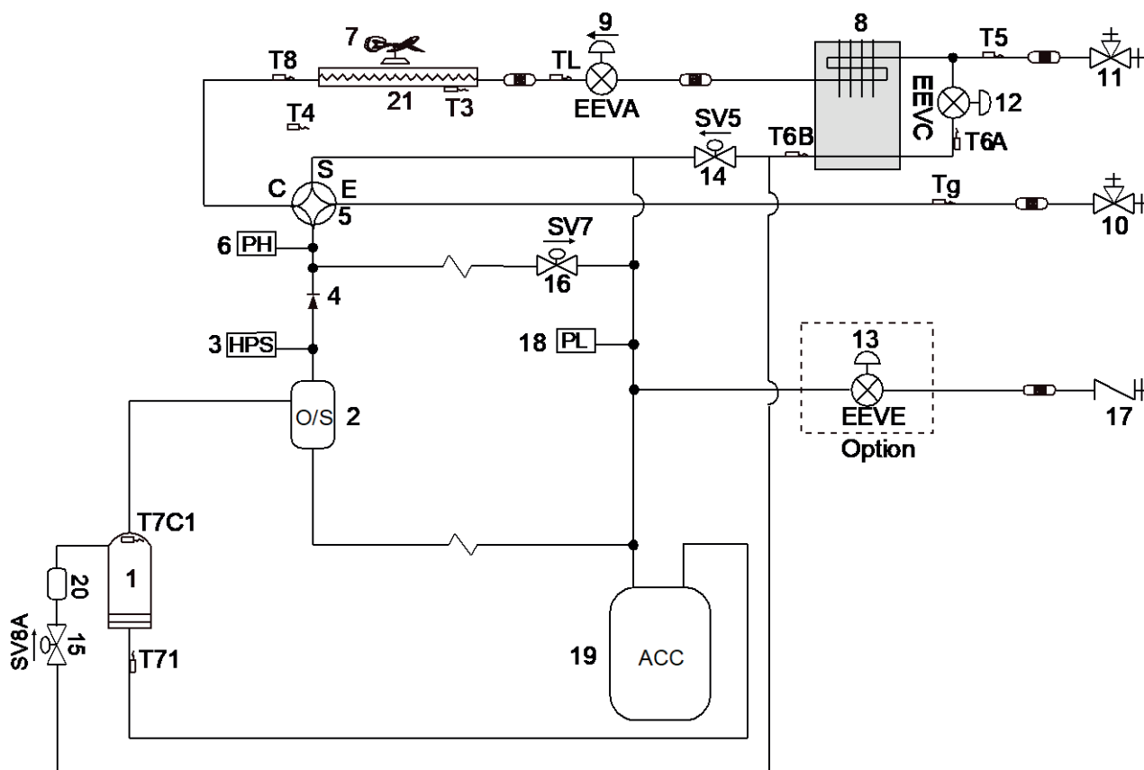
Figura 2-3.1: Diagramas de tubulação 8-18HP
