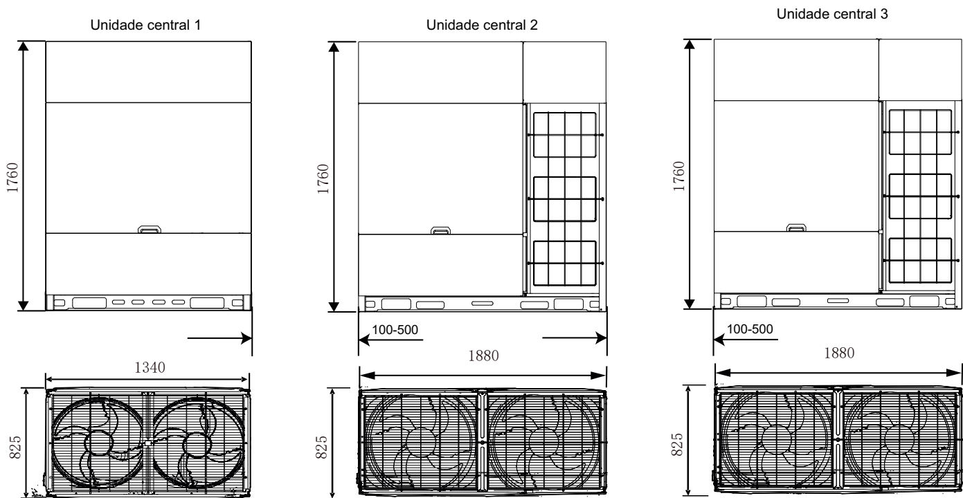
Figura 2-2.12: Dimensões das unidades 92/94/96/98/102HP (dimensões em mm)
