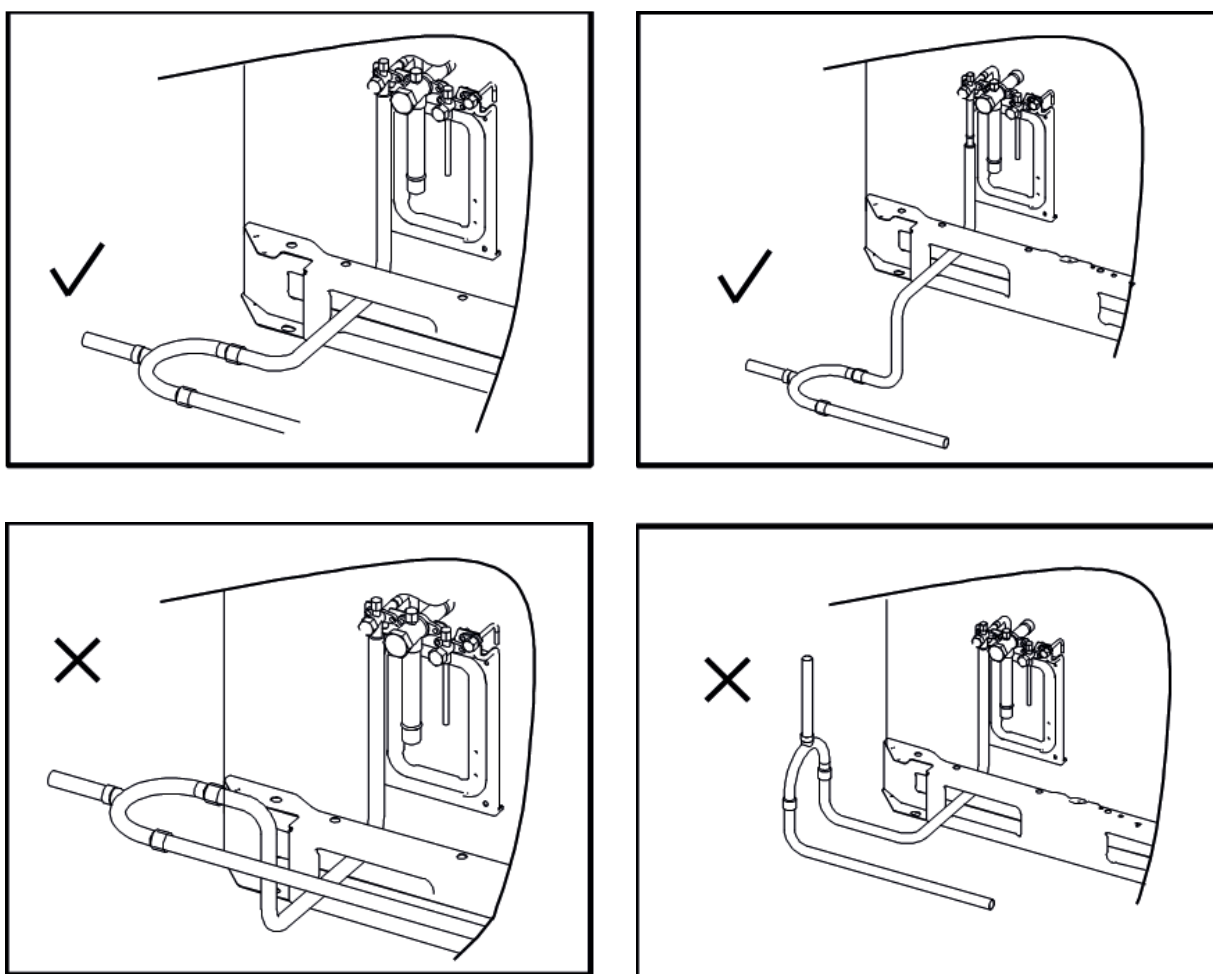
Figura 3-5.9: Instalação de juntas de derivação externas
