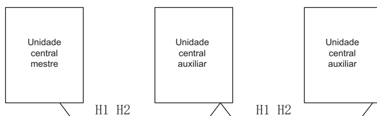
Figura 3-9.6: Comunicação das unidades centrais
