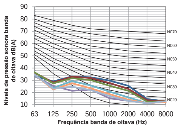
Figura 8.5: MIH36Q1DHN1(A) níveis banda de oitava
