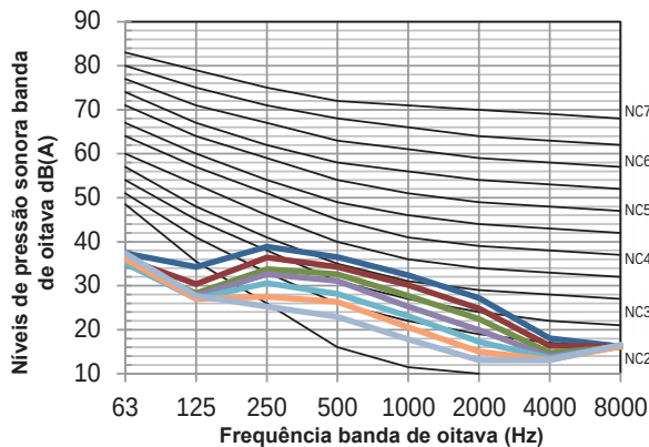
Figura 8.8: MIH-71Q1DHN1(A) níveis banda de oitava
