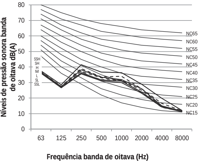
Figura 8.4: MIH-45Q1DHN1 níveis banda de oitava
