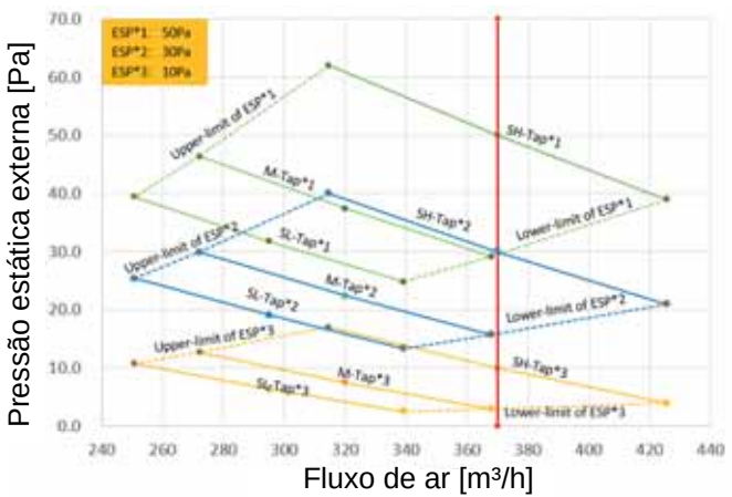
Figura 9.12: MIH22T3HN18
