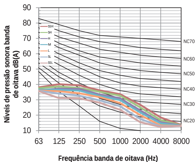
Figura 8.9: MIH80T3HN18 níveis banda de oitava
