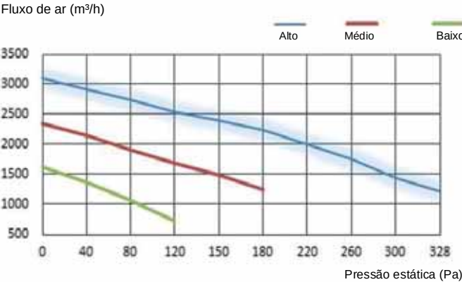
Figura 8.8: HRV-D2000(C)
