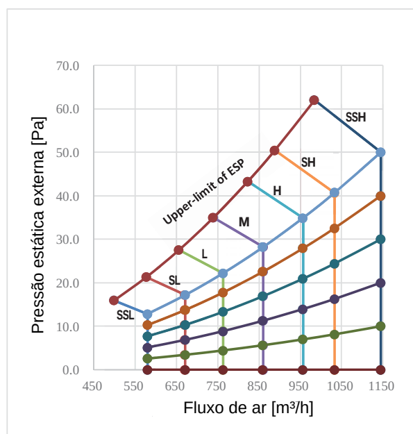
Figura 9.7: MIH71T3HN18
