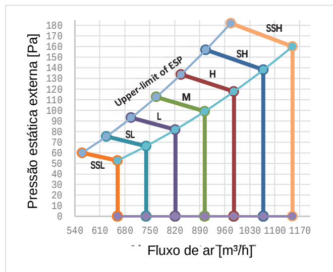
Figura 9.7: MIH71T2HN18
