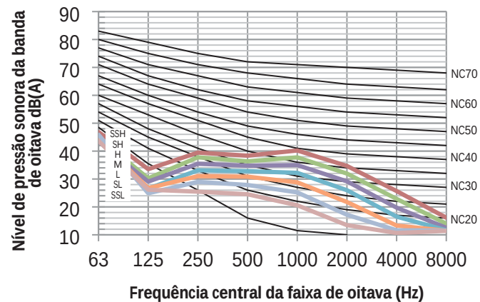
Figura 8.9: MIH80GHN18 níveis banda de oitava
