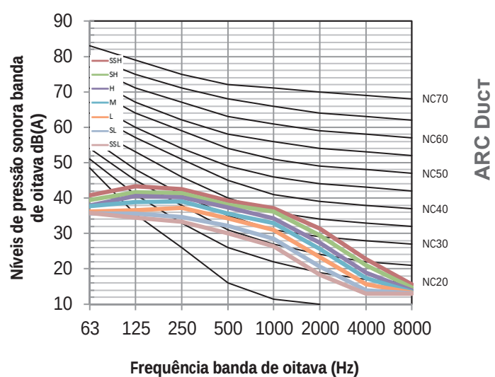
Figura 8.11: MIH112T3HN18 níveis banda de oitava
