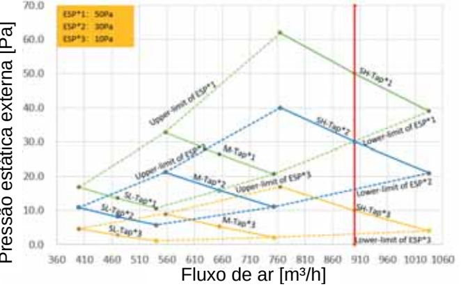
Figura 9.16: MIH56T3HN18
