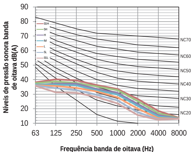
Figura 8.10: MIH90T3HN18 níveis banda de oitava
