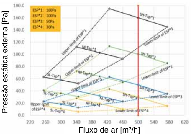
Figura 9.14: MIH22T2HN18
