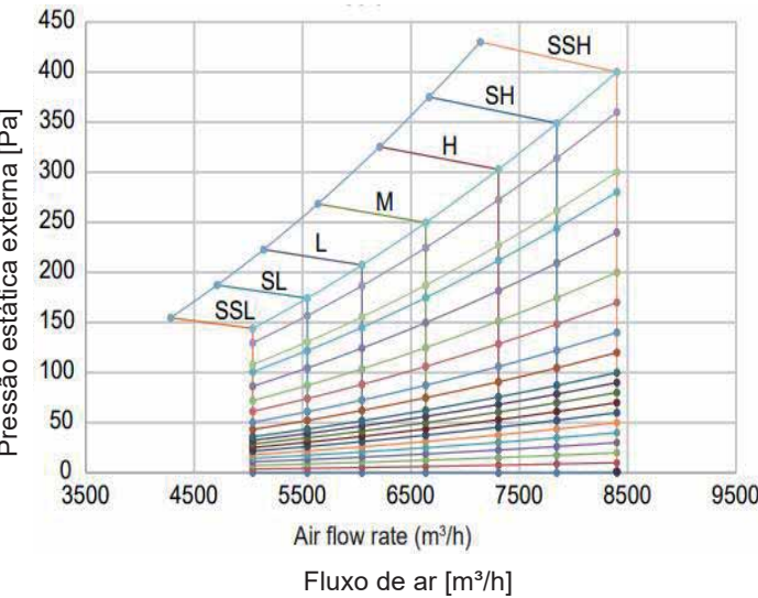
Figura 9.10: MIH560T1HN18
