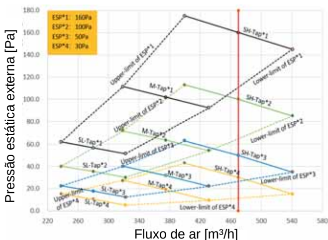
Figura 9.13: MIH15T2HN18
