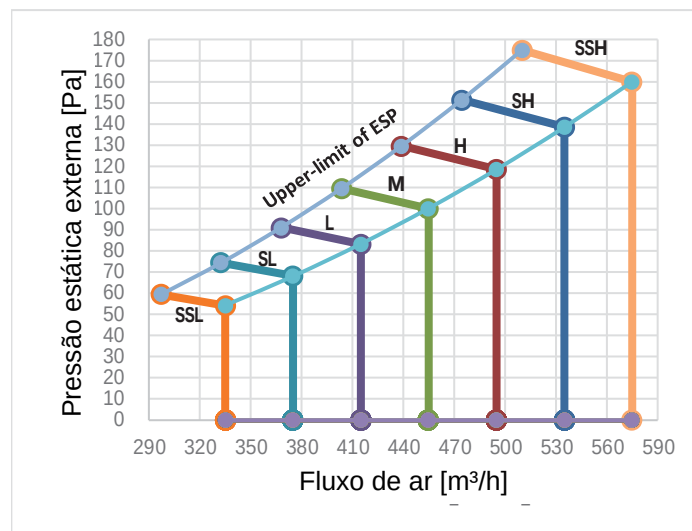
Figura 9.6: MIH56T2HN18
