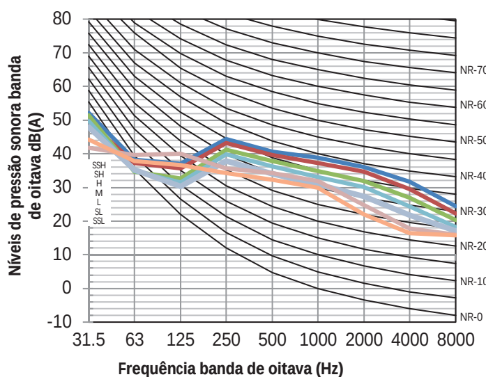
Figura 8.6: MIH140T1HN18 níveis banda de oitava
