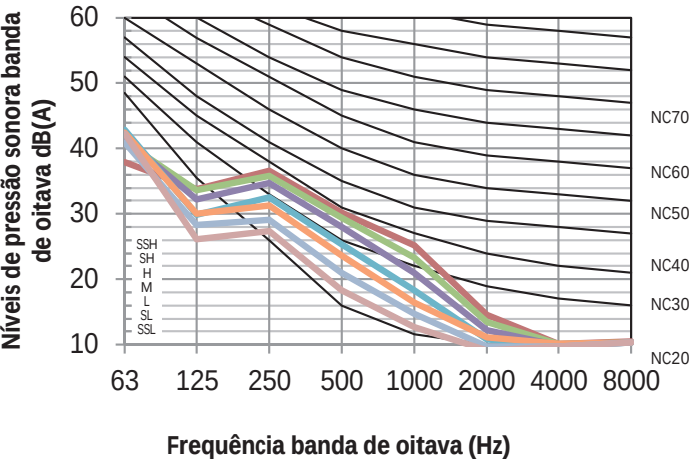
Figura 8.2: MIH28Q4HN18 níveis banda de oitava
