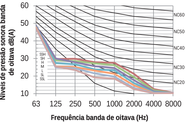
Figura 8.3: MIH22GHN18 níveis banda de oitava
