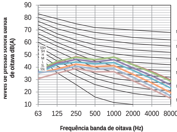
Figura 8.12: MIH160DLHN18 níveis banda de oitava
