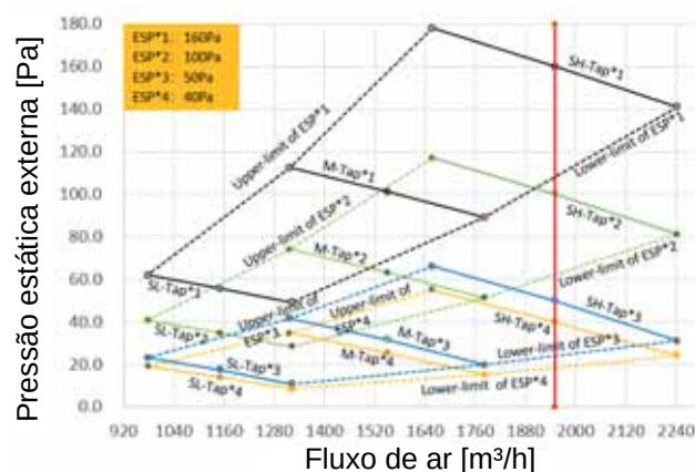
Figura 9.22: MIH112T2HN18
