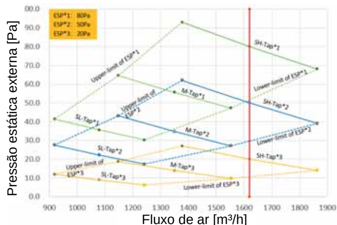
Figura 9.20: MIH112T3HN18
