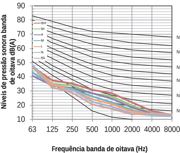
Figura 8.4: MIH28T3HN18 níveis banda de oitava
