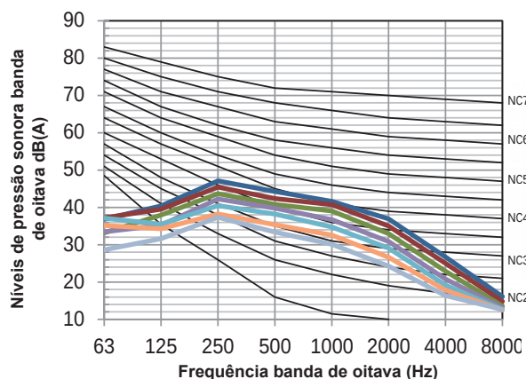
Figura 8.8: MIH-71Q1DHN1(A) níveis banda de oitava
