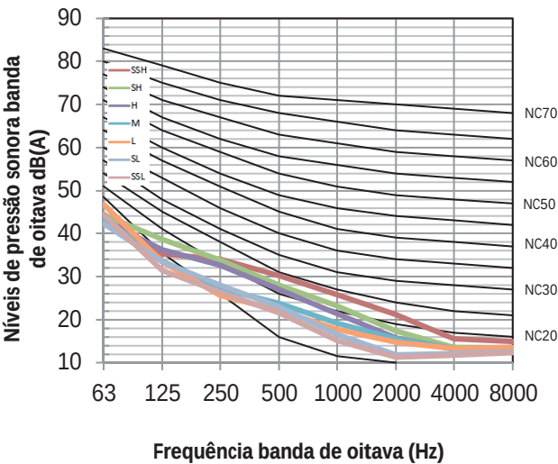
Figura 8.5: MIH36T3HN18 níveis banda de oitava
