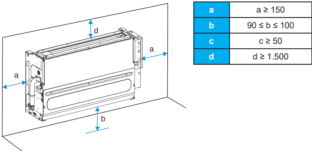
Figura 3.2: Requisitos de espaço de unidade de piso oculta da série F3 (unidade: mm)
