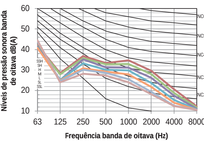
Figura 8.4: MIH28GHN18 níveis banda de oitava
