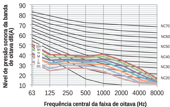
Figura 8.8: MIH71GHN18 níveis banda de oitava
