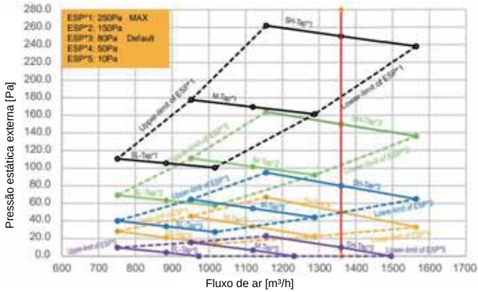
Figura 9.7: MIH56(71,80)T1HN18
