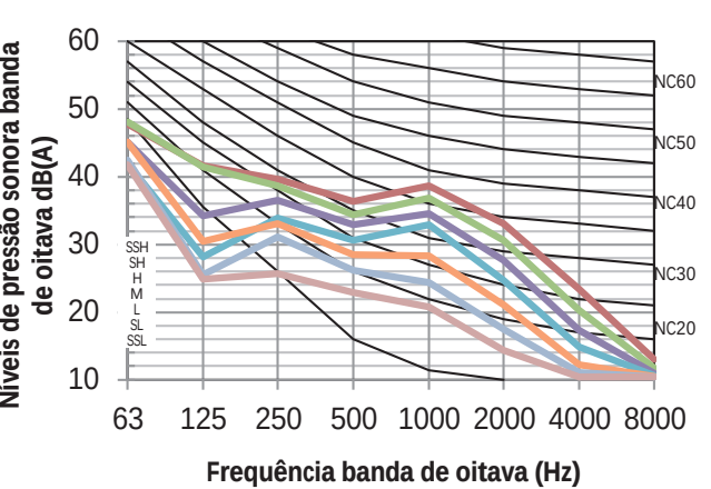
Figura 8.7: MIH56GHN18 níveis banda de oitava
