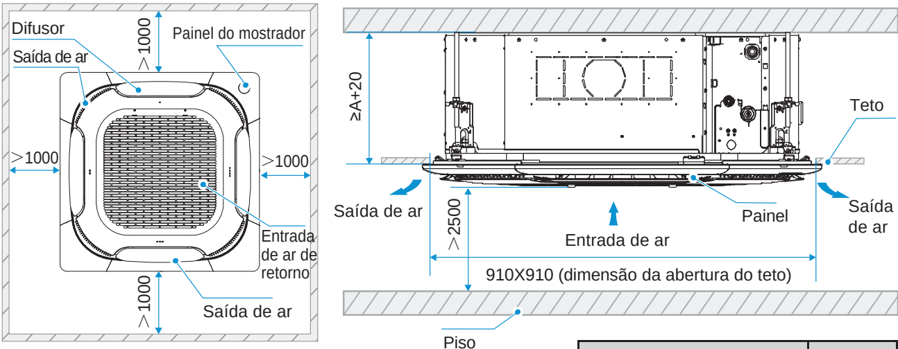
Figura 3.1: Requisitos de espaço do Cassette Quatro Vias de 2.8-14.0kW (unidade: mm)
