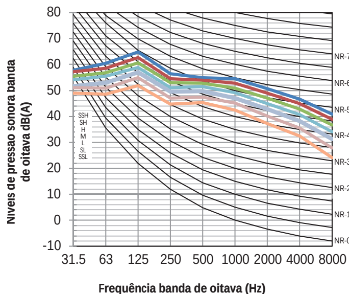
Figura 8.13: MIH400T1HN18 níveis banda de oitava
