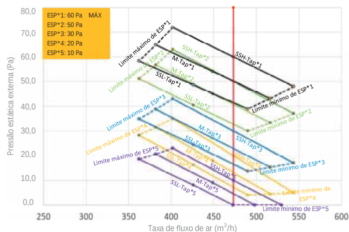
Figura 9.2: Desempenho do ventilador MIH28F3HN18
