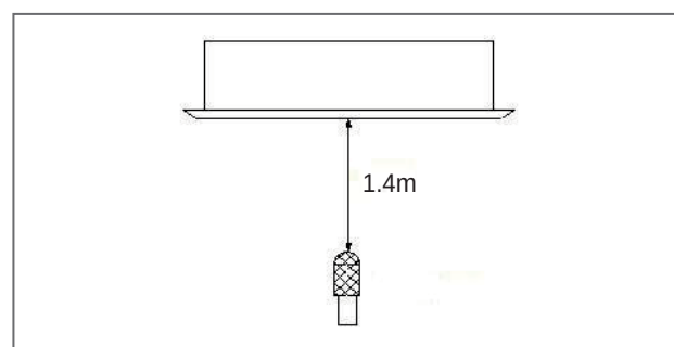
Figura 8.1: Medição do nível de pressão sonora do Cassete de Uma Via
