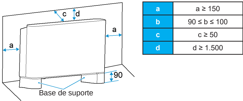
Figura 3.2: Requisitos de espaço de unidade de piso exposta da série F5 (entrada de ar por baixo) (unidade: mm)
