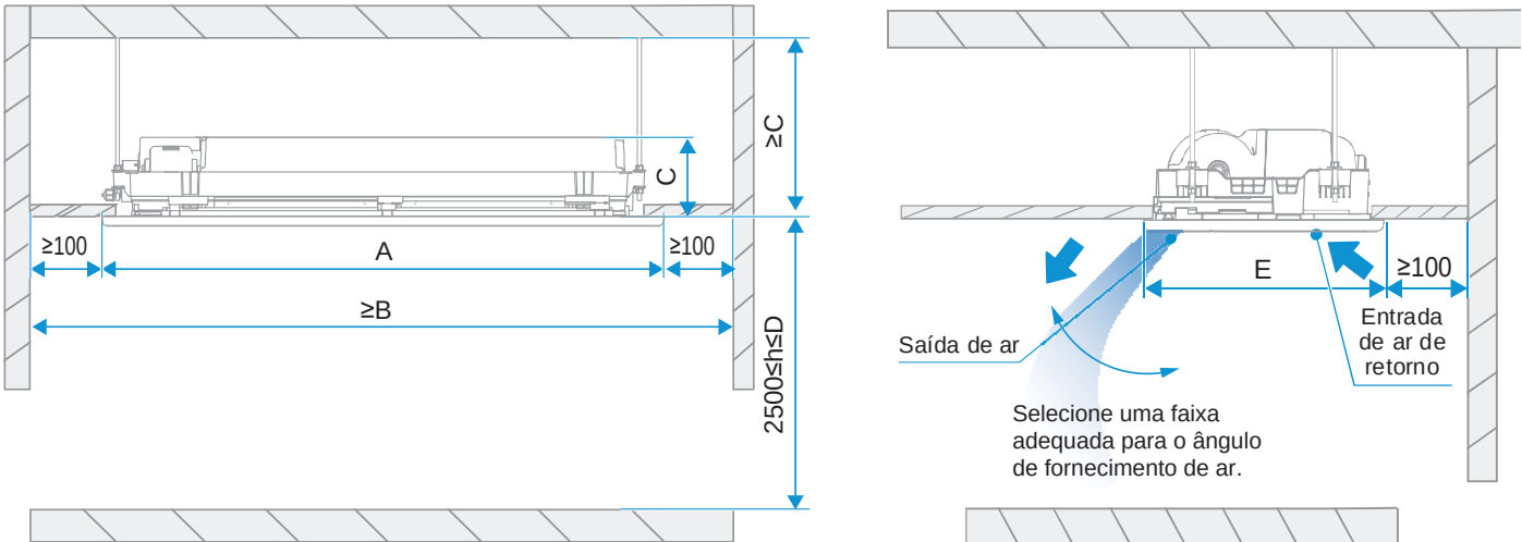
Figura 3.1: Requisitos de espaçamento do Cassete de Uma Via (unidade: mm)
