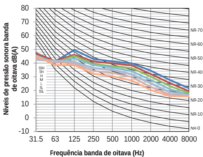
Figura 8.5: MIH125T1HN18 níveis banda de oitava
