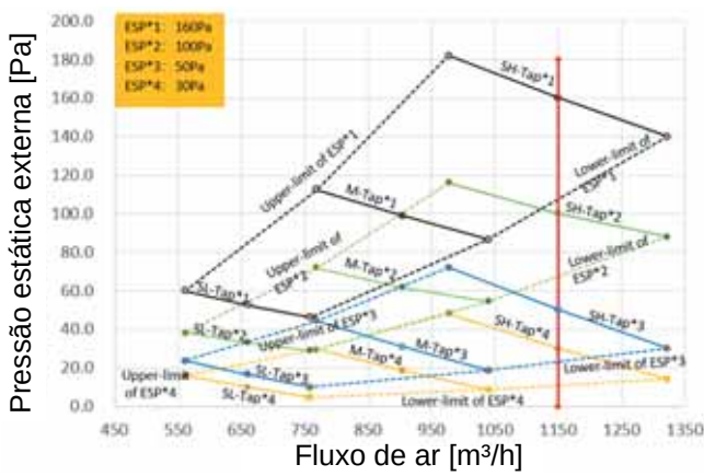
Figura 9.19: MIH71T2HN18
