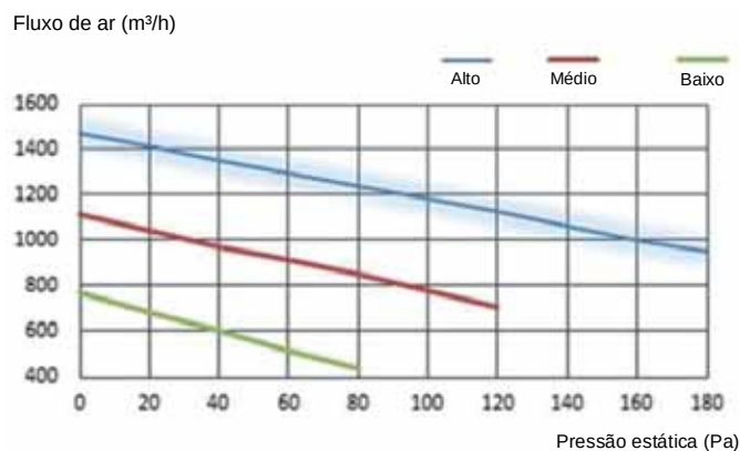
Figura 8.6: HRV-D1000(C)
