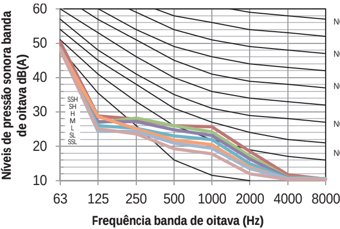
Figura 8.2: MIH15GHN18 níveis banda de oitava
