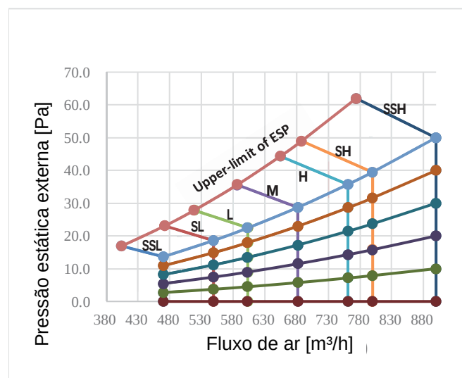
Figura 9.6: MIH56T3HN18
