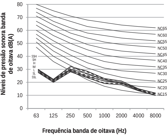
Figura 8.2: MIH-18(22)Q1DHN1 níveis banda de oitava
