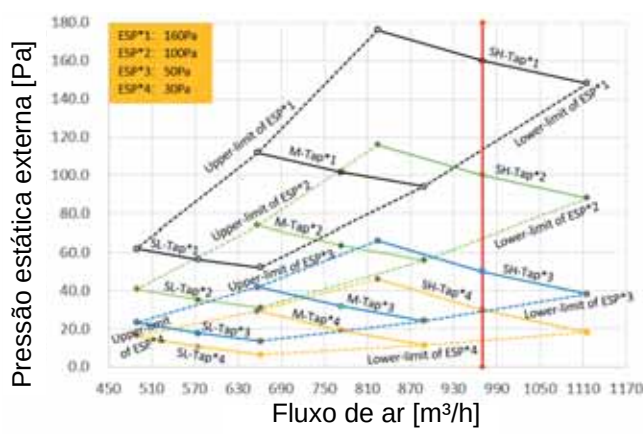
Figura 9.18: MIH56T2HN18
