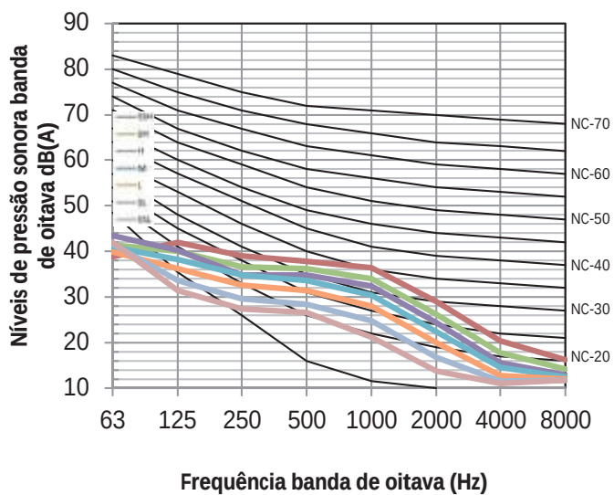
Figura 8.11: MIH90T2HN18 níveis banda de oitava
