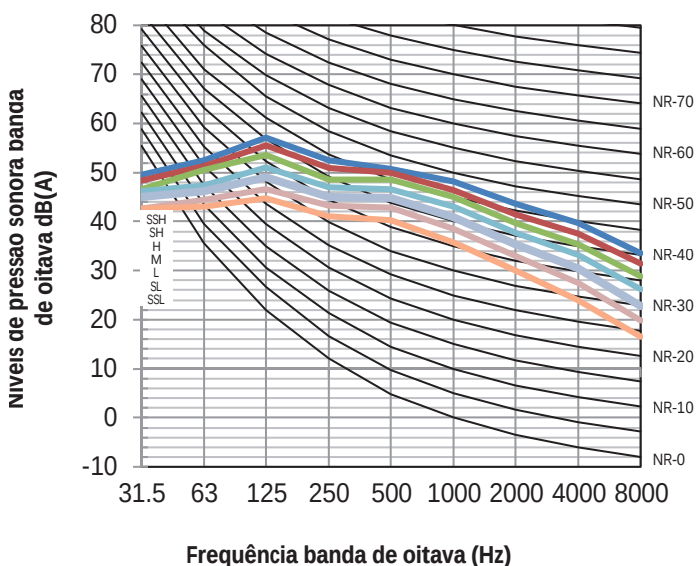
Figura 8.9: MIH224T1HN18 níveis banda de oitava
