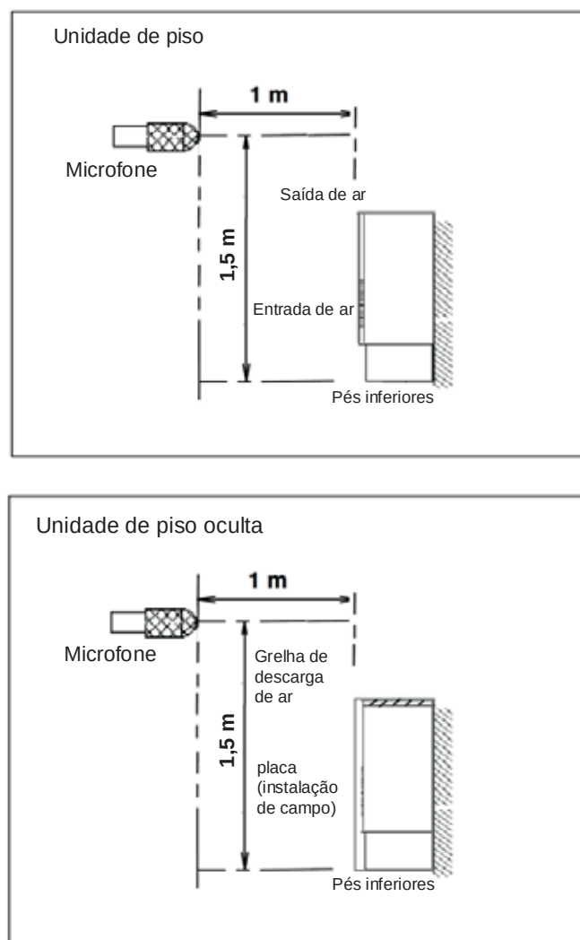
Figura 10.1: Medição dos níveis de pressão sonora da unidade de piso
