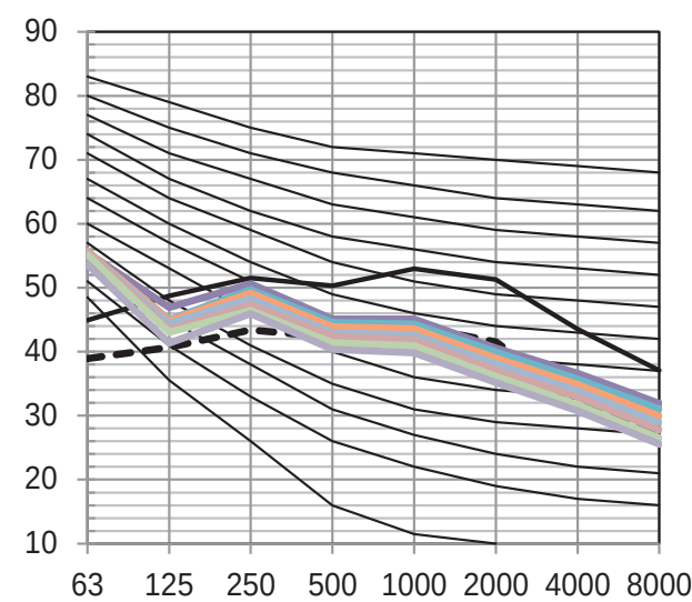
Figura 9.2: Níveis banda de oitava MIH200(224)FAHN18
