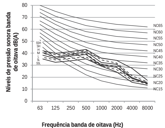
Figura 8.6: MIH-71Q2DHN1 níveis banda de oitava
