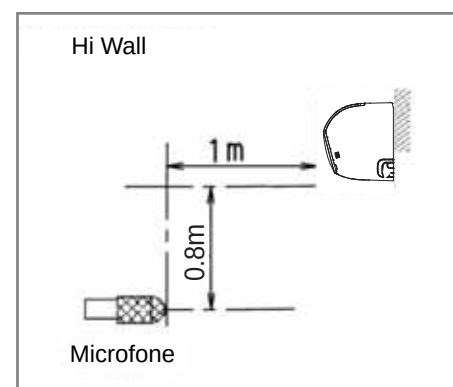
Figura 8.1: Medição do nível de pressão sonora do Hi Wall
