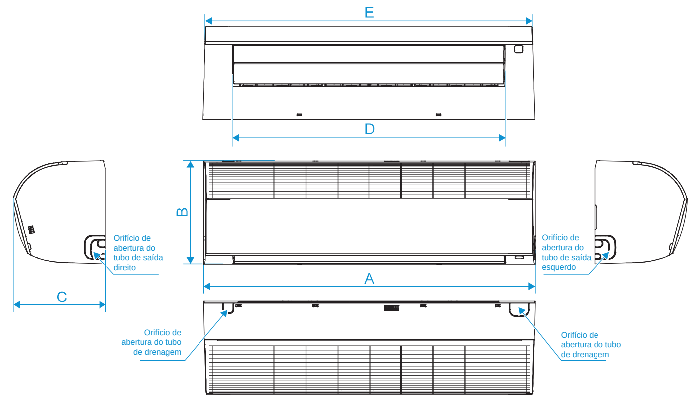
Figura 2.1: Dimensões do Hi Wall (unidade: mm)
