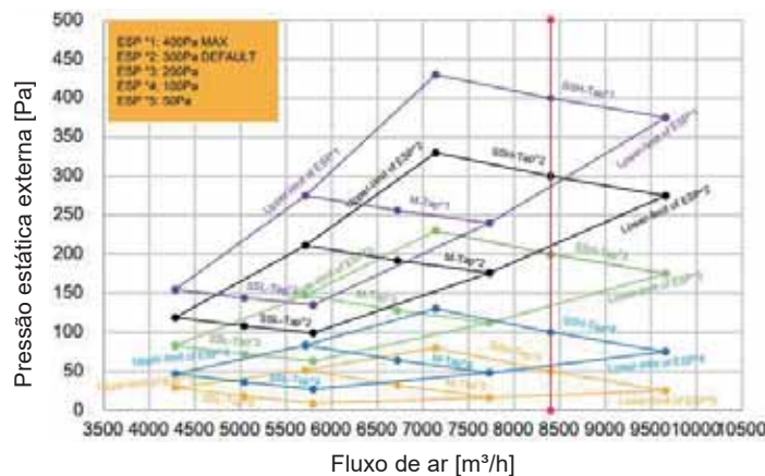
Figura 9.20: MIH560T1HN18
