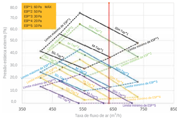
Figura 9.4: Desempenho do ventilador MIH45F3HN18
