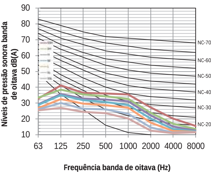
Figura 8.9: MIH71T2HN18 níveis banda de oitava
