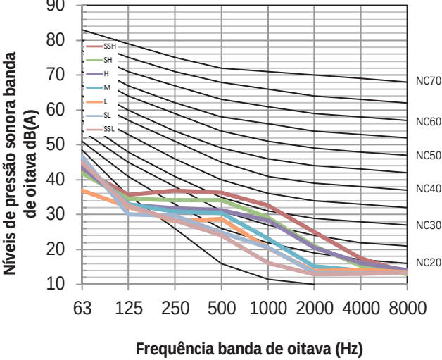
Figura 8.7: MIH56T3HN18 níveis banda de oitava
