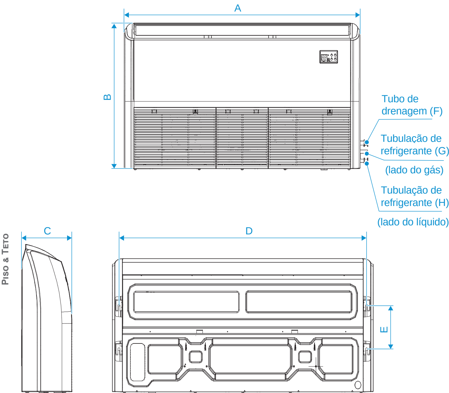
Figura 2.1: Dimensões do Piso-Teto (unidade: mm)
