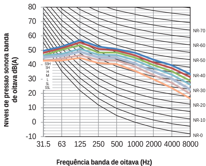
Figura 8.11: MIH280T1HN18 níveis banda de oitava
