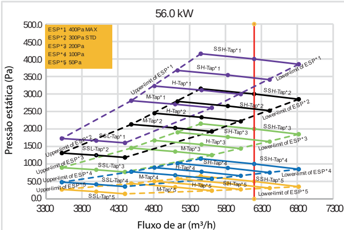
Figura 6.6: Performance do ventilador MIH560FAHN18
