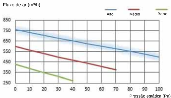
Figura 8.6: HRV-D1000(C)
