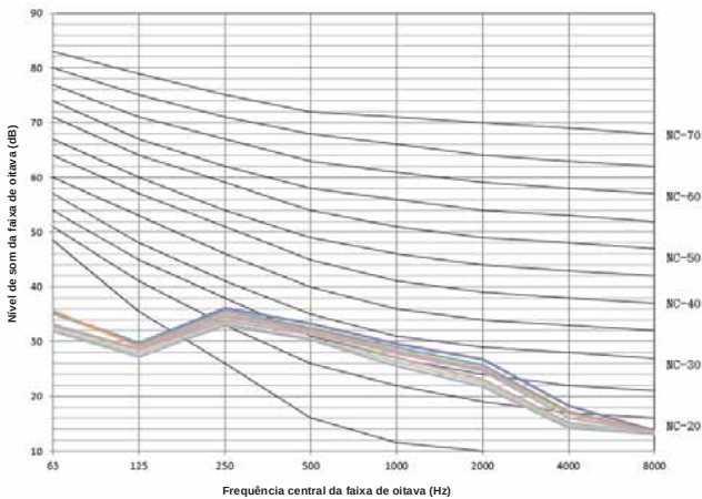
Figura 10.9: Níveis de banda de oitava MIH22F4HN18, MIH22F5HN18
