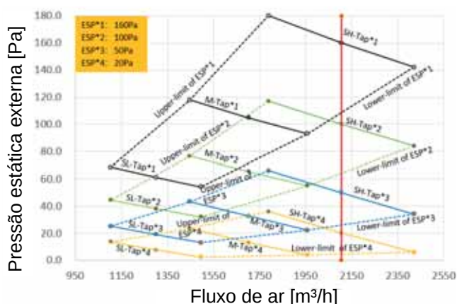
Figura 9.23: MIH140T2HN18
