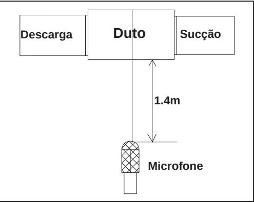
Figura 9.1: Medição do nível de pressão sonora
