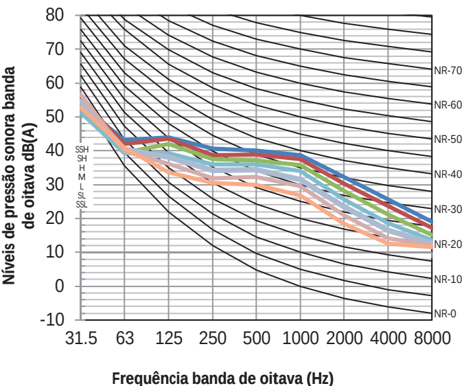
Figura 8.3: MIH90T1HN18 níveis banda de oitava
