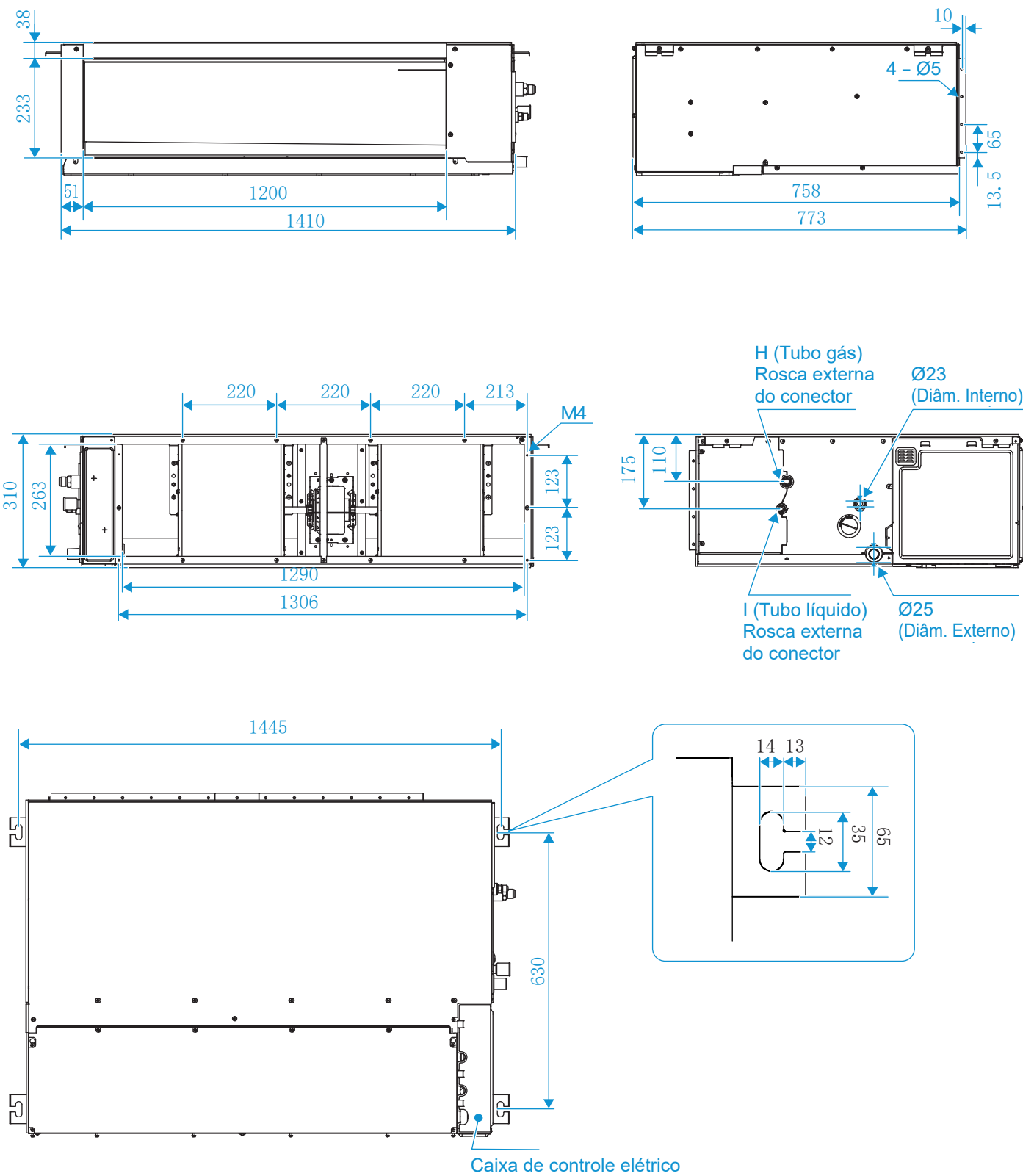
Figura 2.2: Dimensões modelos MIH224(280)FASHN18 (unidade: mm)
