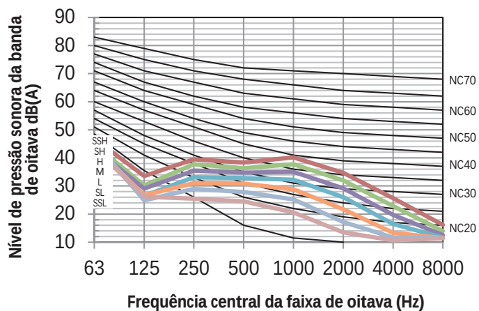
Figura 8.10: MIH90GHN18 níveis banda de oitava
