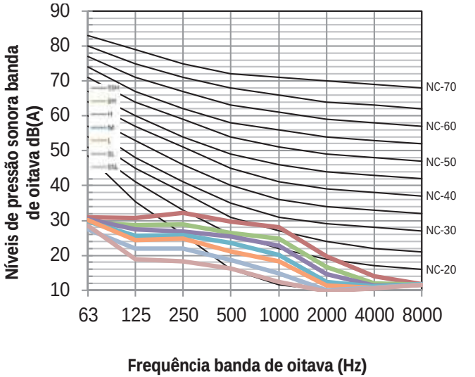
Figura 8.6: MIH36T2HN18 níveis banda de oitava
