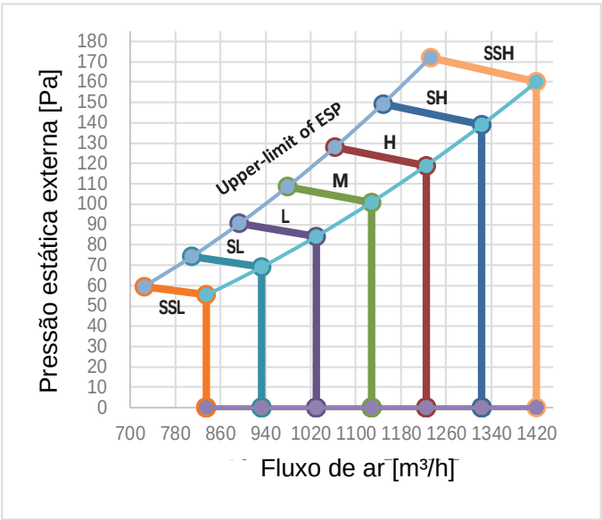
Figura 9.9: MIH90T2HN18
