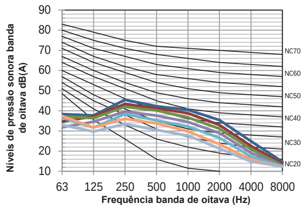
Figura 8.7: MIH56Q1DHN1(A) níveis banda de oitava
