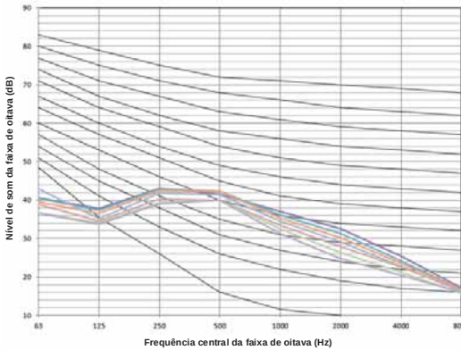
Figura 10.9: Níveis de banda de oitava MIH22F4HN18, MIH22F5HN18
