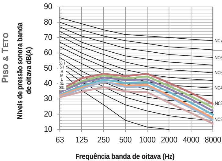
Figura 8.10: MIH125DLHN18 níveis banda de oitava
