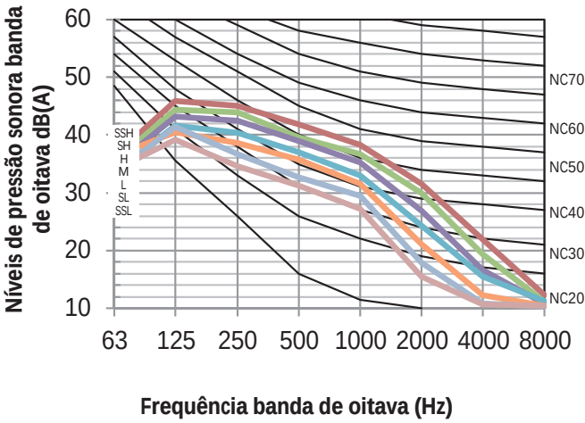
Figura 8.11: MIH140Q4HN18 níveis banda de oitava
