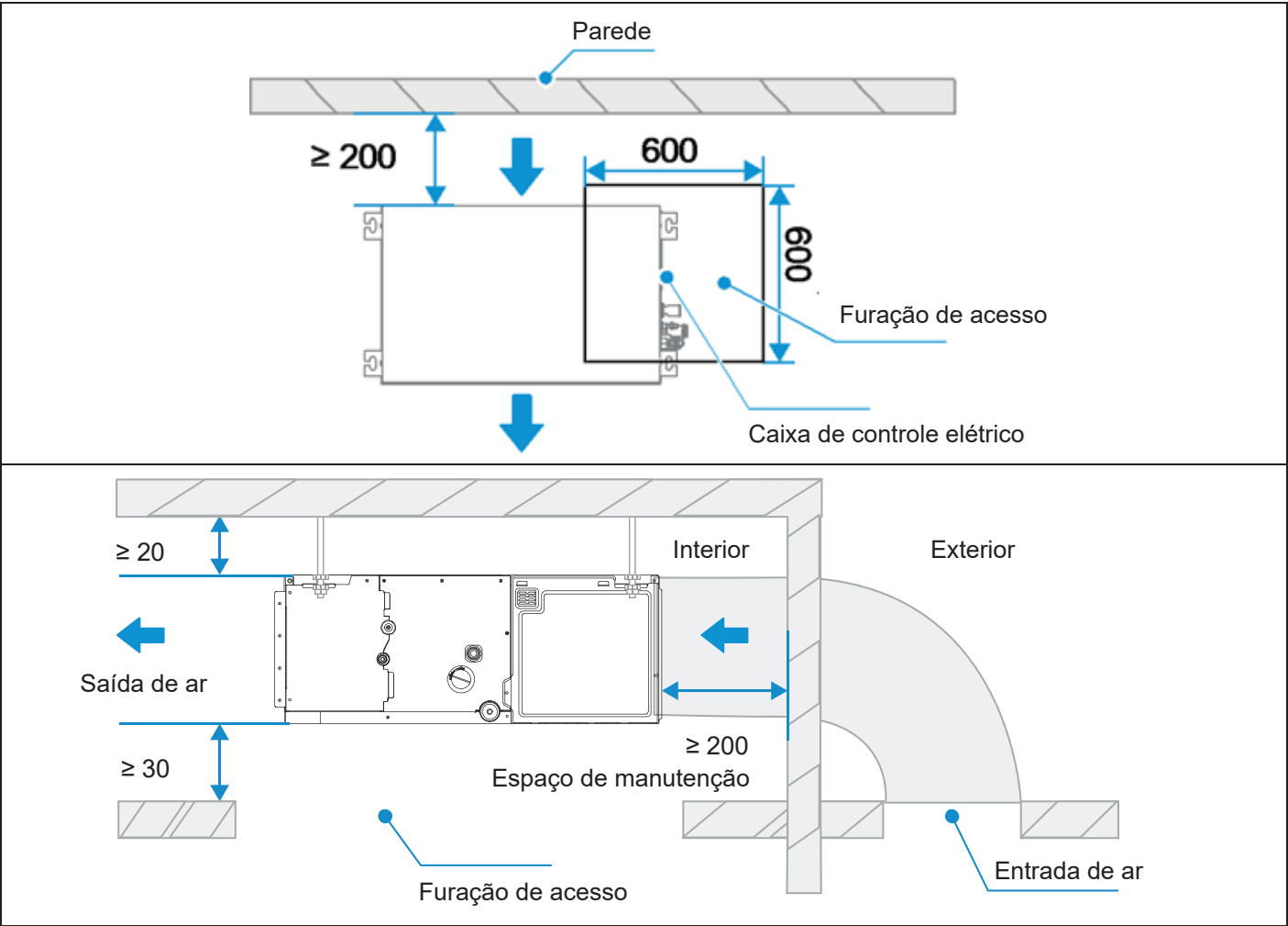
Figura 3.1: Requisitos de espaçamento da Unidade de Procesamento de Ar Externo Small (unidade: mm)
