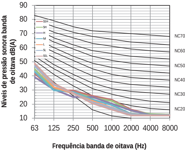
Figura 8.3: MIH22T3HN18 níveis banda de oitava
