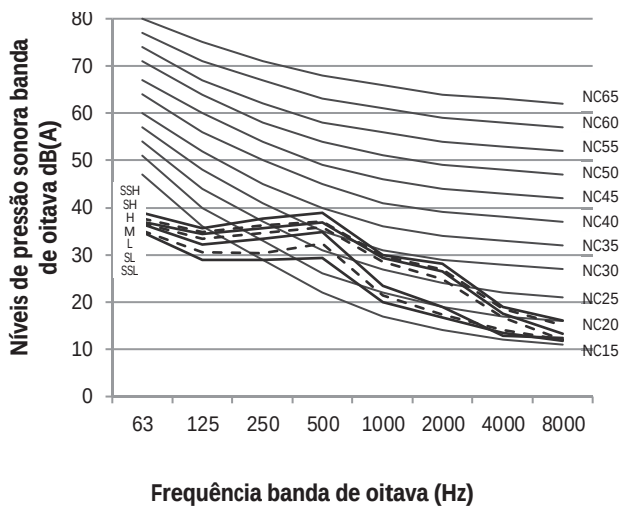
Figura 8.5: MIH-56Q2DHN1 níveis banda de oitava
