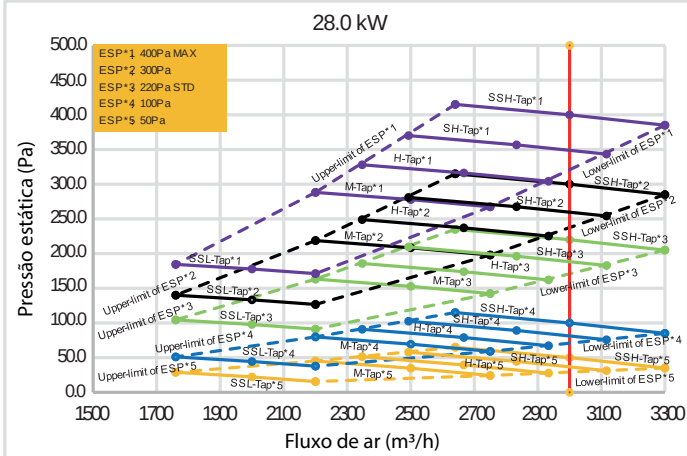
Figura 6.3: Performance do ventilador MIH280FAHN18
