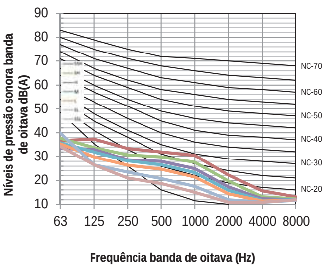
Figura 8.8: MIH56T2HN18 níveis banda de oitava
