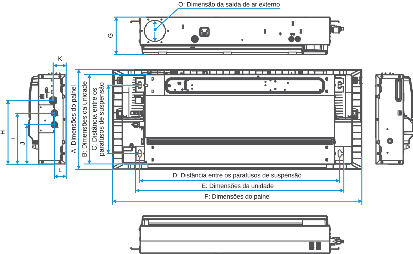
Figura 2.1: Dimensões modelos MIH18Q1HN18(A) até MIH71Q1HN18(A) (unidade: mm)
