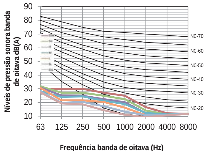
Figura 8.4: MIH22T2HN18 níveis banda de oitava
