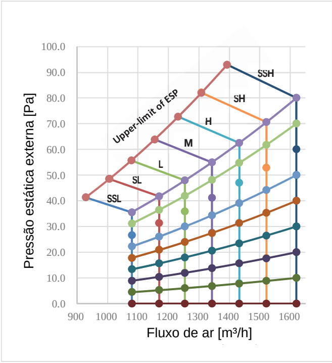
Figura 9.10: MIH112T3HN18
