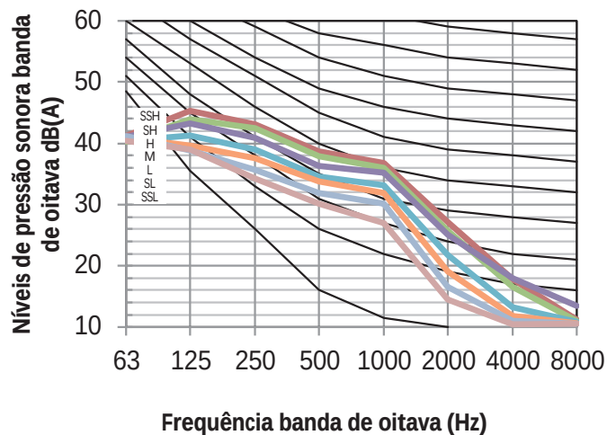
Figura 8.9: MIH100Q4HN18 níveis banda de oitava
