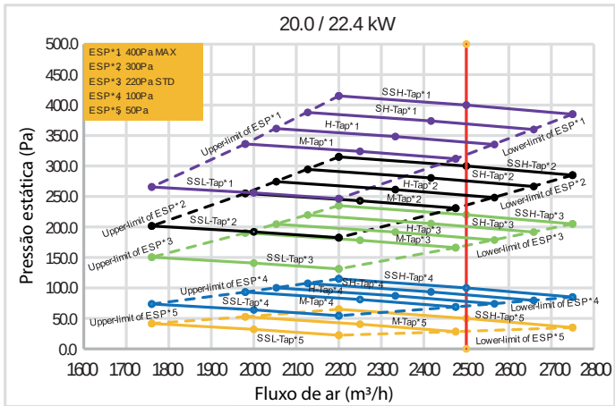
Figura 6.1: Performance do ventilador MIH200(224)FAHN18
