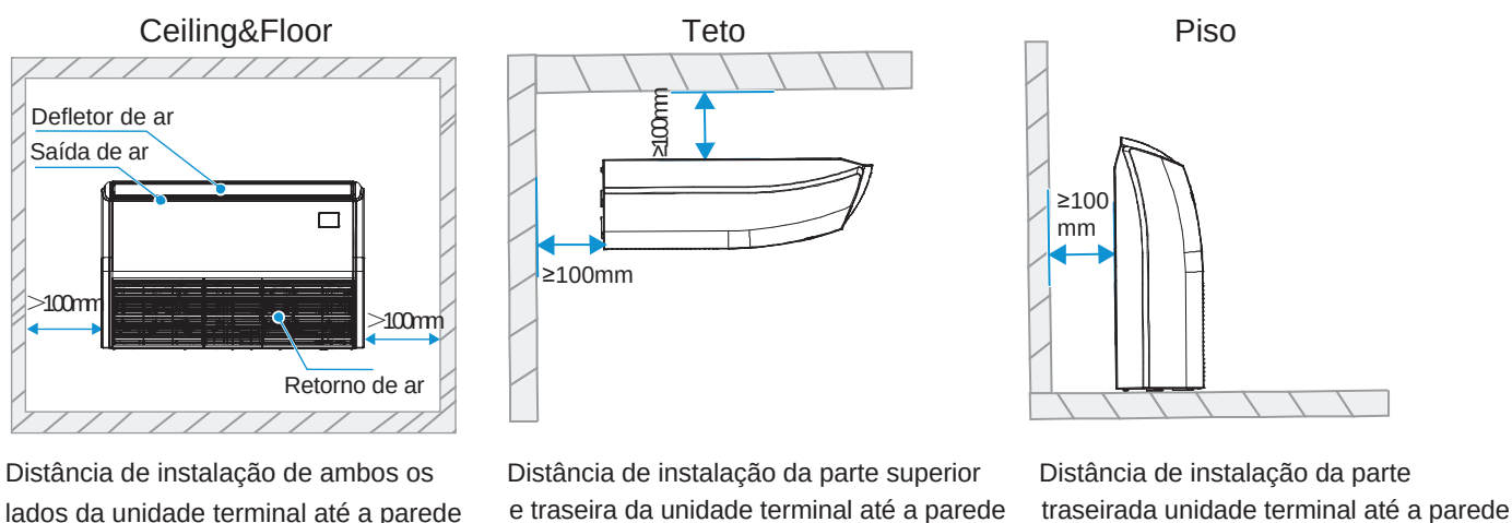
Figura 3.1: Requisitos de espaço para o Piso-Teto (unidade: mm)
