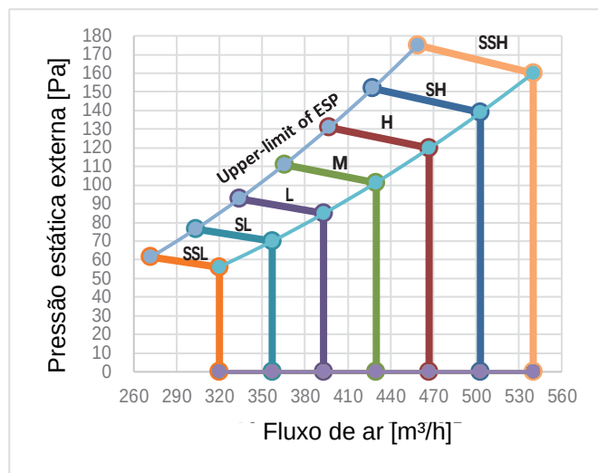
Figura 9.3: MIH28T2HN18
