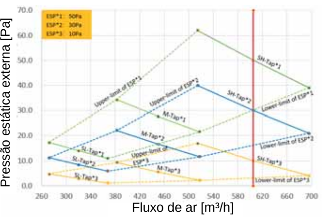
Figura 9.14: MIH36T3HN18
