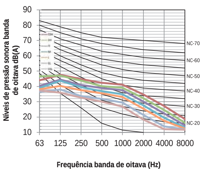
Figura 8.14: MIH160T2HN18 níveis banda de oitava
