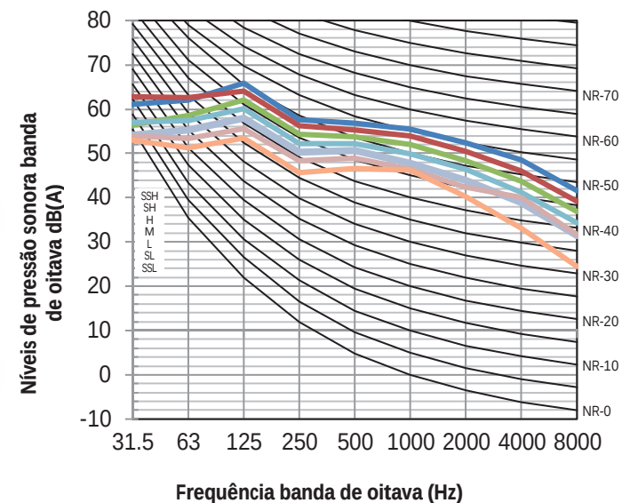
Figura 8.15: MIH560T1HN18 níveis banda de oitava
