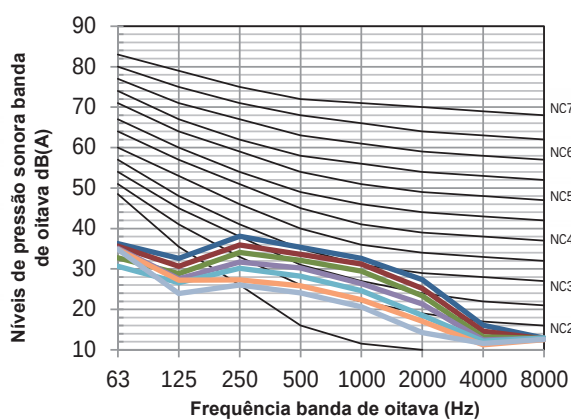
Figura 8.7: MIH56Q1DHN1(A) níveis banda de oitava
