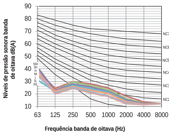
Figura 8.2: MIH36DLHN18 níveis banda de oitava
