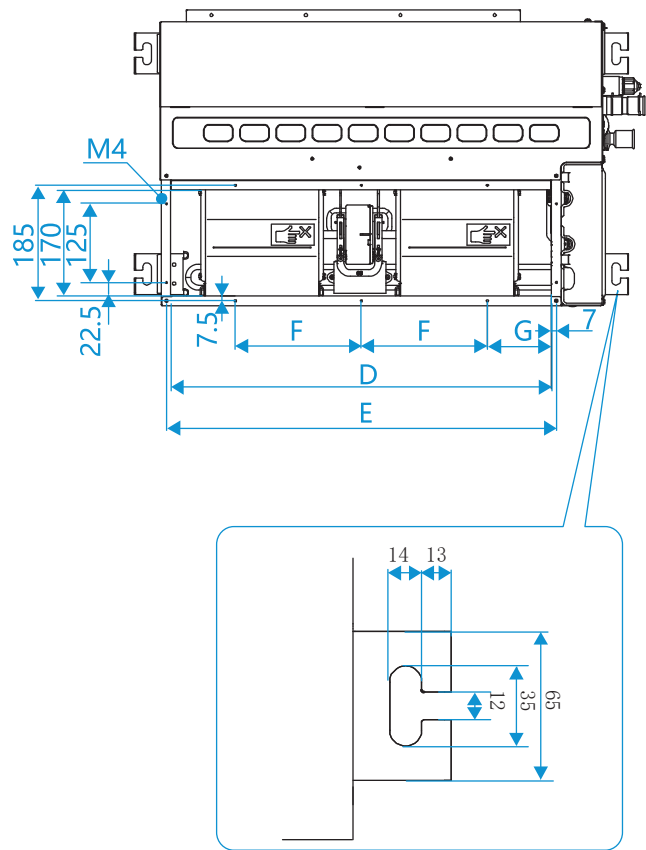
Figura 2.3: Dimensão da entrada de ar de retorno (modo de ar de retorno inferior) e distância entre as alças de elevação (unidade: mm)
