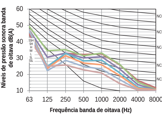
Figura 8.6: MIH45GHN18 níveis banda de oitava
