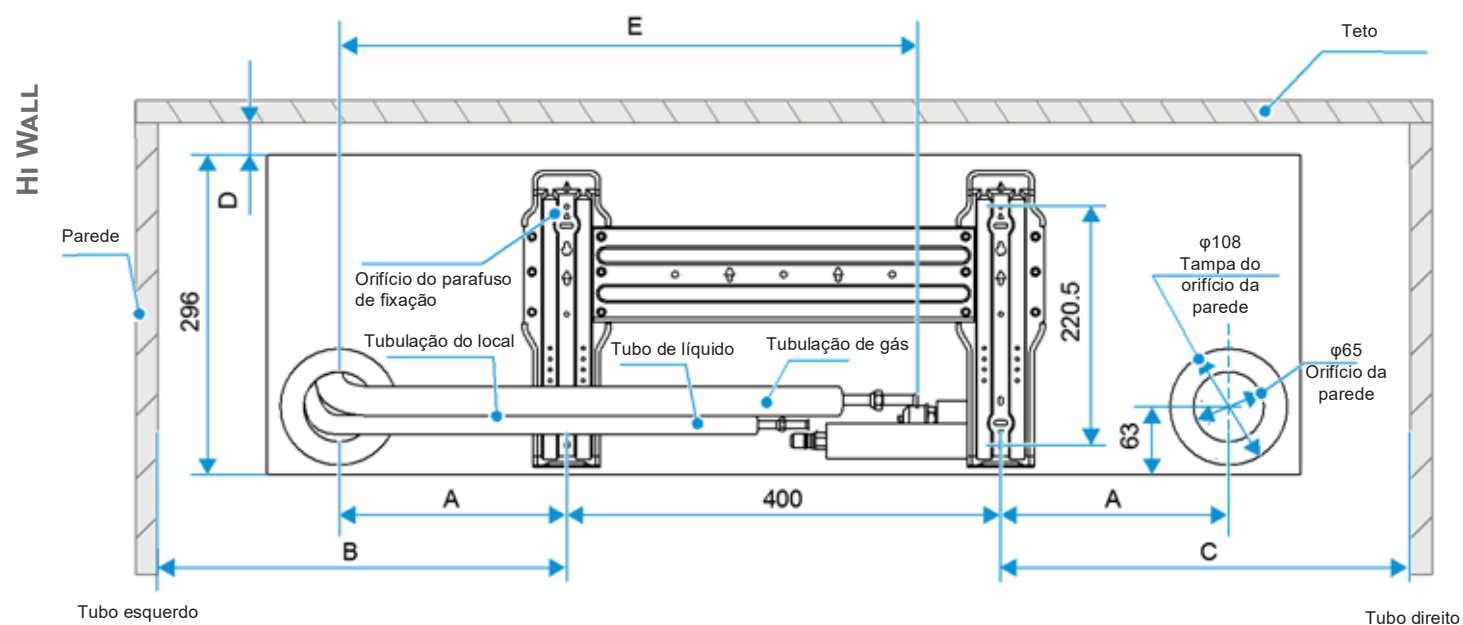
Figura 3.2: Posicionamento da placa de montagem
