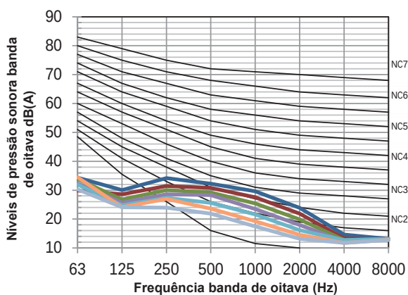
Figura 8.6: MIH45Q1DHN1(A) níveis banda de oitava
