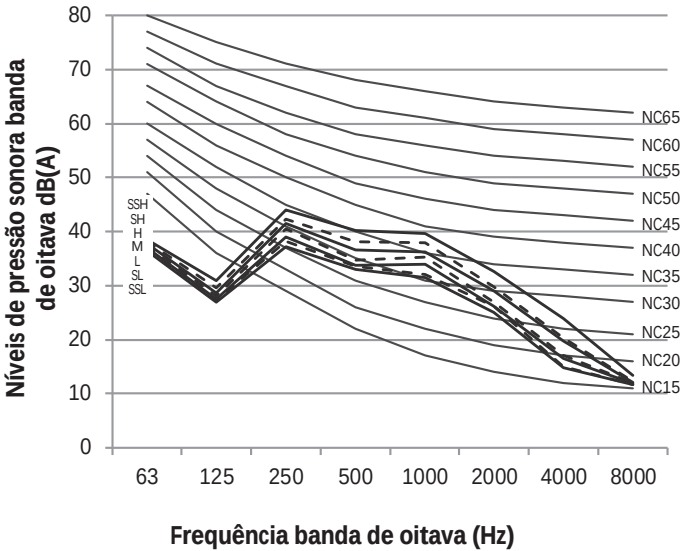
Figura 8.6: MIH-71Q1DHN1 níveis banda de oitava
