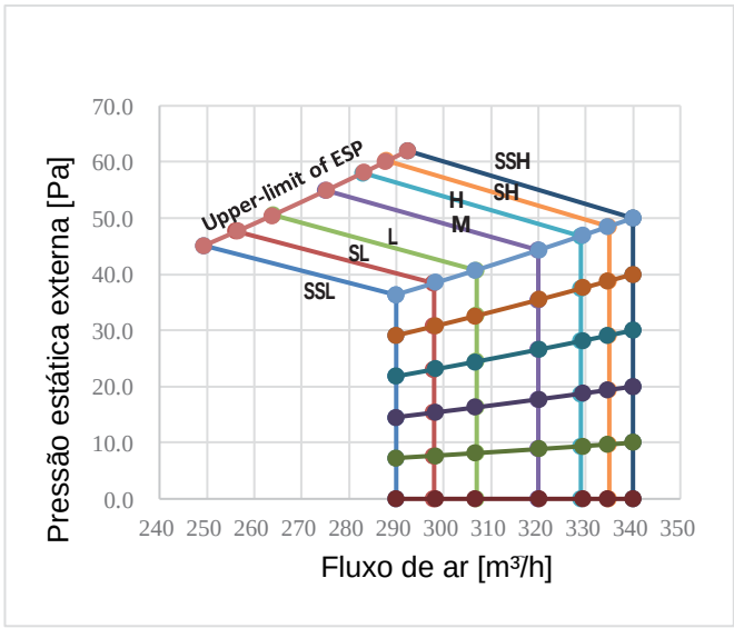
Figura 9.1: MIH15T3HN18
