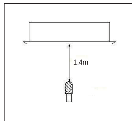
Figura 8.1: Medição do nível de pressão sonora do Cassete de Uma Via
