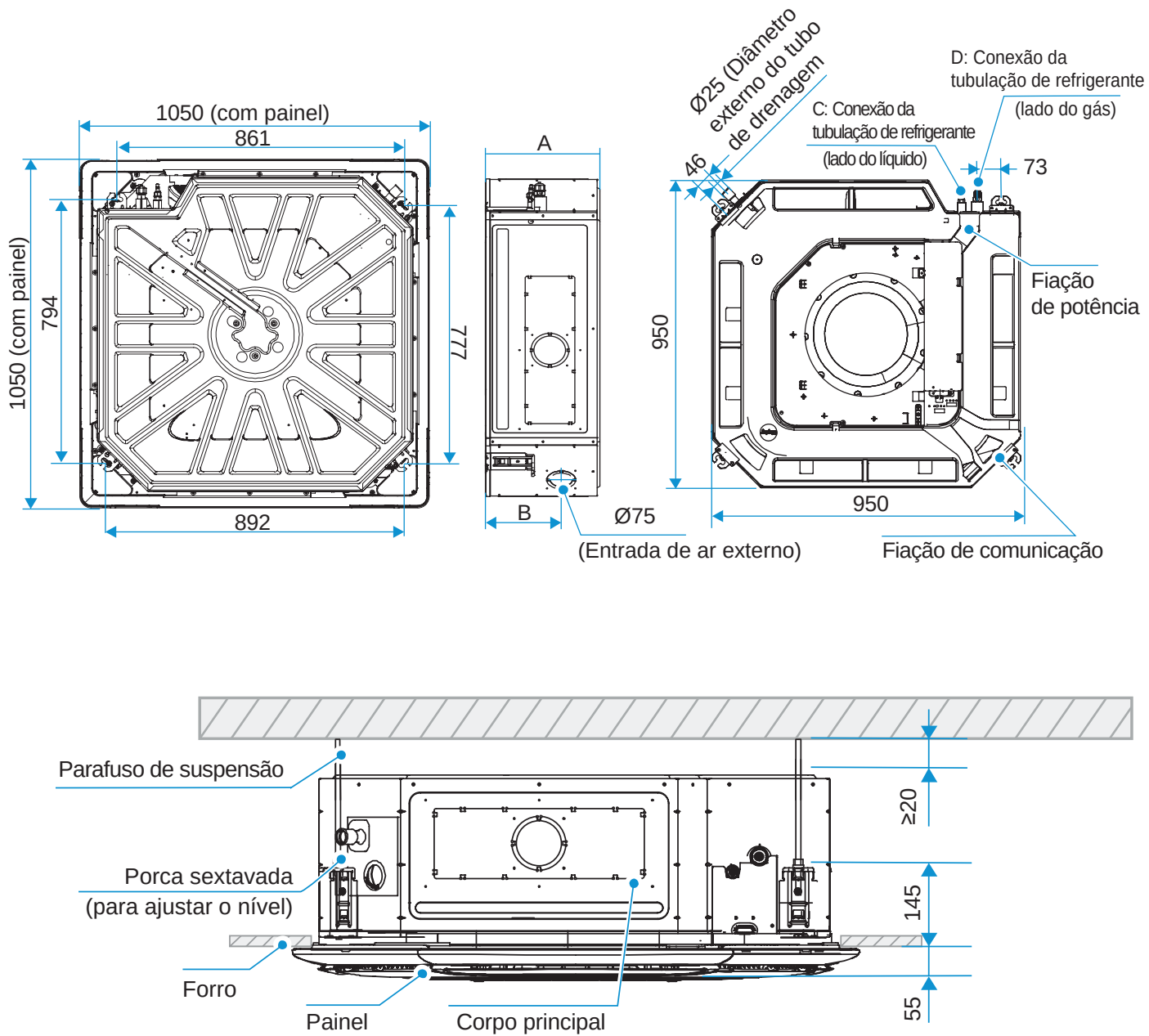
Figura 2.2: Dimensões do Cassete Quatro Vias de 16.0-18.0kW (unidade: mm)
