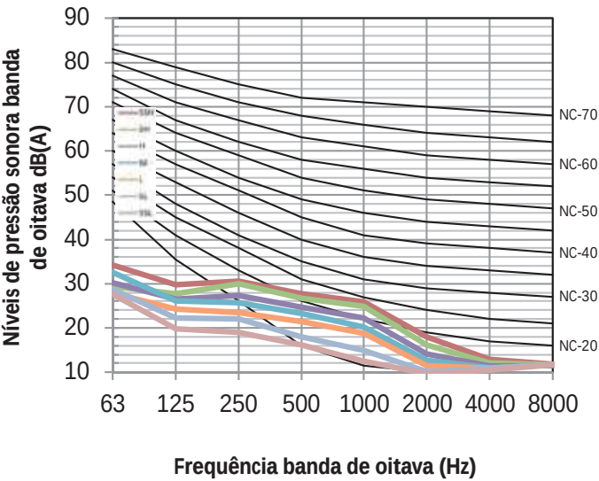
Figura 8.5: MIH28T2HN18 níveis banda de oitava
