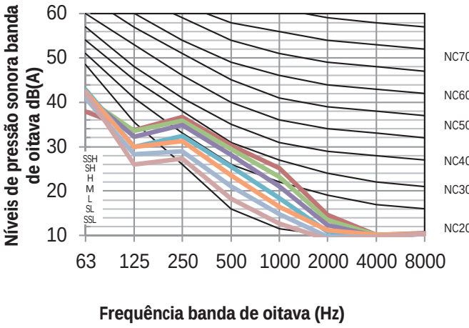
Figura 8.3: MIH36Q4HN18 níveis banda de oitava
