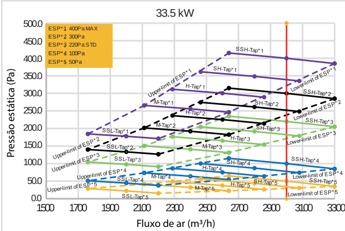
Figura 6.4: Performance do ventilador MIH335FAHN18
