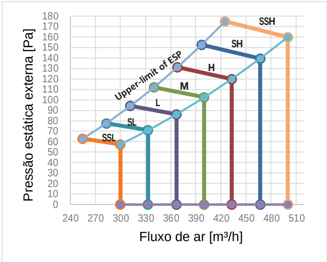
Figura 9.2: MIH22T2HN18
