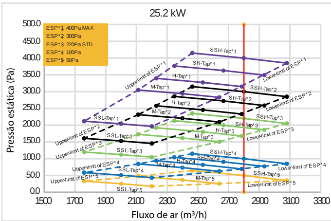
Figura 6.2: Performance do ventilador MIH252FAHN18
