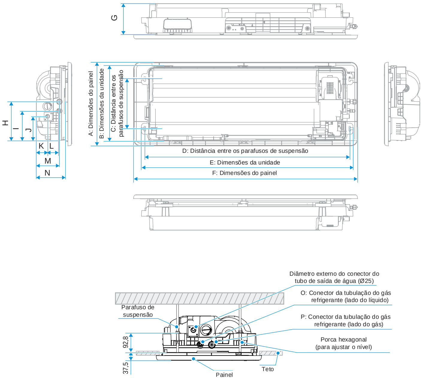
Figura 2.1: Dimensões modelos MIH18Q1HN18 até MIH71Q1HN18 (unidade: mm)
