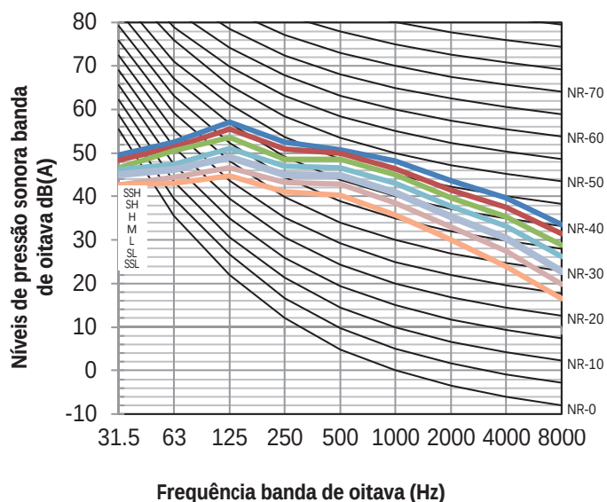
Figura 8.8: MIH200T1HN18 níveis banda de oitava
