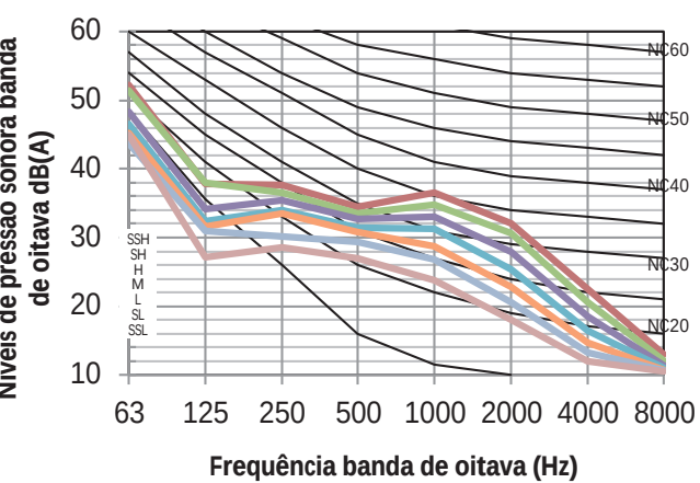
Figura 8.5: MIH36GHN18 níveis banda de oitava
