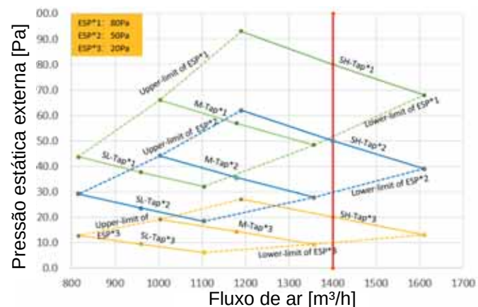
Figura 9.19: MIH90T3HN18
