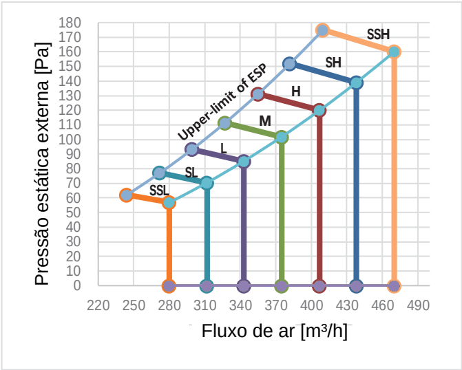
Figura 9.1: MIH15T2HN18
