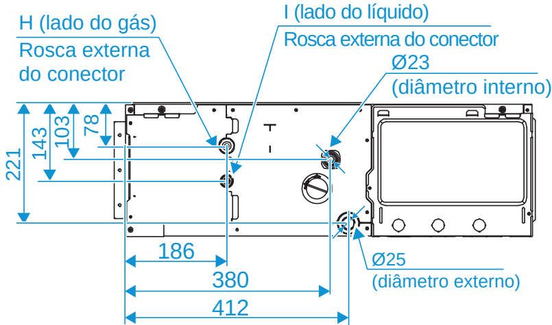
Figura 2.3: Conexões da tubulação de refrigerante e de drenagem da água (unidade: mm)
