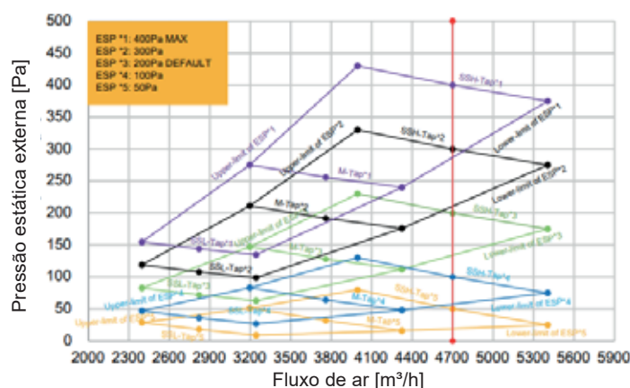
Figura 9.20: MIH560T1HN18
