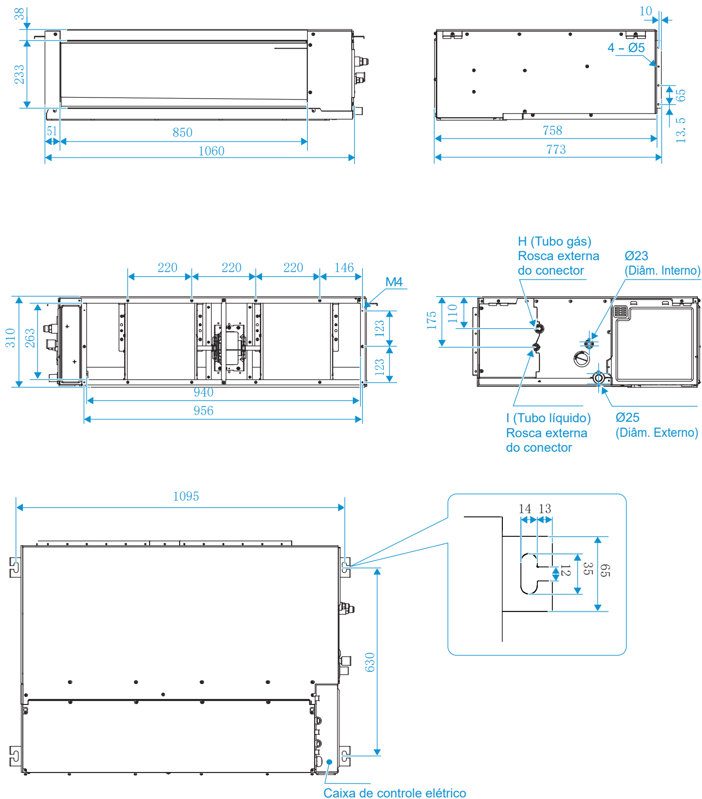
Figura 2.1: Dimensões modelos MIH90(140, 160)FASHN18 (unidade: mm)
