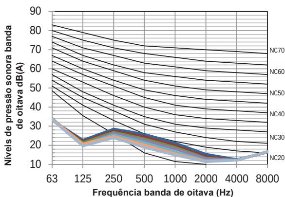
Figura 8.4: MIH28Q1DHN1(A) níveis banda de oitava
