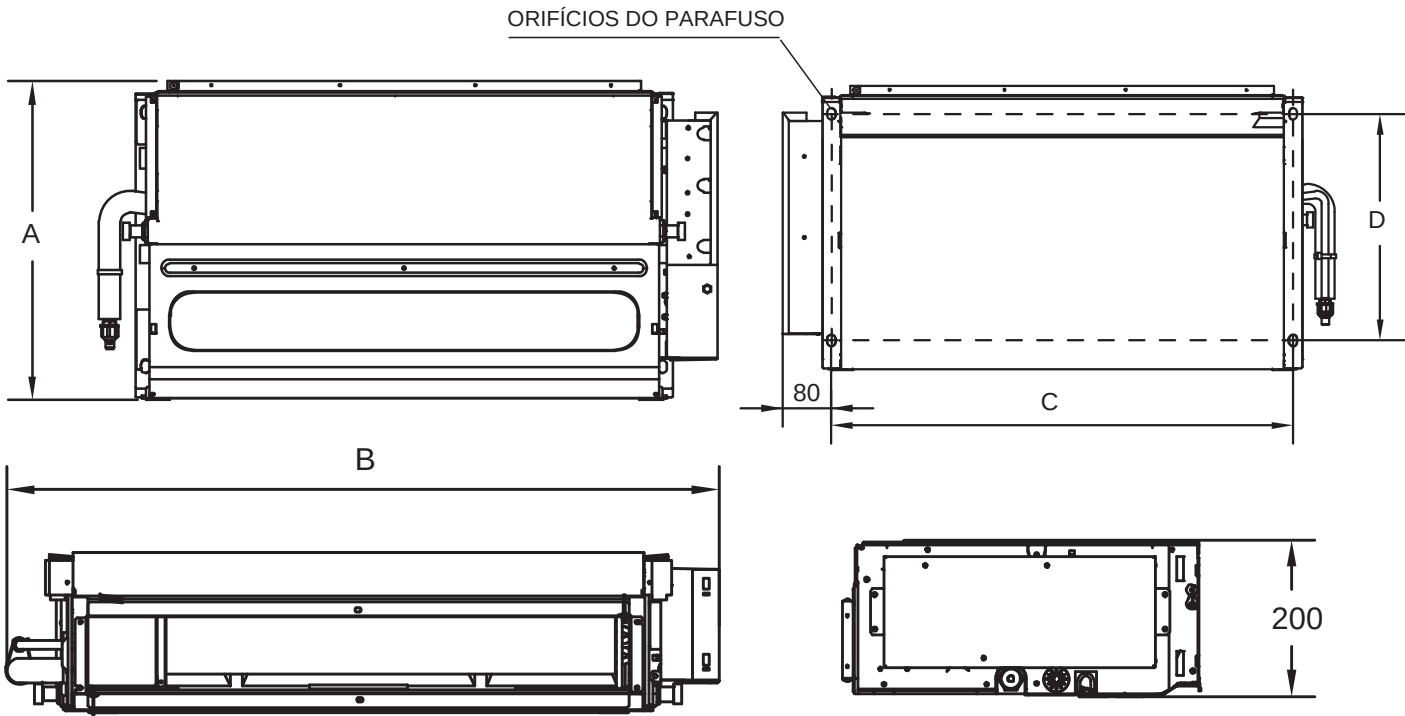
Figura 2.2: Dimensões da unidade de piso oculta da série F3 (unidade: mm)
