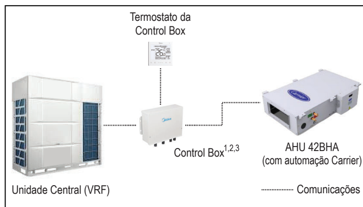
Diagrama de Conexões – Com controle e automação para VRF.
