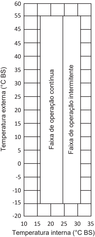
Figura 2-8.1: Limites de operação de refrigeração
