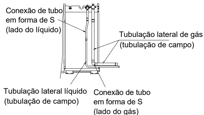
Figura 3-5.19: Método de conexão do tubo de saída para baixo.
