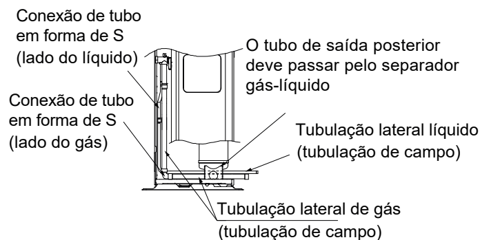
Figura 3-5.19: Método de conexão do tubo de saída para baixo.
