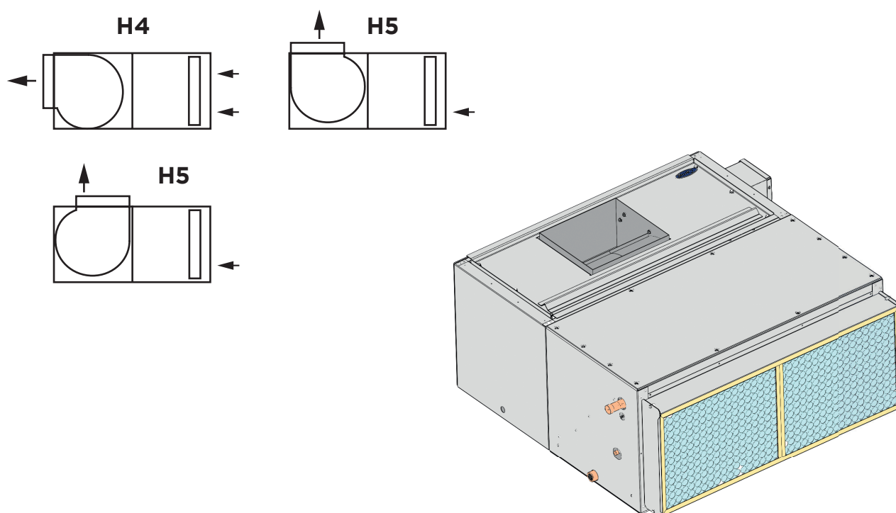
Fig. 7 - Posições de Montagem
