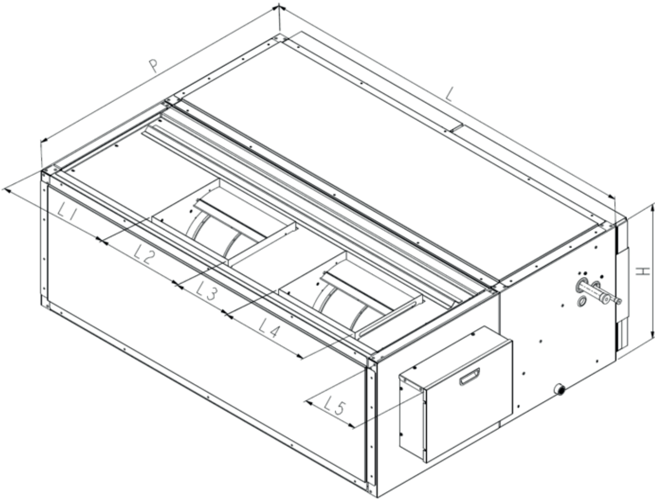
Unidades Evaporadoras 40MX - Configuração dos Módulos: Horizontal
