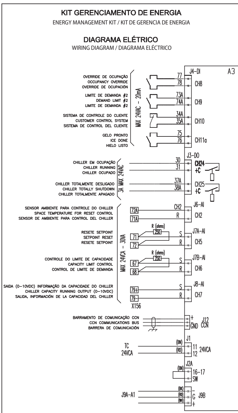
Fig. 21 - Kit gerenciamento de energia
