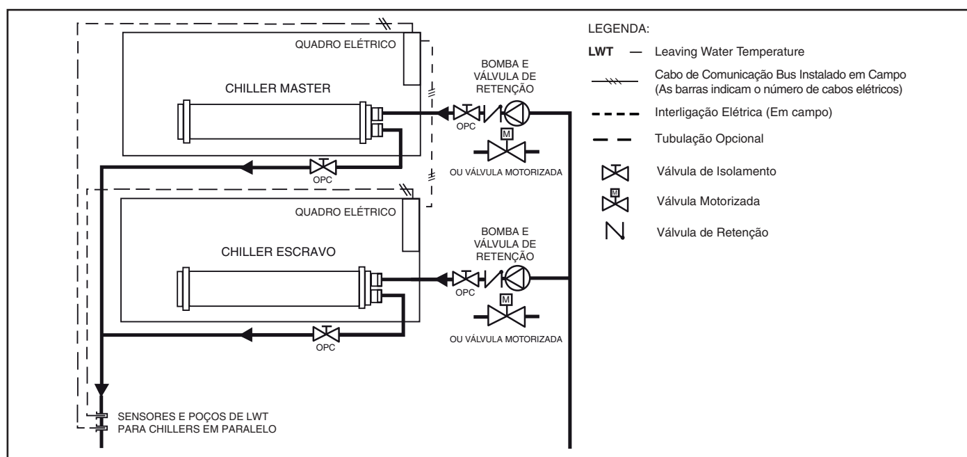
Fig. 15 - Operação de chillers duplos em paralelo
