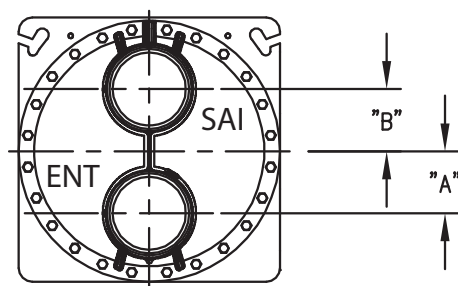
DESCARGA
