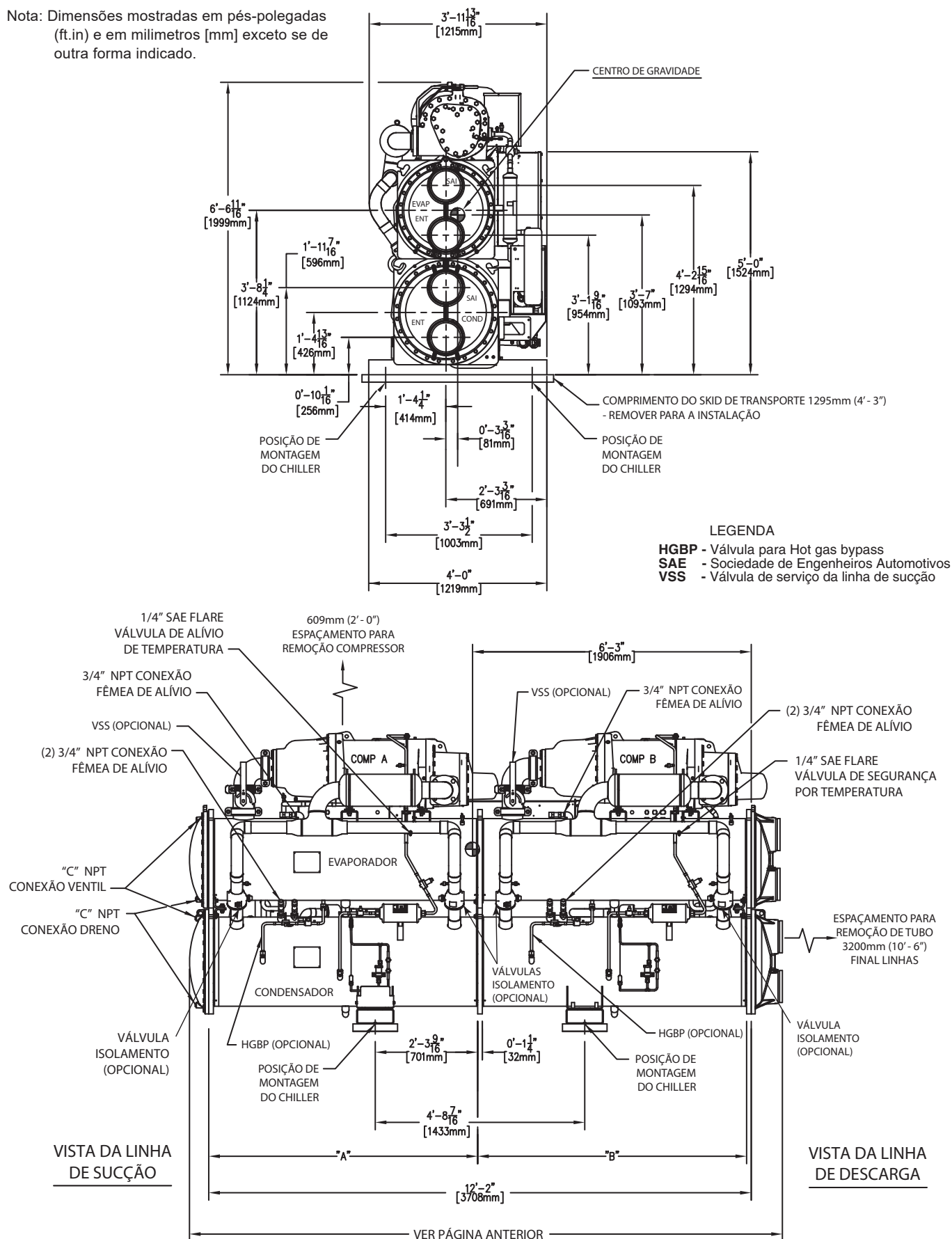
Fig. 4 – Dimensões Unidades 30XW325-400 (cont.)
