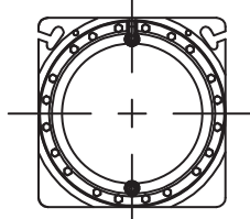
Fig. 2 – Dimensões Unidades 30XW150-200 (cont.)
