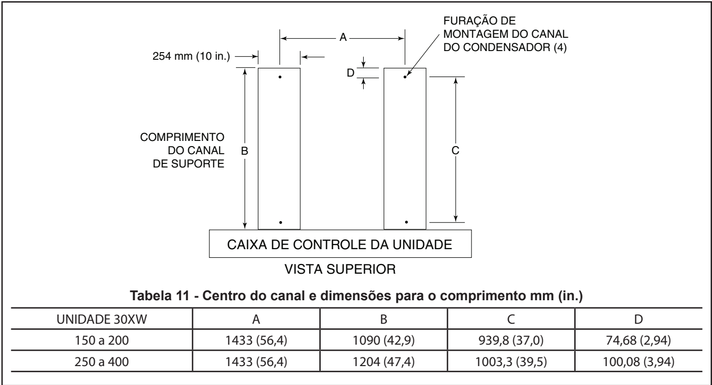
Fig. 24 - Dimensões do Canal do Condensador.
