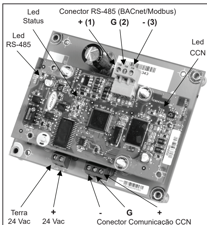
Fig. 20 - Placa Tradutor BACNet/Modbus
