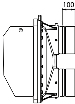
ADAPTADOR FLANGE-VICTAULIC
