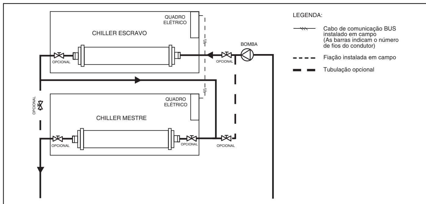
Fig. 16 - Operação de chillers duplos em série
