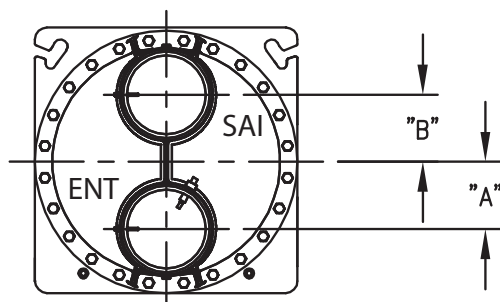
DESCARGA
