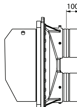
ADAPTADOR SOLDA-VICTAULIC
