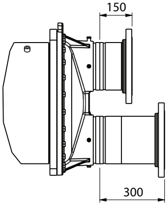
ADAPTADOR FLANGE-VICTAULIC
