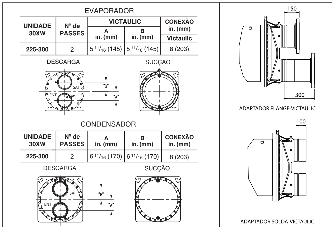
Fig. 3 – Dimensões Unidades 30XW225-300 (cont.)
