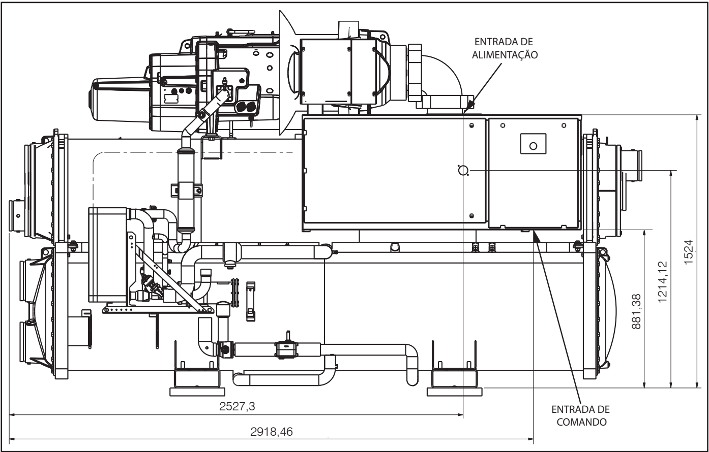
Fig. 2 – Dimensões da Caixa Elétrica - Unidades 30XW150-200 (cont.)
