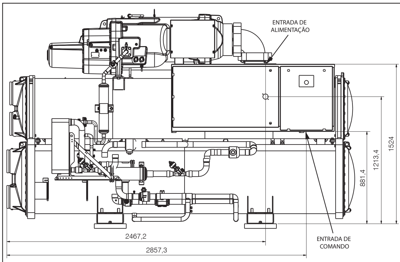
Fig. 3 – Dimensões da Caixa Elétrica - Unidades 30XW225-300 (cont.)
