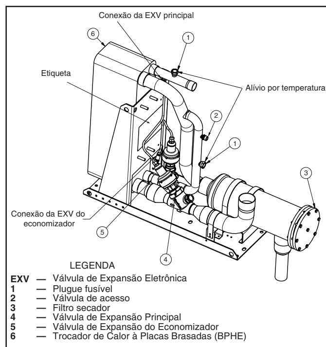
Fig. 13 – Montagem Típica do Economizador
