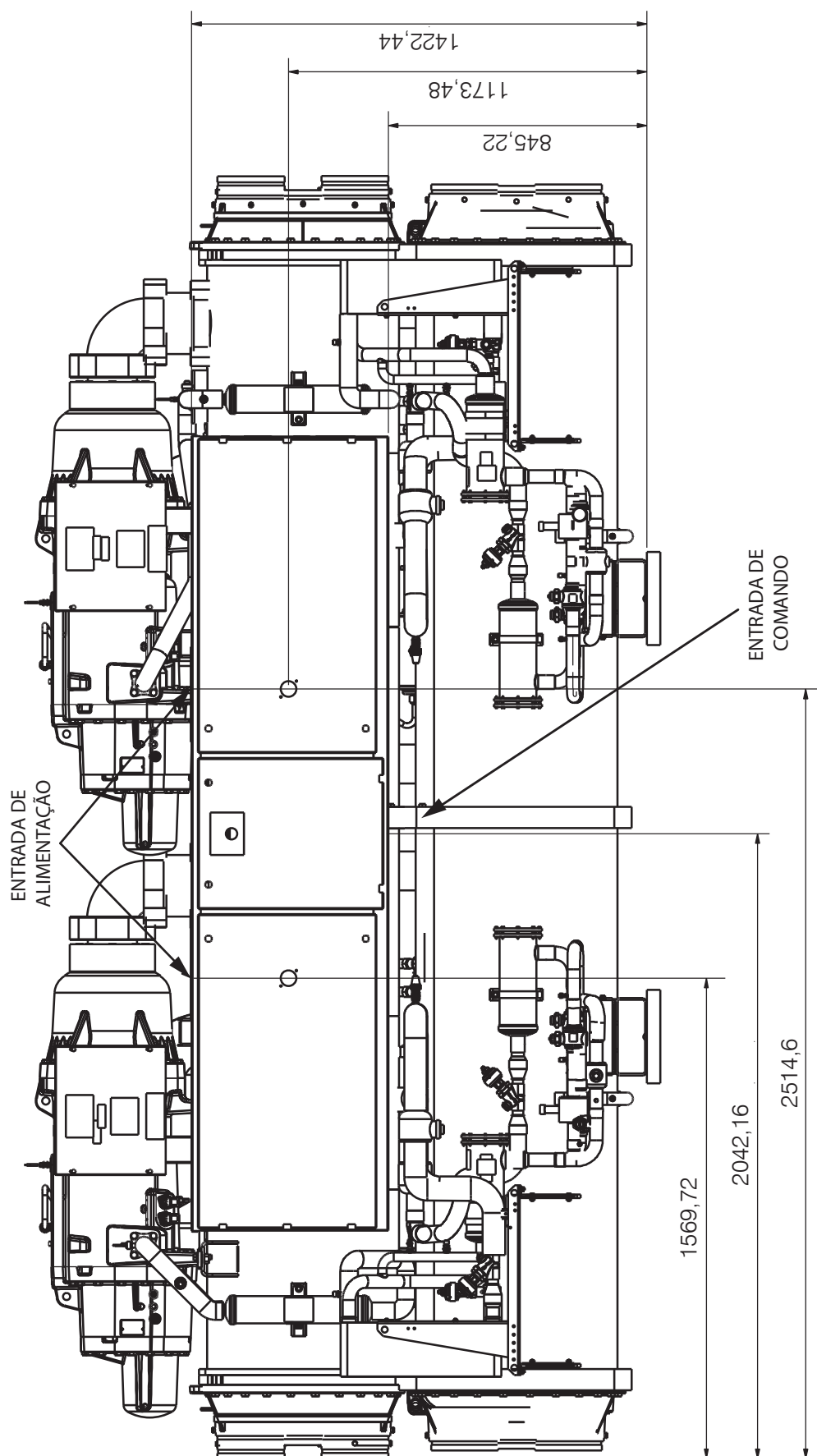
Fig. 4 – Dimensões da Caixa Elétrica - Unidades 30XW325-400 (cont.)
