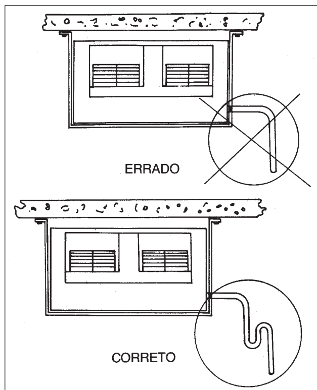
Figura 9 - Conexões para dreno
