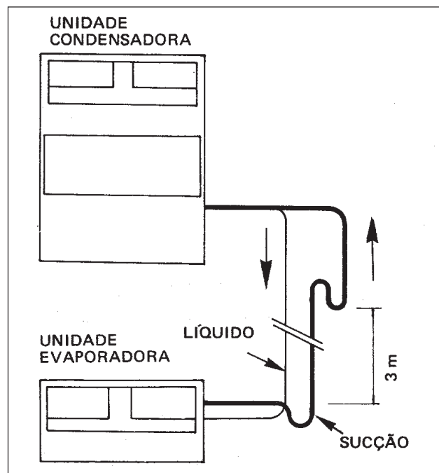
Figura 8b - Tubulações de refrigerante quando condensadora está acima da evaporadora.
