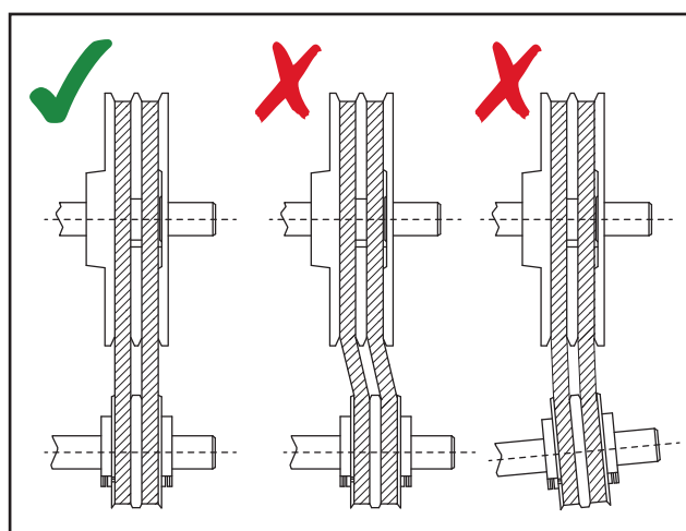
Figura 12 - Ajuste das polias
