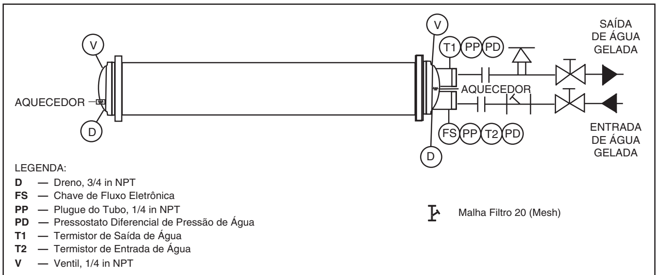
Figura 14- Diagrama de tubulação típica em unidades 30XS
