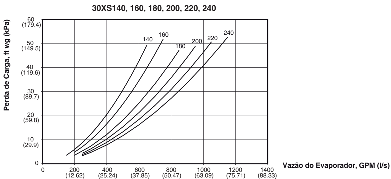
Gráficos das Curvas da queda de pressão no evaporador tipo padrão.
