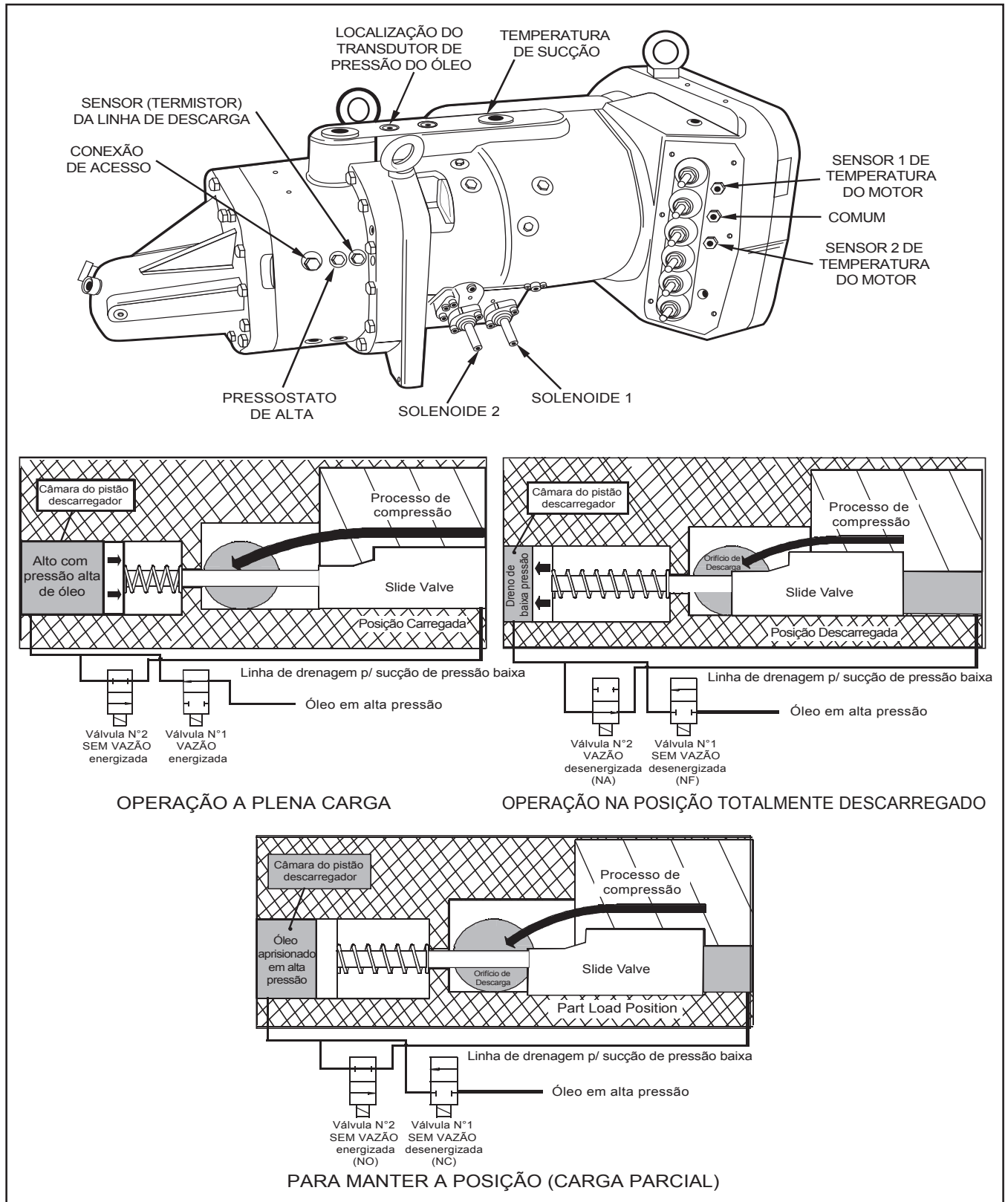
Figura 27 - Sistema de Óleo Típico (Todas Unidades)
