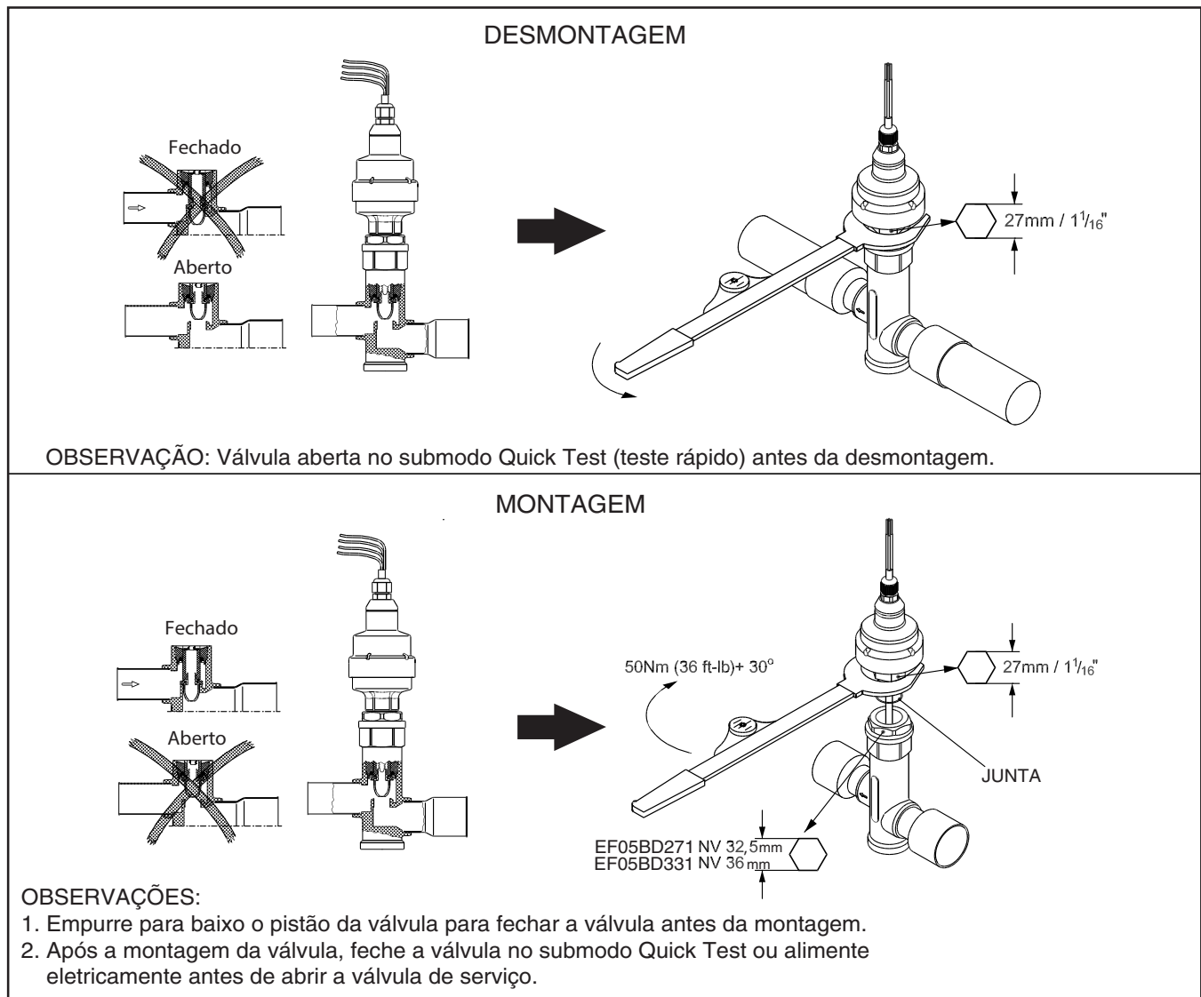
Figura 26 - Desmontagem e Montagem do Motor da EXV
