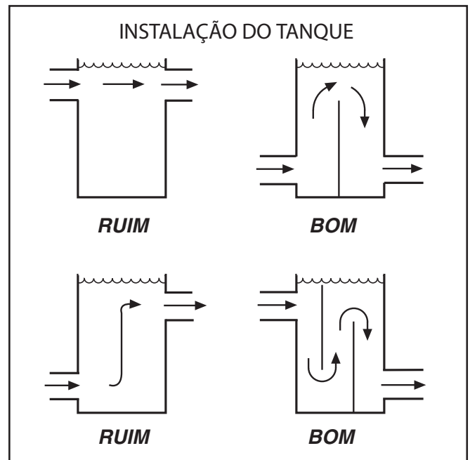
Figura 19 - Defletores do tanque
