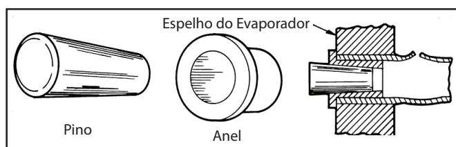
Figura 30 - Tubo Tampão Elliott
