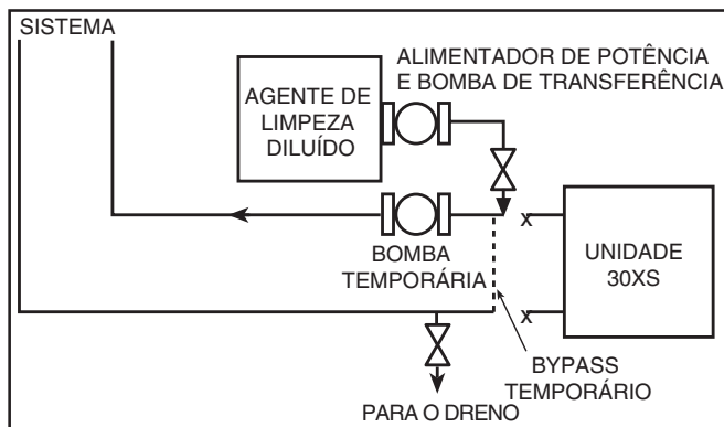
Figura 15 - Configuração Típica para o Processo de Limpeza
