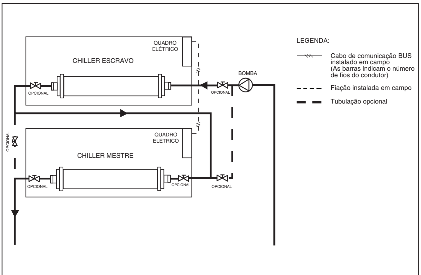
Figura 8 - Operação de chillers duplos em série
