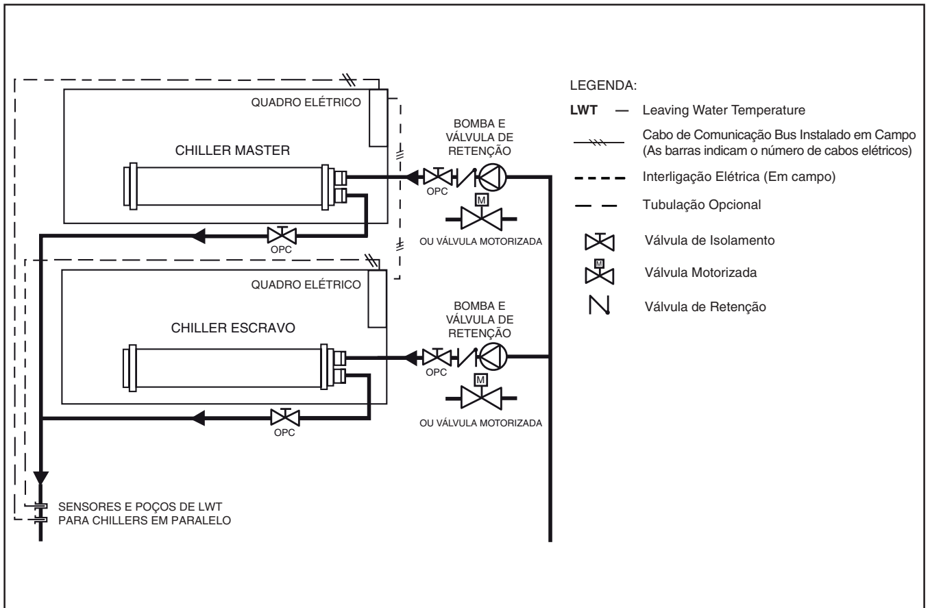
Figura 7 - Operação de chillers duplos em paralelo
