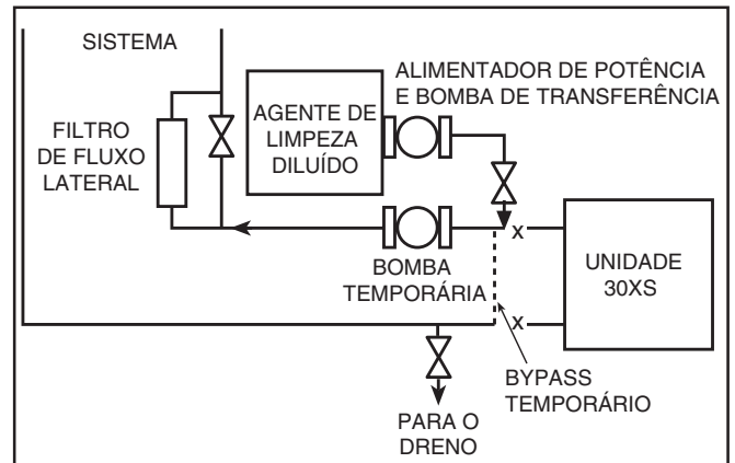
Figura 16 - Limpeza Utilizando um Filtro de Fluxo Lateral
