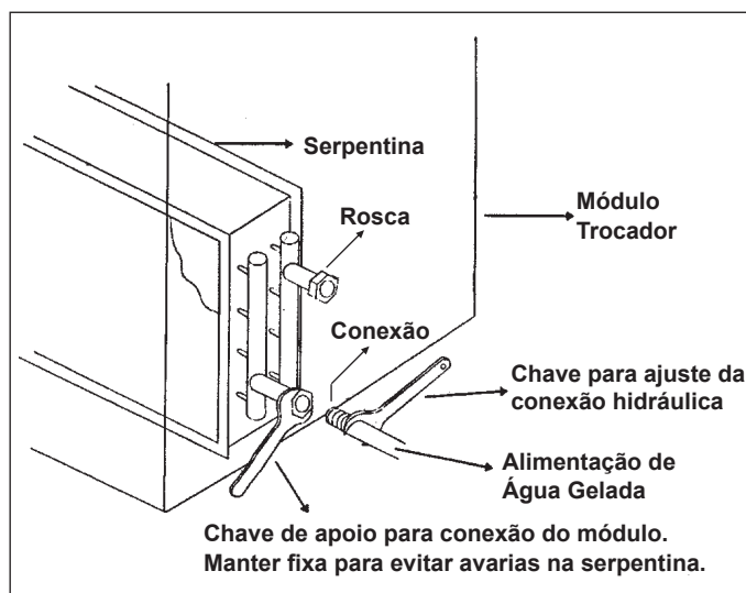
Fig. 3 - Ajuste das conexões
