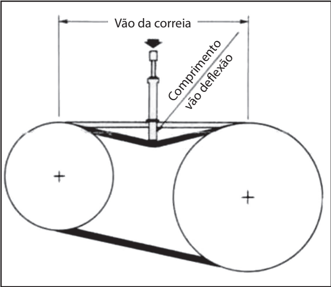
Fig. 15 - Ajuste tensão correia
