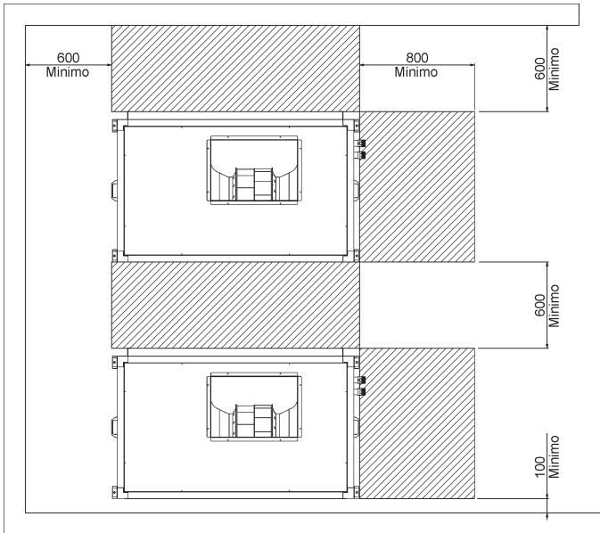
Disposição em Série
