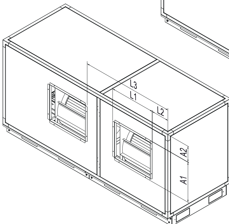
Dimensões do Bocal
