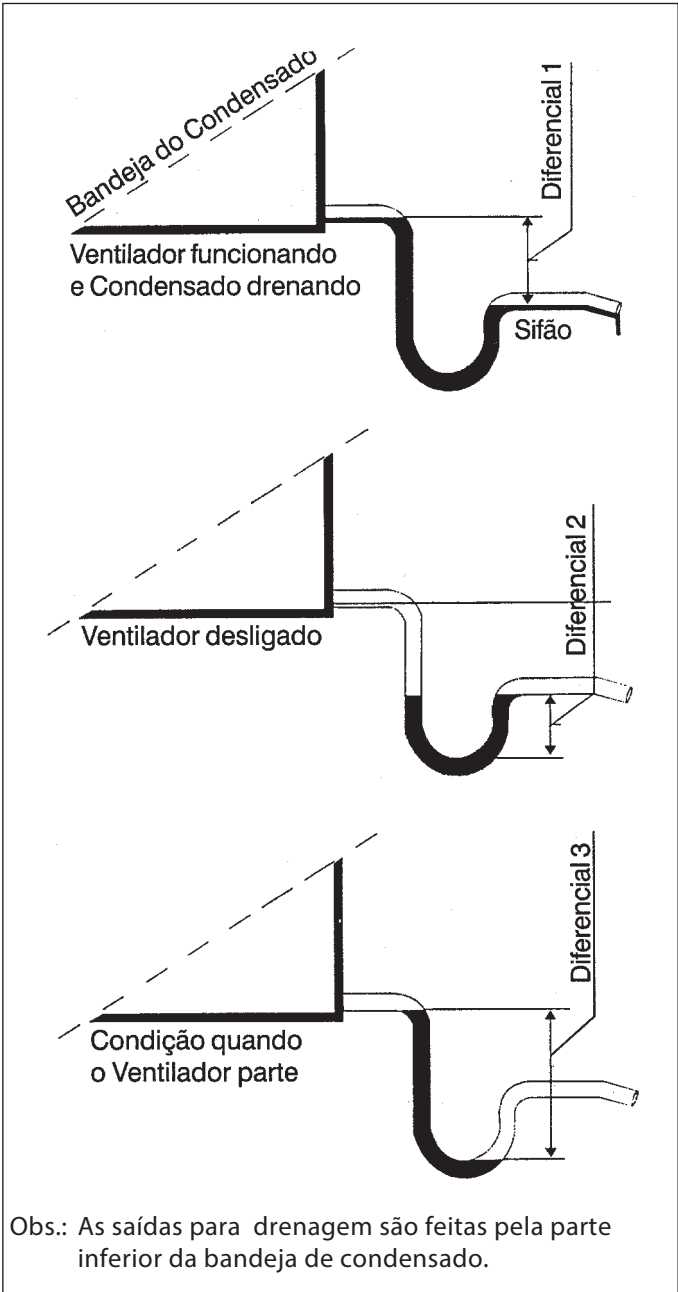
Fig. 4 - Saídas para drenagem - Figura meramente ilustrativa
