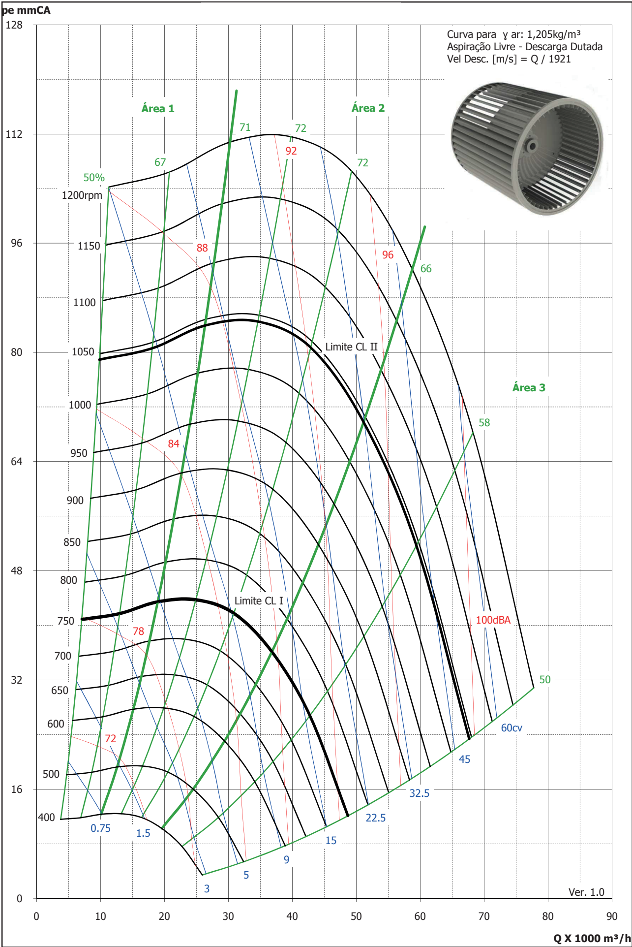
Curva de vazão dos ventiladores - Sirocco 2 x 18-18
