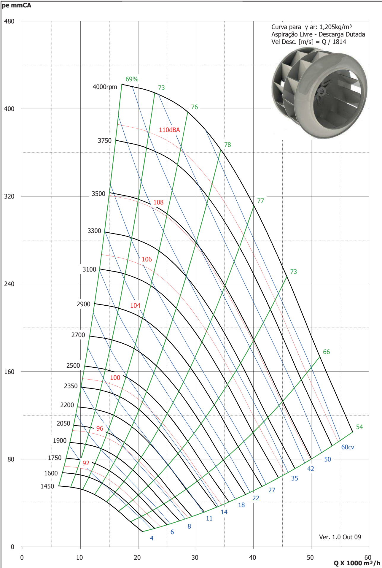
Curva de Vazão dos Ventiladores - Limit Load D400
