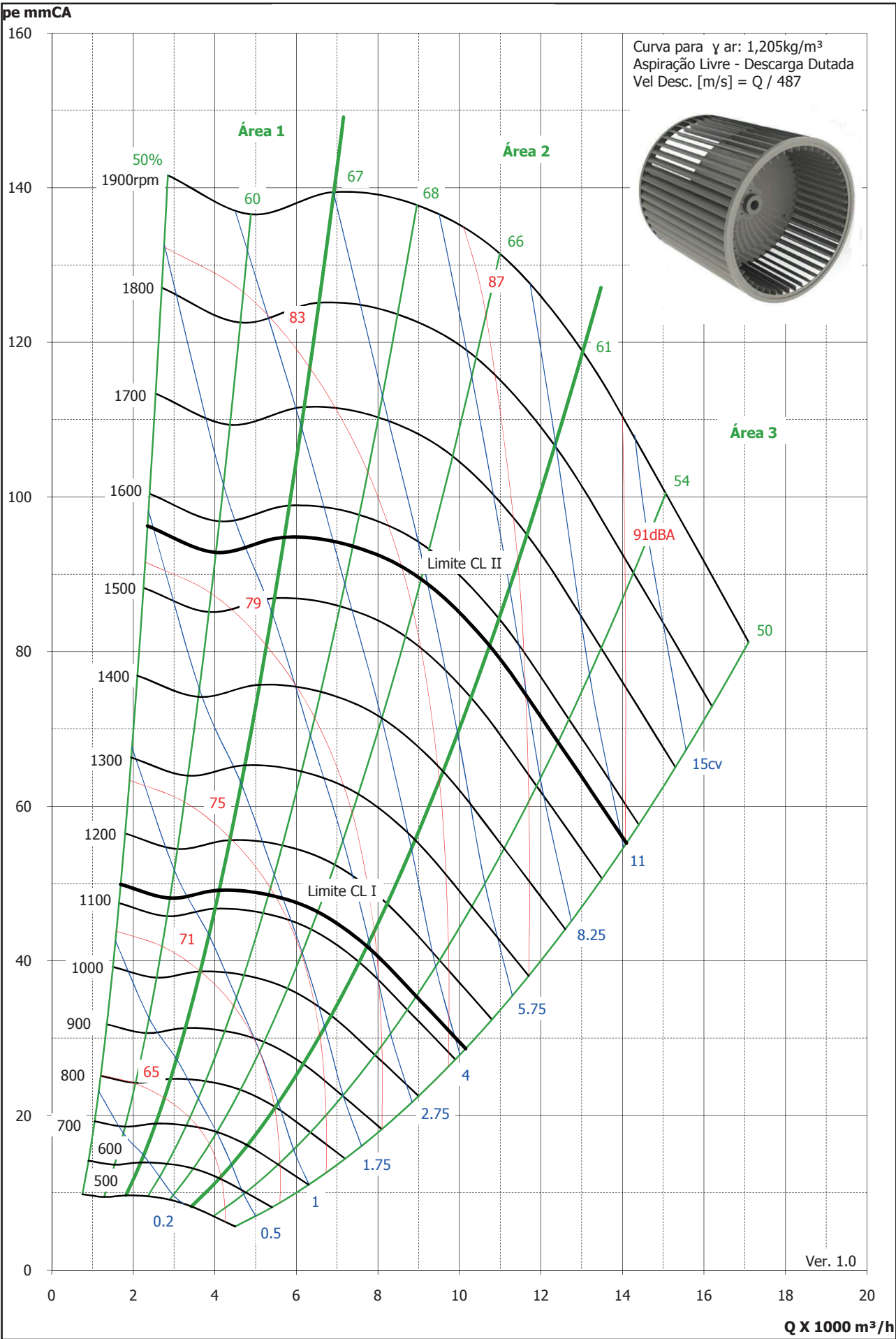
Curva de vazão dos ventiladores - Sirocco 12-12
