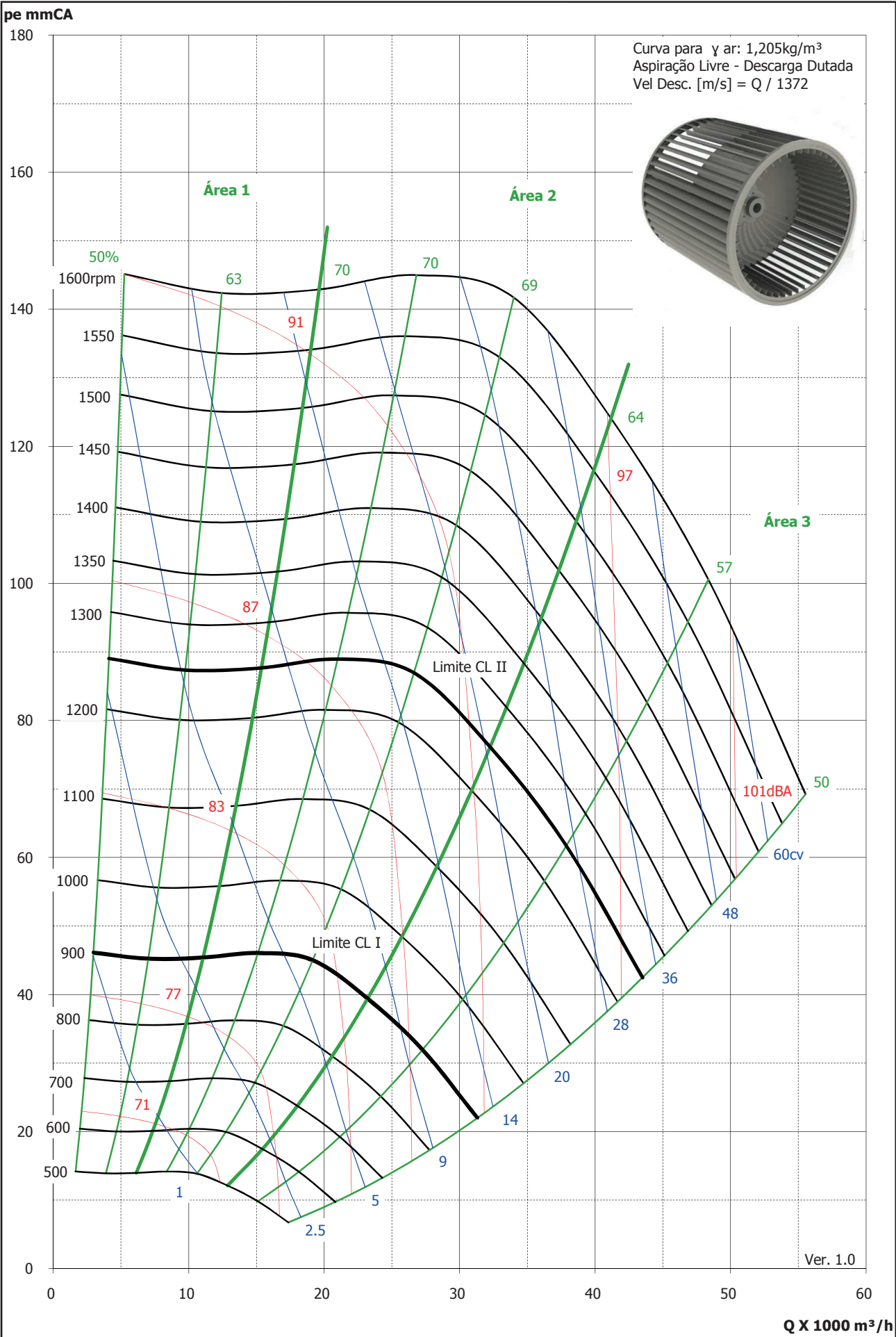
Curva de vazão dos ventiladores - Sirocco 2 x 15-15
