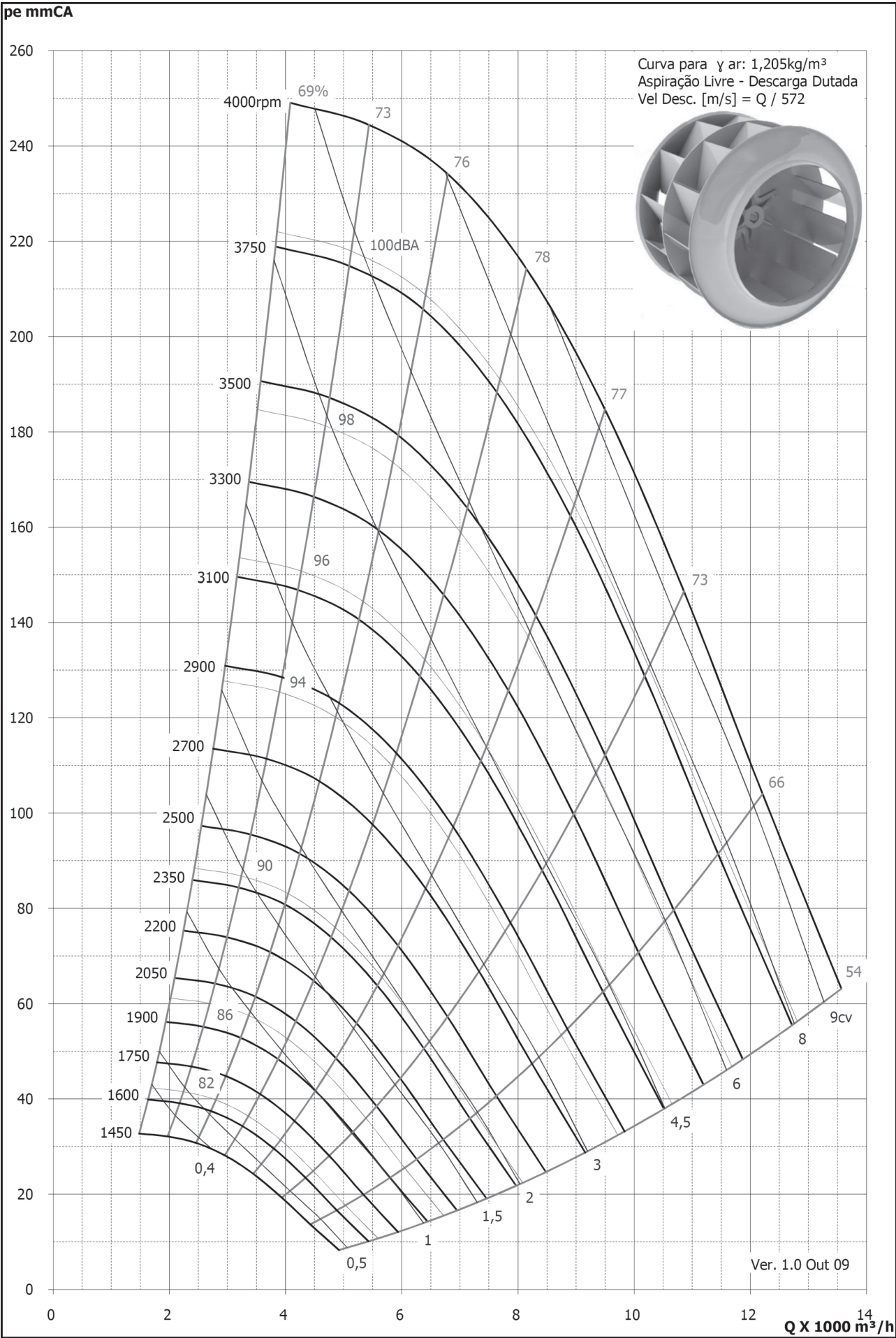
Curva de Vazão dos Ventiladores - Limit Load D315
