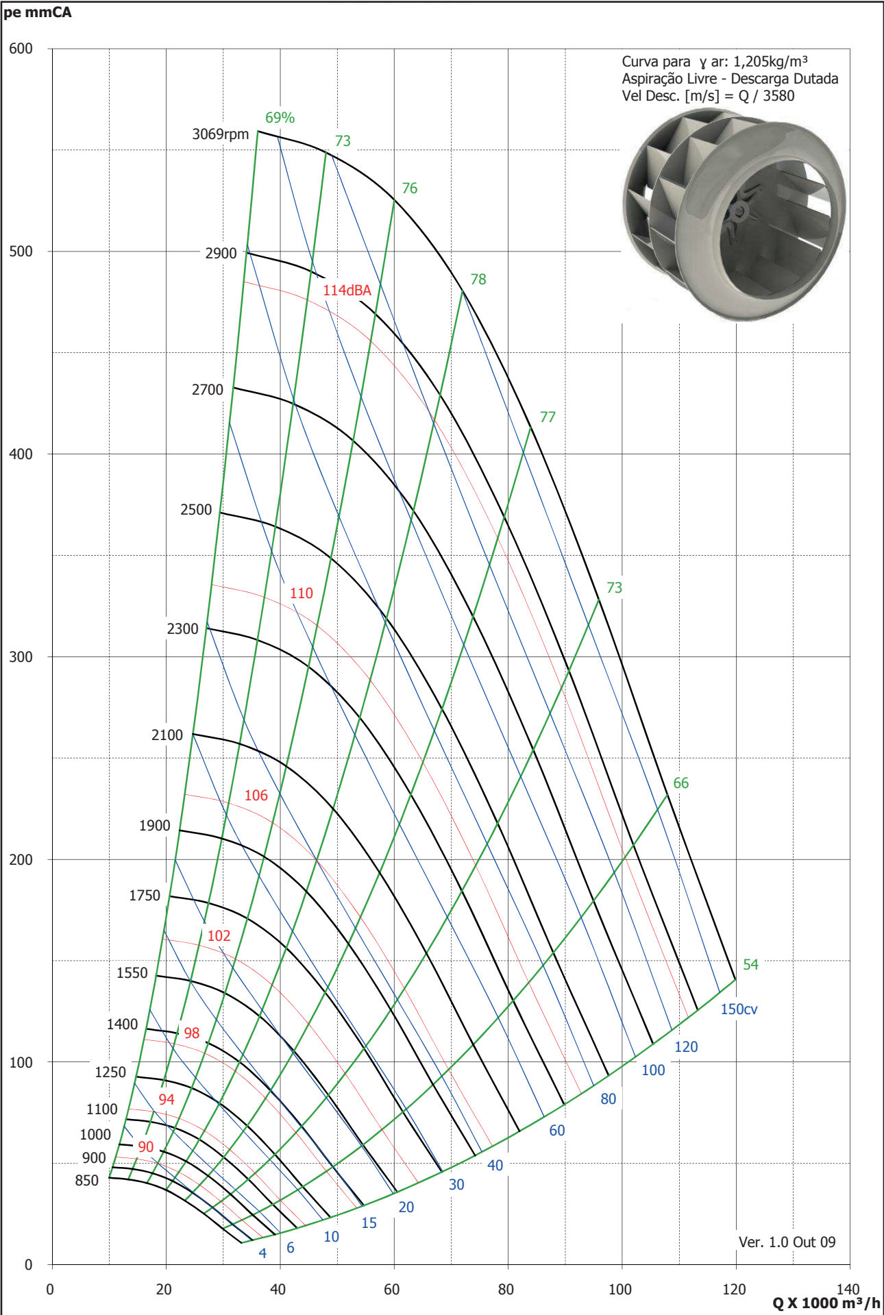
Curva de Vazão dos Ventiladores - Limit Load 2 x D560
