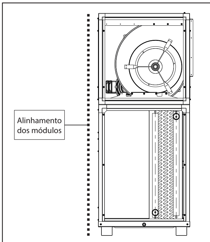
Figura 7 - Alinhamento de montagem dos módulos
