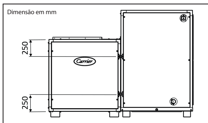
Fig. 17a - Distância entre os pontos de fixação montagem horizontal - Módulos Ventilador e Trocador
