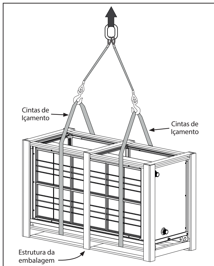
Fig. 4 - Indicação típica para içamento de módulos com a estrutura da embalagem
