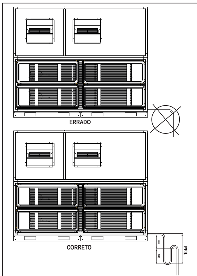
Figura 21 - Conexões para dreno
