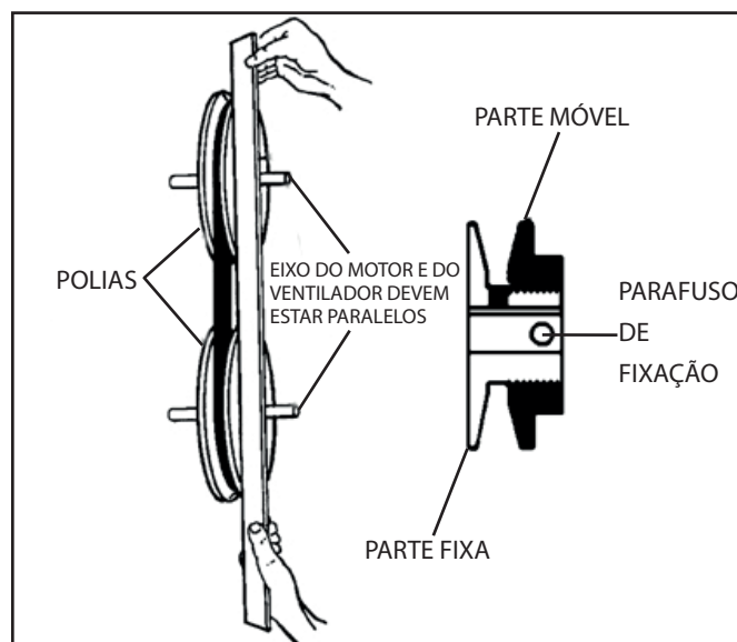
Figura 4 - Ajuste das polias.
