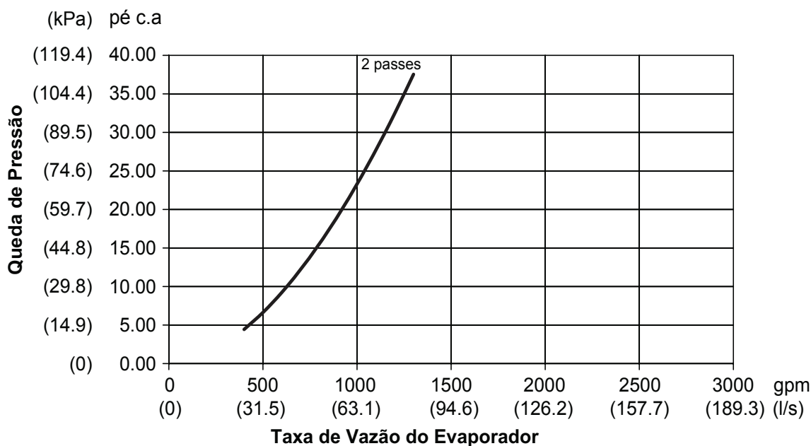
30XW325-400 EVAPORADOR
