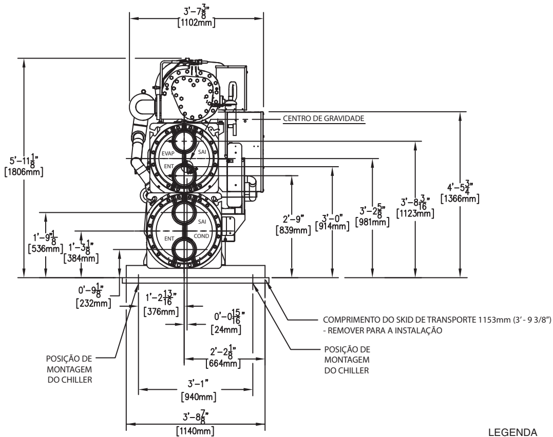
DIMENSÕES DA UNIDADE 30XW150-200 (cont.)
