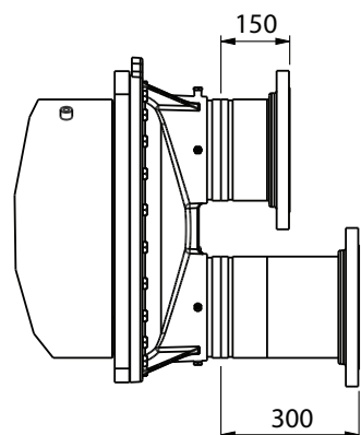
ADAPTADOR FLANGE-VICTAULIC
