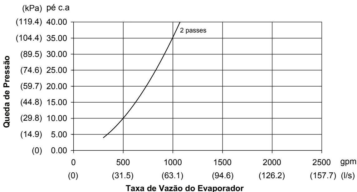
30XW225-300 EVAPORADOR
