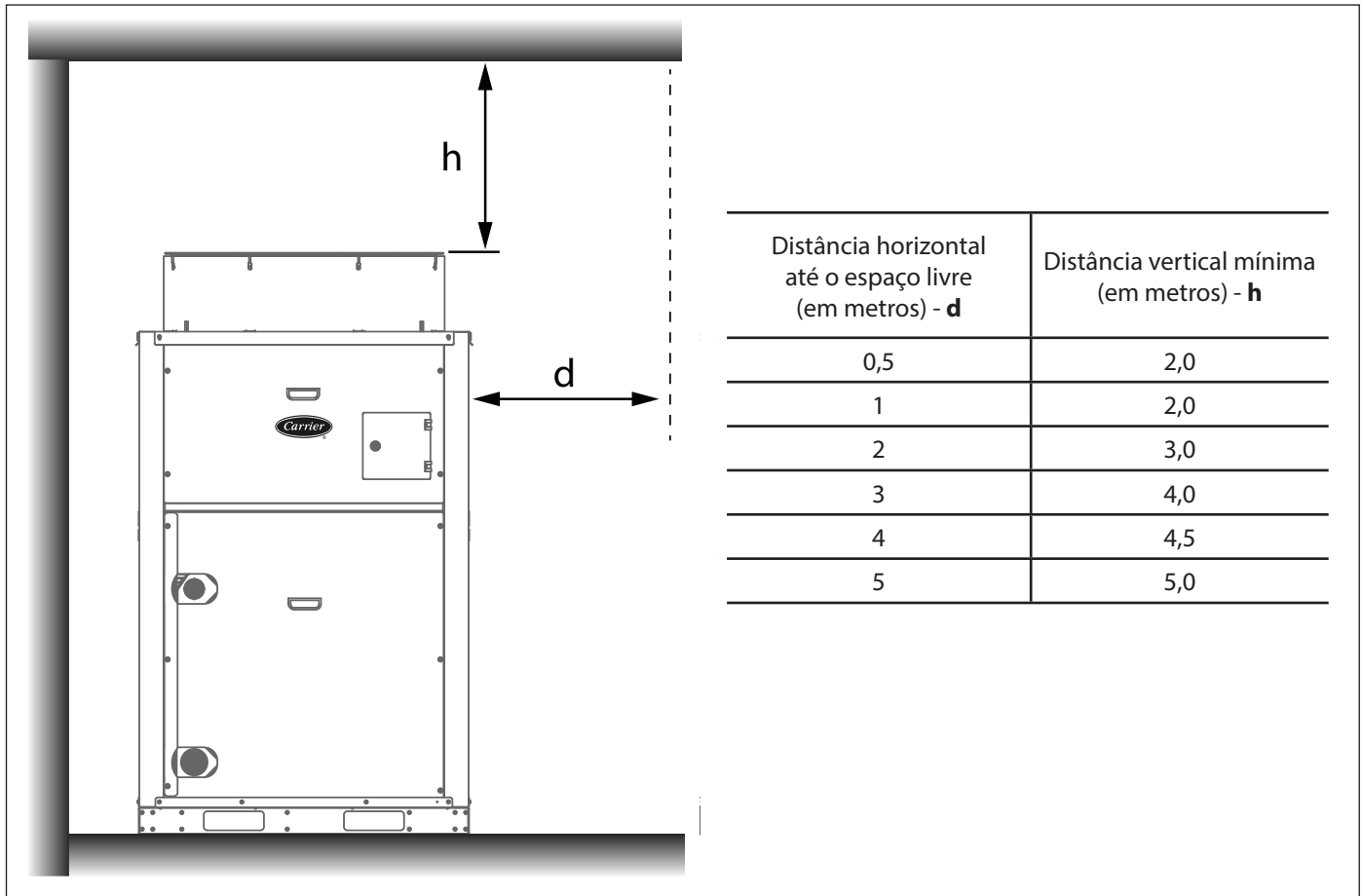
Figura 15 - Espaços mínimos
