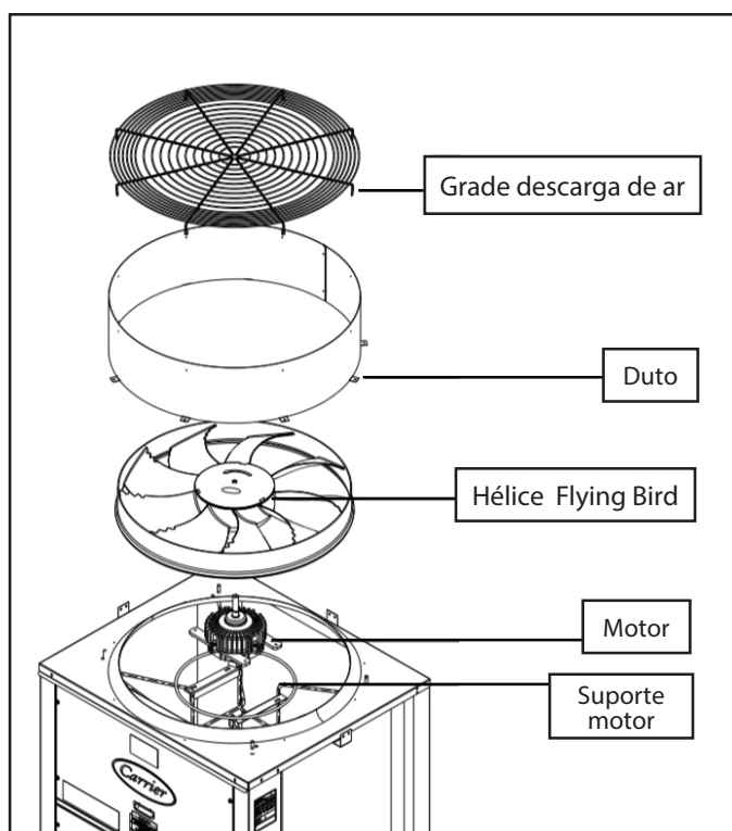
Figura 3: Vista explodida ventilador
