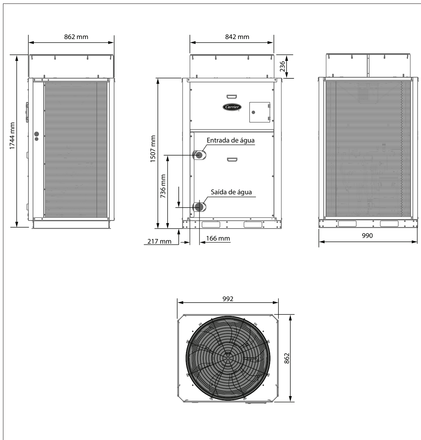
Figura 13 - Dimensional
