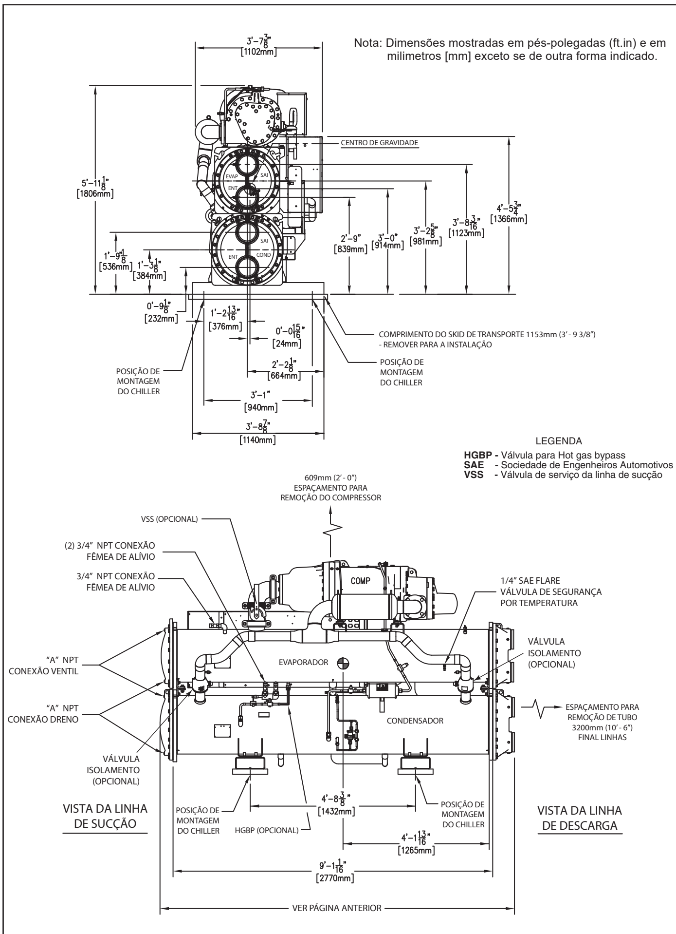
Fig. 2 – Dimensões Unidades 30XW150-200 (cont.)
