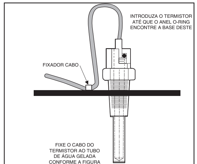
Fig. 19 — Termistor Duplo da Saída de Água (Número da peça 00PPG000008105)
