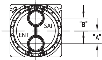
Fig. 2 – Dimensões Unidades 30XW150-200 (cont.)
