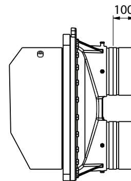
ADAPTADOR SOLDA-VICTAULIC
