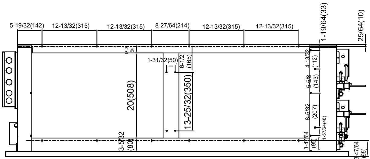
Vista traseira (Respiro de retorno de ar)
