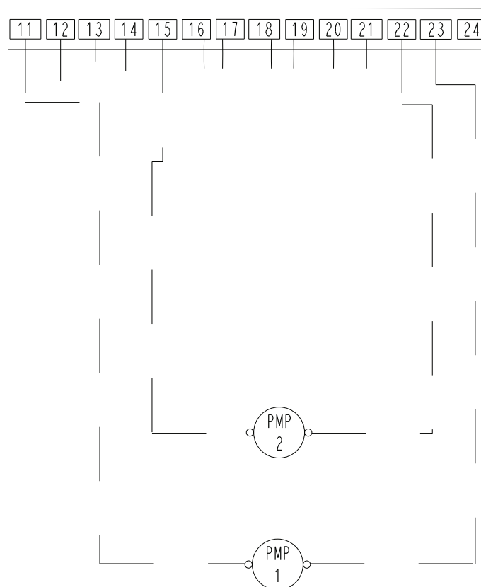
Fig. 38 — Fiação para controle da bomba do evaporador
