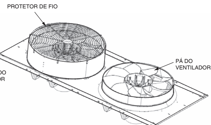
Fig. 73 — Montagem do ventilador
