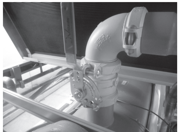
Fig. 68 — Válvula bloqueio da sucção – aberta
