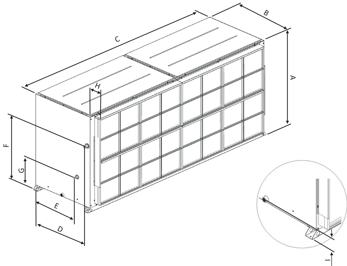
Dimensões em mm
