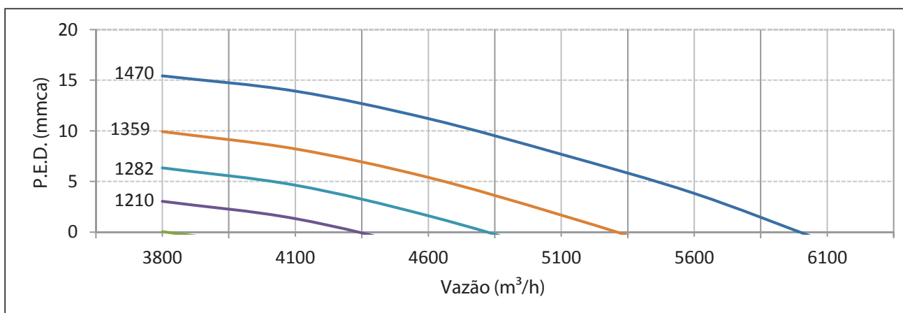
Módulo 40MV_252VH (G4 + M5)
