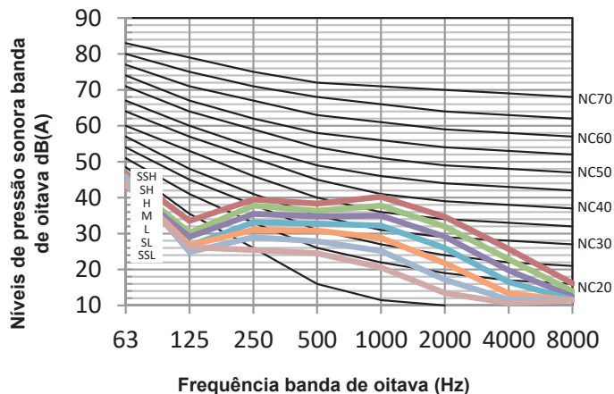
Figura 8.9: 42ATMQB28M5 níveis banda de oitava
