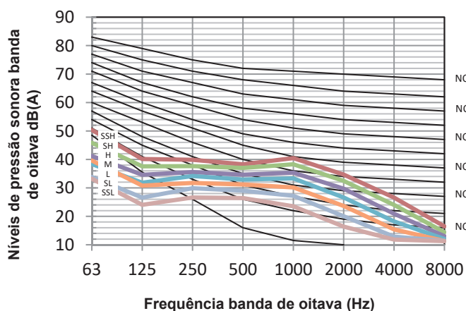
Figura 8.8: 42ATMQB24M5 níveis banda de oitava
