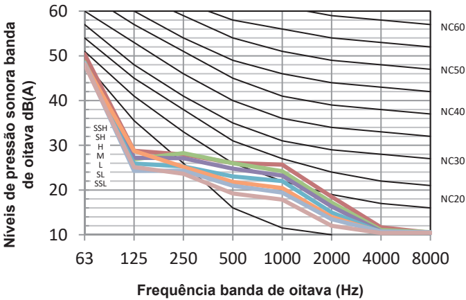
Figura 8.2: 42ATMQB05M5 níveis banda de oitava
