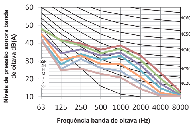
Figura 8.7: 42ATMQB18M5 níveis banda de oitava
