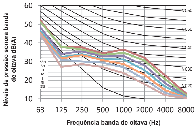
Figura 8.5: 42ATMQB12M5 níveis banda de oitava
