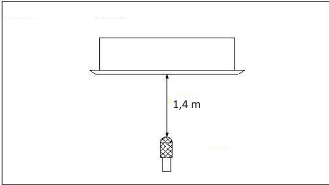
Figura 8.1: Medição do nível de pressão sonora do Cassette Uma Via
