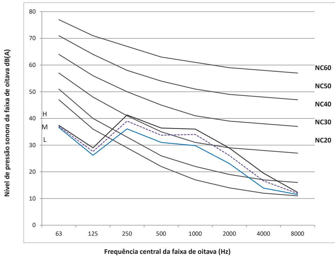
Figura 8.2: Níveis da faixa de oitava 40ATAQA09M5 / 40ATAQA12M5
