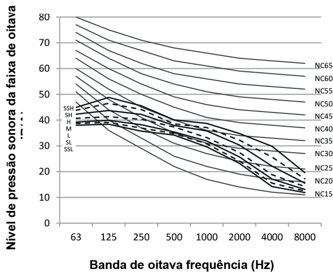
Figura 8.6: MI2-71(80)GDHN1 níveis banda de oitava
