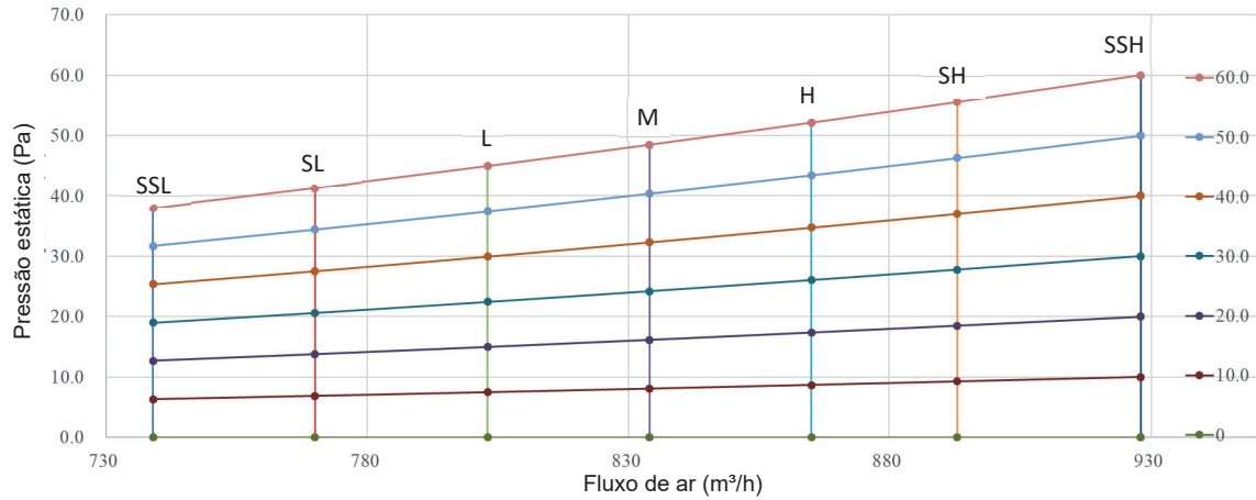
Figura 8.7: Dutado de Piso MI2-80F3DN1(A)
