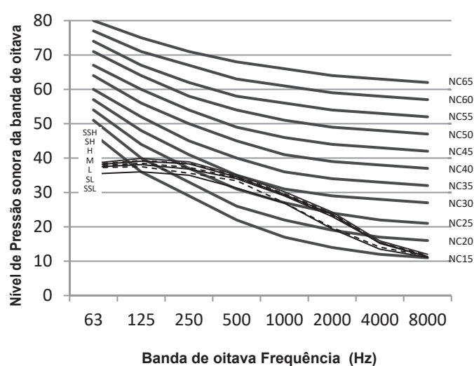
Figura 9.9: MI2-560T1DHN1 níveis banda de oitava
