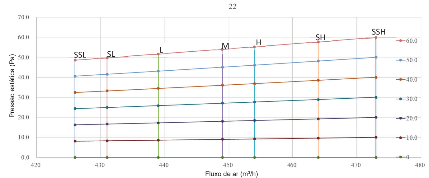
Figura 8.2: Dutado de Piso MI2-28F3DN1(A)
