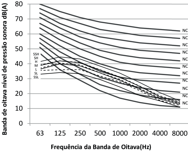
Figura 9.9: MI2-140T2DHN1 níveis banda de oitava
