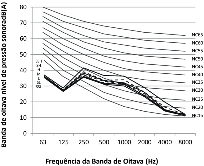
Figura 8.5: MI2-56Q1DHN1 níveis banda de oitava
