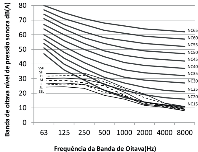
Figura 9.2: MI2-22(28)T2DHN1 níveis banda de oitava
