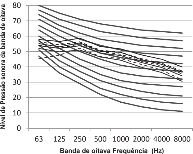
Figura 9.4: MI2-450FADHN1 níveis banda de oitava
