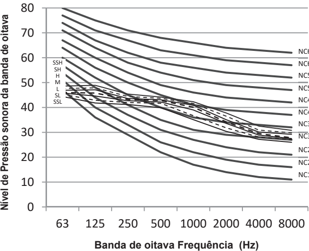
Figura 9.2: MI2-125(140)FADHN1 níveis banda de oitava
