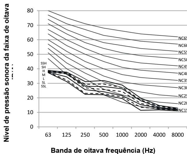
Figura 8.4: MI2-45GDHN1 níveis banda de oitava
