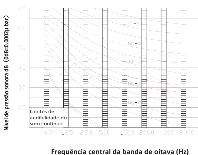
Figura 9.7: MDV-D112T2VN1BA5-B níveis banda de oitava
