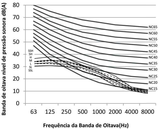
Figura 9.5: MI2-56T2DHN1 níveis banda de oitava
