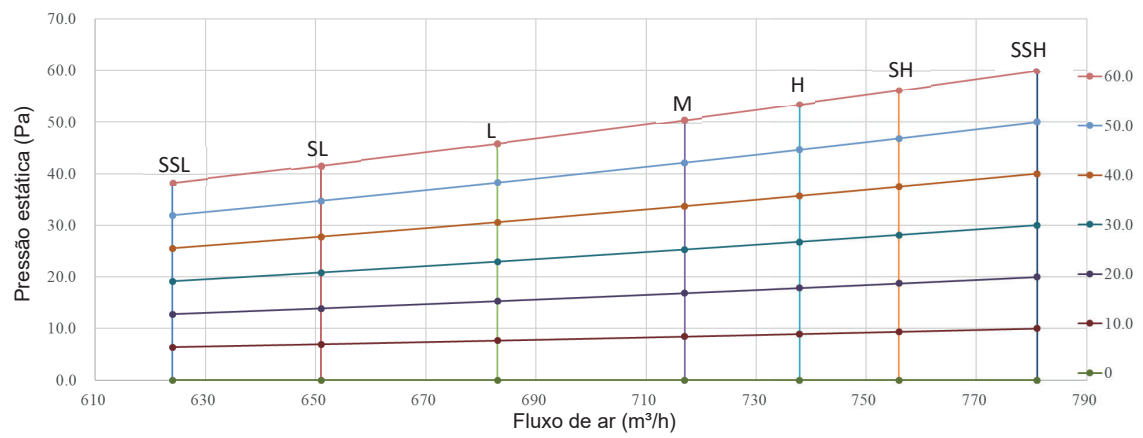
Figura 8.6: Dutado de Piso MI2-71F3DN1(A)
