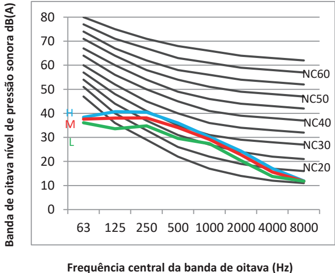
Figura 9.3: MDV-D28T2VN1DA5-B níveis banda de oitava
