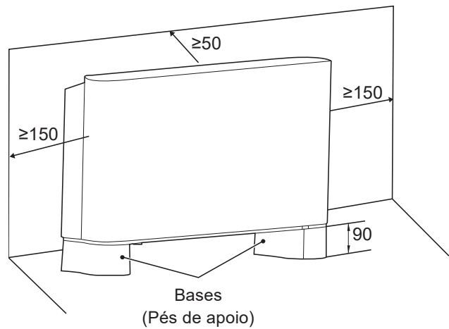
Figura 3.2: Modelos - Consoles de Retorno Inferior F5 (unidade: mm)
