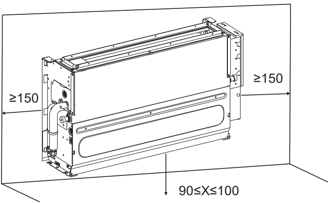
Figura 3.3: Modelos - Dutados de Piso F3 (unidade: mm)
