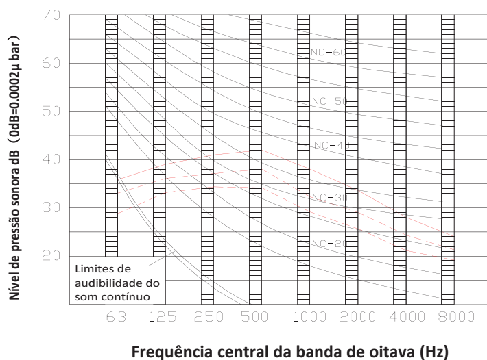
Figura 9.6: MDV-D80(90)T2VN1BA5-B níveis banda de oitava
