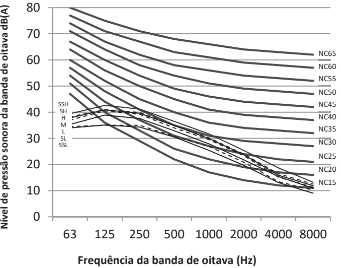
Figura 9.8: MI2-112T2DHN1(A) níveis banda de oitava
