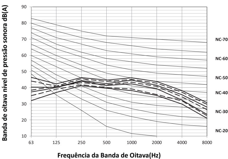
Figura 8.4: MI2-160DL DHN1 níveis banda de oitava
