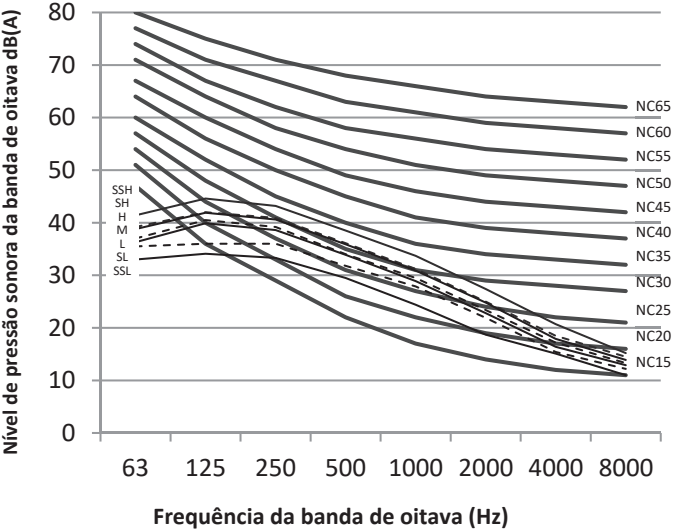
Figura 9.9: MI2-140T2DHN1(A) níveis banda de oitava
