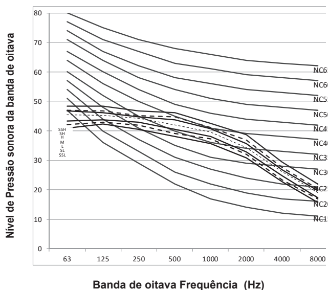
Figura 9.4: MI2-112T1DHN1 níveis banda de oitava
