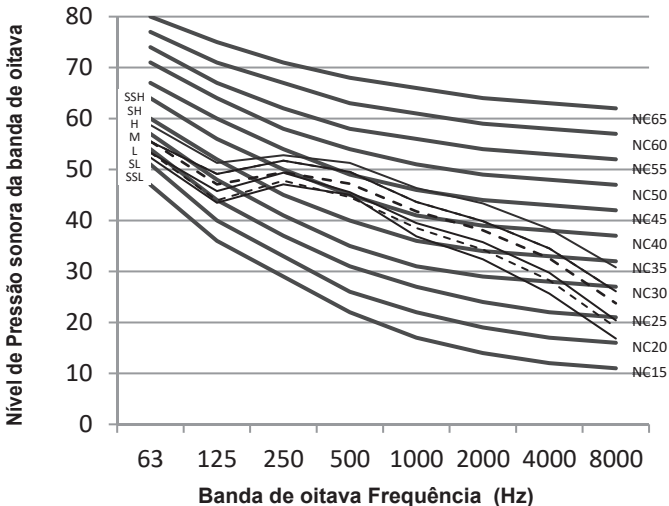
Figura 9.5: MI2-560FADHN1 níveis banda de oitava
