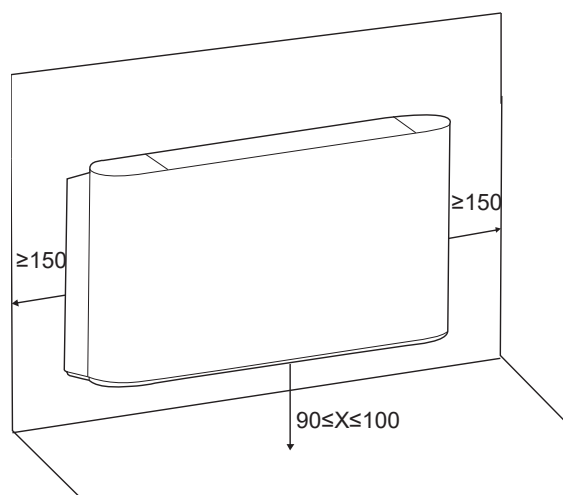
Figura 3.1: Modelos - Consoles de Retorno Frontal F4 (unidade: mm)
