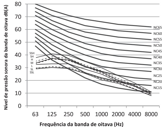
Figura 9.7: MI2-90T2DHN1(A) níveis banda de oitava
