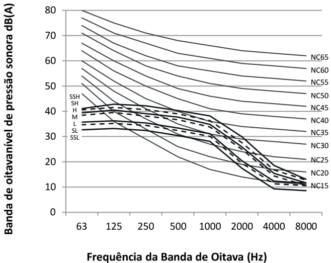
Figura 8.2: MI2-28(36)Q4DHN1 níveis banda de oitava
