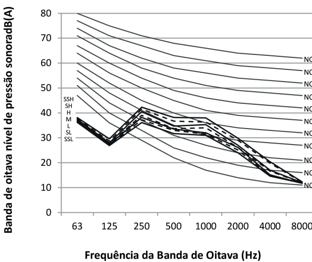
Figura 8.6: MI2-71Q1DHN1 níveis banda de oitava
