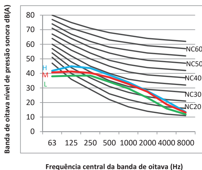
Figura 9.5: MDV-D71T2VN1DA5-B níveis banda de oitava
