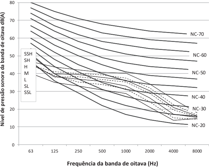
Figura 9.10: MI2-160T2DHN1(A) níveis banda de oitava
