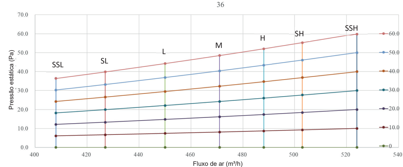
Figura 8.3: Dutado de Piso MI2-36F3DN1(A)
