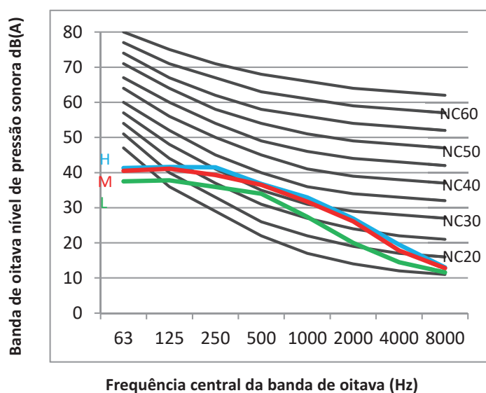
Figura 9.4: MDV-D36(45,56)T2VN1DA5-B níveis banda de oitava
