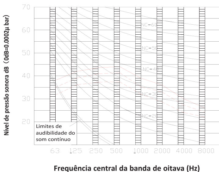
Figura 9.8: MDV-D140T2VN1BA5-B níveis banda de oitava
