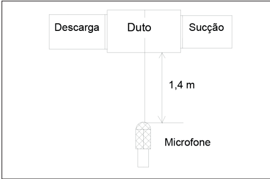
Figura 9.1: Medição do nível de pressão Sonora da unidade de processamento de ar externo
