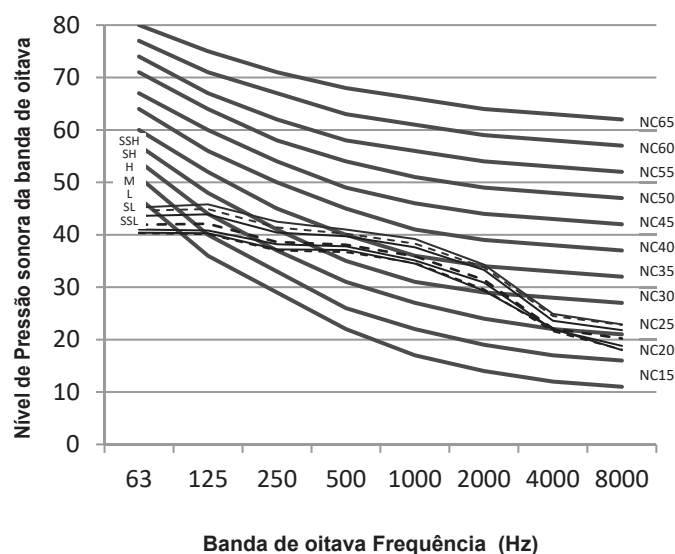
Figura 9.5: MI2-140T1DHN1 níveis banda de oitava
