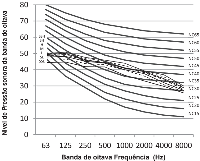
Figura 9.3: MI2-200(250, 280)FADHN1 níveis banda de oitava
