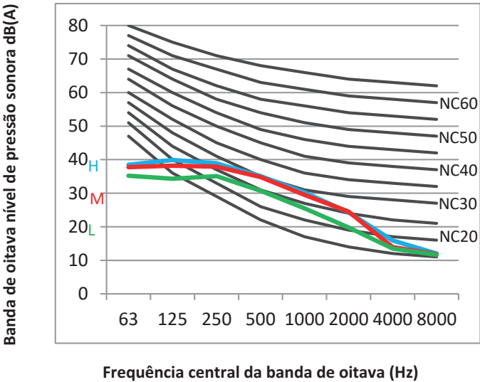
Figura 9.2: MDV-D22T2VN1DA5-B níveis banda de oitava
