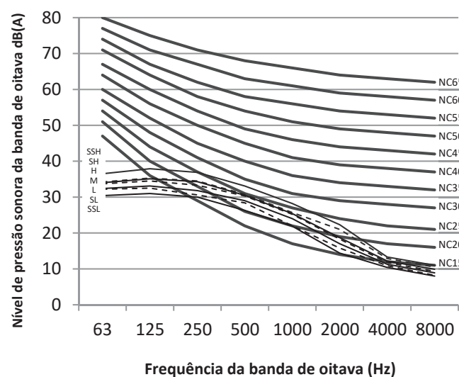
Figura 9.5: MI2-56T2DHN1(A) níveis banda de oitava
