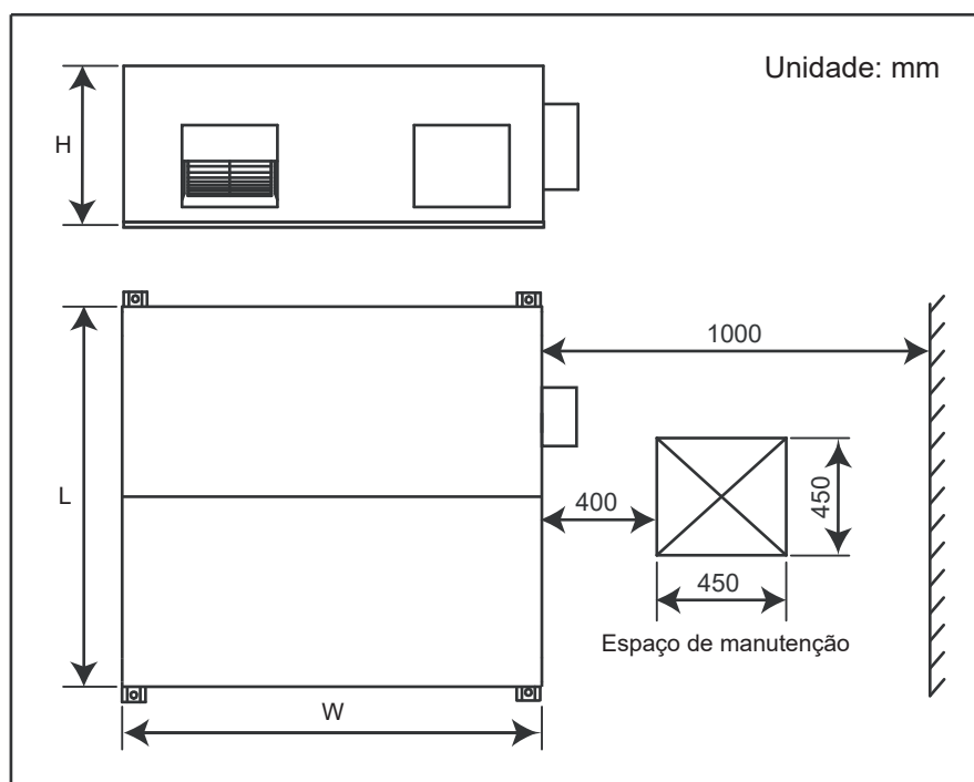
Figura 3.1: Modelos - HRV-D400(A) até HRV-D2000(A)
