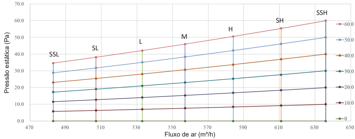
Figura 8.5: Dutado de Piso MI2-56F3DN1(A)
