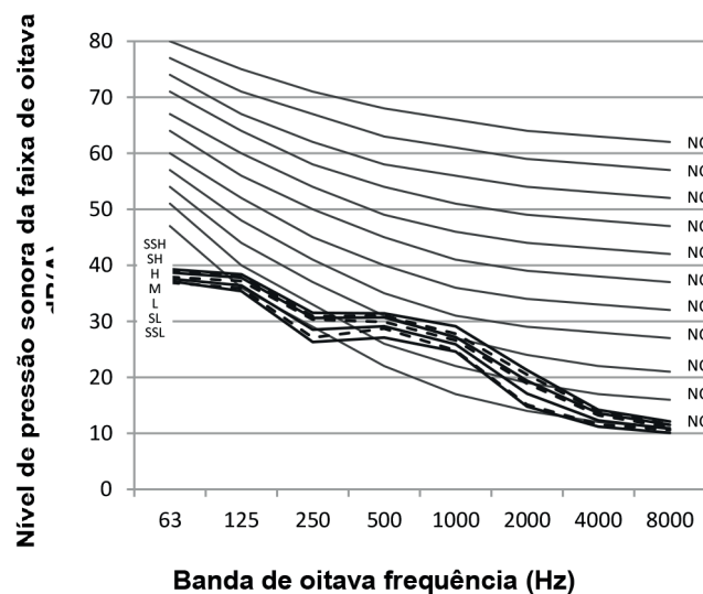
Figura 8.5: MI2-56GDHN1 níveis banda de oitava
