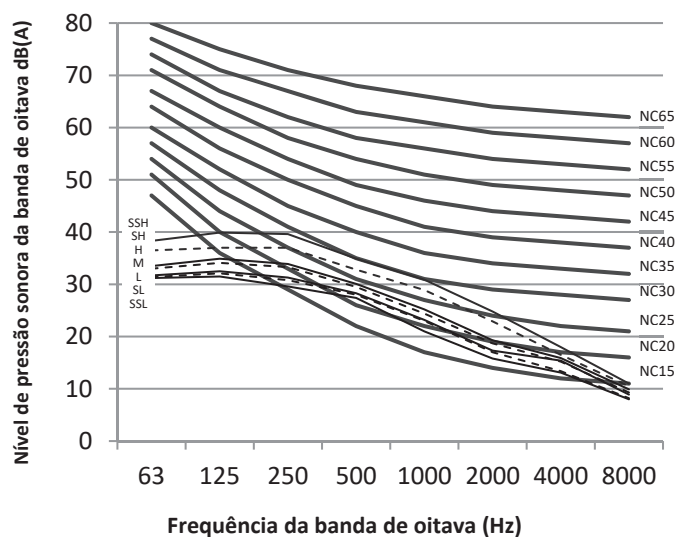
Figura 9.6: MI2-71T2DHN1(A) níveis banda de oitava
