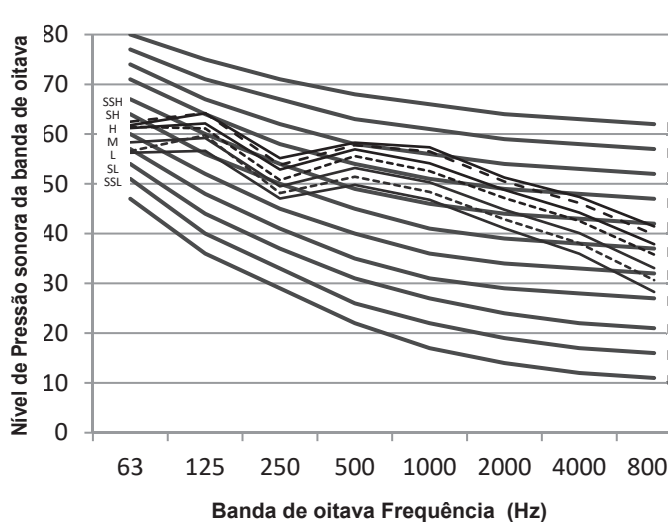
Figura 9.8: MI2-400(450)T1DHN1 níveis banda de oitava
