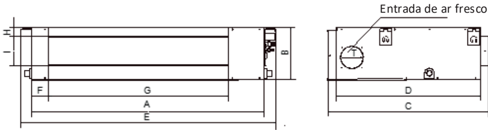
Figura 2.1: Dimensões do duto de média pressão estática
