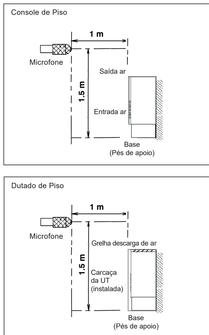
Figura 9.1: Medição do nível de pressão sonora no Console de Piso
