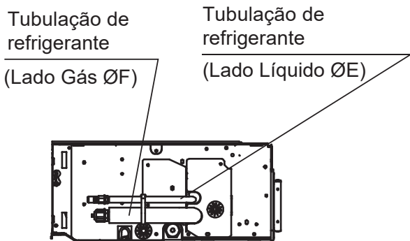
Figura 2.1: Conexões das tubulações - Dutados de Piso
