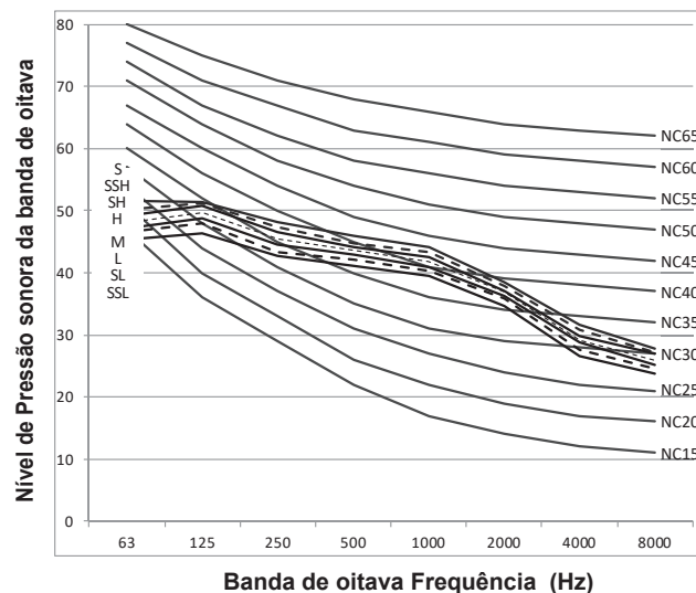
Figura 9.7: MI2-200(250,280)T1DHN1 níveis banda de oitava
