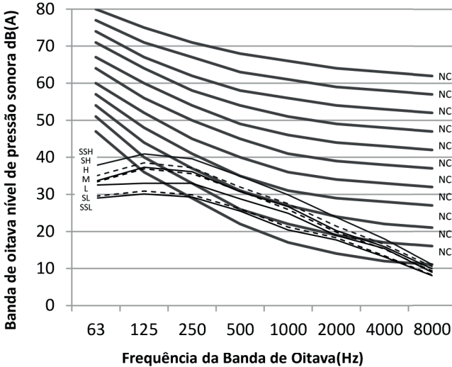
Figura 9.7: MI2-80(90)T2DHN1 níveis banda de oitava
