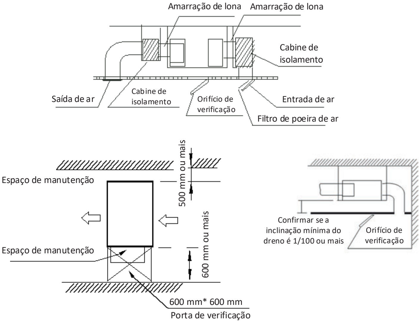
Figura 3.1: Requisitos de espaço para o Duto de Pressão Estática Média (unidade: mm)
