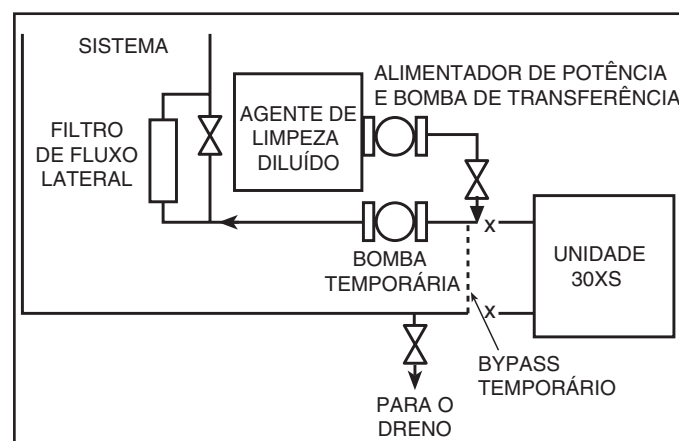
Figura 16 - Limpeza Utilizando um Filtro de Fluxo Lateral
