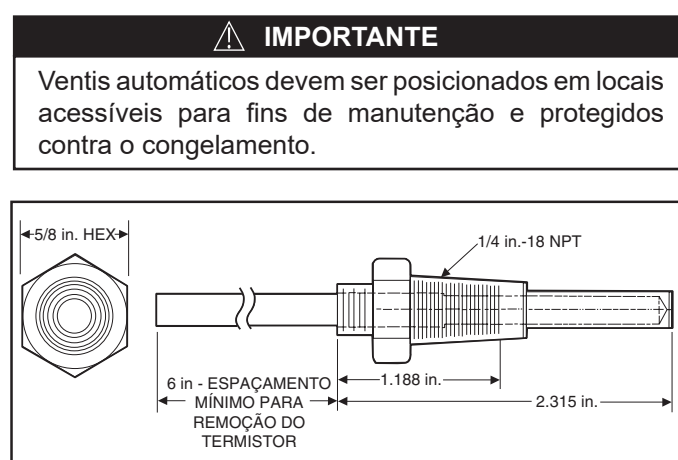
Figura 11 - Poço do Termistor Duplo da Saída de Água (Número da peça 00PPG000008000)
