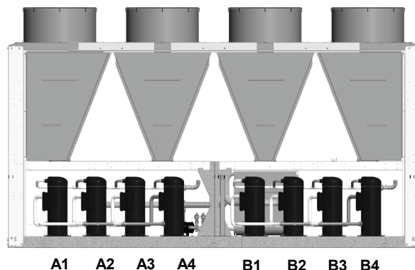
Figura 8 - Posição Compressores 30RSB
