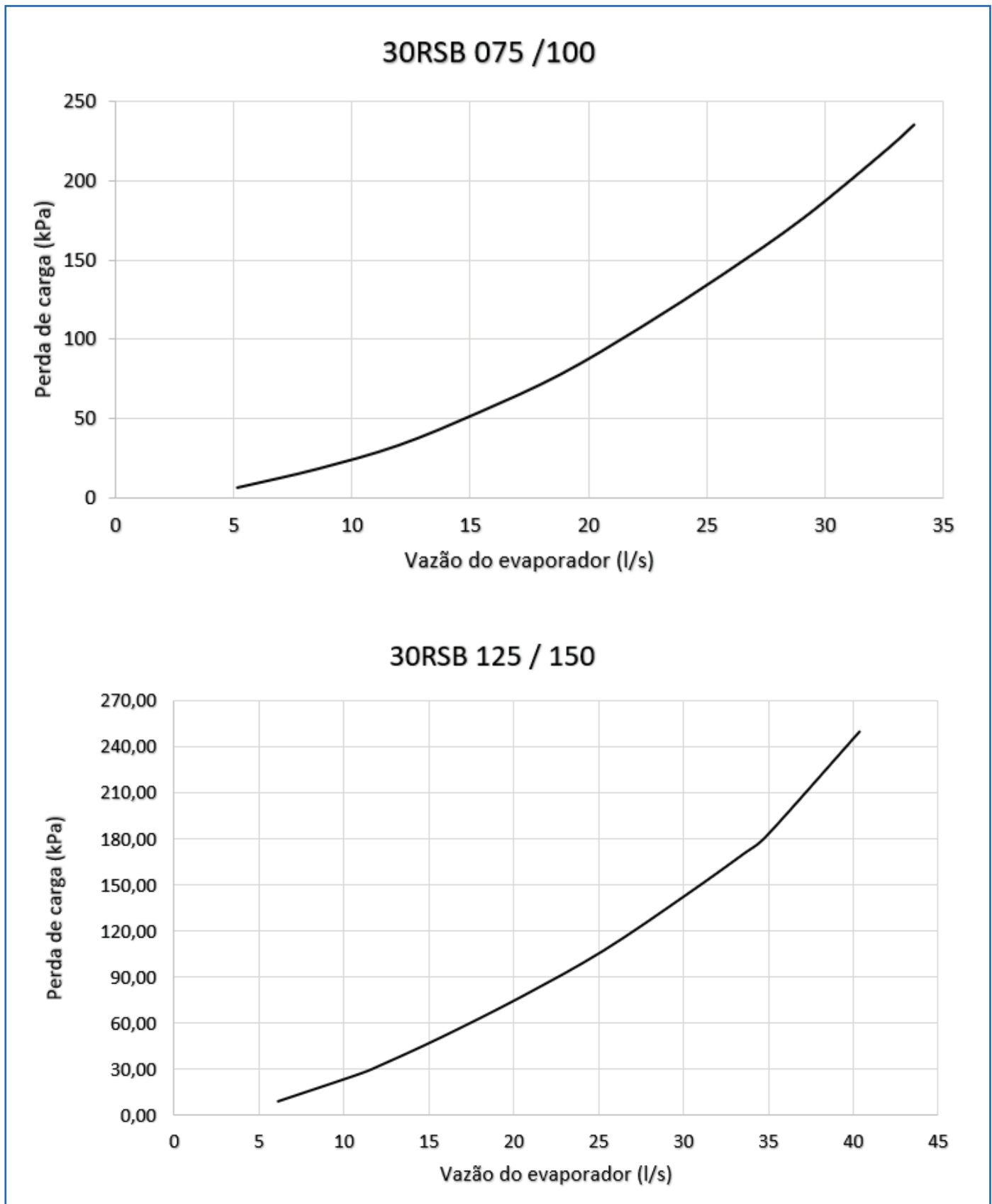
Figura 20a - Gráficos Perda de Carga
