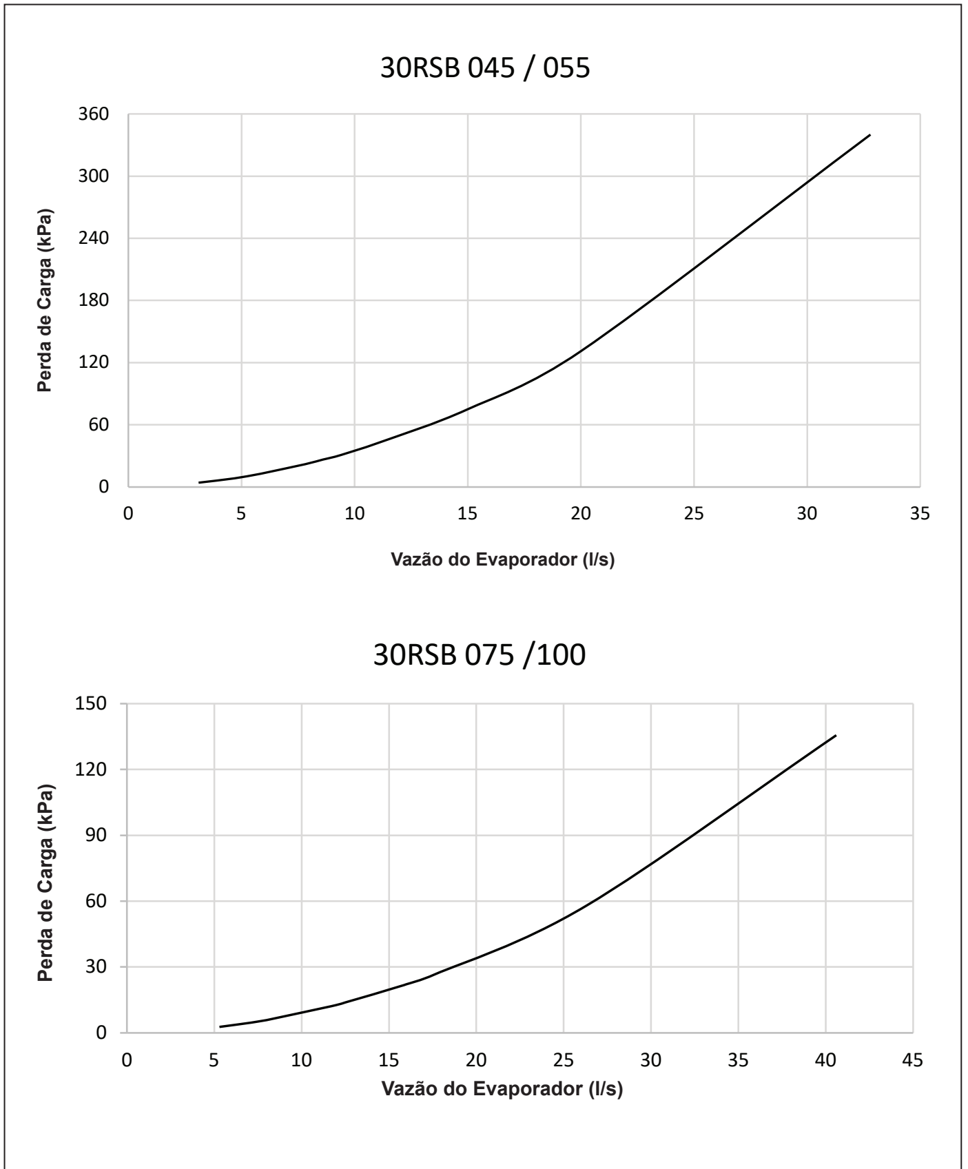
Figura 19a - Gráficos Perda de Carga
