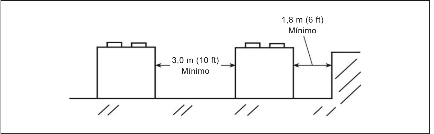
Figura 6 - Dimensional das Unidades 30RSB - Instalação de Múltiplas Unidades - Espaçamentos Mínimos Recomendados
