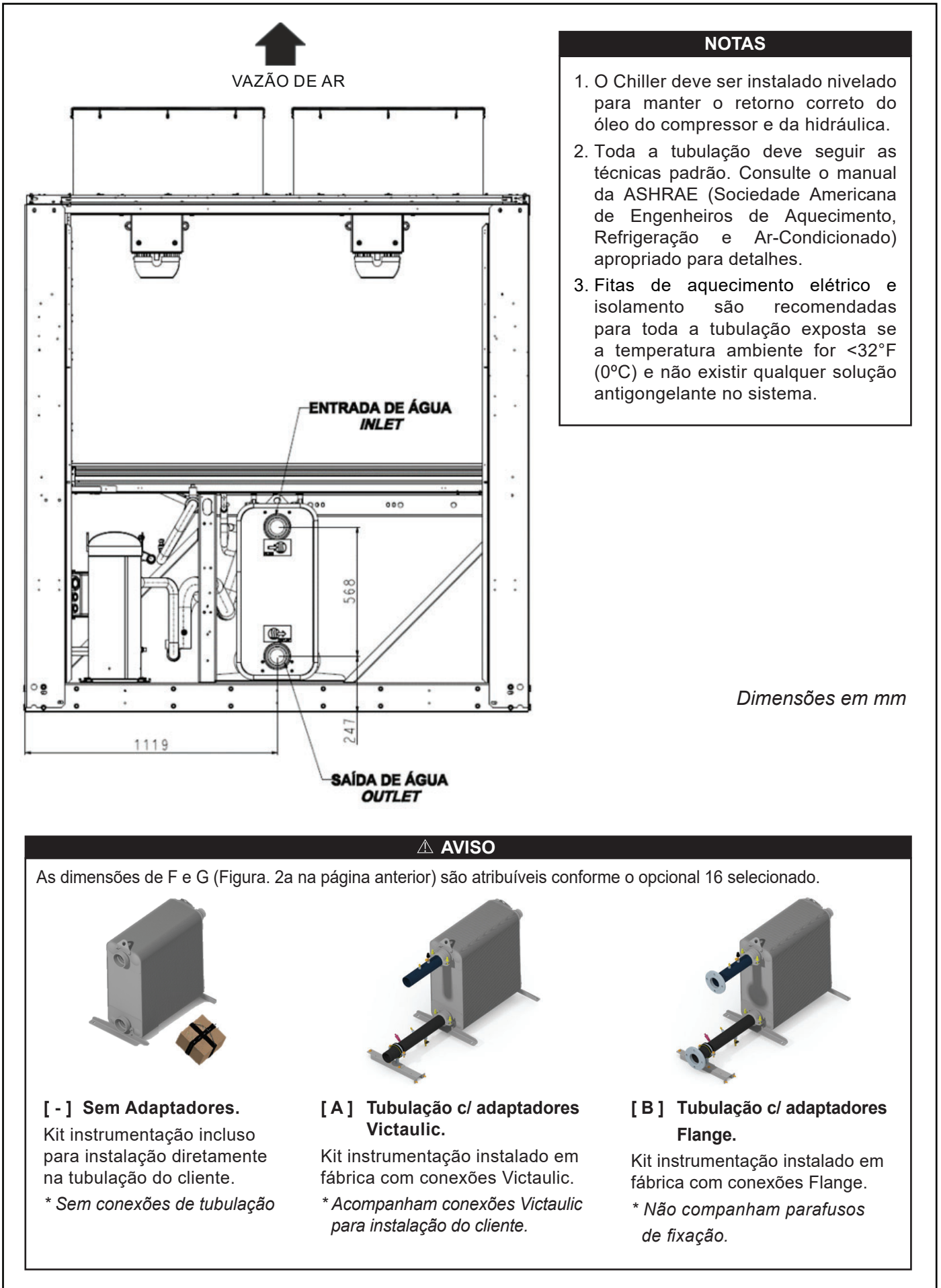
Figura 3b - Dimensional das Unidades 30RSB (cont.)
