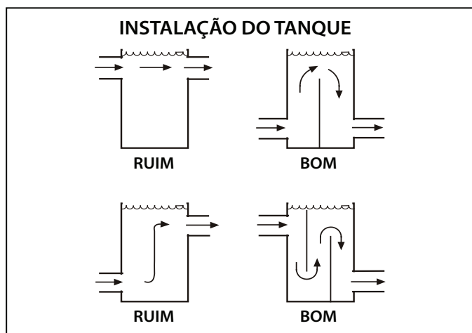
Figura 14 - Fluxo Tanque
