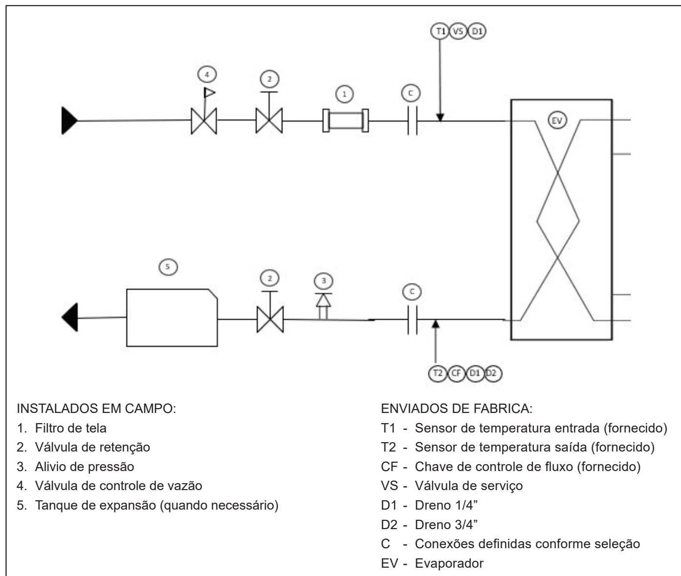
Figura 16 - Esquema típico de instrumentação do sistema
