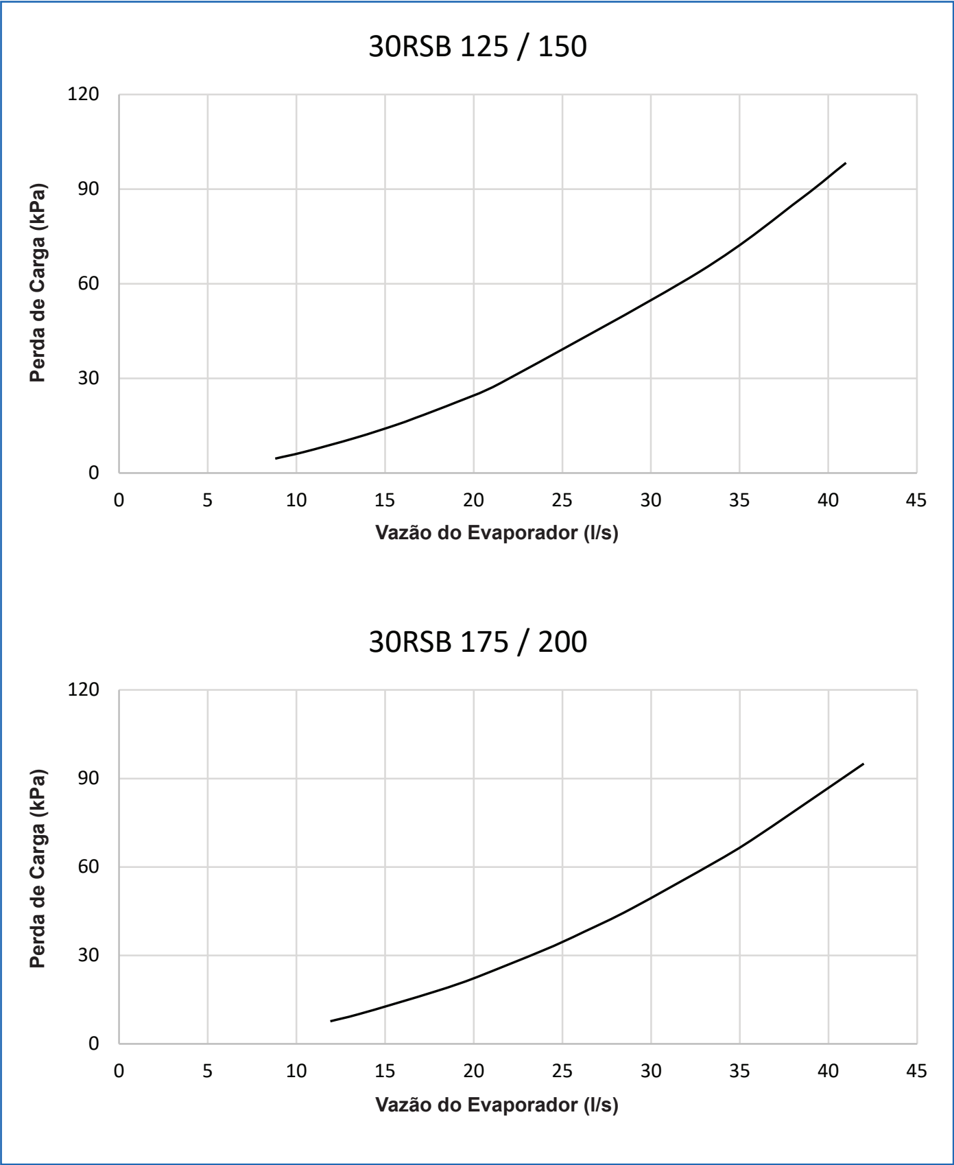
FIG. 8b - Gráficos Perda de Carga (cont.)
