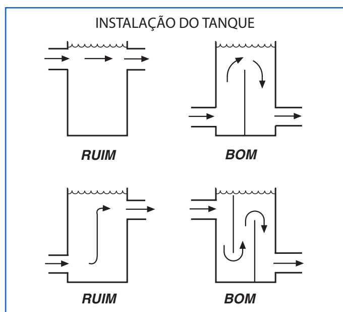
FIG. 13 - Instalação do Tanque
