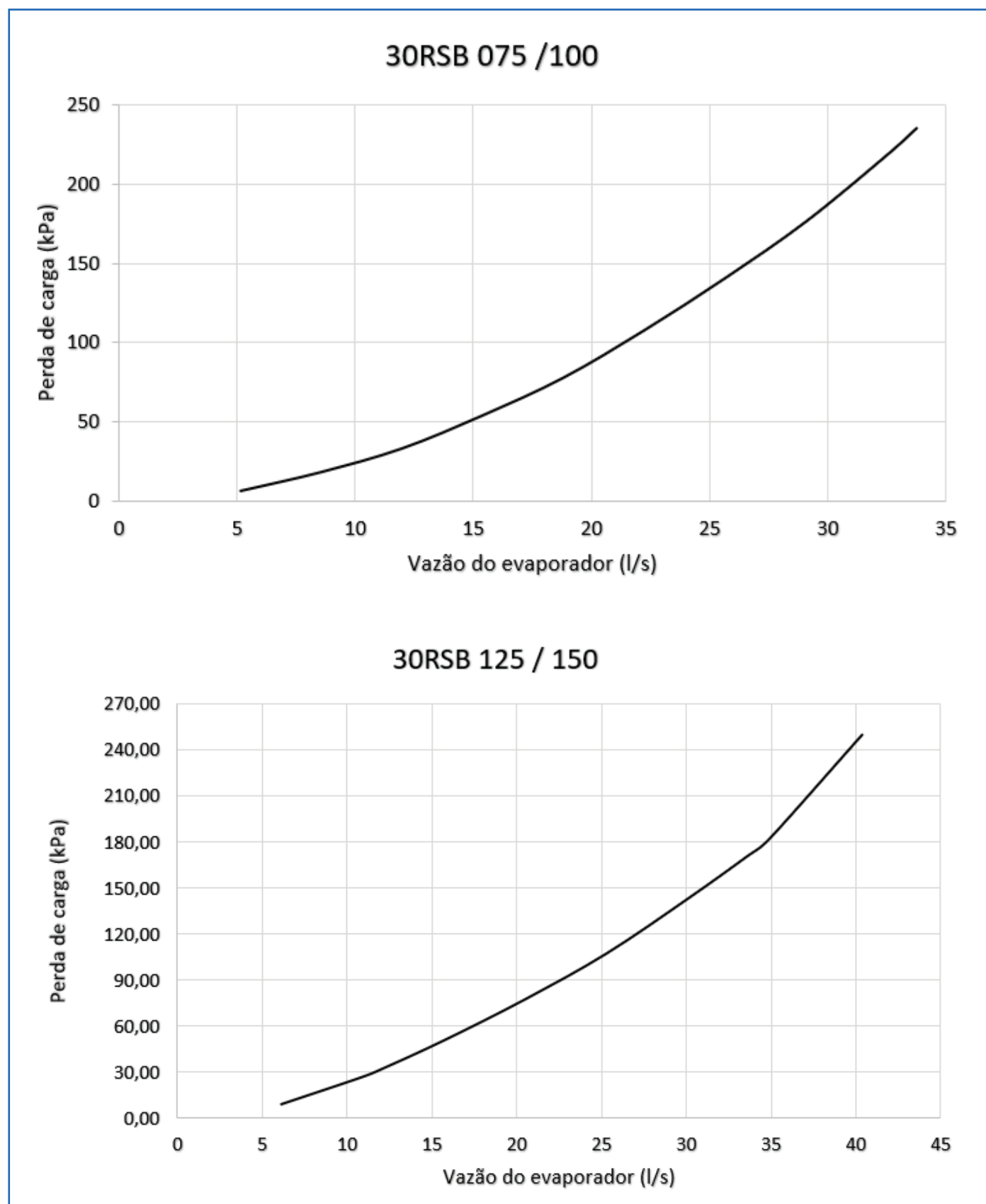
FIG. 9a - Gráficos Perda de Carga
