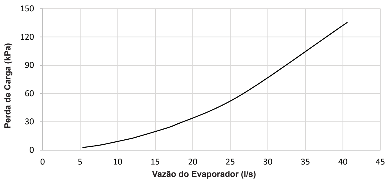
FIG. 8a - Gráficos Perda de Carga
