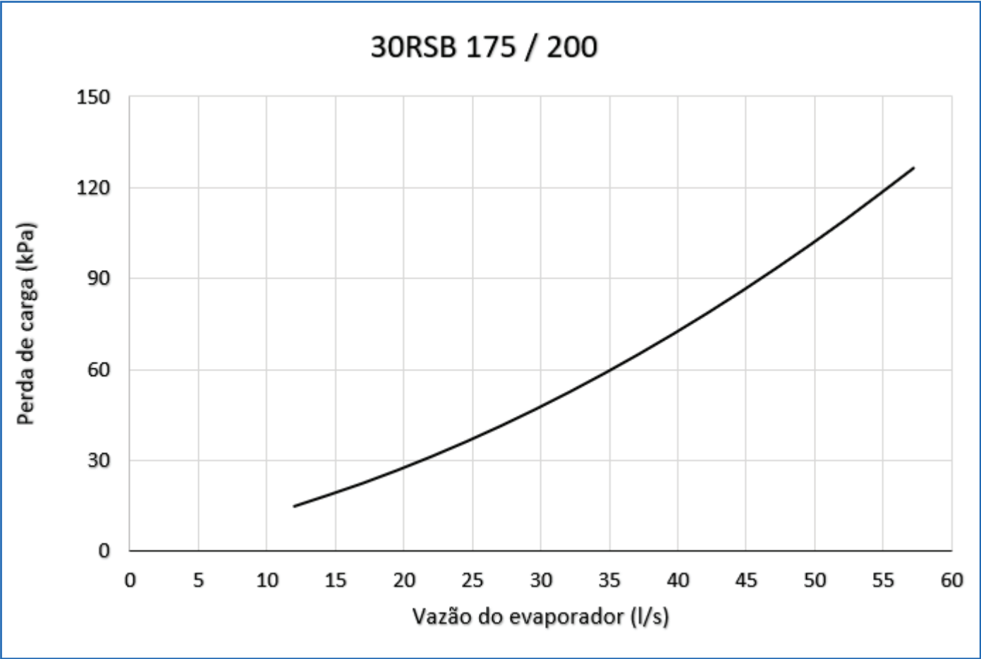
FIG. 9b - Gráficos Perda de Carga
