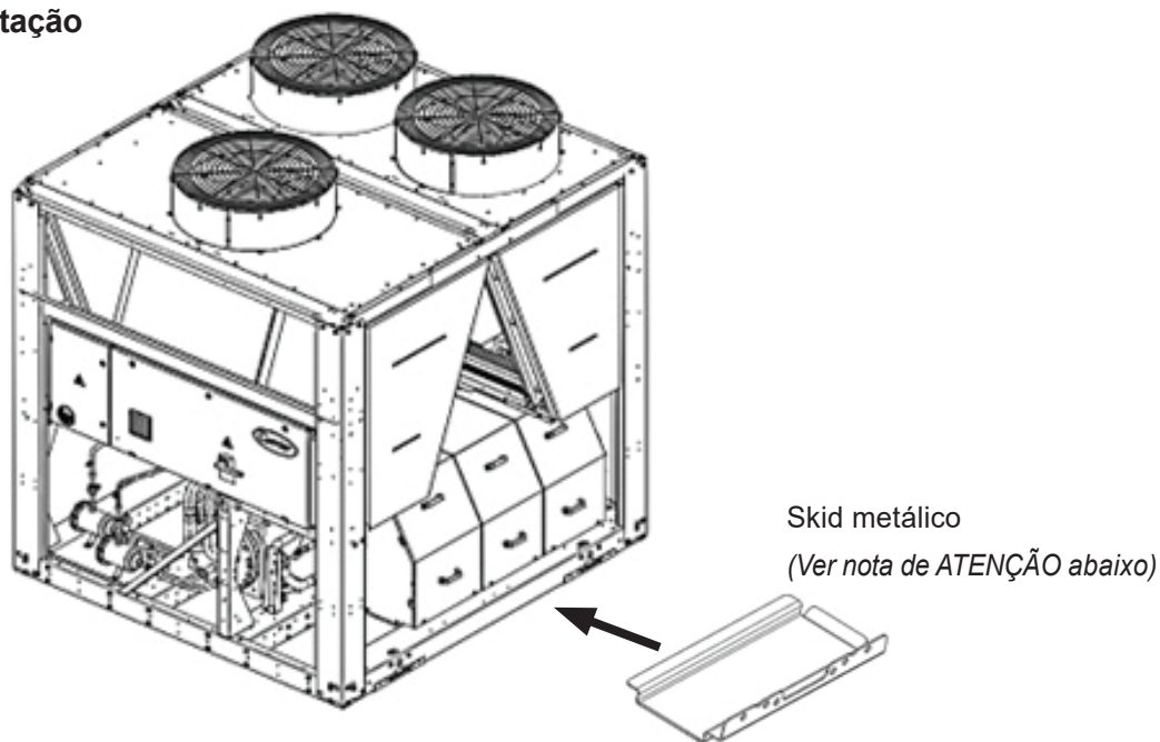
FIG. 2 - Configuração Exportação 30RSB
