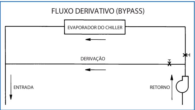
FIG. 12 - Fluxo Derivativo
