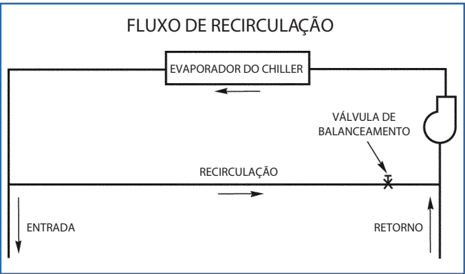
FIG. 11 - Fluxo de Recirculação
