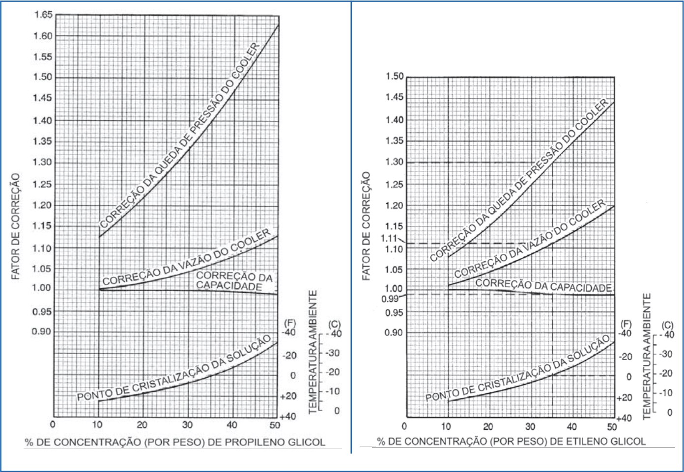
FIG. 7 - Gráficos Fator de Correção
