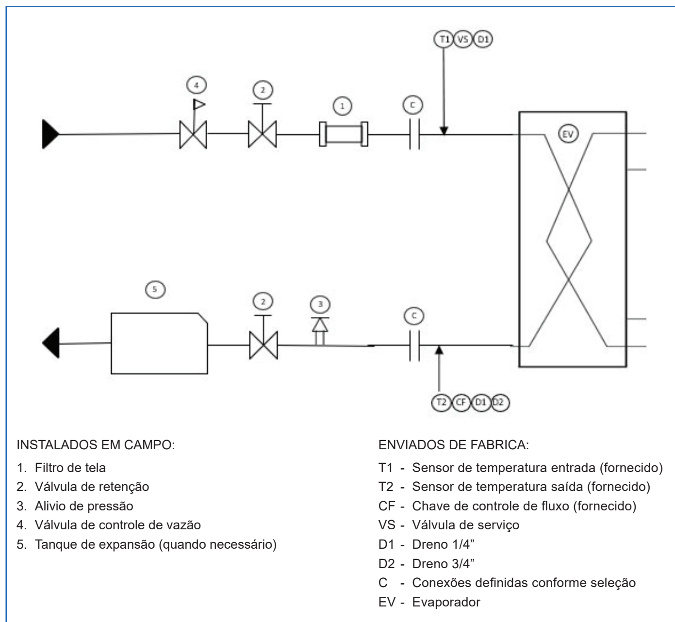
FIG. 10 - Diagrama Tubulação
