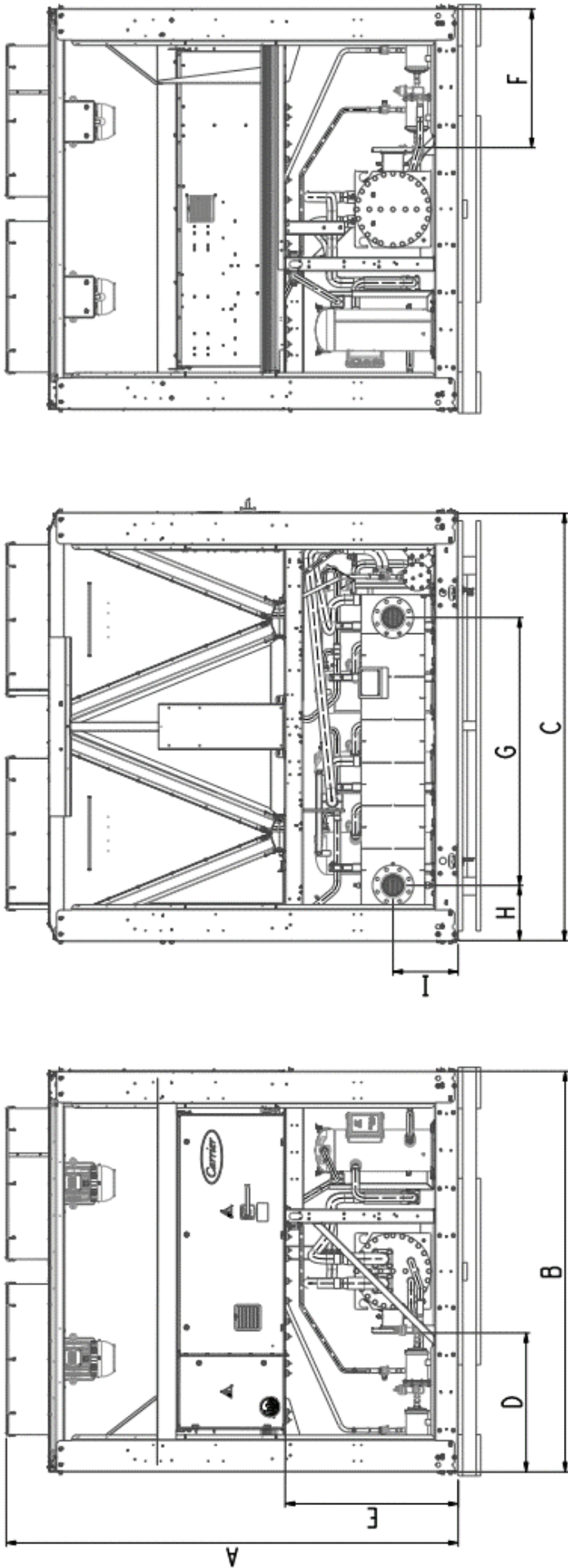
FIG. 6a - Dimensional das Unidades 30RSB S&T
