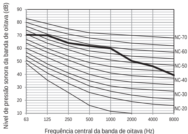
Figura 2-9.6 Nível da banda de oitava de 16HP
