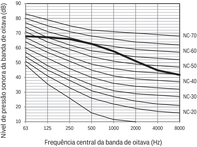
Figura 2-9.8 Nível da banda de oitava de 20HP
