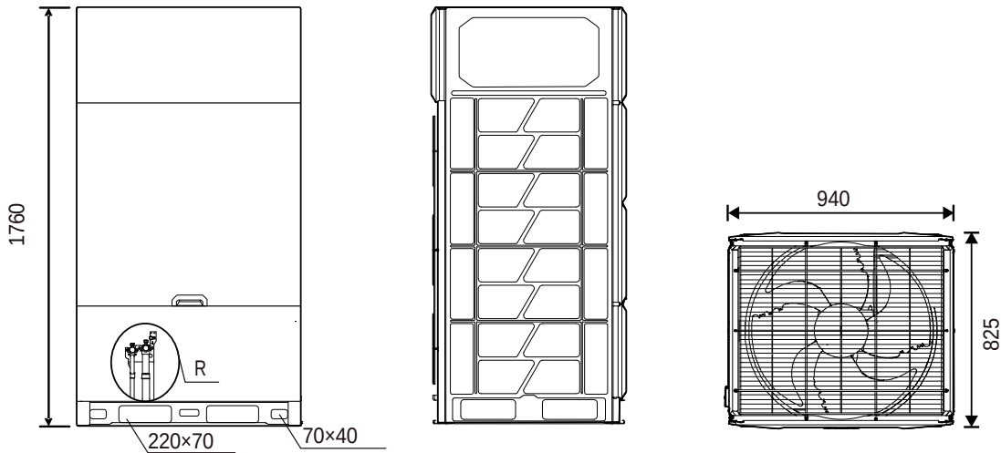
Figura 2-2.1: Dimensões 8/10/12/14/16HP (dimensões em mm)
