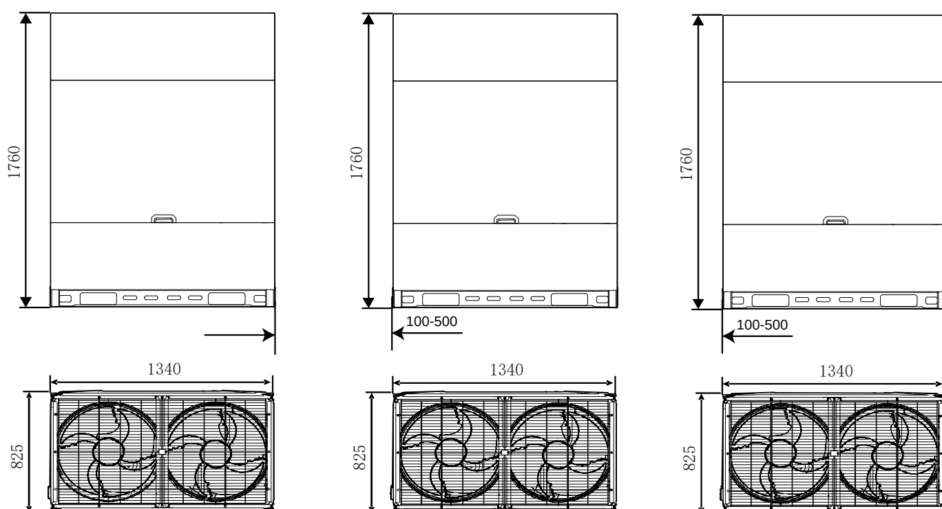
Figura 2-2.10: Dimensões das unidades 78/80/82/84/86/88/90HP (dimensões em mm)
