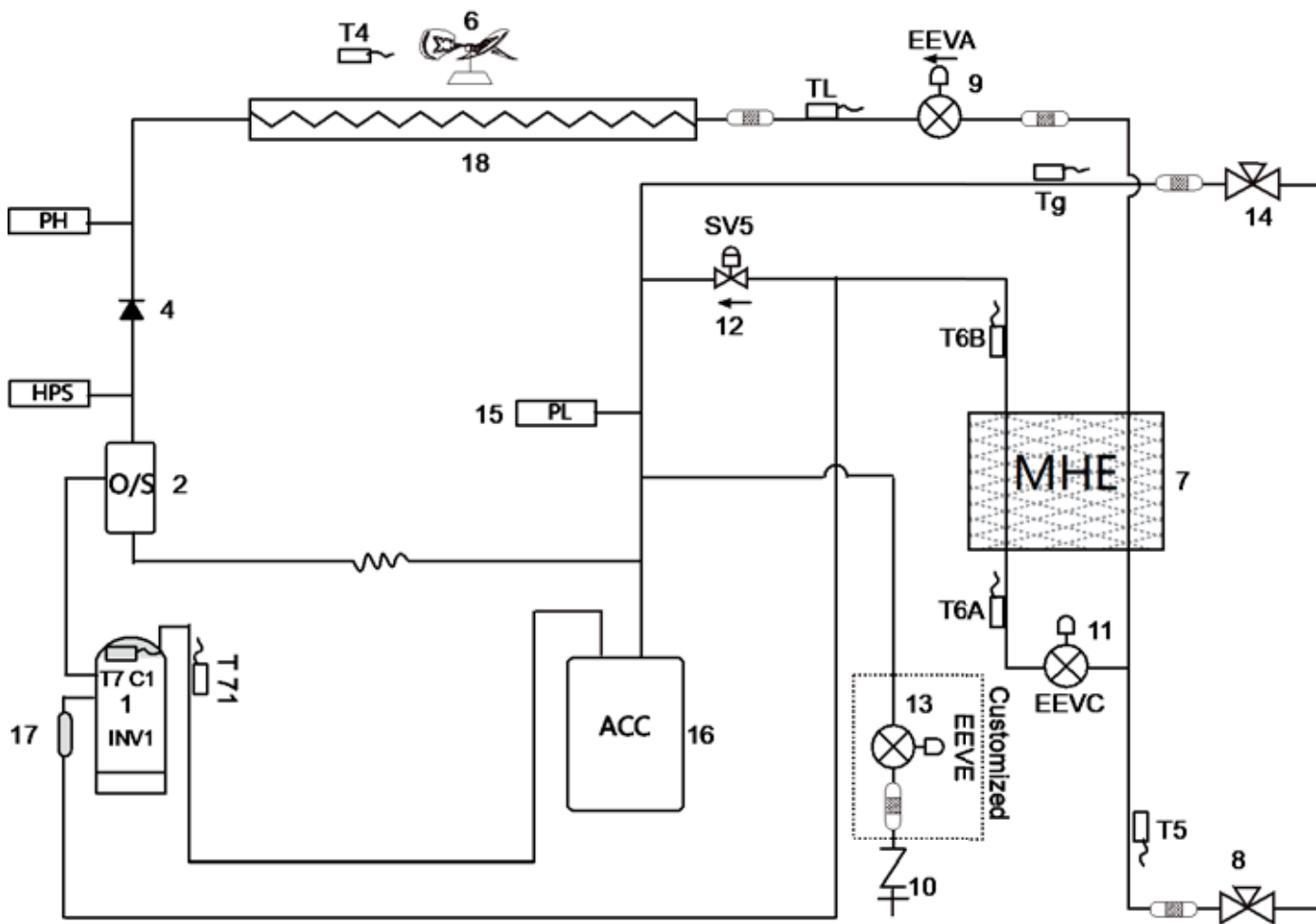
Figura 2-3.2: Diagramas de tubulação 14-16HP
