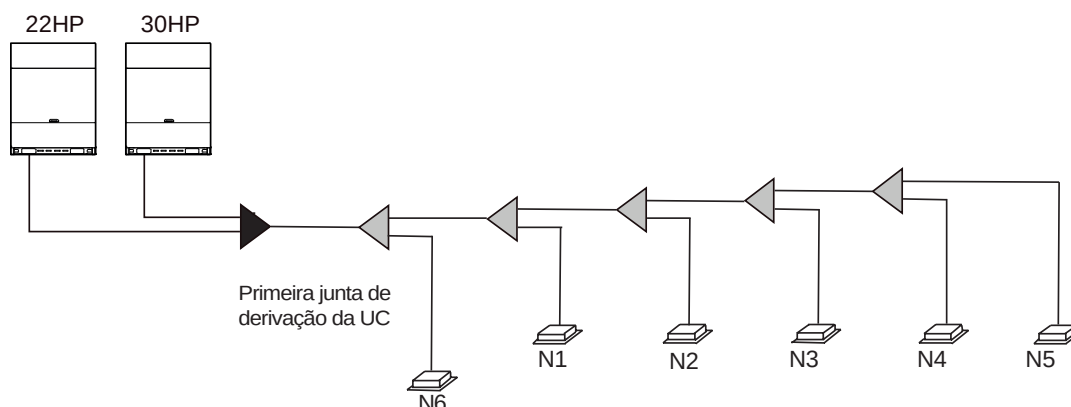
Figura 3-2.4: Posicionamento das unidades centrais mestre & auxiliar
