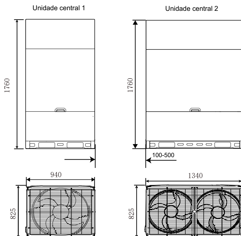
Figura 2-2.6: Dimensões das unidades 34/36/38/40/42/44/46HP (dimensões em mm)
