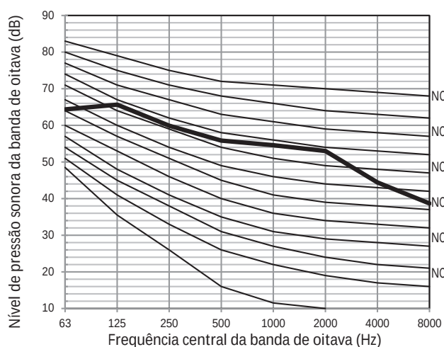
Figura 2-9.4 Nível da banda de oitava de 12HP
