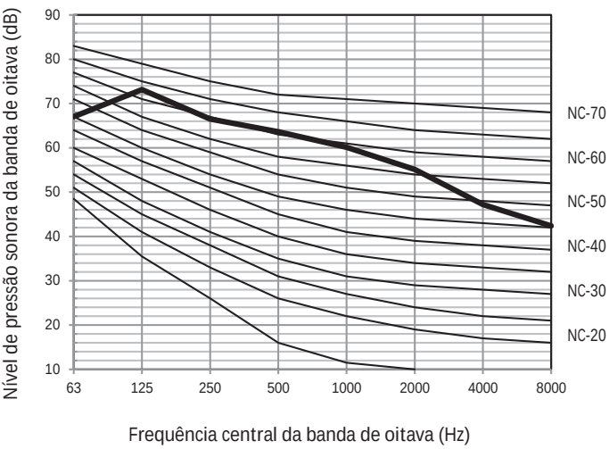
Figura 2-9.13 Nível da banda de oitava de 30HP
