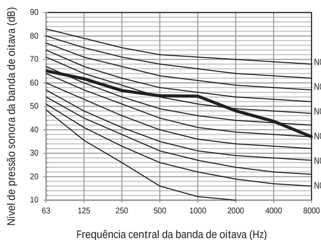
Figura 2-9.3 Nível da banda de oitava de 10HP
