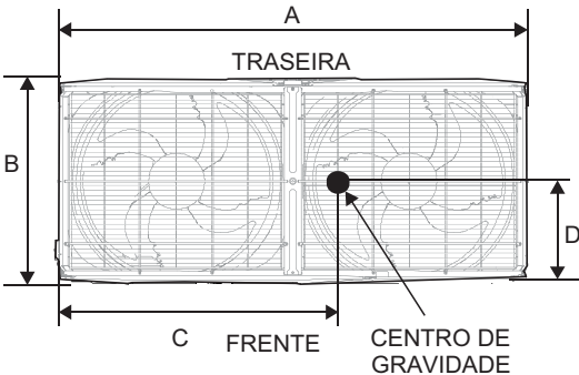
Figura 3-2.9: Centro de gravidade 18-40HP
