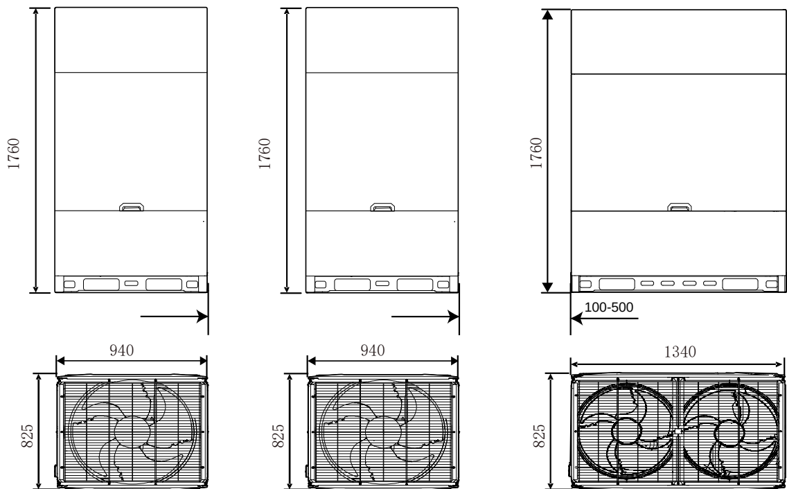
Figura 2-2.8: Dimensões das unidades 62HP (dimensões em mm)
