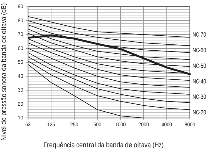
Figura 2-9.11 Nível da banda de oitava de 26HP
