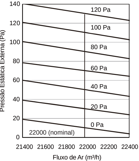
Figura 3-3.6: Desempenho do ventilador 18-30HP
