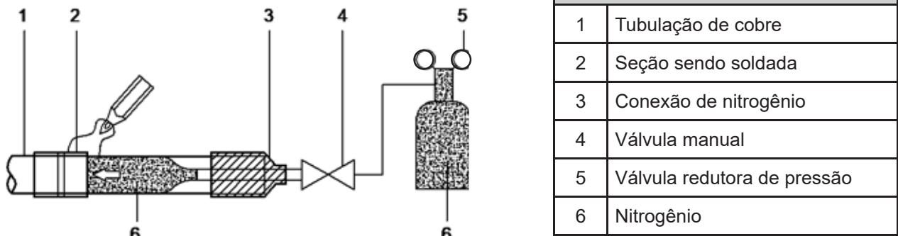
Figura 3-5.4: Fluxo de nitrogênio pela tubulação durante a soldagem
