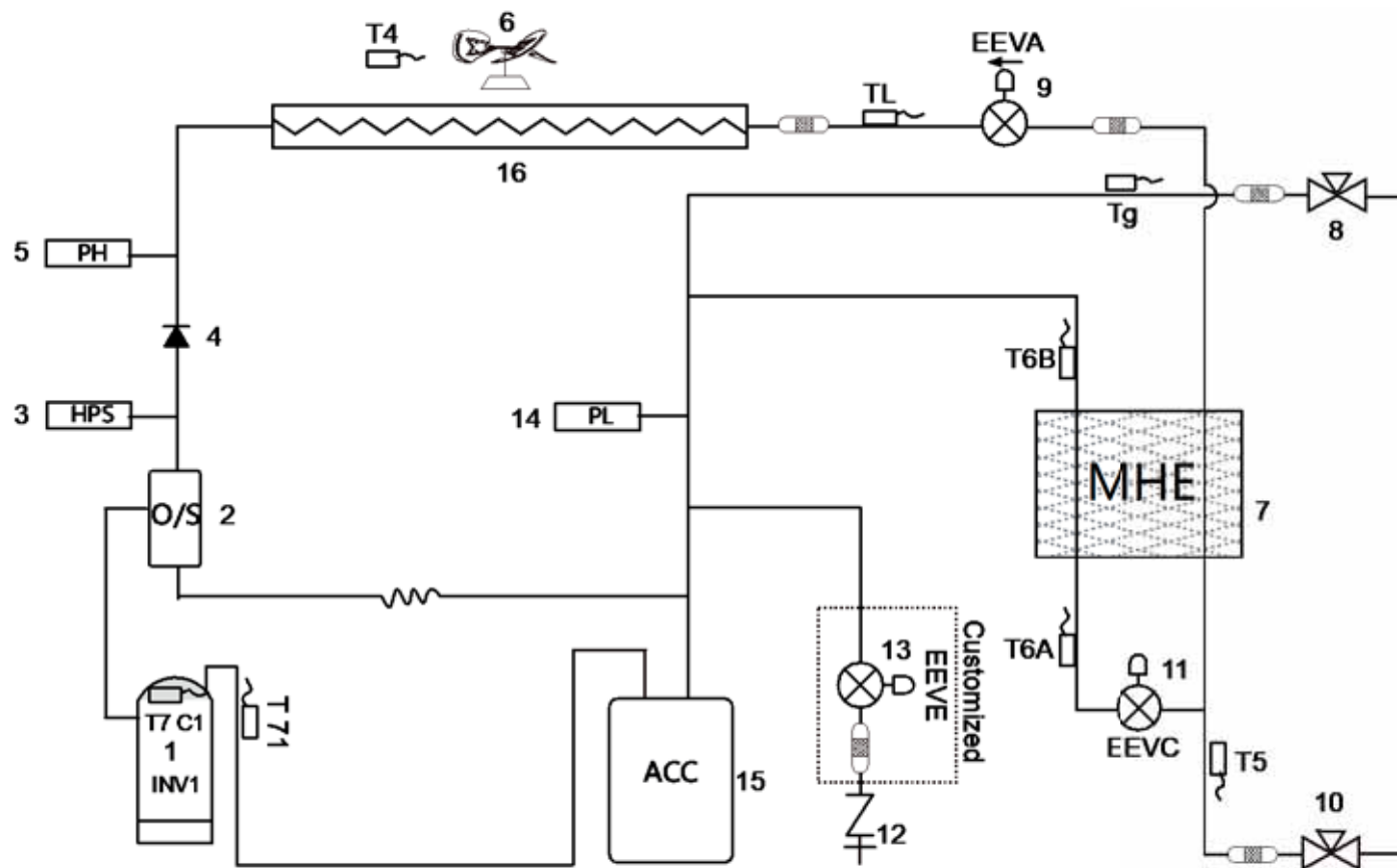
Figura 2-3.1: Diagramas de tubulação 8-12HP
