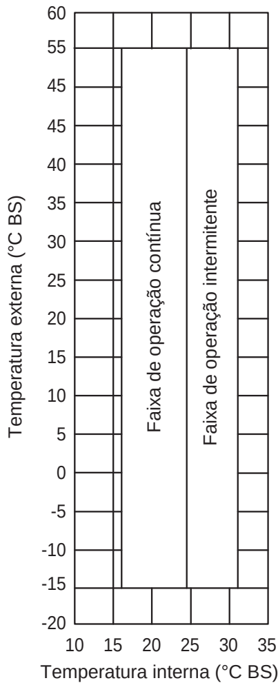
Figura 2-8.1: Limites de operação de resfriamento
