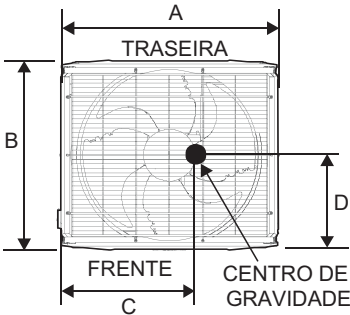
Figura 3-2.9: Centro de gravidade 18-40HP
