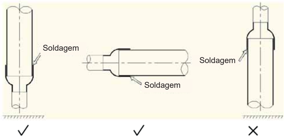
Figura 3-5.6: Orientação da tubulação durante a soldagem
