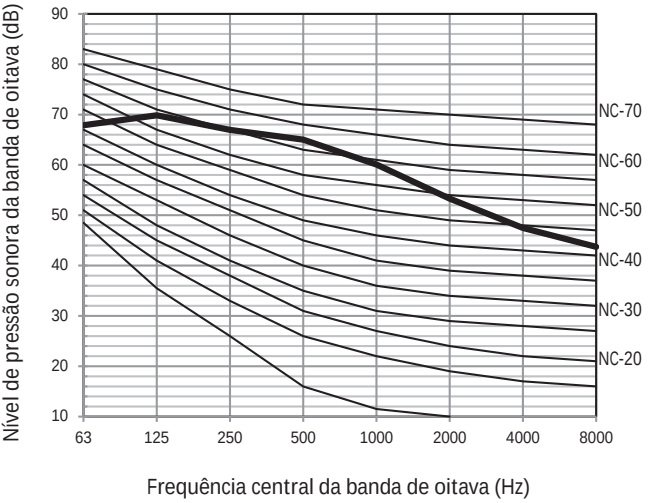
Figura 2-9.12 Nível da banda de oitava de 28HP
