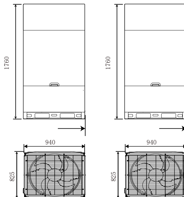
Figura 2-2.5: Dimensões da unidade 32HP (dimensões em mm)
