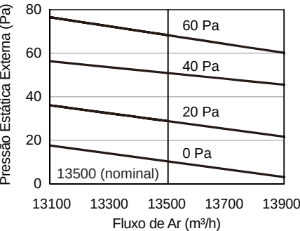
Figura 3-3.4: Desempenho do ventilador 8-12HP
