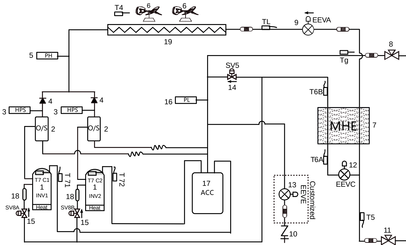
Figura 2-3.3: Diagramas de tubulação 18-24HP
