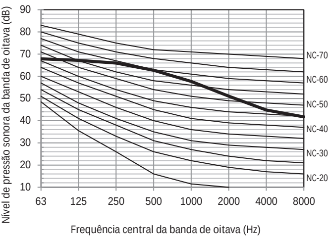
Figura 2-9.9 Nível da banda de oitava de 22HP
