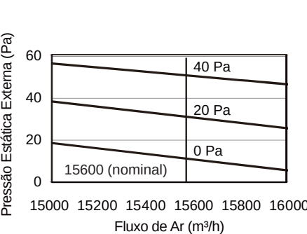
Figura 3-3.5: Desempenho do ventilador 14-16HP
