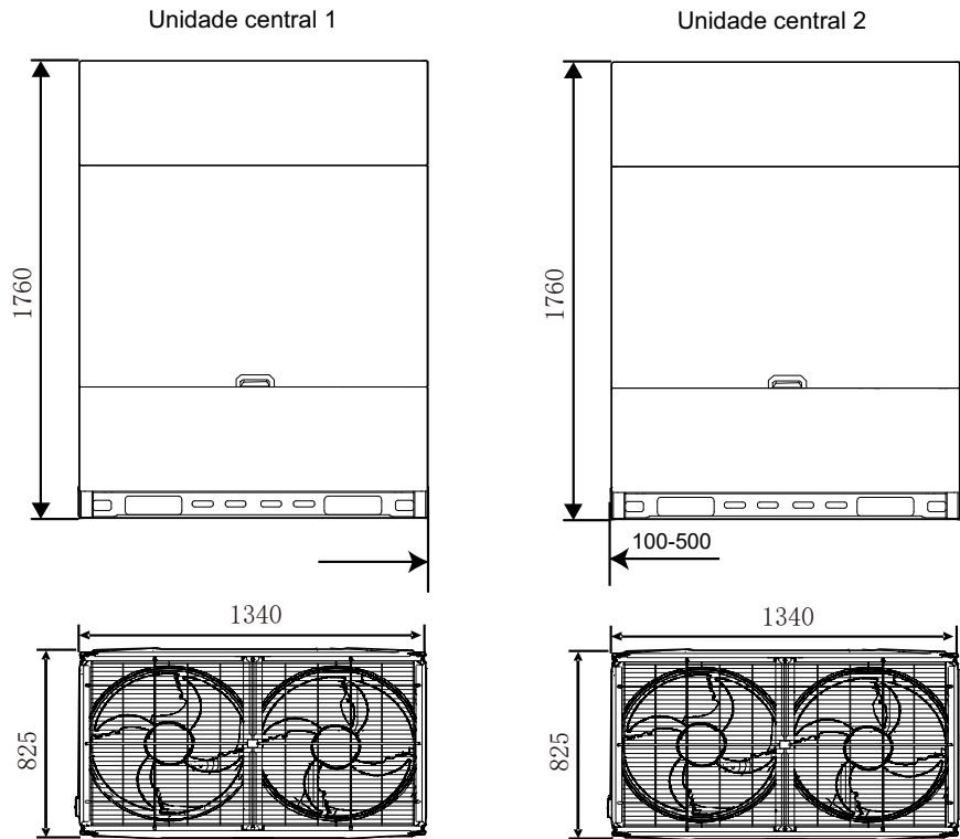
Figura 2-2.7: Dimensões da unidade 48/50/52/54/56/58/60HP (dimensões em mm)
