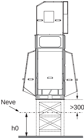
Figura 3-3.7: Blindagem de neve de unidade central (unidade: mm)
