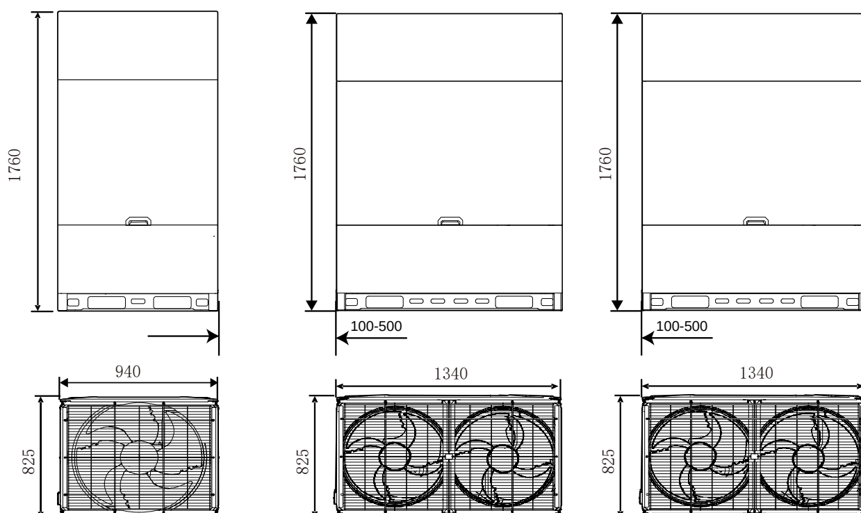
Figura 2-2.9: Dimensões das unidades 64/66/68/70/72/74/76HP (dimensões em mm)
