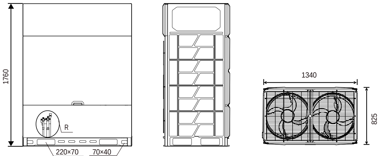
Figura 2-2.2: Dimensões 18/20/22/24/26/28/30HP (dimensões em mm)
