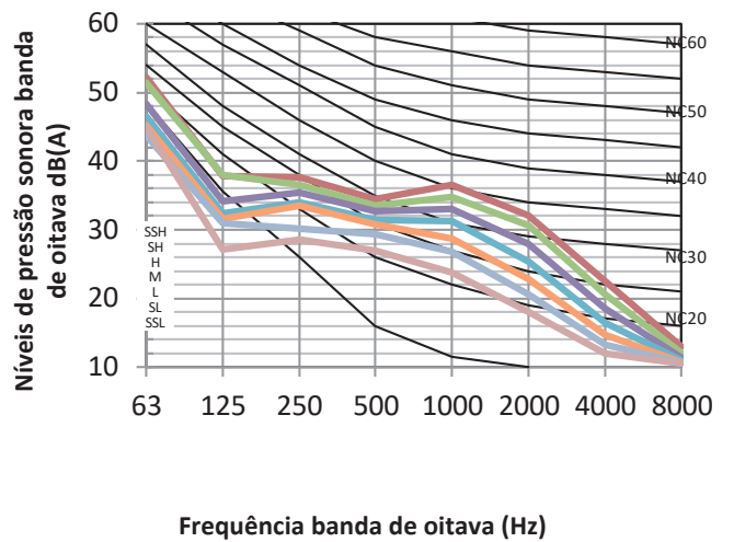
Figura 8.5: MIH36GHN18 níveis banda de oitava
