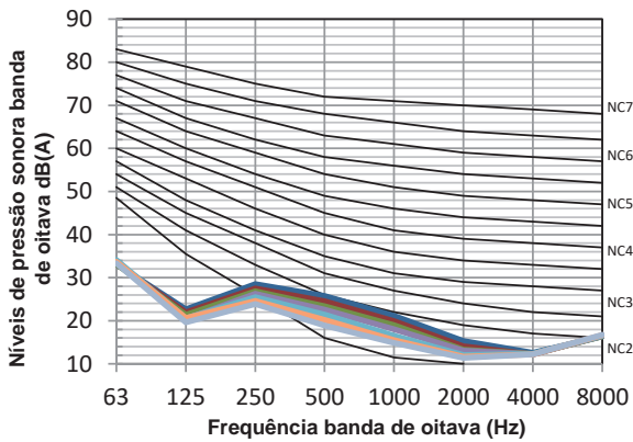
Figura 8.4: MIH28Q1DHN1(A) níveis banda de oitava
