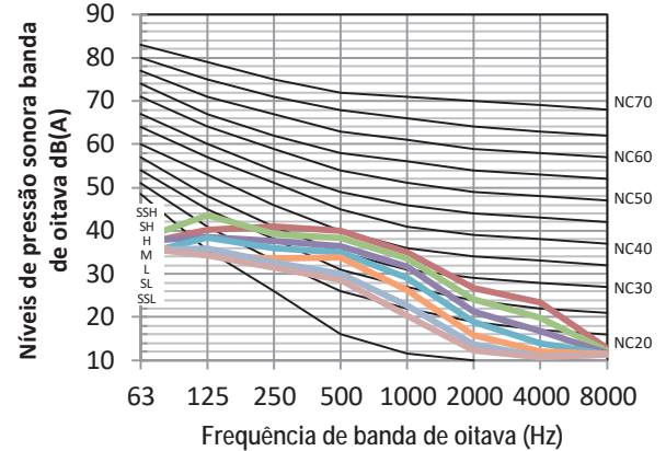
Figura 8.8: MIH63Q4CHN18 níveis banda de oitava
