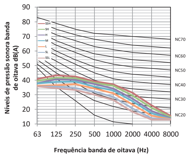
Figura 8.11: MIH112T3HN18 níveis banda de oitava
