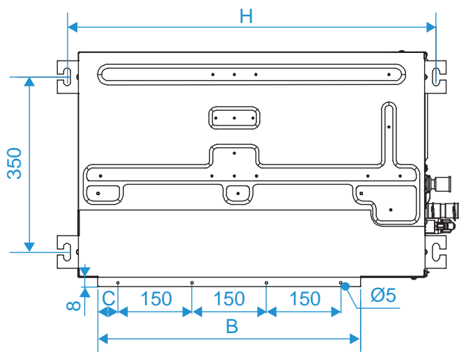
Figura 2.2: Dimensão da entrada de ar de retorno (modo de ar de retorno traseiro) (unidade: mm)
