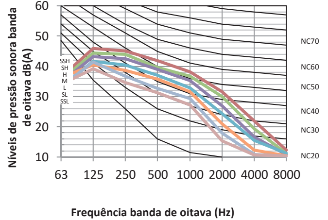
Figura 8.13: MIH180Q4HN18 níveis banda de oitava
