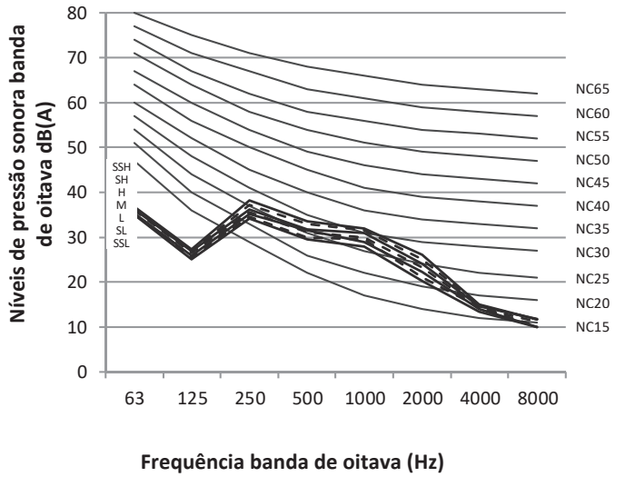
Figura 8.3: MIH-28(36)Q1DHN1 níveis banda de oitava
