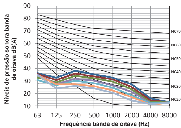
Figura 8.7: MIH56Q1DHN1(A) níveis banda de oitava
