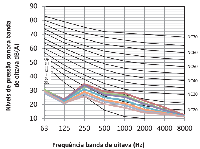
Figura 8.5: MIH71DLHN18 níveis banda de oitava
