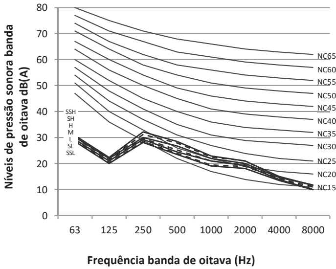
Figura 8.2: MIH-18(22)Q1DHN1 níveis banda de oitava
