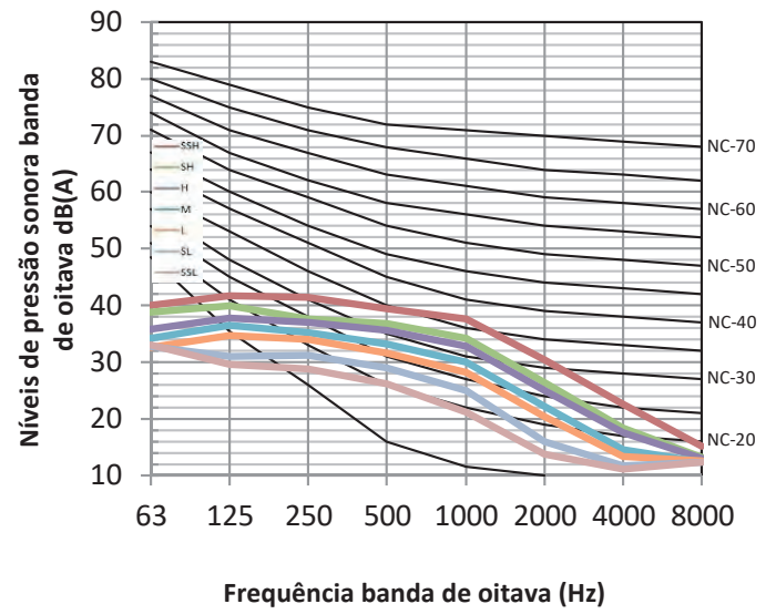
Figura 8.12: MIH112T2HN18 níveis banda de oitava
