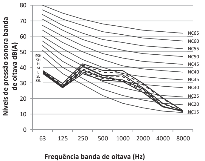
Figura 8.5: MIH-56Q1DHN1 níveis banda de oitava
