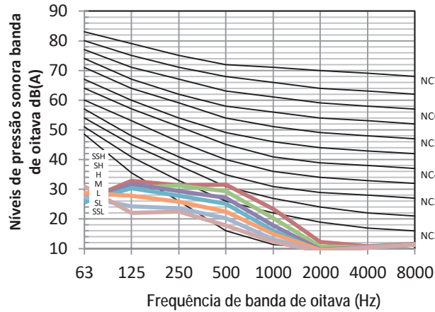
Figura 8.6: MIH45Q4CHN18 níveis banda de oitava
