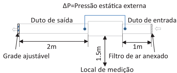
Figura 8.1: Medição do nível de pressão Sonora do Duto de Pressão Estática Média
