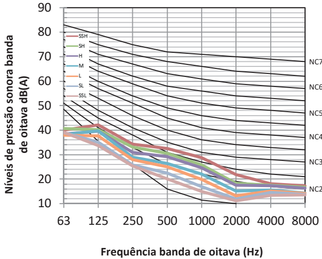
Figura 8.6: MIH45T3HN18 níveis banda de oitava
