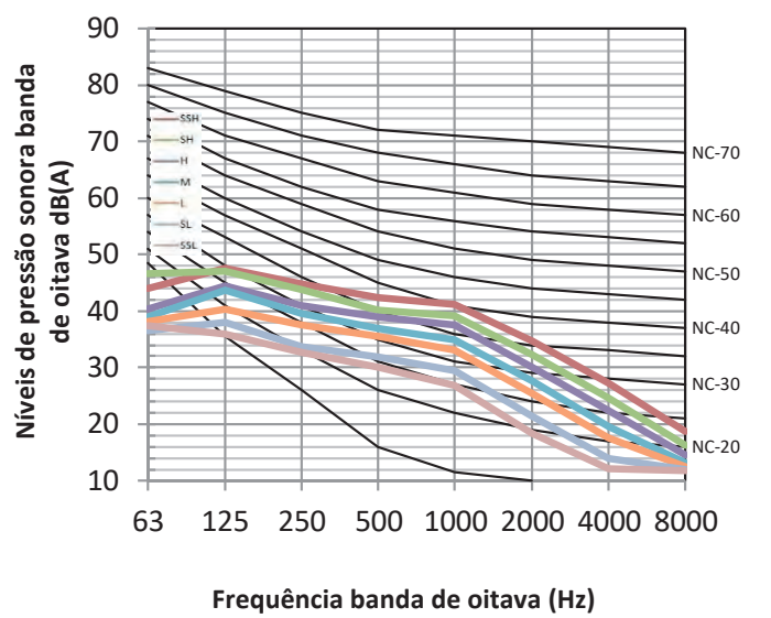
Figura 8.14: MIH160T2HN18 níveis banda de oitava
