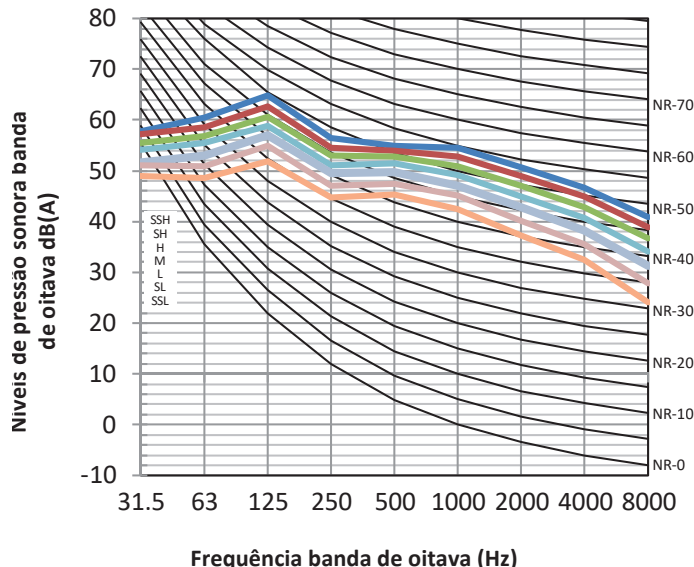
Figura 8.13: MIH400T1HN18 níveis banda de oitava
