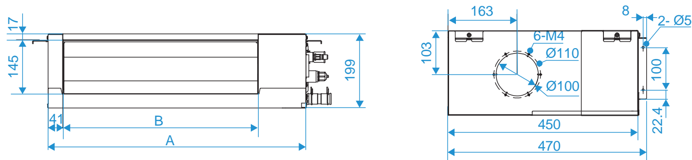
Figura 2.1: Dimensão externa da saída de ar e da saída de ar externo (unidade: mm)
