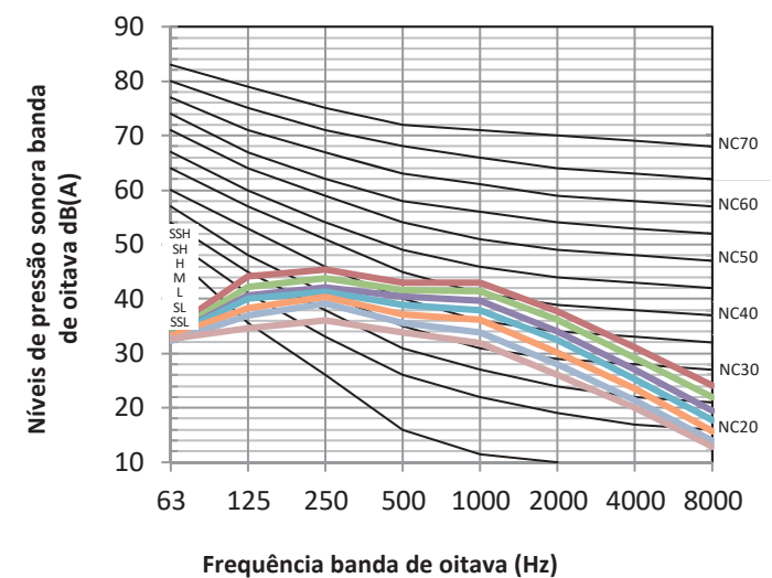
Figura 8.7: MIH90DLHN18 níveis banda de oitava
