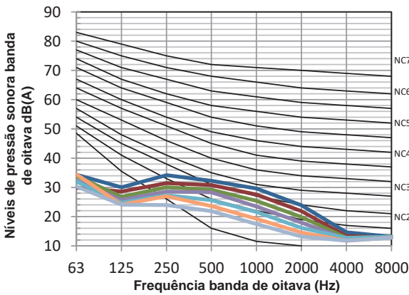
Figura 8.6: MIH45Q1DHN1(A) níveis banda de oitava
