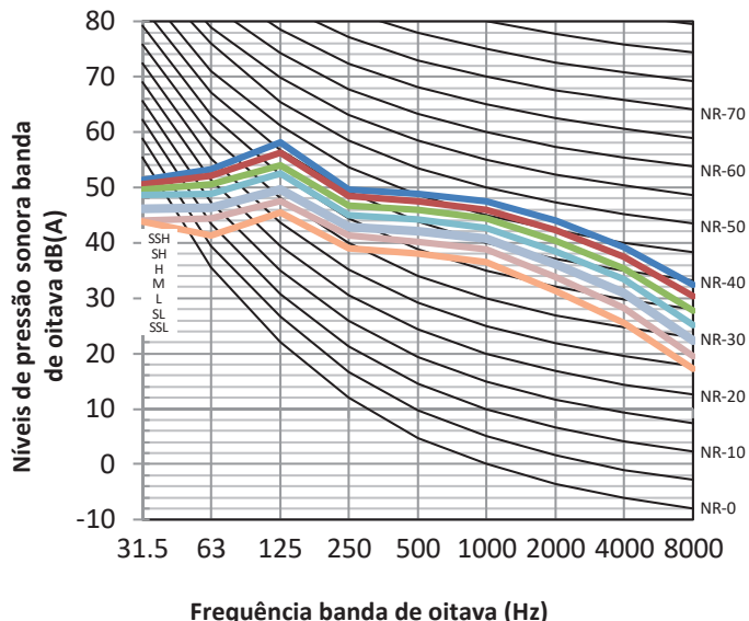
Figura 8.12: MIH335T1HN18 níveis banda de oitava
