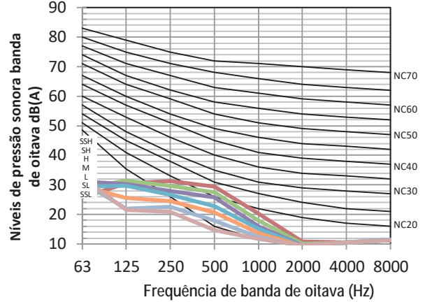
Figura 8.5: MIH36Q4CHN18 níveis banda de oitava
