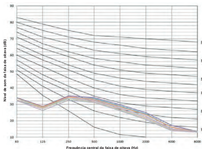
Figura 10.2: Níveis da faixa de oitava MIH22F3HN18
