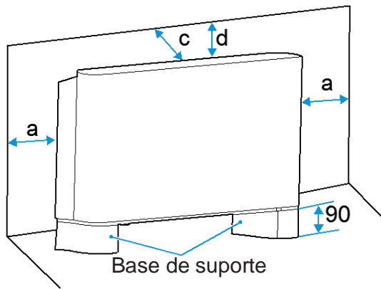
Figura 3.2: Requisitos de espaço de unidade de piso exposta da série F5 (entrada de ar por baixo) (unidade: mm)
