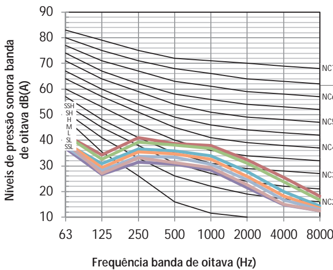
Figura 8.4: MIH56DLHN18 níveis banda de oitava
