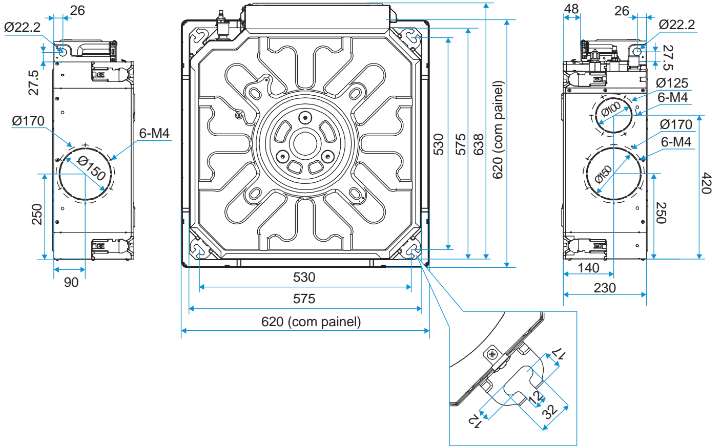
Figura 2.1: Dimensões do Cassete Quatro Vias Compacto (unidade: mm)
