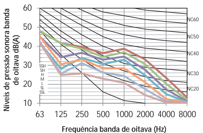
Figura 8.7: MIH56GHN18 níveis banda de oitava
