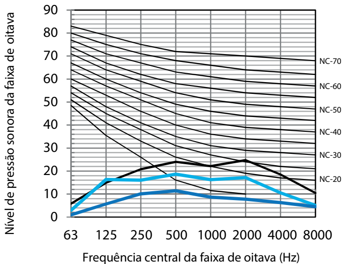
Figura 7.2: Níveis da faixa de oitava HRV-D200(C)
