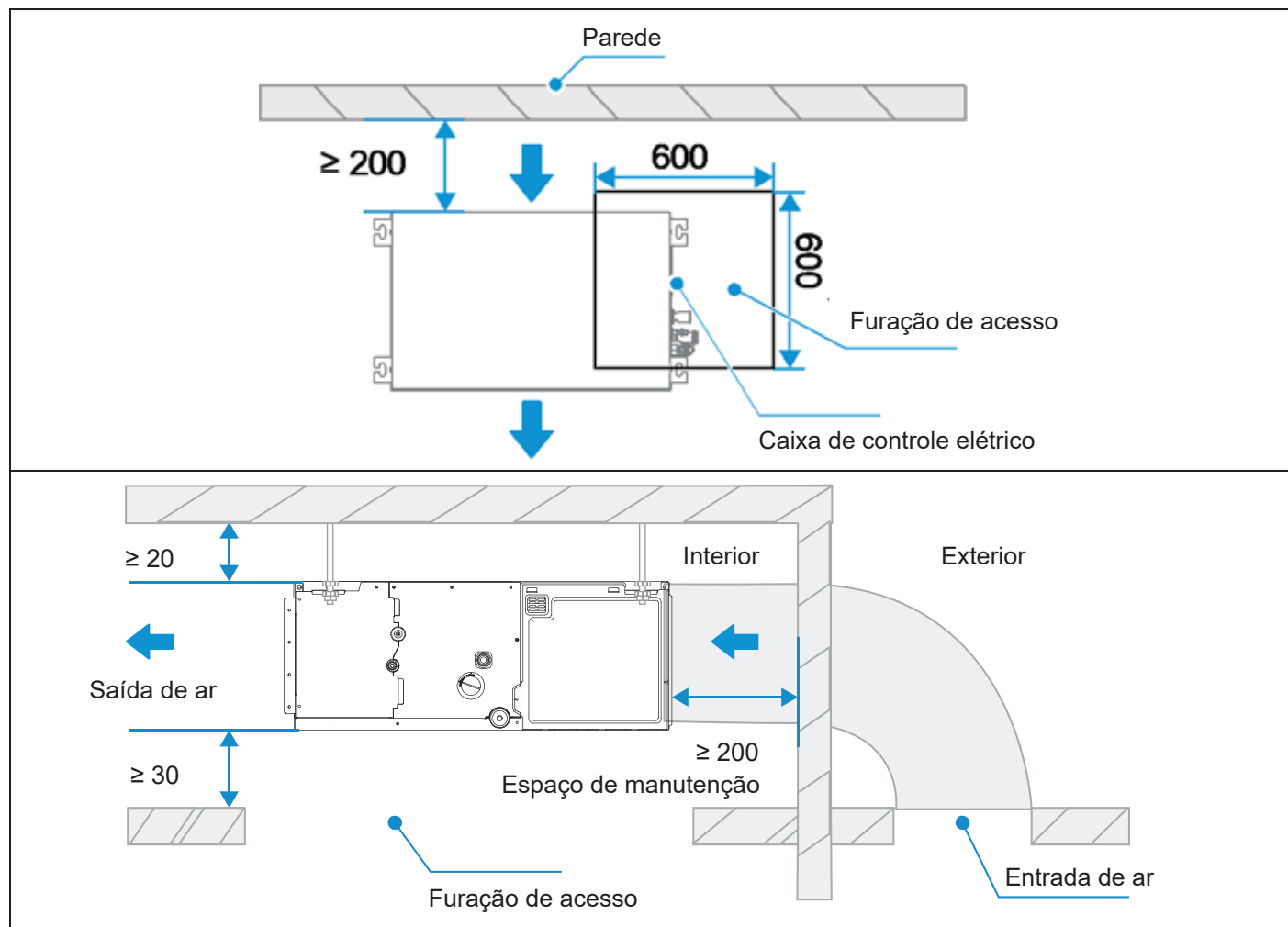
Figura 3.1: Requisitos de espaçamento da Unidade de Processamento de Ar Externo Small (unidade: mm)
