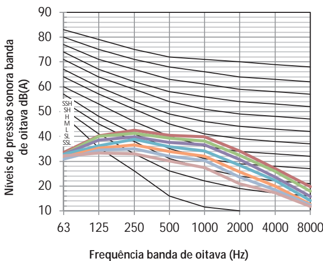
Figura 8.6: MIH80DLHN18 níveis banda de oitava
