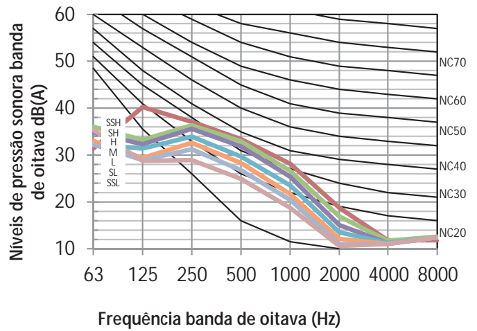
Figura 8.5: MIH56Q4HN18 níveis banda de oitava
