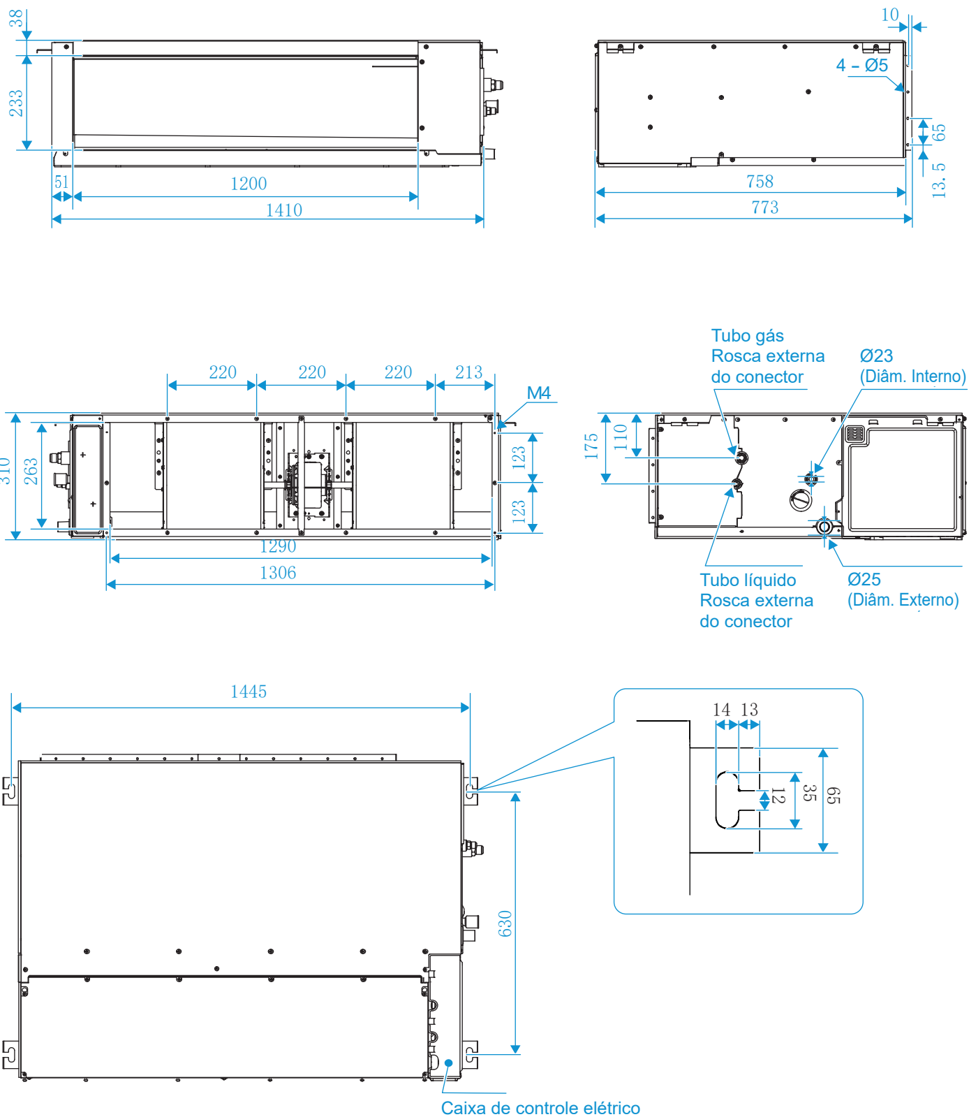
Figura 2.2: Dimensões modelos MIH224(280)FASHN18 (unidade: mm)
