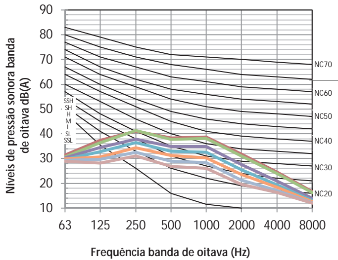
Figura 8.8: MIH100DLHN18 níveis banda de oitava
