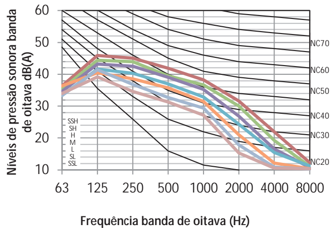
Figura 8.10: MIH112Q4HN18 níveis banda de oitava
