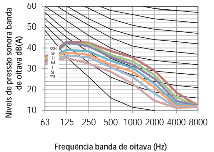
Figura 8.7: MIH80Q4HN18 níveis banda de oitava
