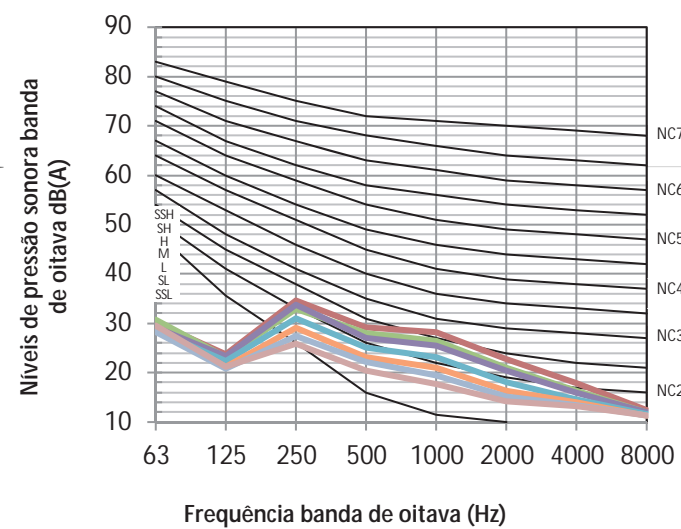
Figura 8.5: MIH71DLHN18 níveis banda de oitava
