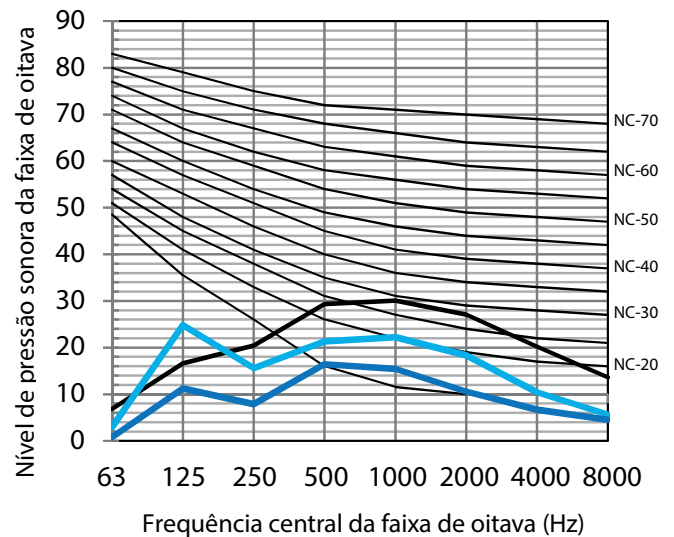
Figura 7.3: Níveis da faixa de oitava HRV-D300(C)
