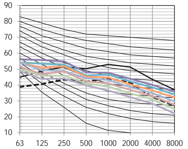
Figura 9.5: Níveis banda de oitava MIH335FAHN18
