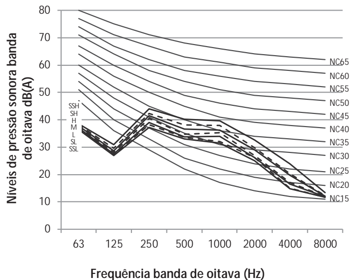
Figura 8.6: MIH-71Q1DHN1 níveis banda de oitava
