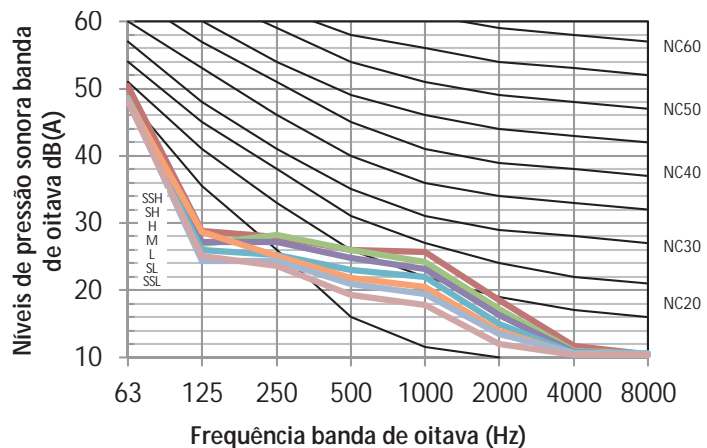
Figura 8.2: MIH15GHN18 níveis banda de oitava
