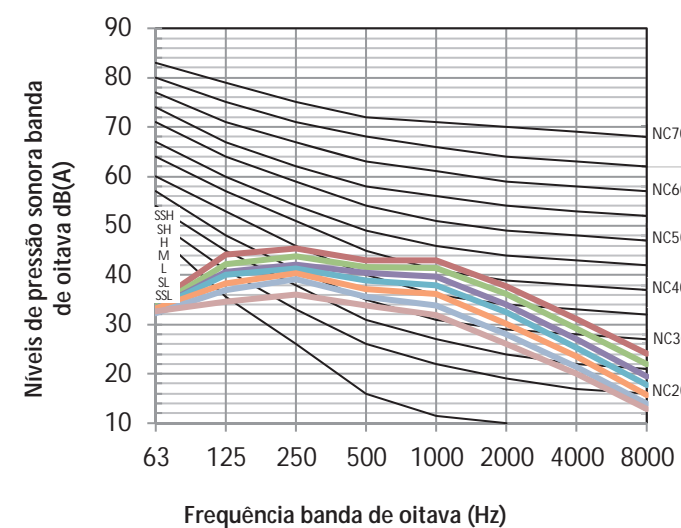
Figura 8.7: MIH90DLHN18 níveis banda de oitava
