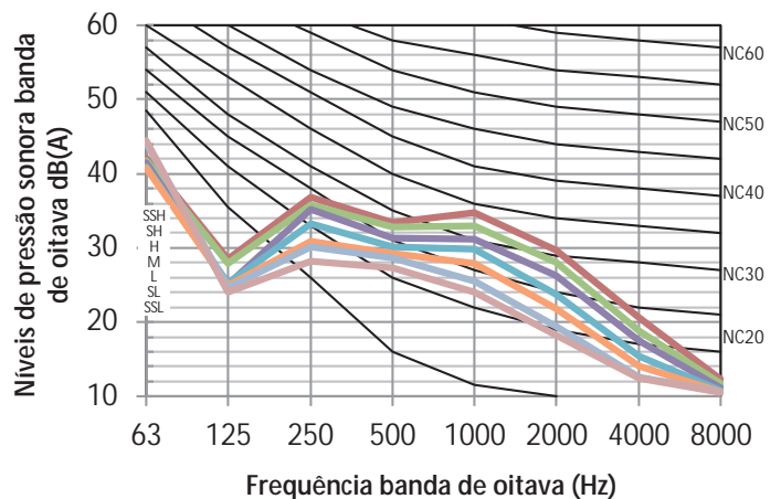
Figura 8.4: MIH28GHN18 níveis banda de oitava
