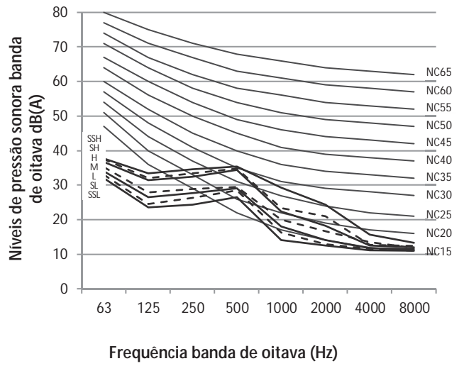
Figura 8.3: MIH-36Q2DHN1 níveis banda de oitava
