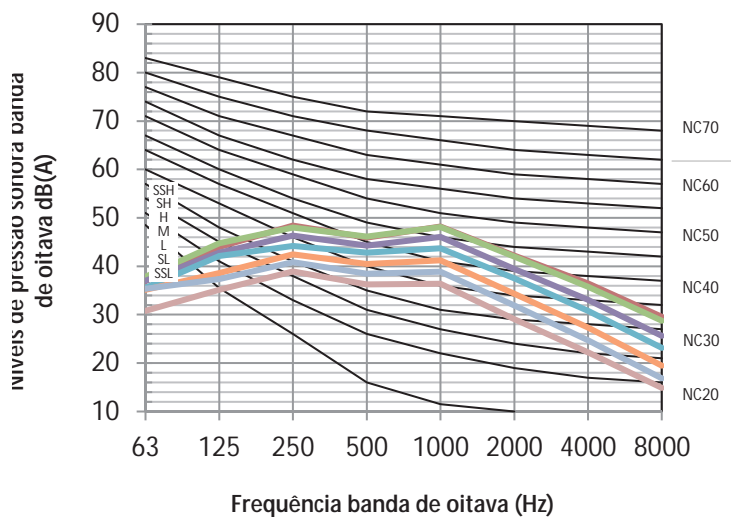
Figura 8.12: MIH160DLHN18 níveis banda de oitava
