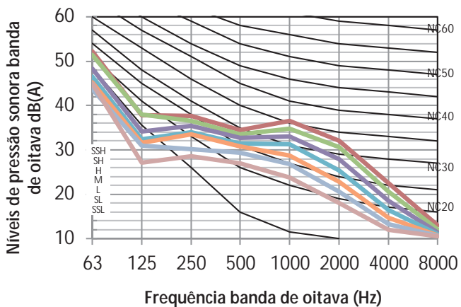
Figura 8.5: MIH36GHN18 níveis banda de oitava
