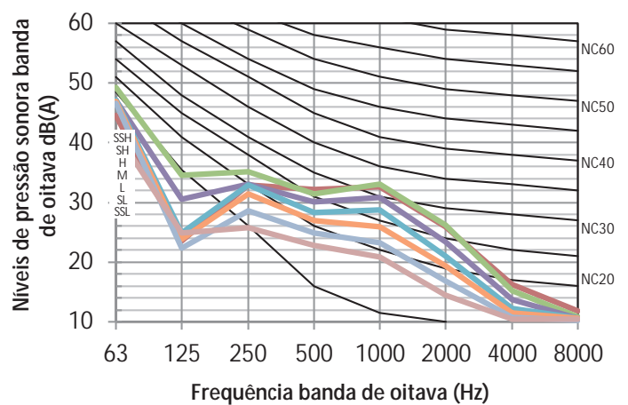
Figura 8.6: MIH45GHN18 níveis banda de oitava
