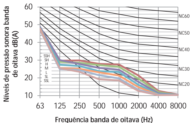
Figura 8.3: MIH22GHN18 níveis banda de oitava
