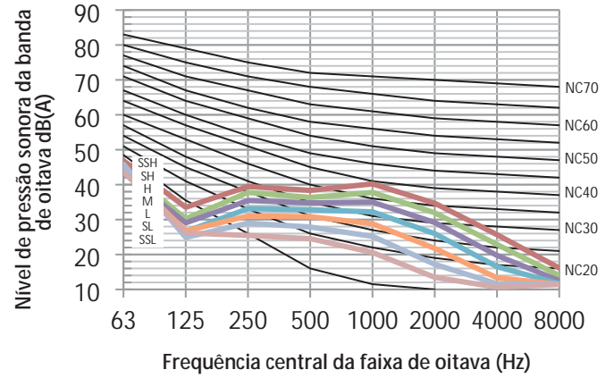
Figura 8.9: MIH80GHN18 níveis banda de oitava
