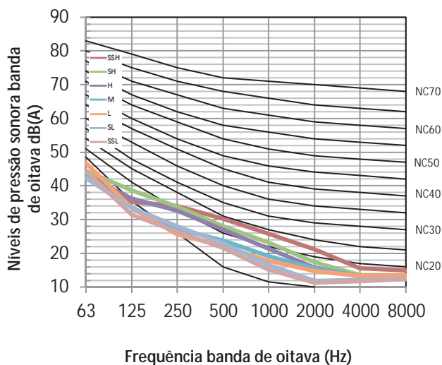
Figura 8.5: MIH36T3HN18 níveis banda de oitava
