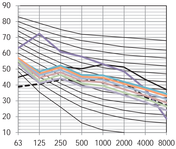
Figura 9.4: Níveis banda de oitava MIH280FAHN18
