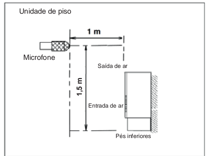
Figura 10.1: Medição dos níveis de pressão sonora da unidade de piso
