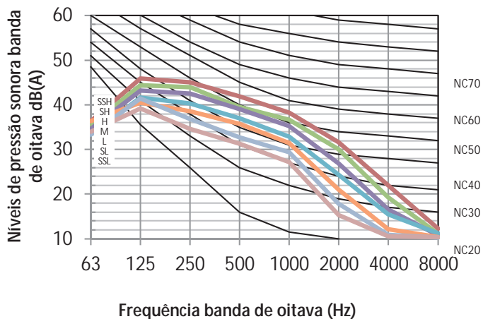
Figura 8.12: MIH160Q4HN18 níveis banda de oitava
