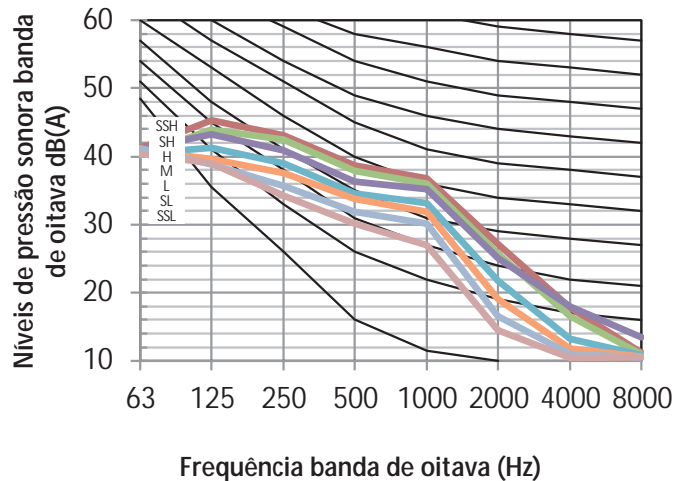
Figura 8.9: MIH100Q4HN18 níveis banda de oitava
