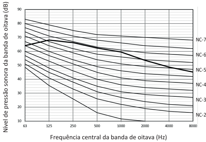
Figura 2-9.10 Nível da banda de oitava de 24HP
