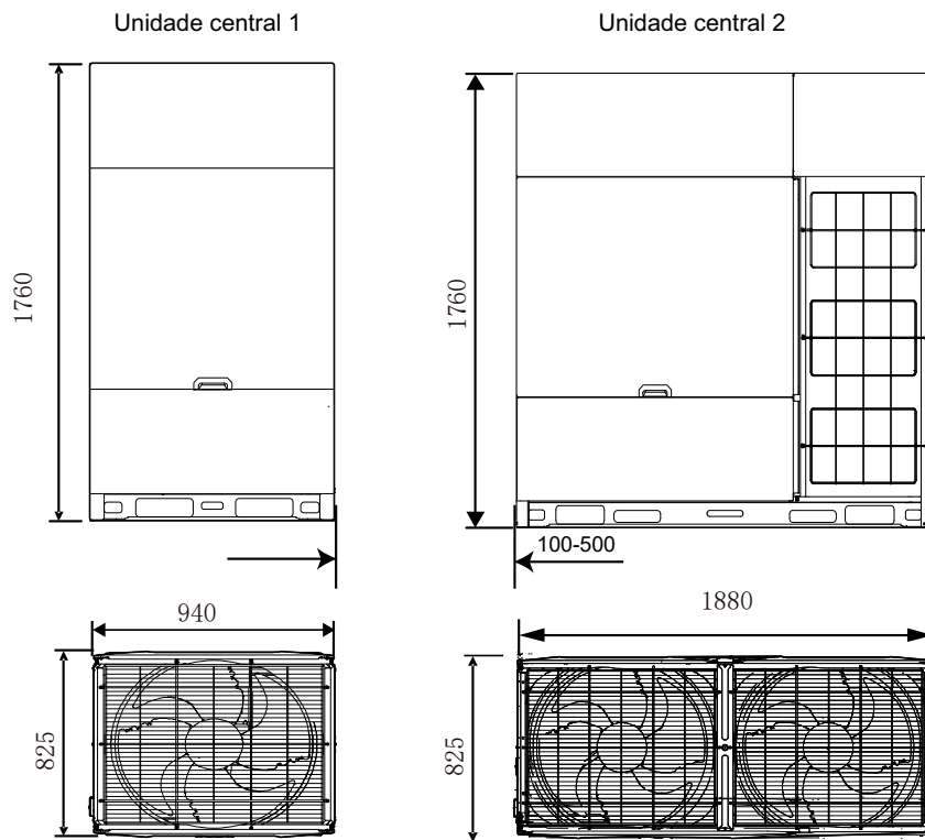
Figura 2-2.7: Dimensões da unidade 42/44HP (dimensões em mm)
