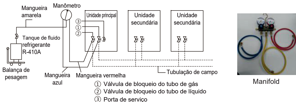
Figura 3-8.1: Carregamento do refrigerante
