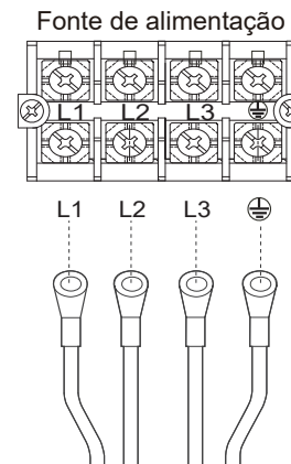
Figura 3-9.4: Terminais da fonte de alimentação trifásica da unidade central
