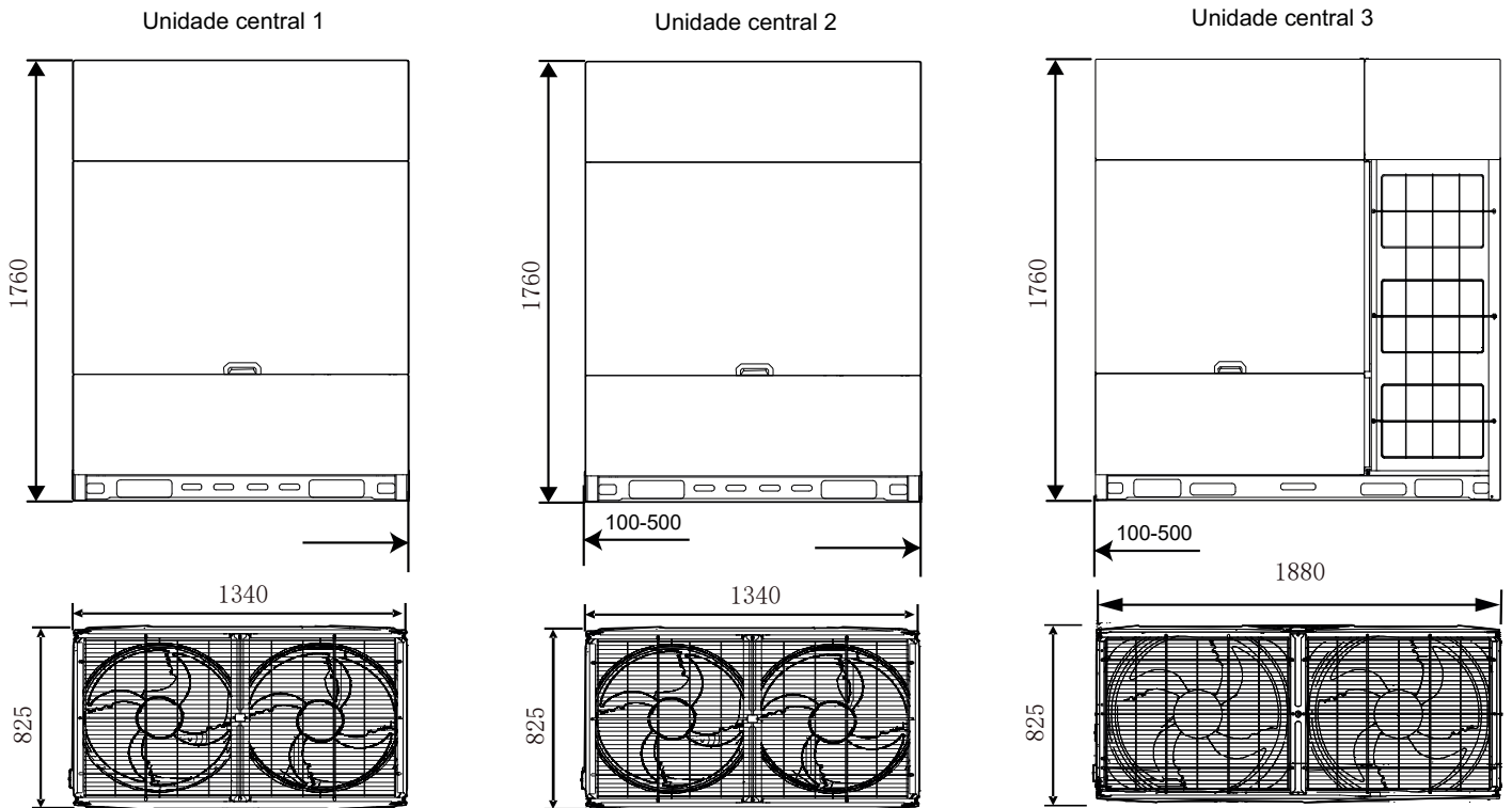
Figura 2-2.14: Dimensões das unidades 74/76HP (dimensões em mm)
