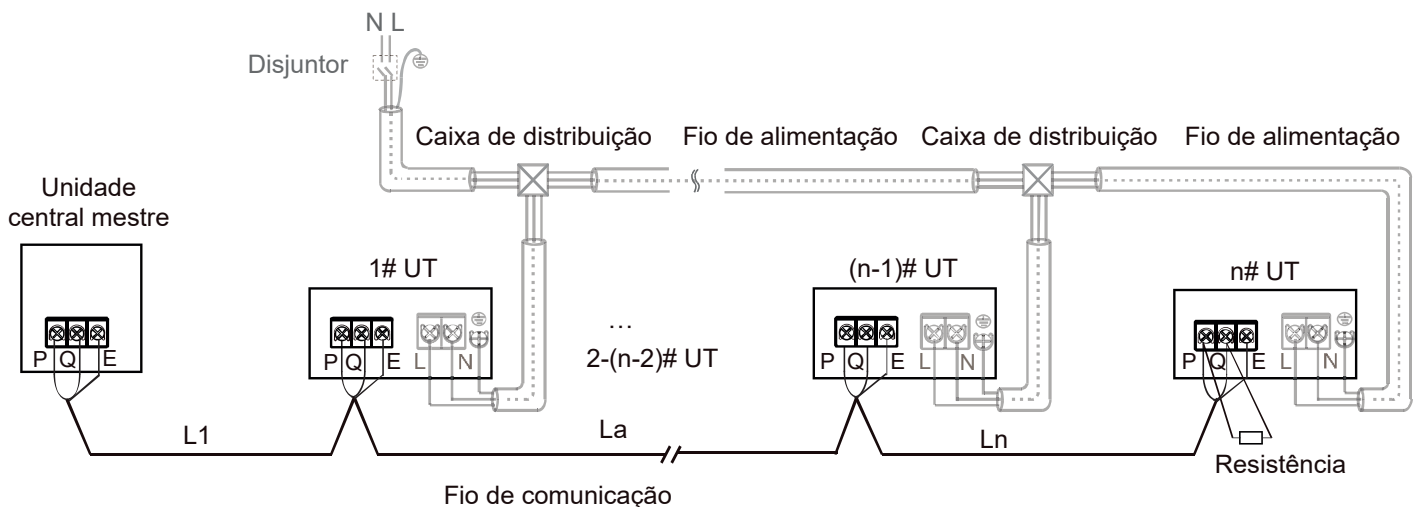
Figura 3-9.7: Configuração da fiação de comunicação P Q E - alimentação unificada de UTs
