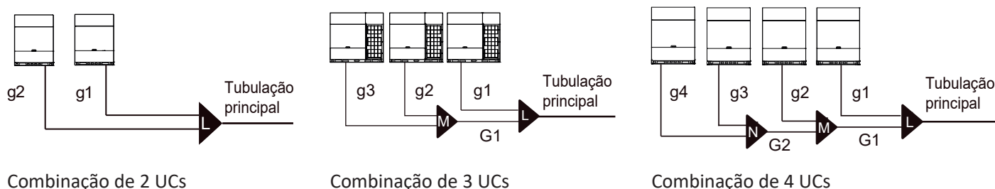
Figura 3-4.4: Conexões das tubulações das unidades centrais
