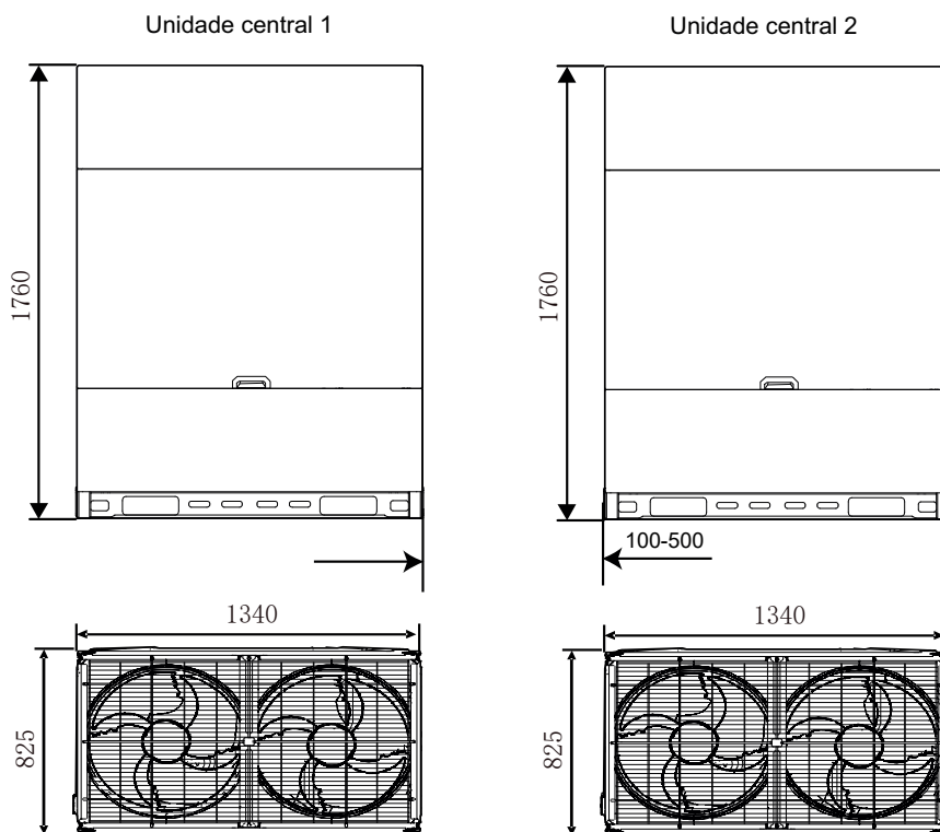
Figura 2-2.8: Dimensões das unidades 46/48HP (dimensões em mm)
