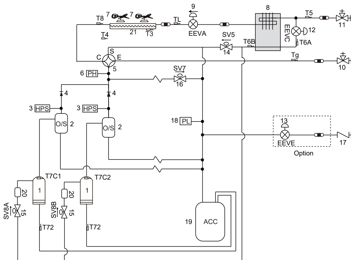
Figura 2-3.2: Diagramas de tubulação 20-24HP
