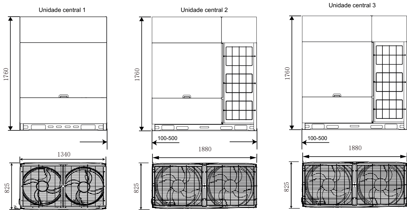
Figura 2-2.15: Dimensões da unidade 78/80HP (dimensões em mm)
