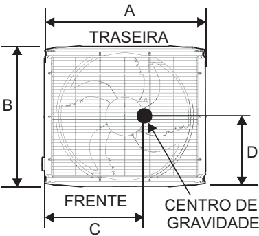
Figura 3-2.9: Centro de gravidade 20-40HP
