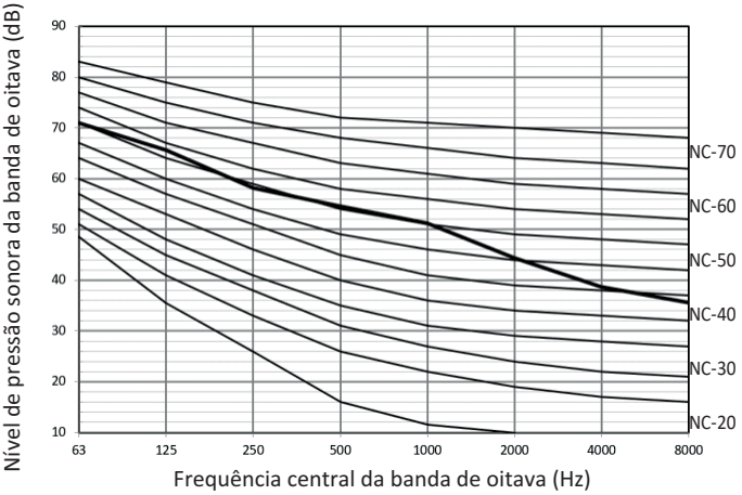
Figura 2-9.3 Nível da banda de oitava de 10HP
