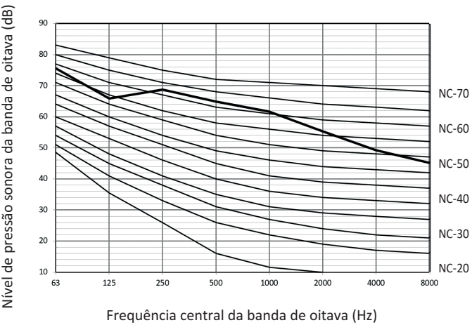
Figura 2-9.15 Nível da banda de oitava de 34HP
