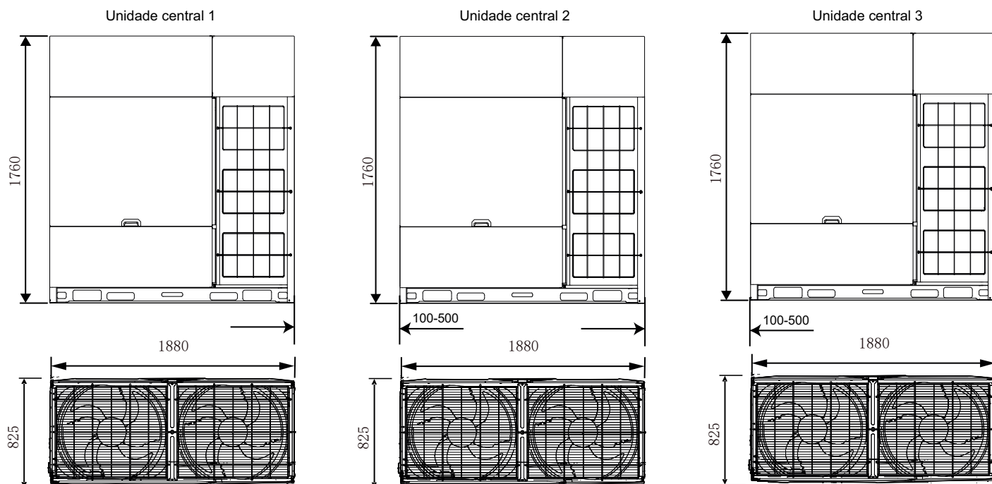
Figura 2-2.13: Dimensões da unidade 100/104/106/108/110/112/114/116/118/120HP (dimensões em mm)
