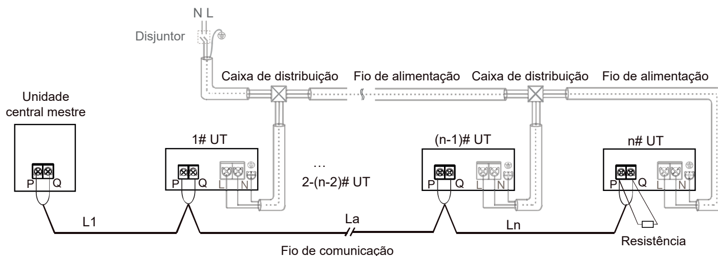
Figura 3-9.8: Configuração da fiação de comunicação P Q - alimentação unificada de UTs
