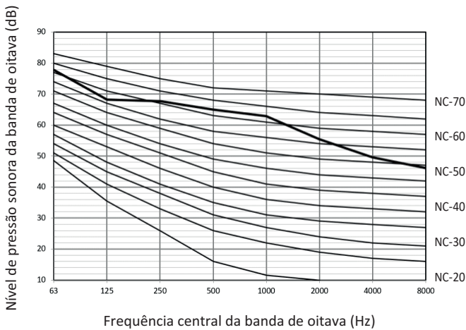
Figura 2-9.16 Nível da banda de oitava de 36HP
