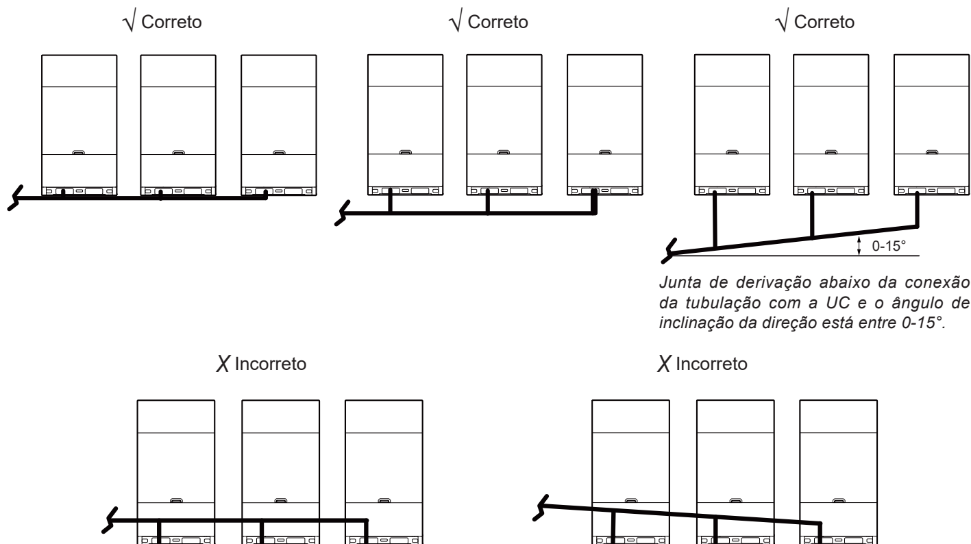
Figura 3-5.10: Conexões de tubulação entre as unidades centrais
