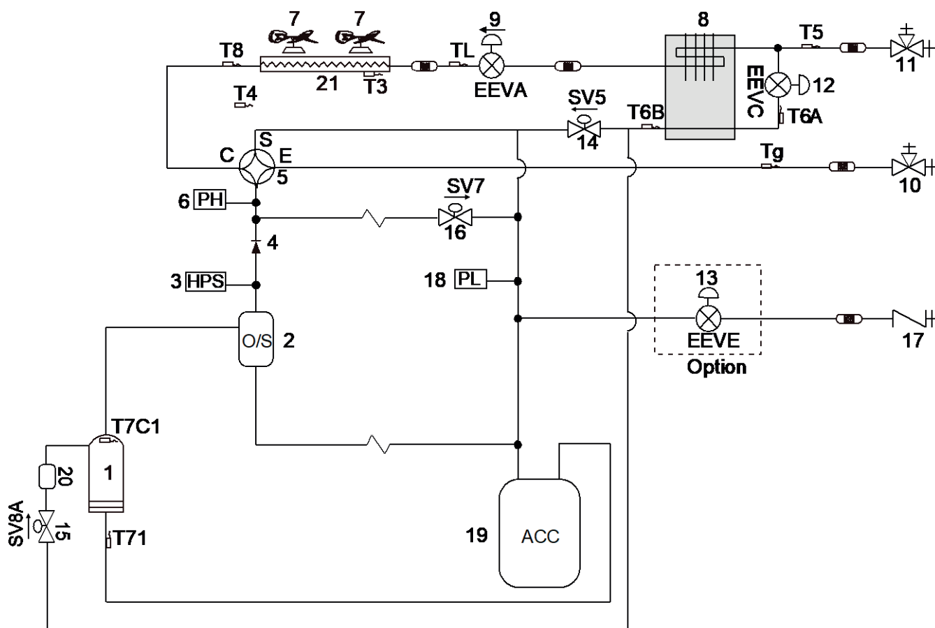
Figura 2-3.2: Diagramas de tubulação 20-24HP
