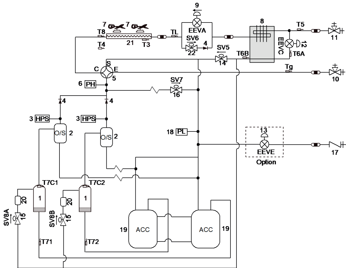
Figura 2-3.3: Diagramas de tubulação 26-36HP
