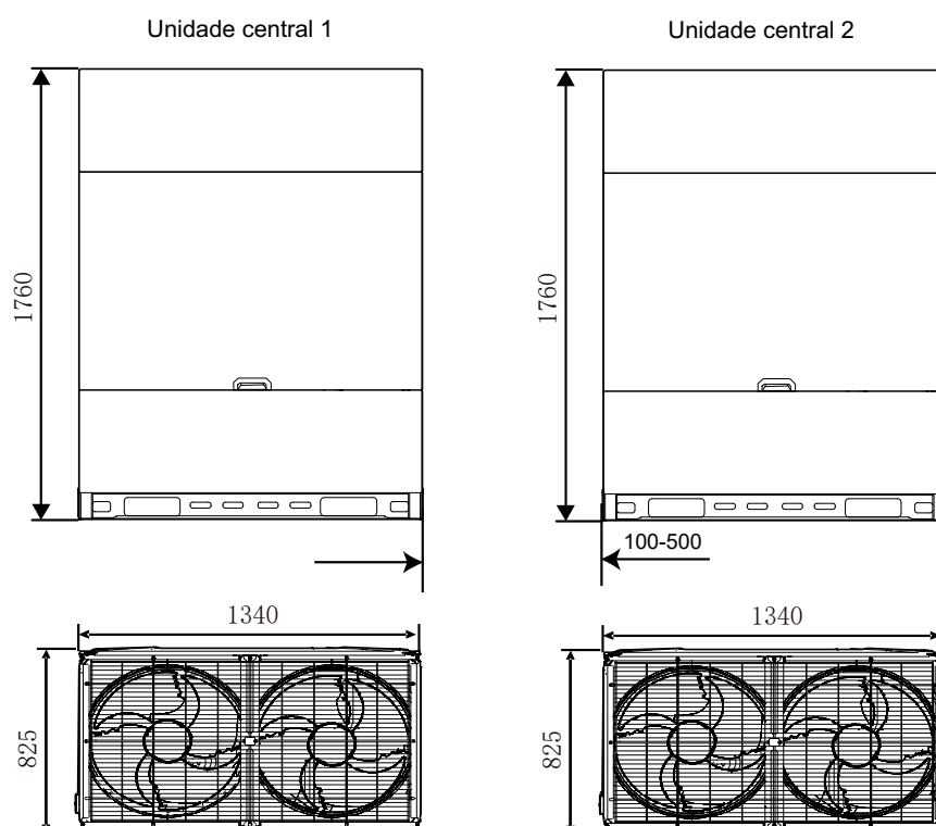
Figura 2-2.6: Dimensões das unidades 44/46/48HP (dimensões em mm)
