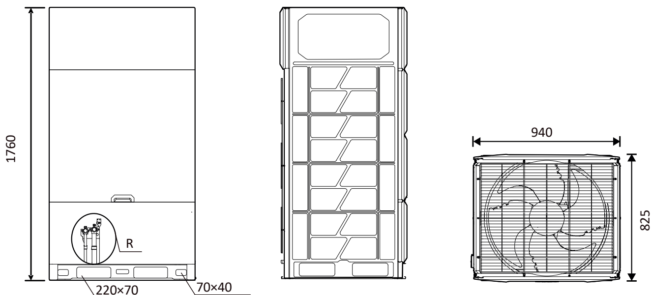
Figura 2-2.1: Dimensões 8/10/12/14/16/18HP (dimensões em mm)
