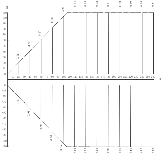
Figura 2-7.2: Taxa de mudança na capacidade de aquecimento
