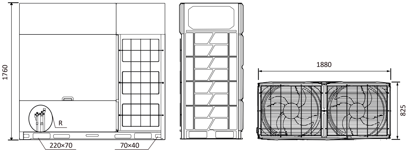
Figura 2-2.3: Dimensões 26/28/30/32/34/36/38/40HP (dimensões em mm)
