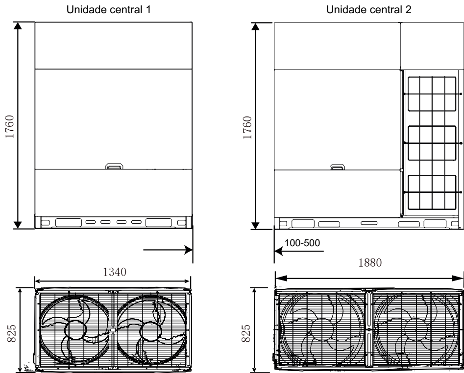
Figura 2-2.8: Dimensões das unidades 54/58/60/62/64HP (dimensões em mm)
