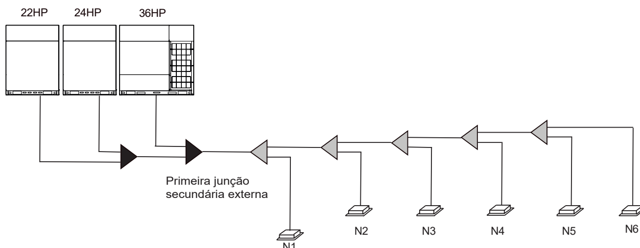
Figura 3-2.4: Posicionamento das unidades centrais mestre & auxiliar
