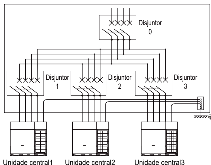
Figura 3-9.2: Fiação da fonte de alimentação da unidade central
