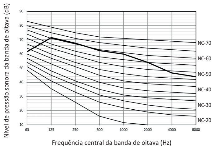
Figura 2-9.8 Nível da banda de oitava de 20HP
