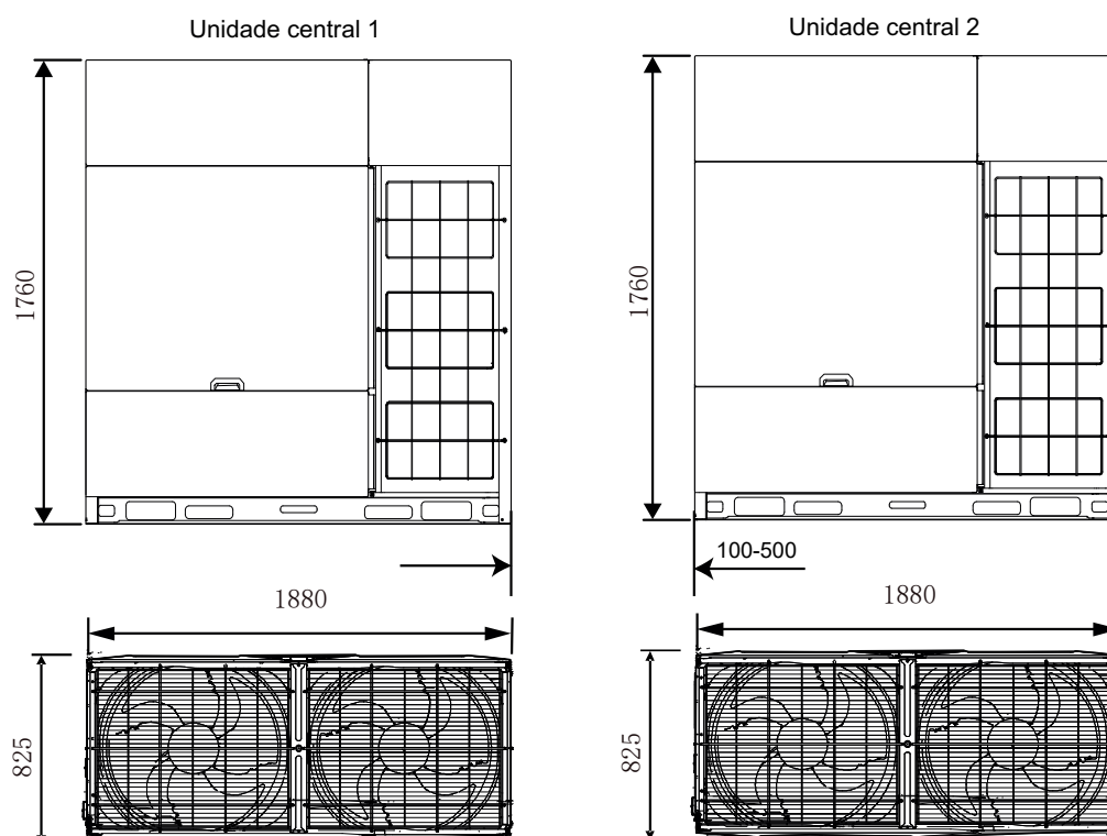
Figura 2-2.9: Dimensões das unidades 66/68/70/72/74/76/78/80HP (dimensões em mm)
