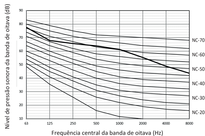
Figura 2-9.12 Nível da banda de oitava de 28HP
