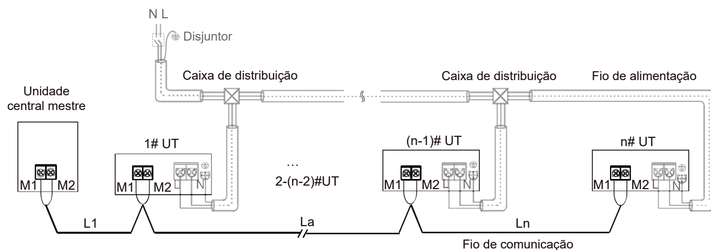
Figura 3-9.9: Configuração da fiação de comunicação M1 M2 - alimentação unificada de UTs
