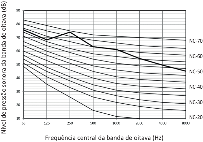
Figura 2-9.14 Nível da banda de oitava de 32HP
