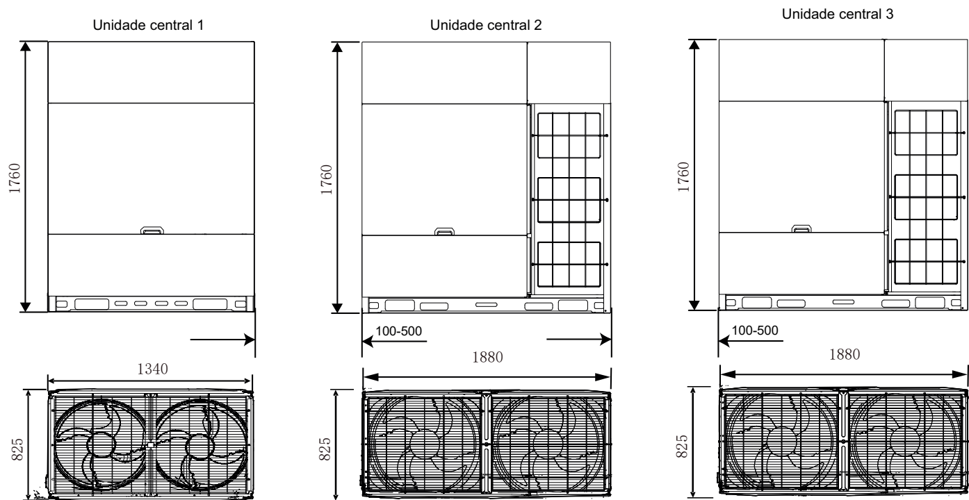
Figura 2-2.12: Dimensões das unidades 92/94/96/98/102HP (dimensões em mm)
