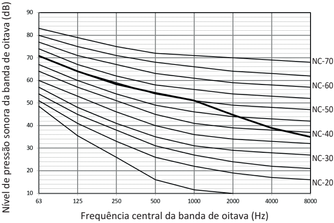
Figura 2-9.2 Nível da banda de oitava de 8HP
