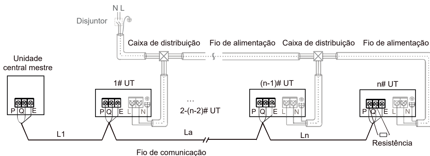
Figura 3-9.7: Configuração da fiação de comunicação P Q E - alimentação unificada de UTs
