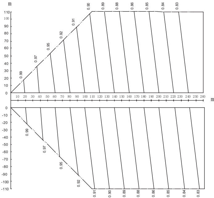
Figura 2-7.1: Taxa de mudança na capacidade de resfriamento
