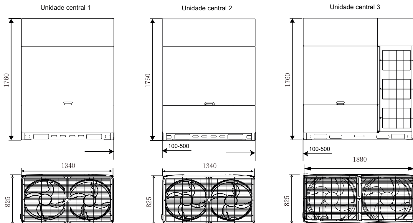
Figura 2-2.10: Dimensões das unidades 82/84/86/88HP (dimensões em mm)
