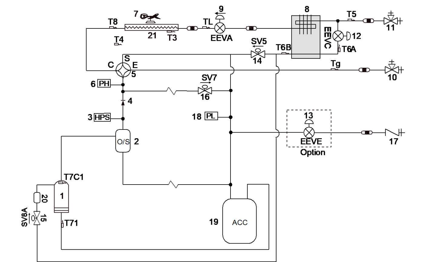
Figura 2-3.1: Diagramas de tubulação 8-18HP
