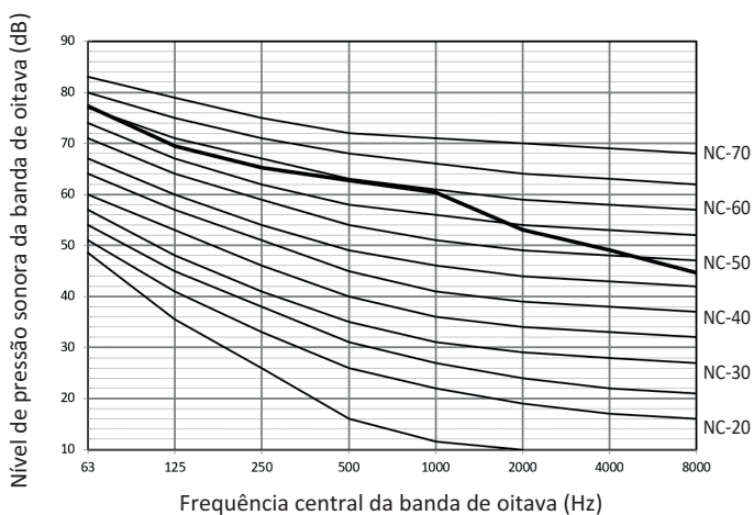
Figura 2-9.13 Nível da banda de oitava de 30HP
