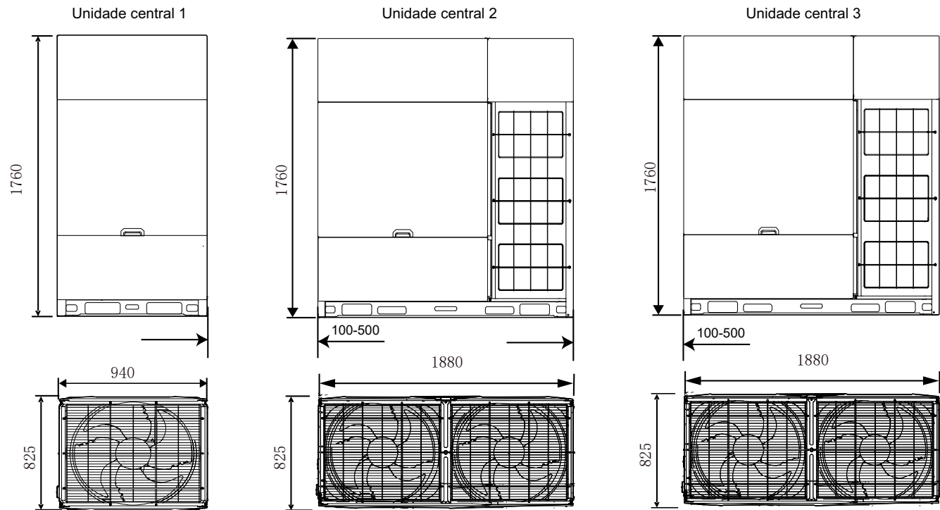
Figura 2-2.11: Dimensões da unidade 90HP (dimensões em mm)
