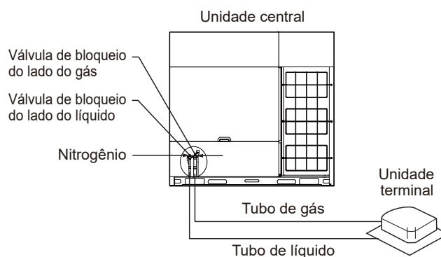
Figura 3-5.13: Teste de estanqueidade
