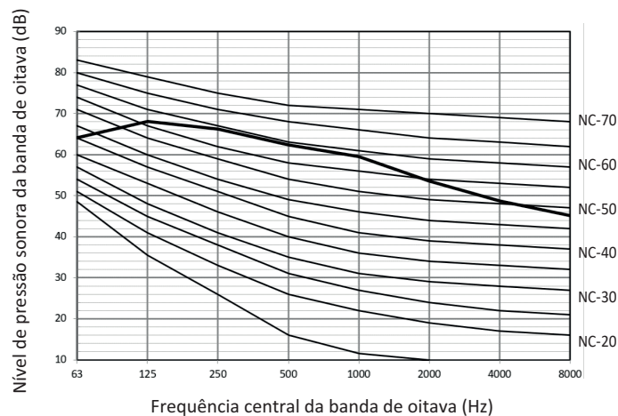
Figura 2-9.10 Nível da banda de oitava de 24HP
