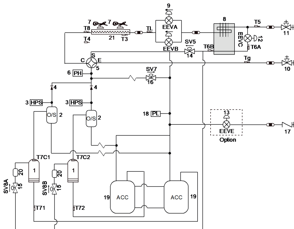
Figura 2-3.4: Diagramas de tubulação 38-40HP
