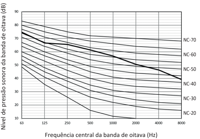
Figura 2-9.6 Nível da banda de oitava de 16HP
