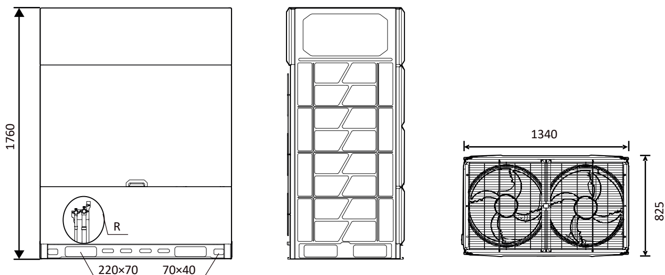
Figura 2-2.2: Dimensões 20/22/24HP (dimensões em mm)
