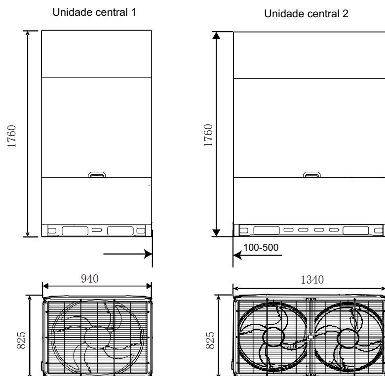
Figura 2-2.5: Dimensões da unidade 42HP (dimensões em mm)
