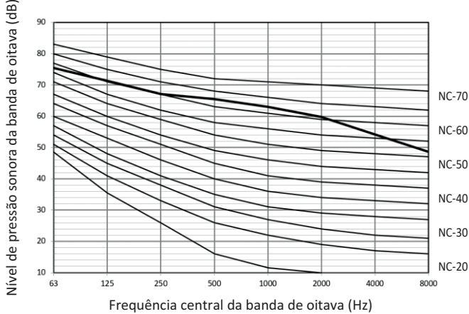
Figura 2-9.18 Nível da banda de oitava de 40HP
