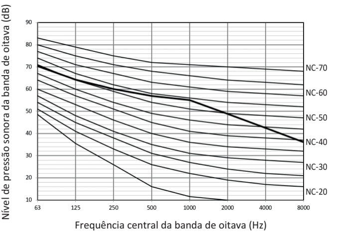
Figura 2-9.4 Nível da banda de oitava de 12HP
