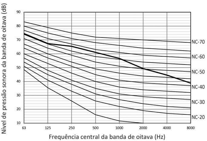
Figura 2-9.5 Nível da banda de oitava de 14HP
