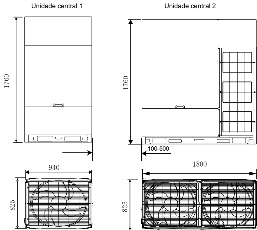
Figura 2-2.7: Dimensões da unidade 50/52/56HP (dimensões em mm)
