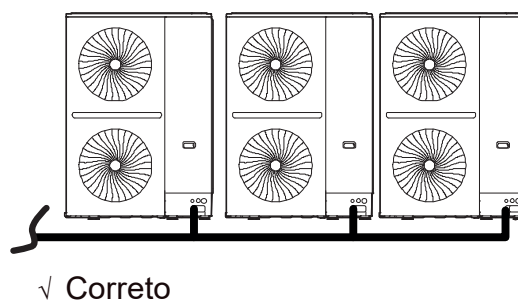
Figura 3-5.13: Conexões de tubulação entre unidades centrais
