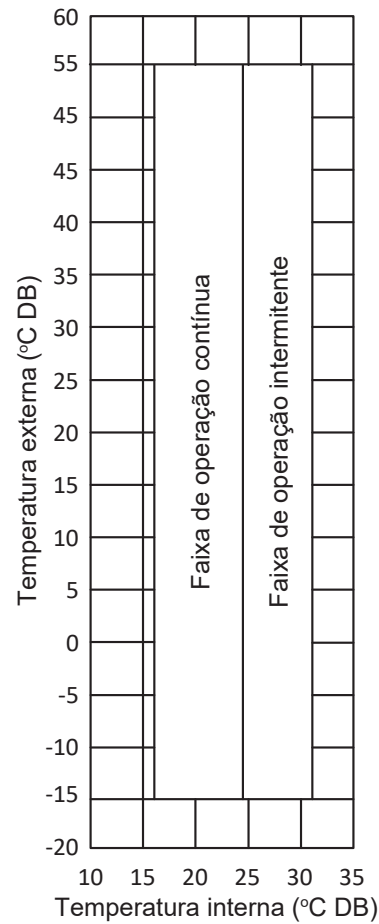
Figura 2-9.1: Limites de operação de resfriamento
