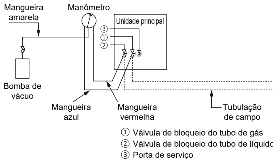
Figura 3-4.14: Secagem a vácuo
