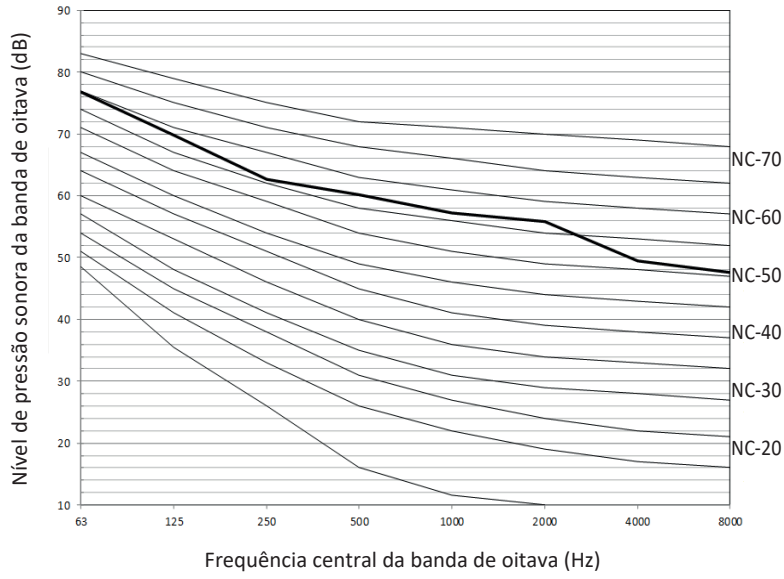
Figura 2-10.3 Nível da banda de oitava de 10HP
