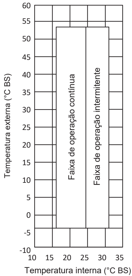
Figura 2-9.1: Limites de operação de resfriamento
