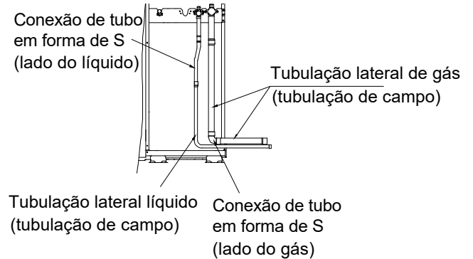
Figura 3-4.15: Método de conexão do tubo de saída para baixo.
